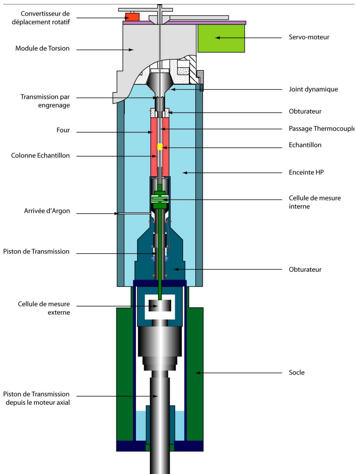
Figure II.10 : Schéma de l'intérieur d'une presse Paterson avec module de torsion (d'après Champallier, 2005)
