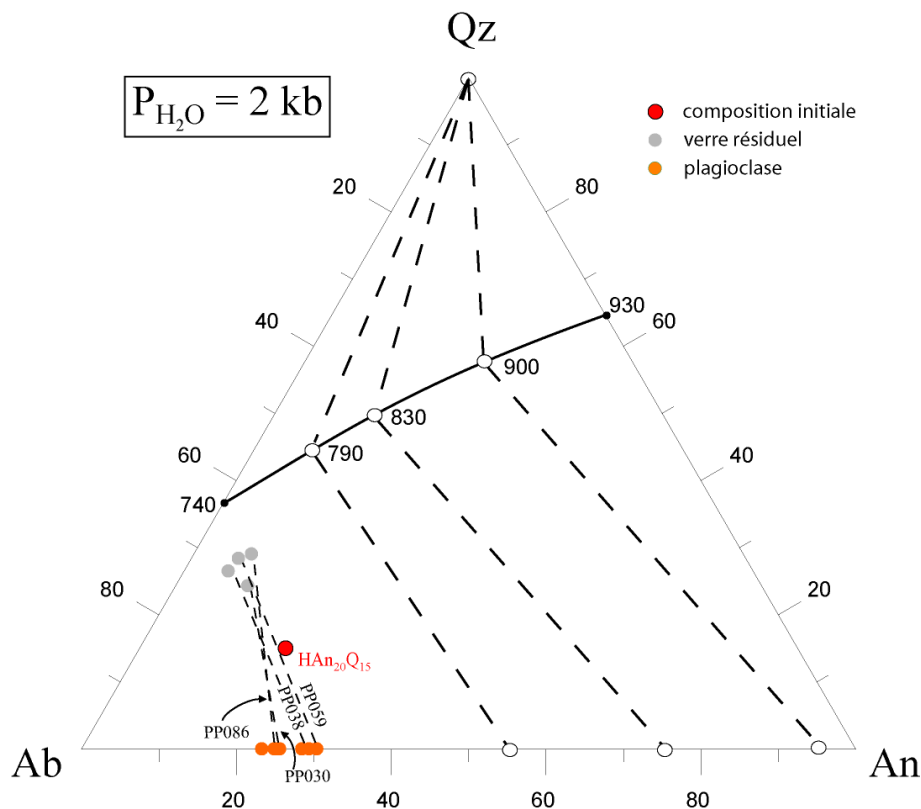
Figure V.21 : Compositions chimiques du verre résiduel et des plagioclases reportées dans un diagramme ternaire Qz-Ab-An. La courbe cotectique (en noir) et les compositions des phases coexistantes sont indiquées pour P_{H_2O} = 2 \text{ kbar} (Johannes et Holtz, 1996). Les lignes pointillées relient les phases coexistantes (indiquées par les cercles) pour des températures de 790, 830 et 900°C. Les points noirs représentent les points eutectiques pour le système binaire Qz-An et Qz-Ab. La composition de départ HAn_{20}Q_{15} est indiquée par un rond rouge. Les compositions chimiques des verres résiduels sont indiquées par des ronds gris. Les compositions des plagioclases après déformation sont indiquées en orange.
