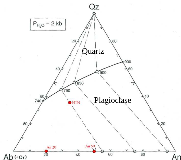
Figure III.1 : Compositions de départ potentielles reportées dans un diagramme ternaire Qz-Ab-An. La courbe cotectique (en noir) et les compositions des phases coexistantes sont indiquées pour P_{H_2O} = 2 \text{ kbar} (Johannes et Holtz, 1996). Les lignes pointillées relient les phases coexistantes (indiquées par les cercles) pour des températures de 790°, 830° et 900°C. Les points noirs représentent les points eutectiques pour le système binaire Qz-An et Qz-Ab. Les compositions de départ potentielles sont indiquées par un rond rouge.
