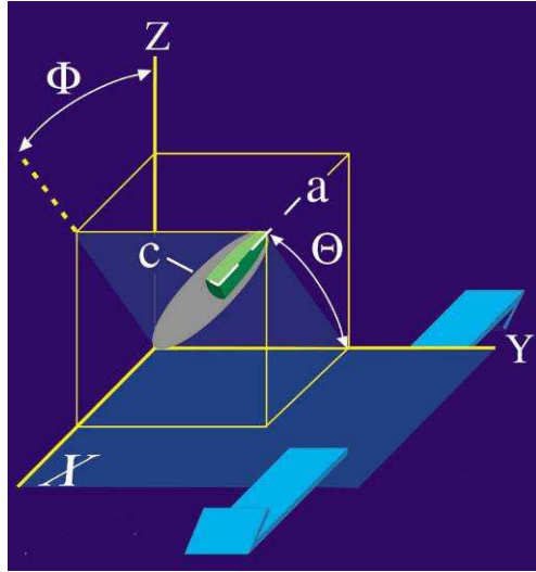
Figure I.10 : Représentation du modèle de Jeffery (1922) . A droite, équations du modèle décrivant le comportement d'une particule ellipsoïdale soumise à un cisaillement simple homogène dans un fluide visqueux. A gauche, représentation schématisée des paramètres géométriques décrivant la position de la particule (azimuts, plongement, référentiel, sens de cisaillement) (d'après Arbaret et al., 2000 ).
