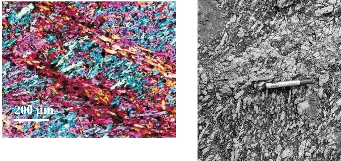
Figure I.17 : Illustration de structures magmatiques. A gauche, organisation structurale de feldspath dans une coulée trachytique (Smith., 2002). A droite, bande de cisaillement marquée par l'orientation des phénocristaux de feldspath potassique au sein d'un granite (Sen et Mamtani., 2006).
