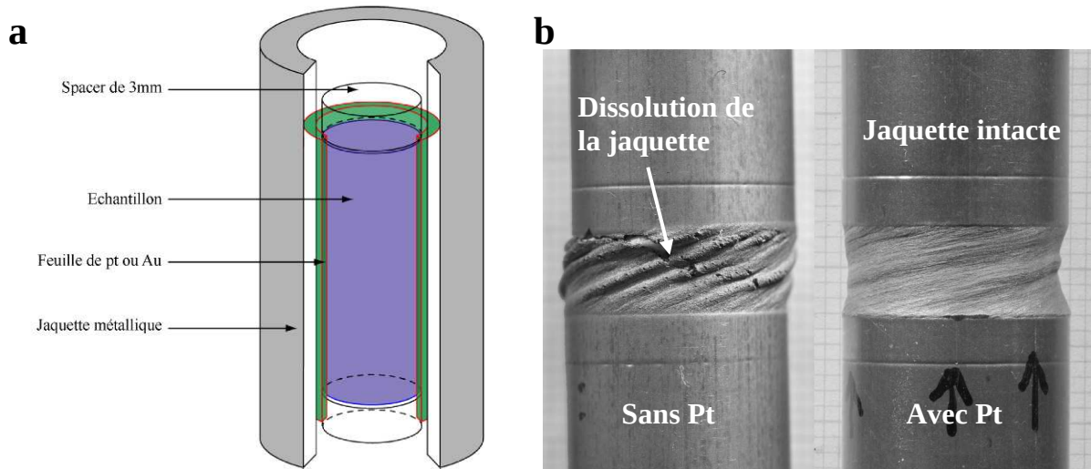
Figure II.6 : Agencement et effet d'une feuille de métal inerté autour de l'échantillon. (a) Arrangement respectif de l'échantillon, de la jaquette et de la feuille de métal (ici du platine) servant à protéger la jaquette de l'interaction avec l'échantillon. (b) Etat de l'échantillon après expérience de déformation sans feuille de platine (à gauche) et avec feuille de platine (à droite) (modifié d'après Champallier (2005) ).
