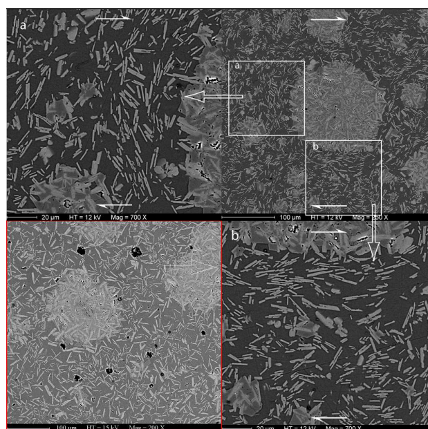
Figure III.3 : Enroulement de plagioclases autour d'un agglomérat de grains de quartz. Etudes menées à 3 kbar, 775°C. L'image en bas à gauche encadrée de rouge représente l'équivalent non déformé. ( Champallier, 2005 ).
