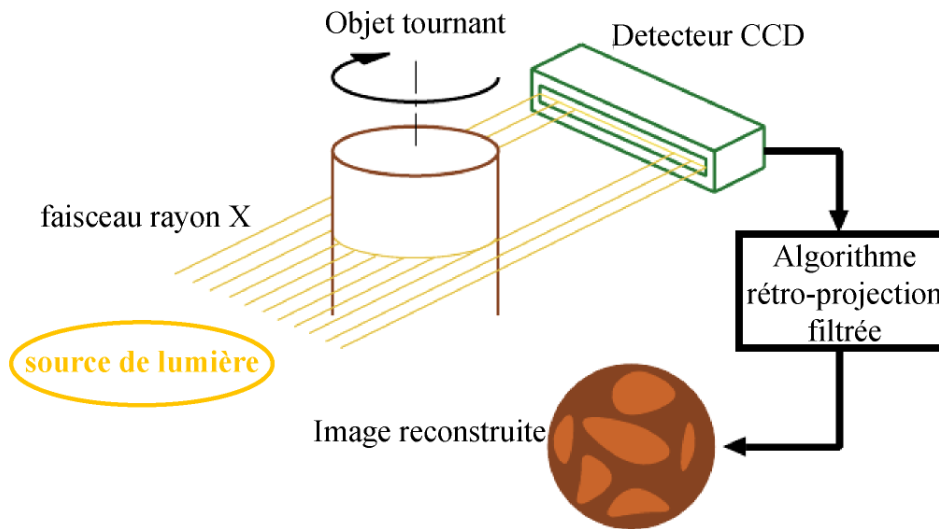
Figure II.34 : Représentation schématique du principe de microtomographie à rayon X.
