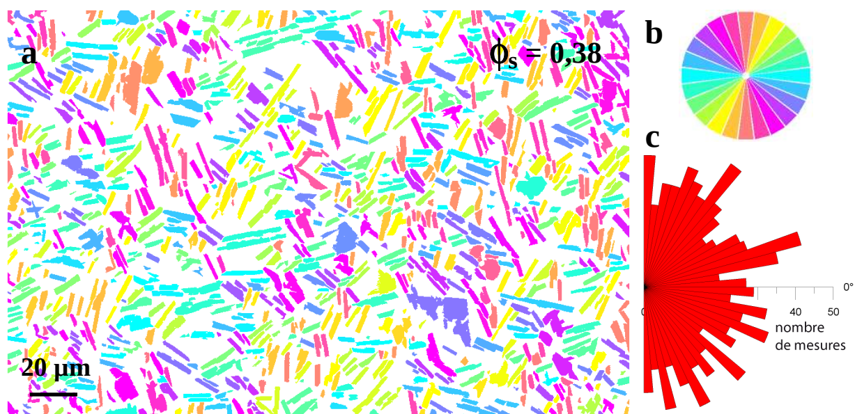
Figure III.12 : Orientations individuelles des cristaux d'une suspension non déformée contenant \phi_s = 0,38 (figure III.10). (a) Cristaux colorés suivant leurs orientations. (b) Rose de couleurs des orientations (c) Rose des directions des orientations individuelles des cristaux.
