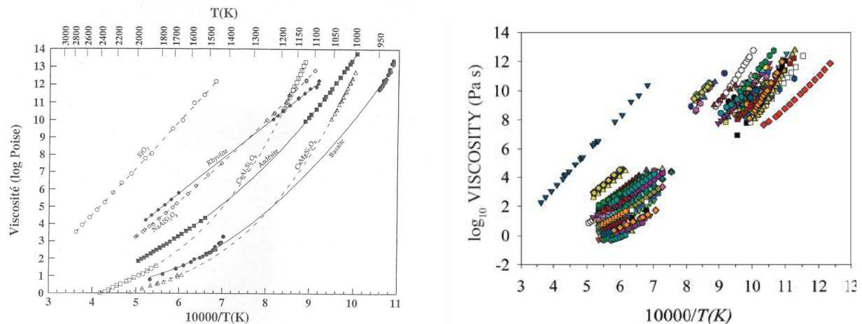
Figure I.4 : Influence de la composition chimique sur la viscosité des liquides silicatés. A gauche d'après Levesque (1999) et à droite d'après Dingwell (2006).
