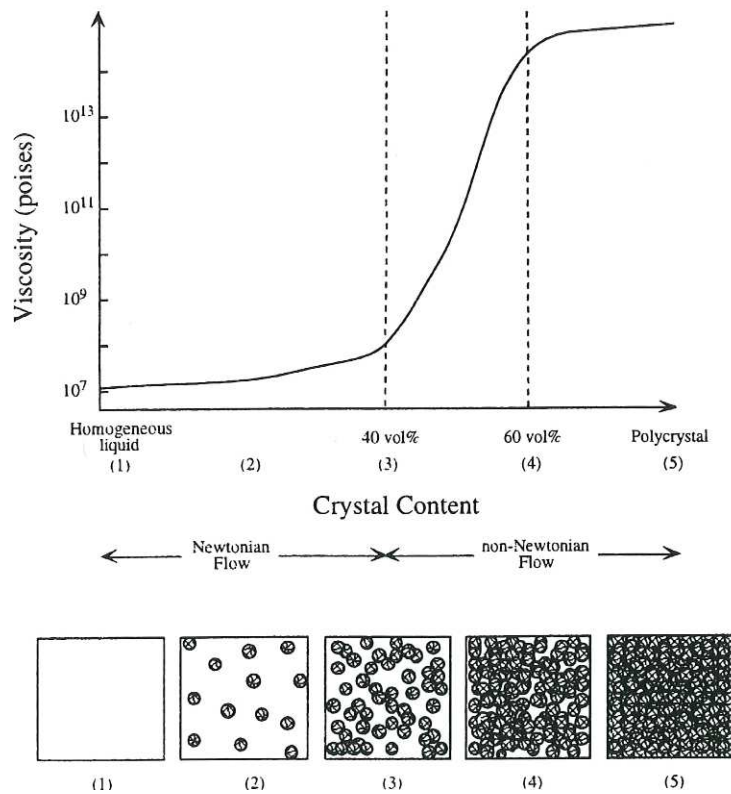
Figure I.13 : Log de la viscosité des suspensions magmatiques en fonction de la fraction cristalline. Un seuil rhéologique correspondant au passage Newtonien – non Newtonien et associé à une interconnectivité des cristaux a été établi entre 40% et 60% de cristaux. Ce seuil est accompagné d'une hausse de la viscosité d'environ 5 ordres de grandeurs. Les schémas ci-dessous représentent l'évolution structurale de la suspension (Lejeune et Richet, 1995).
