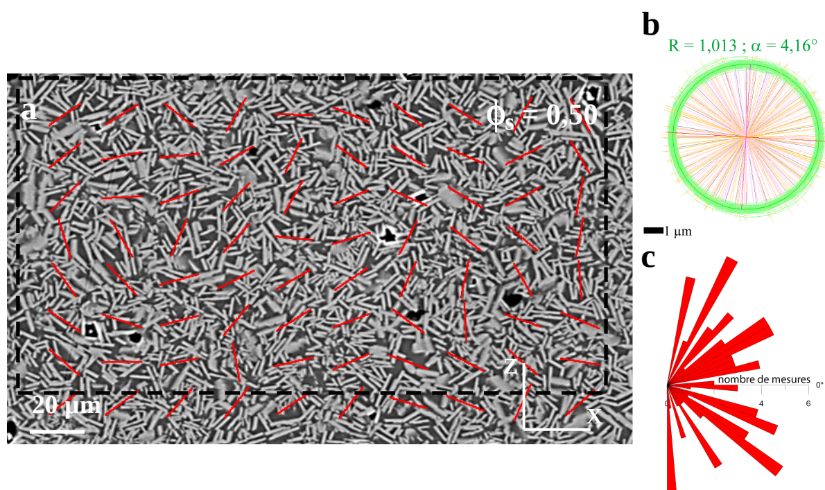
Figure III.11 : Détermination des textures pour une suspension non déformée contenant \phi_s = 0,50 . (a) Image MEB en électrons rétrodiffusés. Les traits rouges représentent les axes longs des ellipses locales tensorielles de fabrication de forme. (b) Ellipses tensorielles locales de fabrication de forme. Les valeurs de l'excentricité de l'ellipse moyenne ( R ) ainsi que la direction d'orientation de l'axe long de cette ellipse ( \alpha ) sont indiquées au dessus de l'ellipse. (c) Roses des directions regroupant les axes longs des ellipses locales tensorielles.
