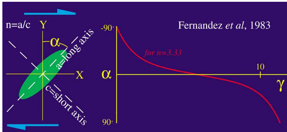
Figure I.11 : Orientation de l'axe long d'une particule soumise à un cisaillement simple. L'orbite effectuée est cyclique et confirme le modèle de Jeffery (1922) ( Fernandez et al., 1983 ).
