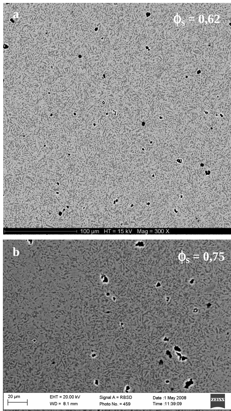
Figure III.18 : Images MEB prises en électrons rétrodiffusés des suspensions initiales non déformées contenant \phi_s = 0,62 (a) et \phi_s = 0,75 (b).
