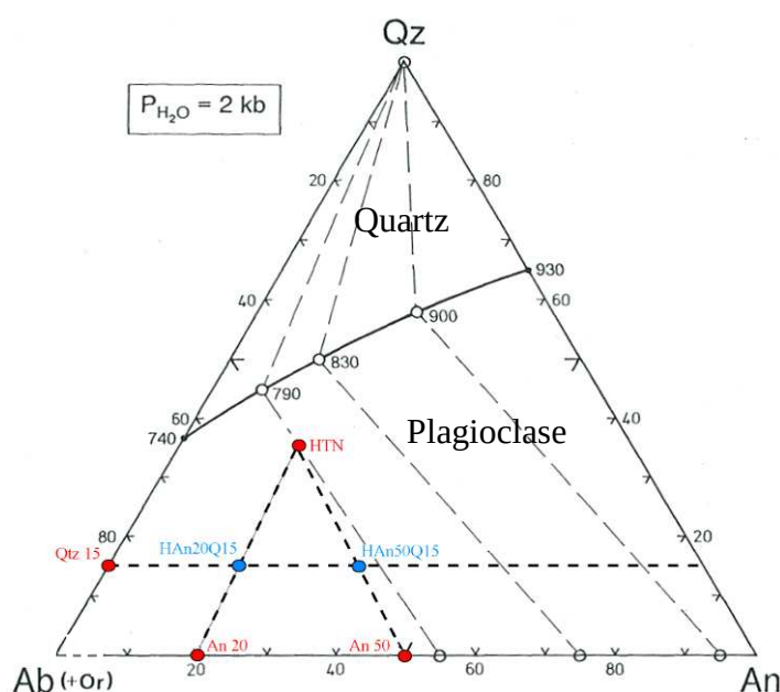
Figure III.4 : Compositions des mélanges reportées dans un diagramme ternaire Qz-Ab-An. La courbe cotectique (en noir) et les compositions des phases coexistantes sont indiquées pour P_{H_2O} = 2\text{ kbar} (Johannes et Holtz, 1996). Les lignes pointillées relient les phases coexistantes (indiquées par les cercles) pour des températures de 790°, 830 et 900°C. Les points noirs représentent les points eutectiques pour le système binaire Qz-An et Qz-Ab. Les compositions de départ sont représentées par un rond rouge et les mélanges obtenus à partir de ces compositions par un rond bleu.
