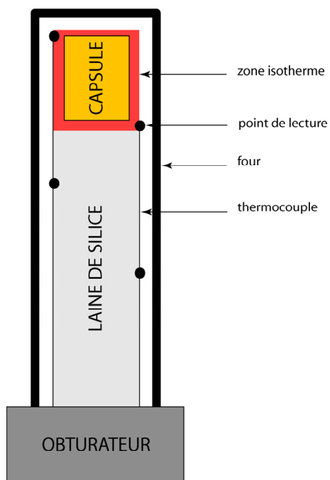
Figure II.2 : Disposition schématique des thermocouples et de la capsule par rapport à la zone isotherme du four.
