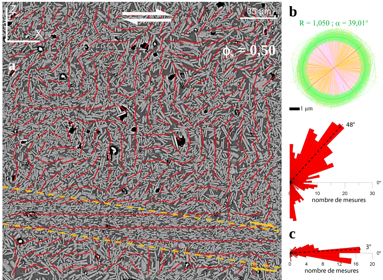
Figure V.7 : Orientation préférentielle de forme d'une fabrique contenant \phi_s = 0,50 . (a) Image MEB prise au cœur d'une section [XZ] de l'échantillon PP058 ( \dot{\gamma} = 1.10^{-4} \text{ s}^{-1} ). Les traits rouges représentent les axes longs des ellipses locales tensorielles de fabrique de forme. La bande de cisaillement est délimitée par les traits pointillés jaunes. (b) Ellipses tensorielles locales de fabrique de forme. Les valeurs de l'excentricité de l'ellipse moyenne ( R ) ainsi que la direction d'orientation de l'axe long de cette ellipse ( \alpha ) sont indiquées au dessus de l'ellipse. (c) Roses des directions regroupant les axes longs des ellipses locales tensorielles : en haut pour la fabrique pénétrative et en bas pour la bande de cisaillement. Les directions d'orientation maximales sont indiquées en noir.
