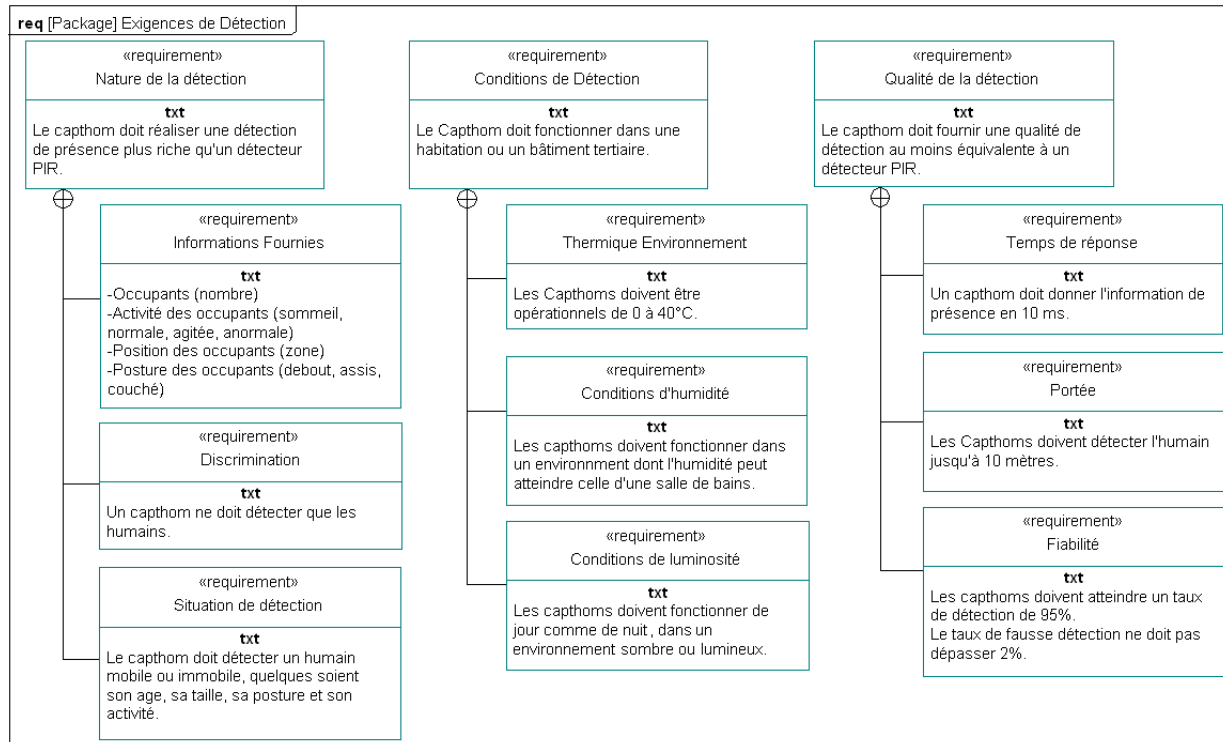
Figure IV.4 Requirement Diagram des Exigences de Détection
