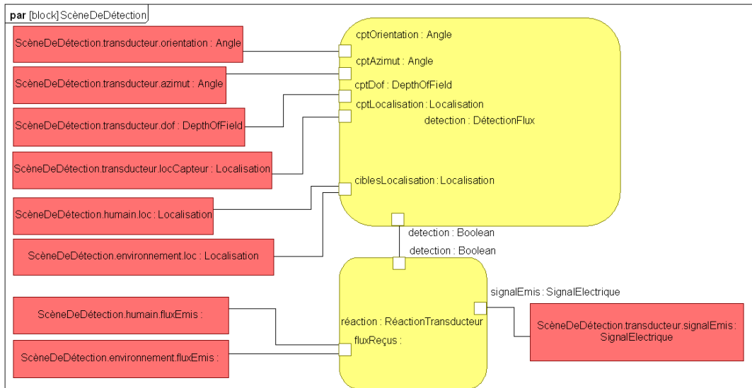
Figure IV.13 Parametric Diagram de la détection de présence
