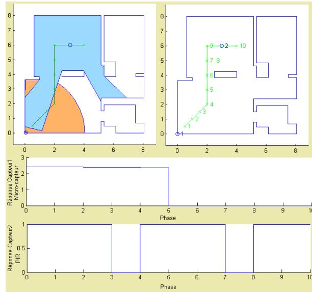
Figure IV.19 Exemple de scénario et réponse du réseau
