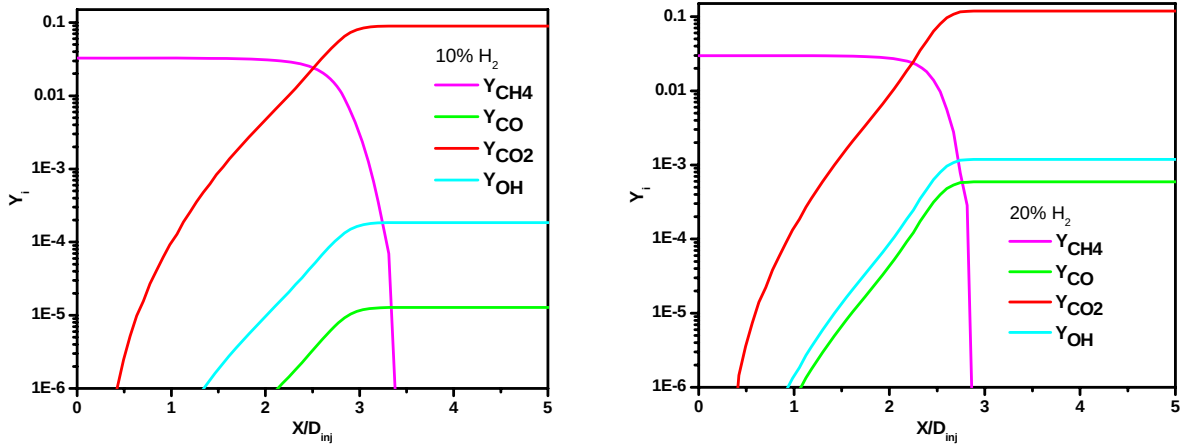
Figure 7.35 Variation de la fraction des espèces le long de l'axe de symétrie.
