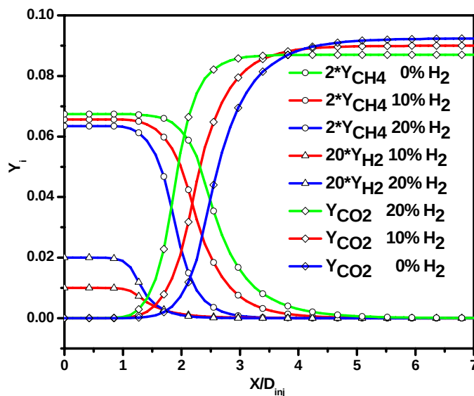
Figure 7. 30 Evolution des espèces sur l'axe de symétrie
