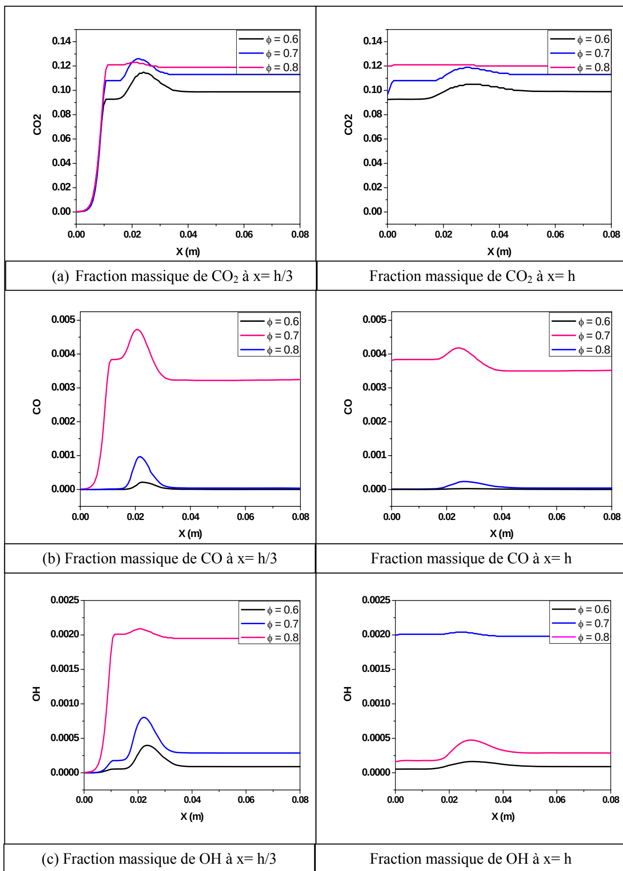
Figure 7.25 Effet de la richesse sur les fractions de \text{CO}_2 , CO et OH.
