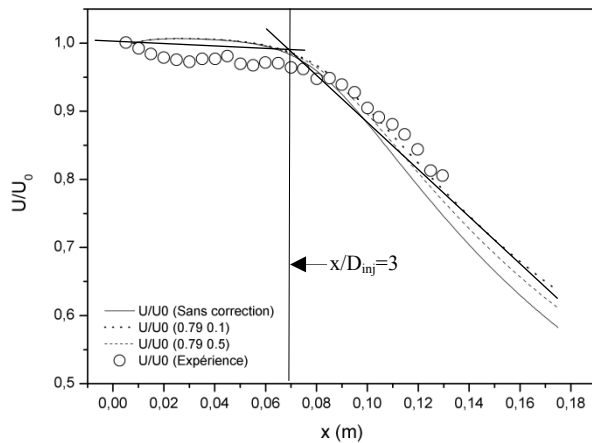
Figure 7.6 Vitesse axiale
