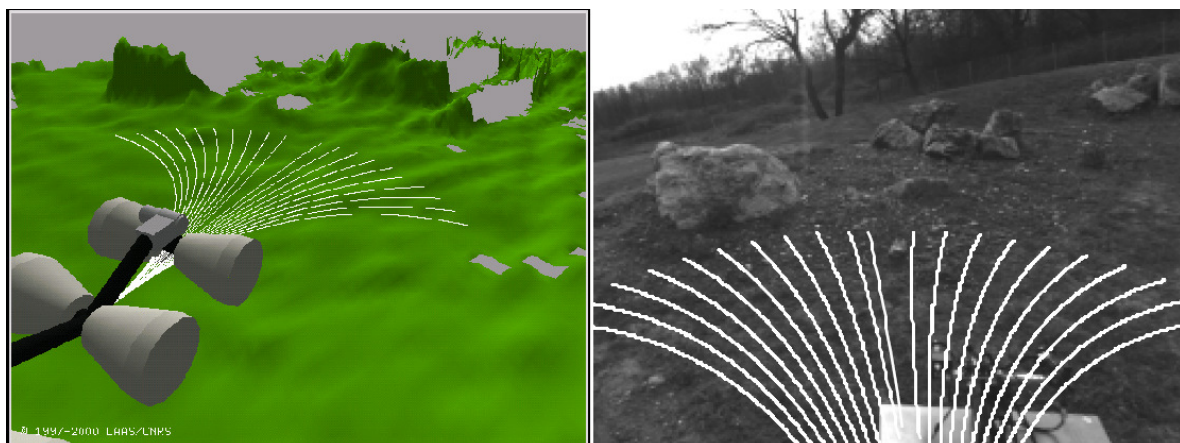
Figure 24 - La méthode Motion Generation appliquée sur le robot LAMA du LAAS
