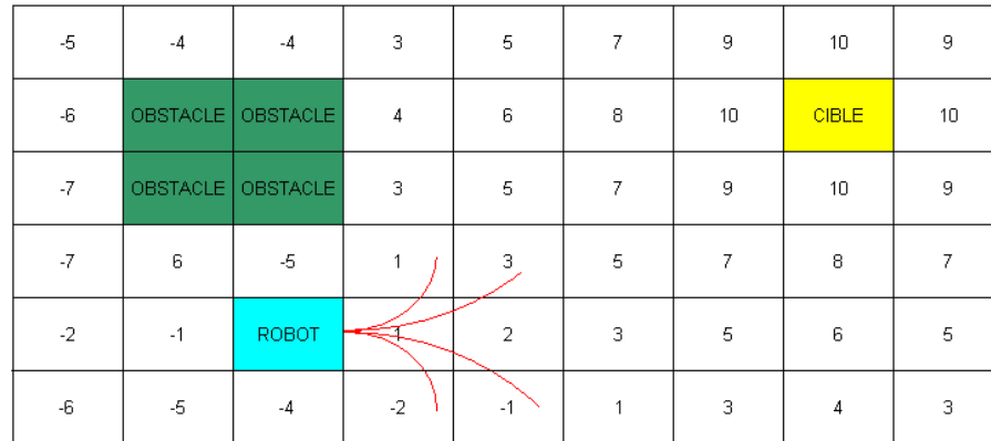
Figure 25 - la méthode Neural Network hybride : projection d'un set de trajectoires réalisables par le robot dans une carte de l'environnement sous forme de grille
