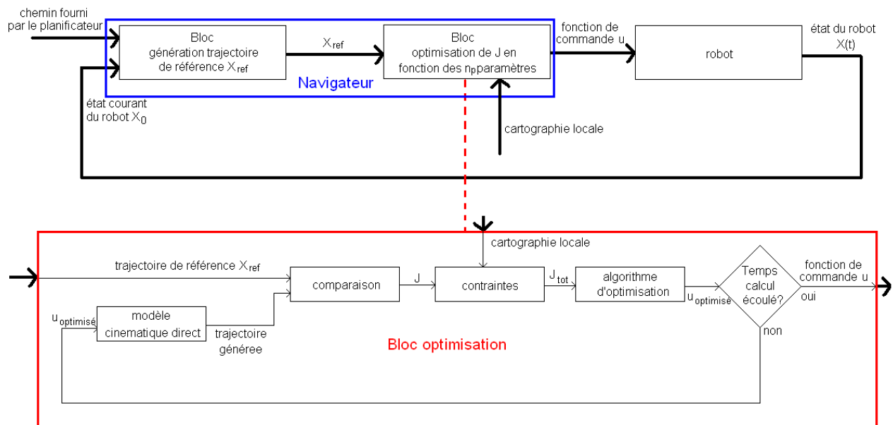
Figure 61- Représentation du principe de la commande
