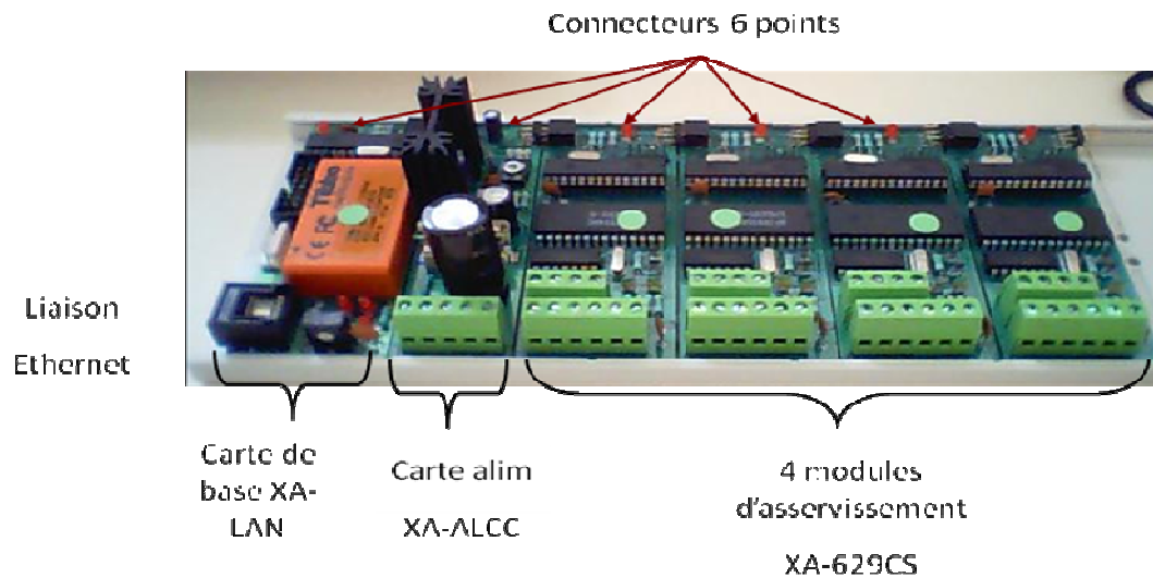
Figure 87- Rail de commande Sidena, avec 4 cartes d'axe, un module d'alimentation et un module ethernet
