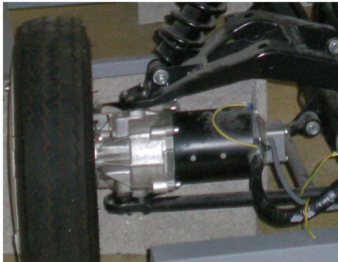
Figure 84- Moteur de traction avec codeur incrémental
