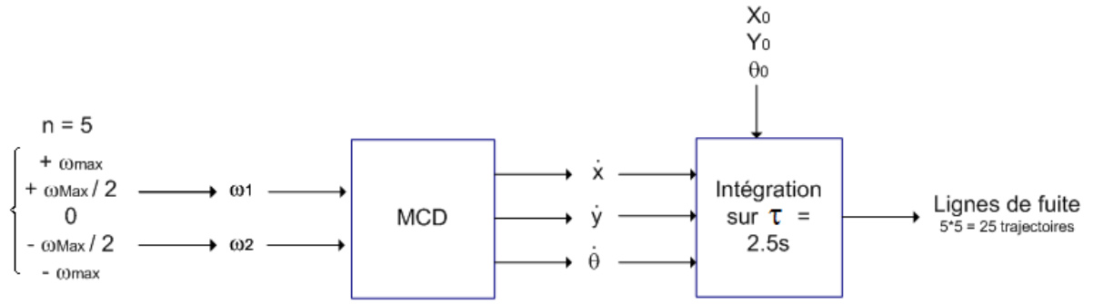
Figure 31 - Discrétisation des entrées du robot et génération des lignes de fuite
