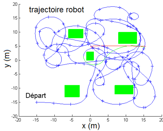
Figure 81 : planificateur fou et robustesse du navigateur à une planification défectueuse
