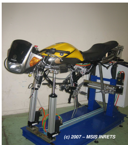
Figure 55 : Le simulateur de conduite moto MSIS/INRETS
