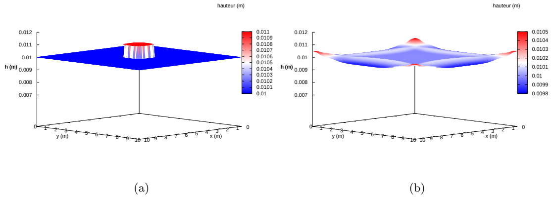
FIG. 7.8: Rupture de barrage radial sur fond mouillé : (a) Condition initiale et (b) au temps t = 5 s.
