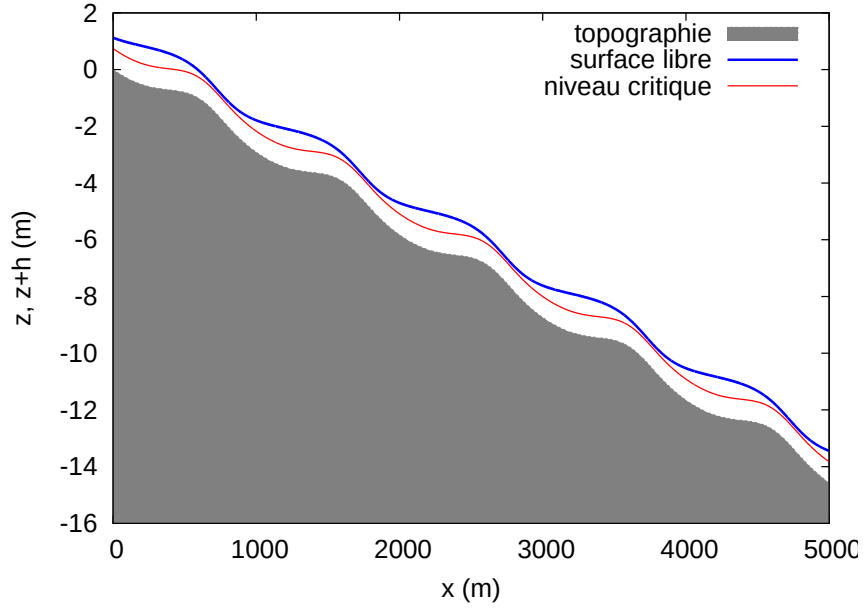
FIG. 3.10: Ecoulement fluvial-fluvial périodique pour la loi de Manning.
