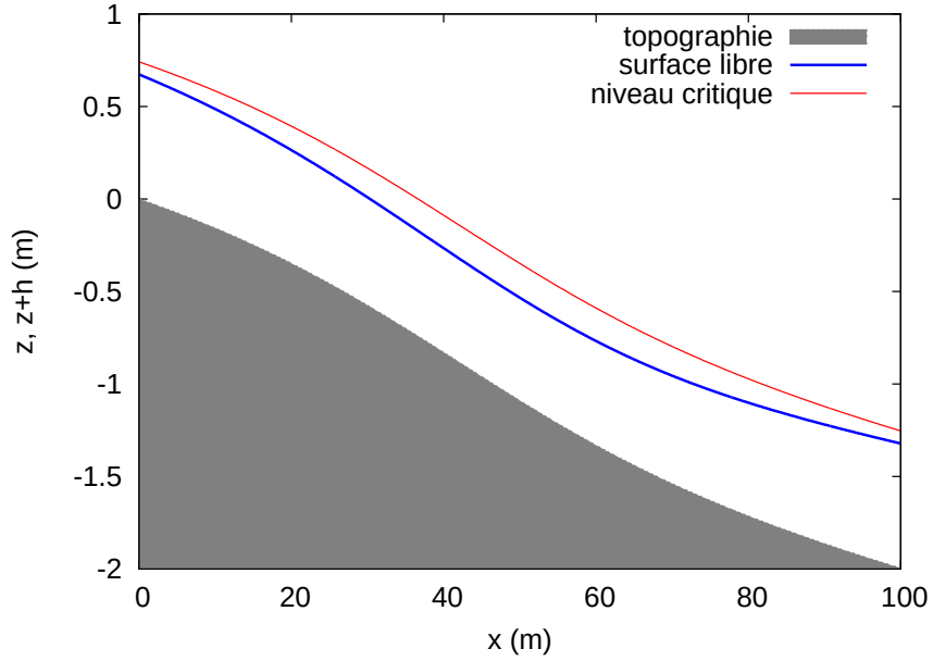
FIG. 3.9: Ecoulement torrentiel-torrentiel pour la loi de Manning.
