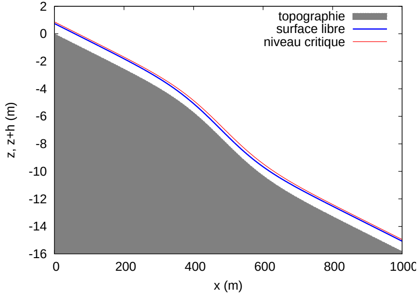
FIG. 3.4: Ecoulement torrentiel-torrentiel pour la loi de Darcy-Weisbach.
