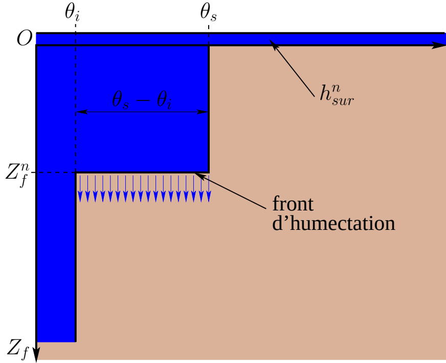
FIG. 5.14: Illustration du modèle de Green-Ampt.
