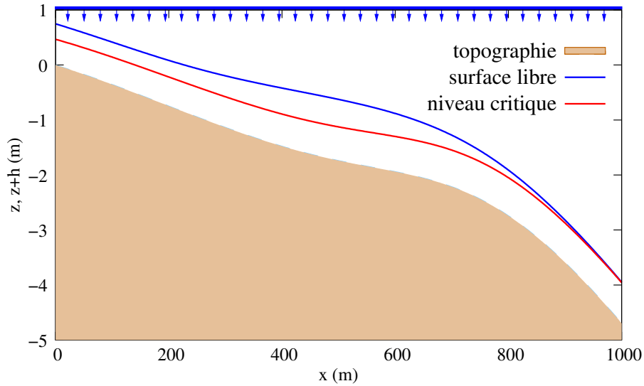
FIG. 5.4: Ecoulement fluvial-fluvial avec de la pluie pour la loi de Darcy-Weisbach.
