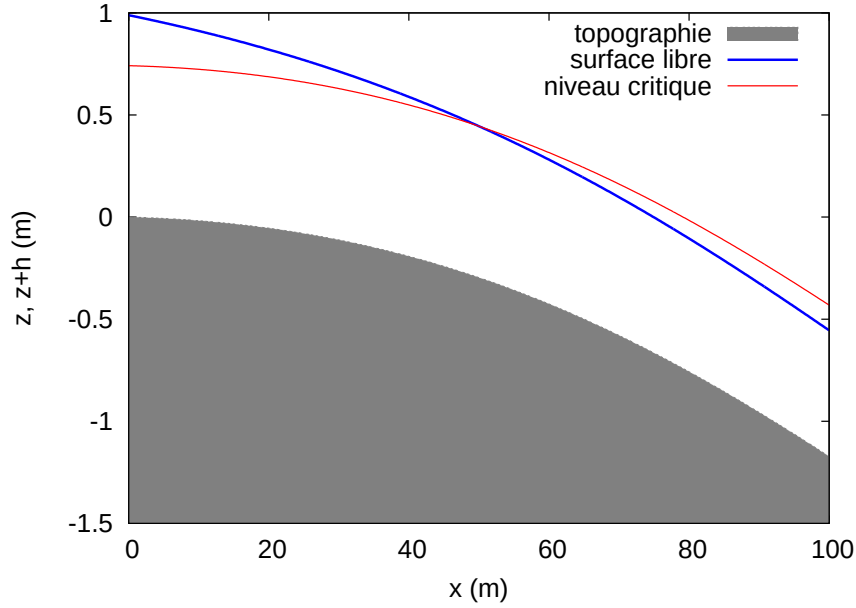
FIG. 3.8: Ecoulement fluvial-torrentiel pour la loi de Manning.
