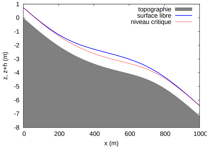
FIG. 3.3: Ecoulement fluvial-fluvial pour la loi de Darcy-Weisbach.
