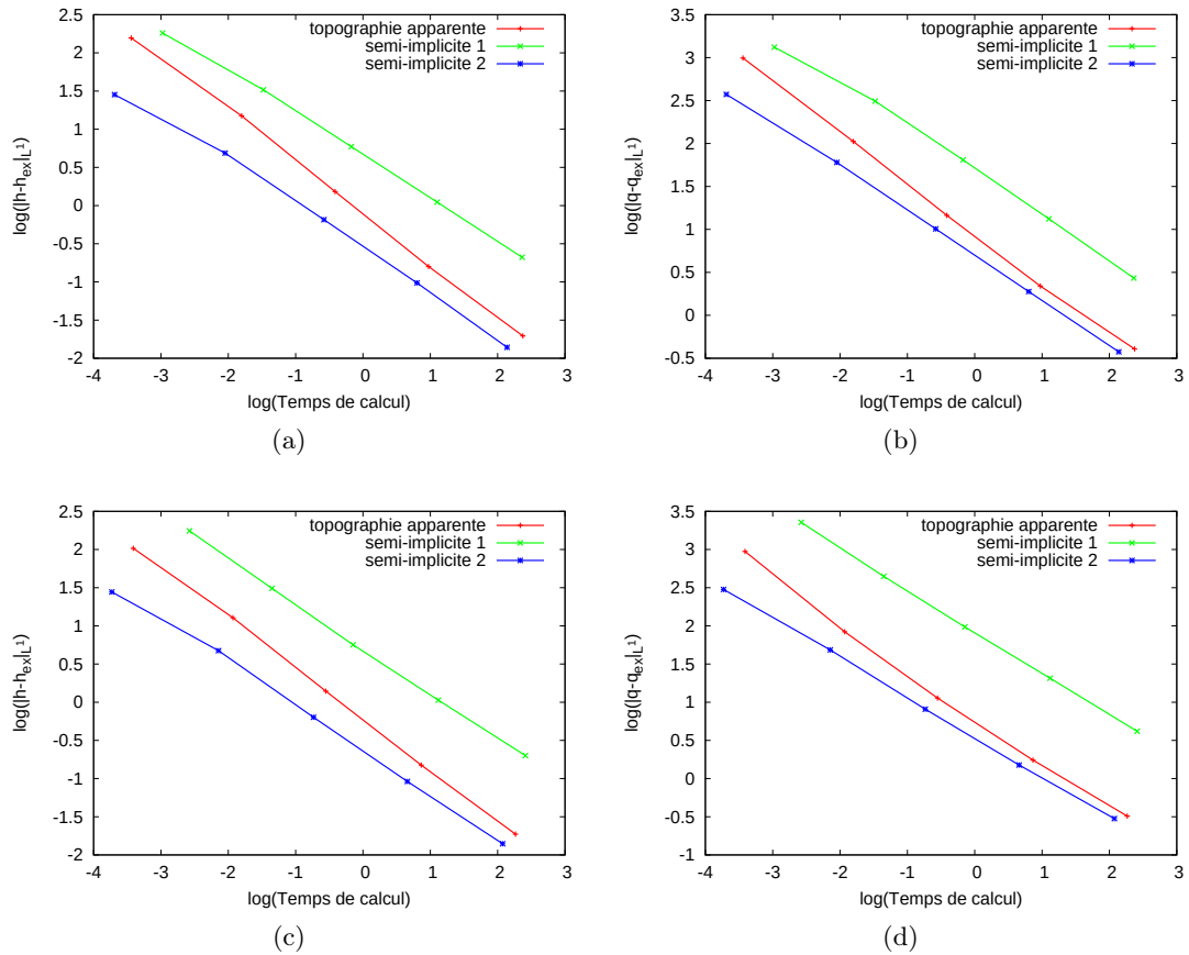
FIG. 3.20: Ecoulement fluvial-torrentiel 1 : comparaison de l'efficacité des méthodes pour le calcul (a) des hauteurs d'eau, (b) des vitesses pour la loi de Manning et (c) des hauteurs d'eau, (b) des vitesses pour la loi de Darcy-Weisbach.
