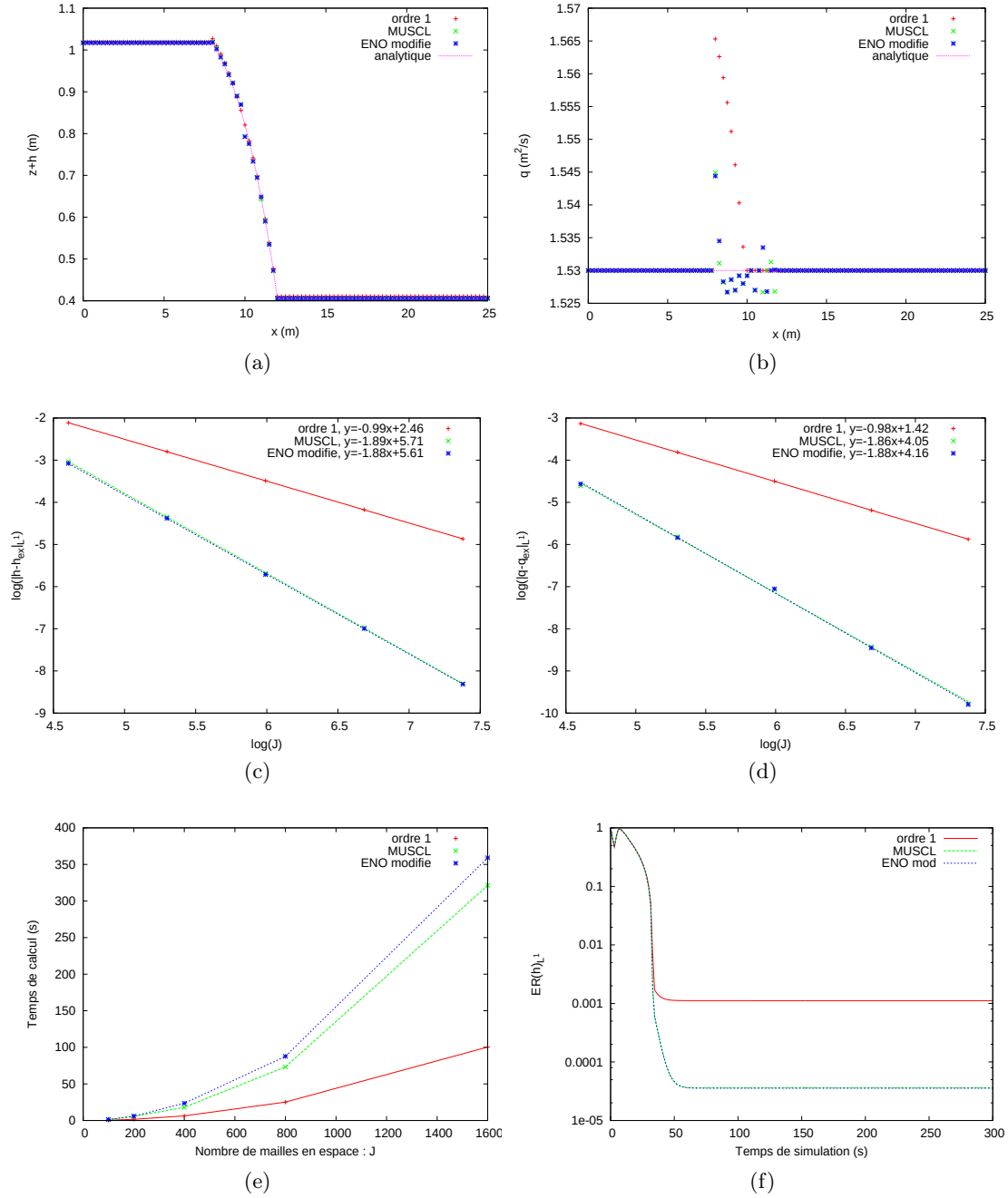
FIG. 2.21: Flux Astat : comparaison (a) des hauteurs d'eau, (b) des débits, des erreurs sur (c) les hauteurs, (d) les débits, (e) des temps de calcul et (f) des convergences en temps.
