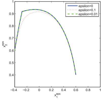
Figure 2.22: Trajectory (x_1^\varepsilon(\cdot), x_2^\varepsilon(\cdot))
