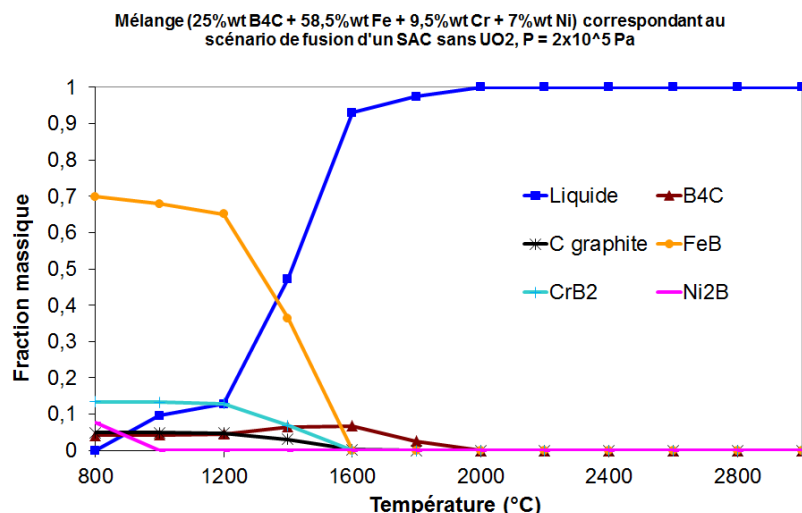
Figure 6-1 : Calcul GEMINI2 + NUCLEA_08 relatif à l'interaction 25% \text{B}_4\text{C} + 58,5% Fe + 9,5% Cr + 7% Ni (composition massique), simulant la fusion d'un assemblage avec un SAC sans prendre en compte l' \text{UO}_2 . Sur le graphe sont tracées les fractions massiques des produits présents en fonction de la température.
