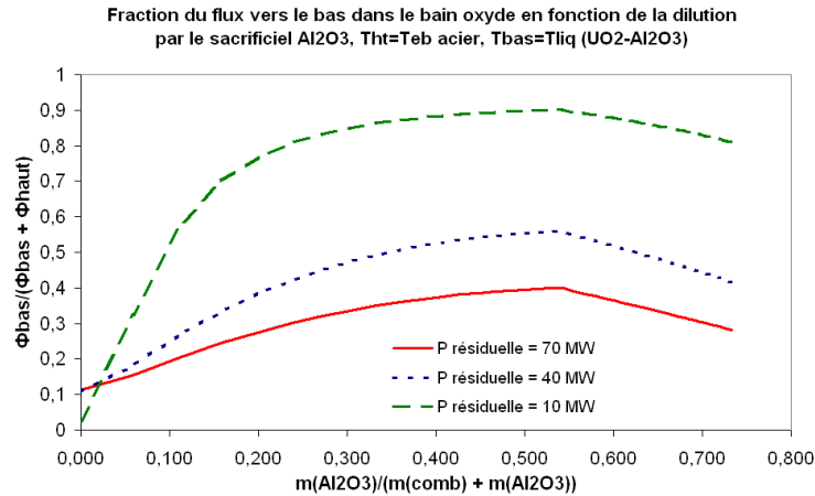
Figure A11-4 : Fraction du flux de chaleur vers le bas dans le bain oxyde en fonction de la dilution par le sacrificiel \text{Al}_2\text{O}_3 , dans le cas de non formation de croûte à la surface supérieure du bain
