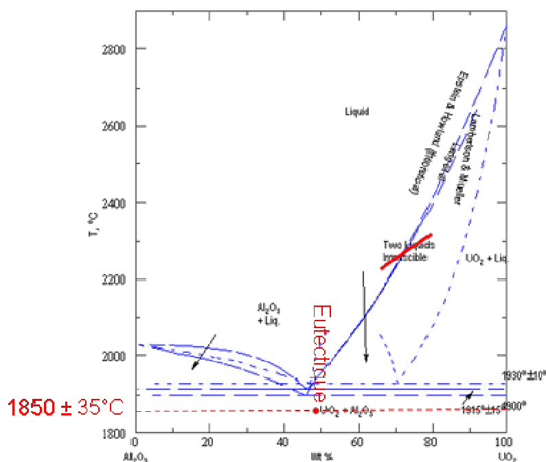
Figure 6-54 : Diagramme de phases \text{Al}_2\text{O}_3 – \text{UO}_2 modifié après les essais CORSICCA 2_Al_1
