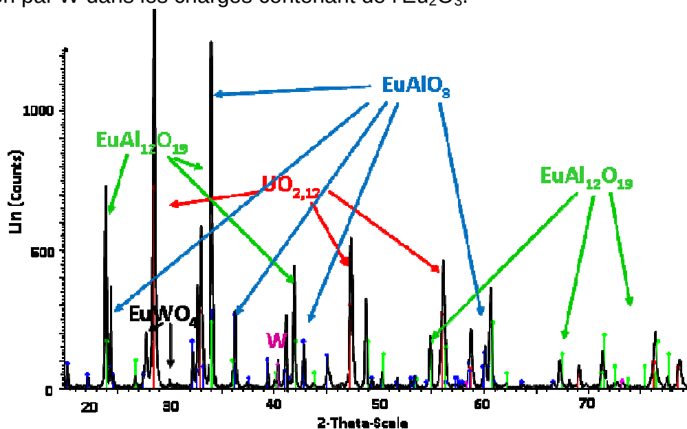
Figure 6-46 : Spectre DRX relatif au mélange initial 20% \text{UO}_2 – 40% \text{Al}_2\text{O}_3 – 40% \text{Eu}_2\text{O}_3 en proportions massiques après le chauffage jusqu'à 1870°C et refroidissement dans un creuset en tungstène
