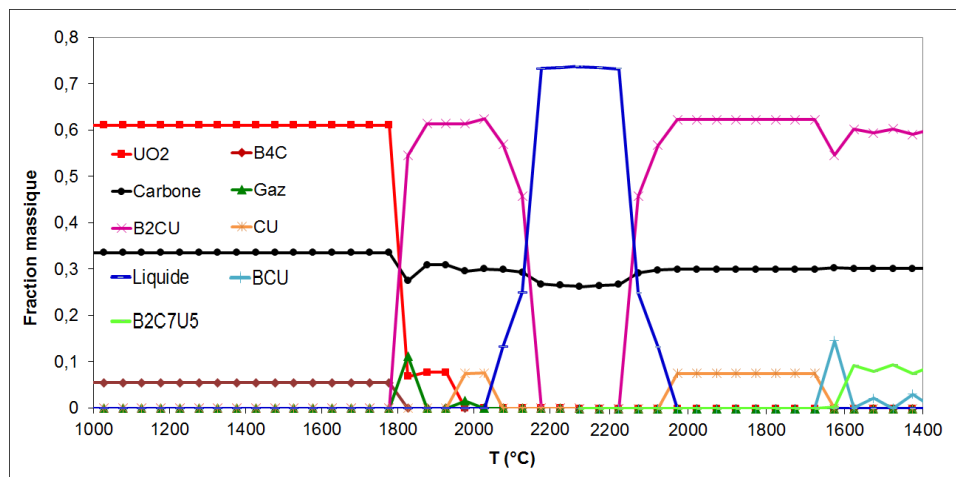
Figure 6-15 : Calcul GEMINI2 + NUCLEA_08 reproduisant l'essai d'interaction 91,5% \text{UO}_2 + 8,5% \text{B}_4\text{C} (composition massique) qui simule la fusion d'un SAC sans acier, avec l'excès de carbone dans le mélange. Sur la courbe sont tracées les fractions massiques des produits présents en fonction de la température, au cours du chauffage puis du refroidissement.
