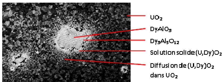
Figure 3-9 : \text{Al}_2\text{O}_3 - \text{Dy}_2\text{O}_3 dans \text{UO}_2 après 1h de frittage à 1600°C sous \text{Ar}-5\%\text{H}_2 , surface attaquée pour l'observation par \text{H}_2\text{O}_2 , x 500
