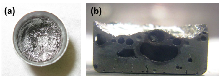
Figure 6-25 : Le mélange 40% \text{Al}_2\text{O}_3 + 60% \text{UO}_2 en proportions massiques après le chauffage jusqu'à 2200°C et le refroidissement. Le diamètre externe du creuset est de 20 mm. (a) Vue du dessus du creuset en tungstène (b) Section longitudinale de la charge.
