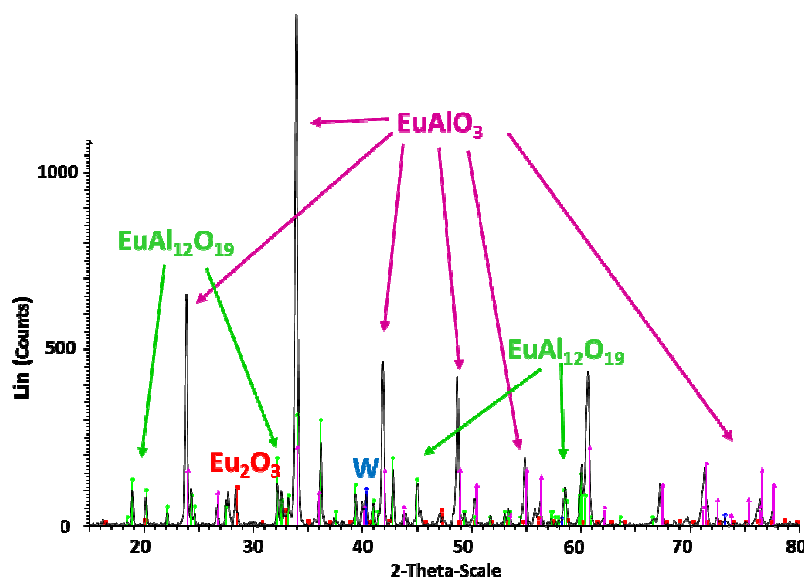
Figure 6-37 : Spectre DRX relatif au mélange initial 53% \text{Eu}_2\text{O}_3 + 47% \text{Al}_2\text{O}_3 en proportions massiques après le chauffage jusqu'à 2200°C et refroidissement dans un creuset en tungstène
