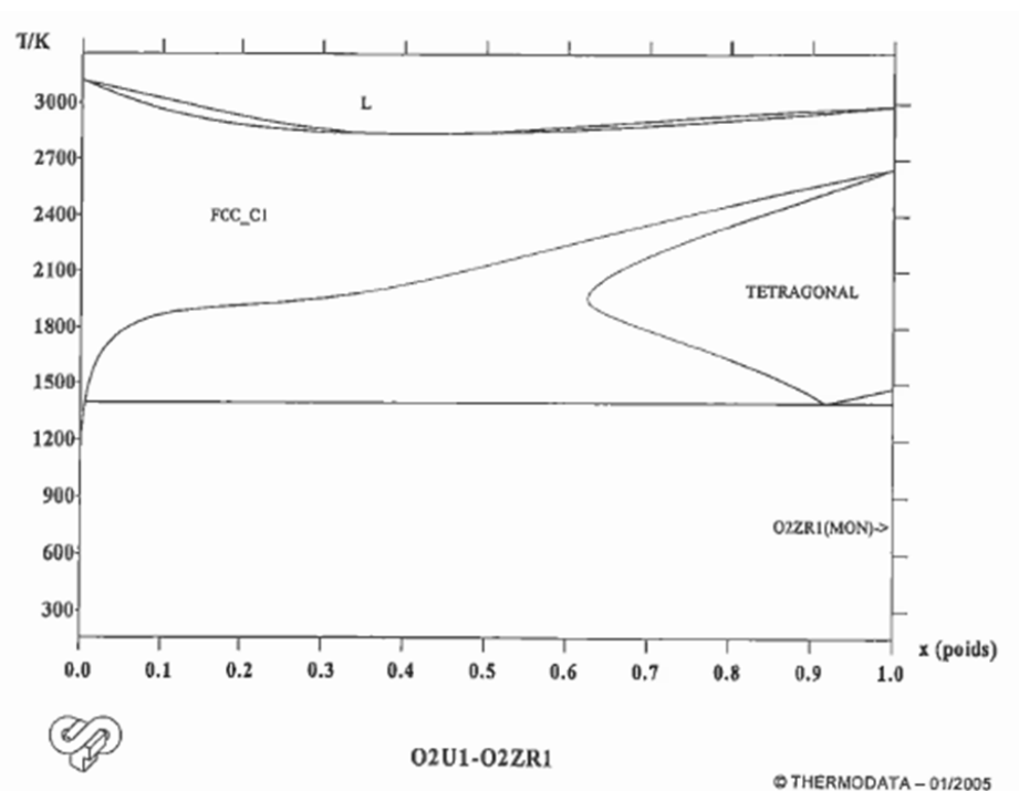
Figure A4-9 : Diagramme de phases \text{ZrO}_2 - \text{UO}_2 contenu dans la base de données Nuclea – Critère de qualité = acceptable
