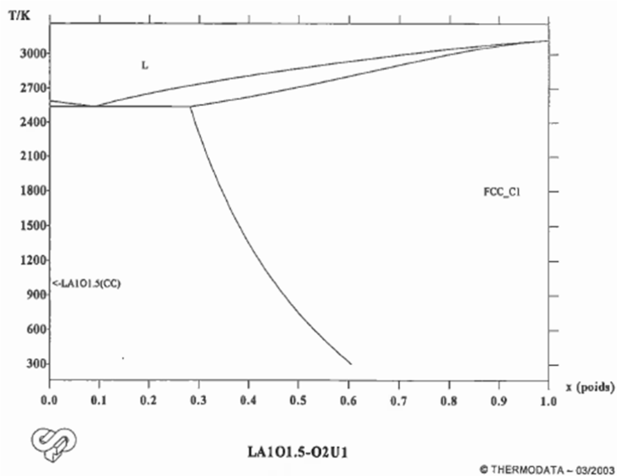
Figure A4-10 : Diagramme de phases \text{La}_2\text{O}_3 - \text{UO}_2 contenu dans la base de données Nuclea – Critère de qualité = acceptable
