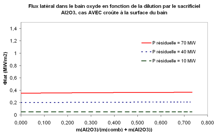
Figure A12-1 : Flux latéral dans le bain oxyde en fonction de la dilution par le sacrificiel \text{Al}_2\text{O}_3 dans le cas de la formation d'une croûte stable à la surface du bain
