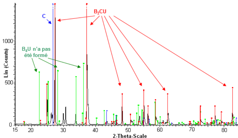
Figure 6-13 : Spectre DRX de la charge fondue \text{UO}_2 - \text{B}_4\text{C} dans un creuset en graphite après le refroidissement
