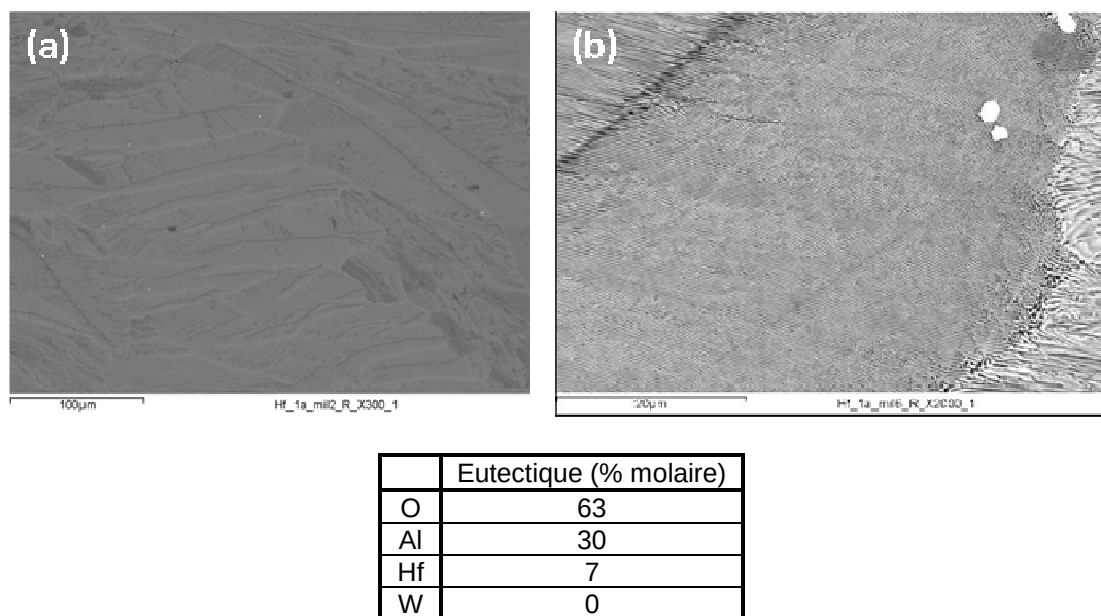
Figure 6-40 : Micrographie MEB accompagnée de l'analyse par EDS du mélange 50% \text{HfO}_2 + 50% \text{Al}_2\text{O}_3 en proportions massiques après le chauffage jusqu'à 2120°C et refroidissement dans un creuset en tungstène.
