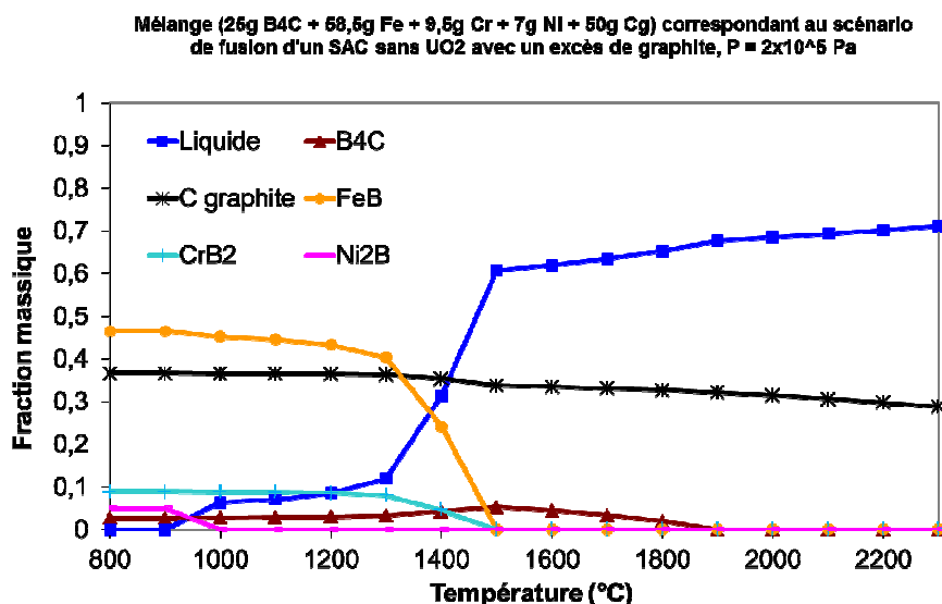
Figure 6-8 : Calcul GEMINI2 + NUCLEA_08 relatif à l'interaction 25% \text{B}_4\text{C} + 58,5% Fe + 9,5% Cr + 7% Ni (composition massique), simulant la fusion d'un assemblage avec un SAC sans prendre en compte \text{UO}_2 en présence de carbone graphite en excès. Sur le graphe sont tracées les fractions massiques des produits présents en fonction de la température.
