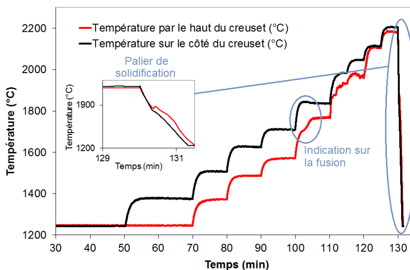
Figure 6-26 : Courbe de températures (température en fonction de la durée de l'essai) enregistrée au cours de l'essai CORSICCA 2_Al_1c relatif à l'interaction 60% \text{UO}_2 – 40% \text{Al}_2\text{O}_3 (composition massique) dans un creuset en tungstène, dans le but d'infirmer l'existence de la lacune de miscibilité. La température maximale de l'essai était de 2200 \pm 35^\circ\text{C} . Le palier de solidification est visible au refroidissement.
