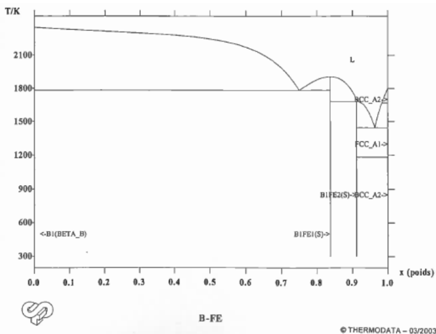
Figure A4-3 : Diagramme de phases B-Fe contenu dans la base de données Nuclea – Critère de qualité = acceptable
