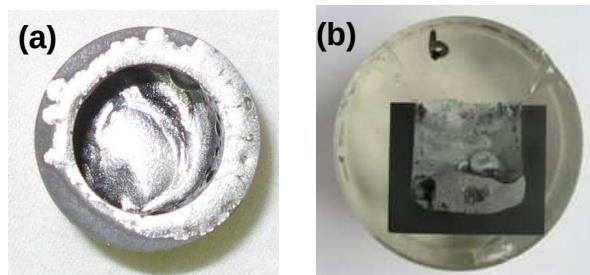
Figure 6-11 : Vue du creuset en graphite après l'essai d'interaction 91,5% \text{UO}_2 + 8,5% \text{B}_4\text{C} (composition massique). Le diamètre externe du creuset est de 25 mm. (a) Vue du dessus avec la charge qui a été projeté à l'extérieur du creuset, (b) Vue de la coupe longitudinale du creuset
