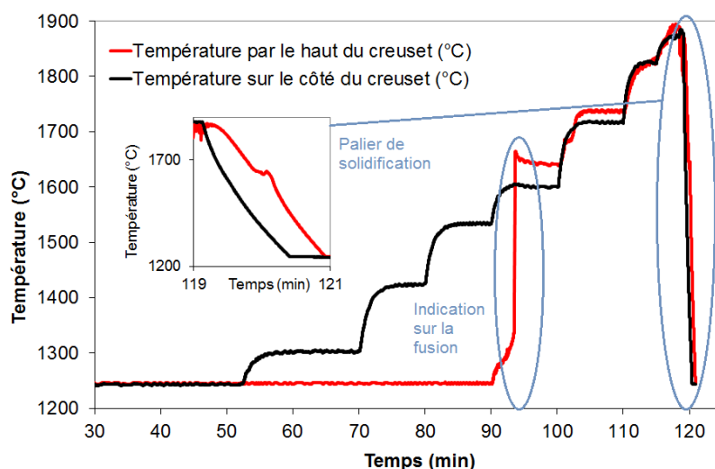
Figure 6-41 : Courbe de températures (température en fonction de la durée de l'essai) enregistrée au cours de l'essai CORSICCA 2_Al_3b relatif à l'interaction 30% \text{UO}_2 – 33% \text{Al}_2\text{O}_3 – 37% \text{Eu}_2\text{O}_3 (composition massique) dans un creuset en \text{UO}_2 . La température maximale de l'essai était de 1870 \pm 35^\circ\text{C} . Un palier de solidification est visible au refroidissement.
