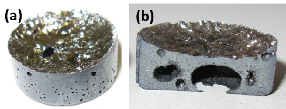
Figure 6-35 : Le mélange 53% \text{Eu}_2\text{O}_3 + 47% \text{Al}_2\text{O}_3 en proportions massiques après le chauffage jusqu'à 2200^\circ\text{C} et le refroidissement dans un creuset en tungstène. Le diamètre de la charge est de 20 mm. (a) Vue de toute la charge (b) Section longitudinale de la charge.
