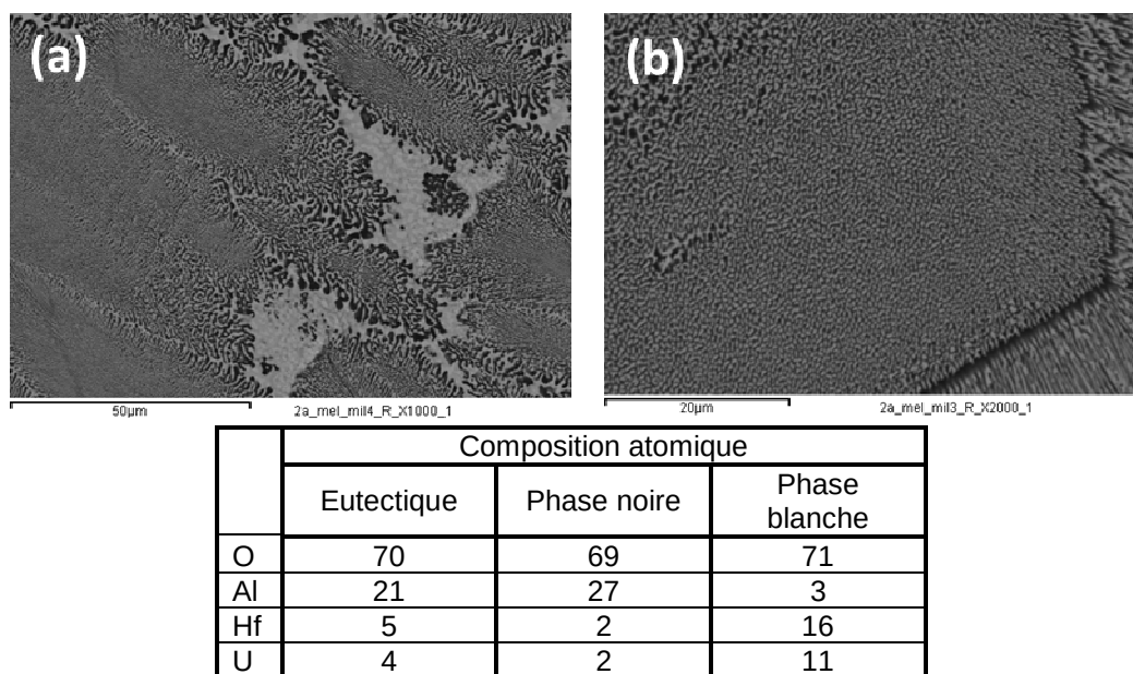
Figure 6-49 : Micrographie MEB accompagnée de l'analyse par EDX du mélange 31% \text{UO}_2 – 34% \text{Al}_2\text{O}_3 – 35% \text{HfO}_2 en proportions massiques après le chauffage jusqu'à 1870^\circ\text{C} et refroidissement dans un creuset en tungstène
