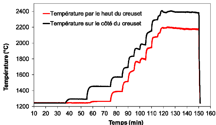
Figure 6-16 : Courbe de températures (température en fonction de la durée de l'essai) enregistrée au cours de l'essai CORSICCA 1_2e relatif à l'interaction \text{UO}_2 – \text{B}_4\text{C} dans un creuset en tungstène. Aucun palier de solidification n'est visible au refroidissement.
