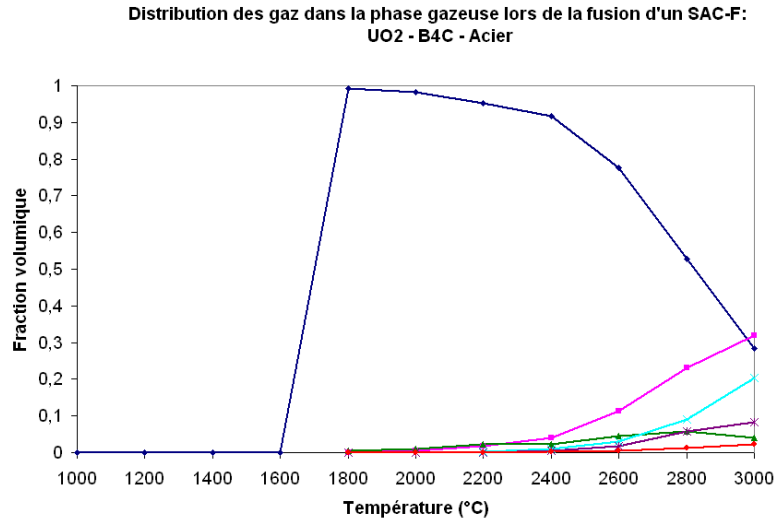
Figure 4-10: Distribution des gaz dans la phase gazeuse lors de la fusion d'un SAC avec acier (interaction 6,8%wt B 11 C 3 – 72,7%wt UO 2 – 16%wt Fe – 2,6%wt Cr – 1,9%wt Ni)
