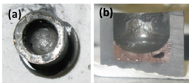
Figure 6-23 : Creuset en graphite initialement revêtu de ZrC, après l'essai d'étude du mélange 52\% \text{ Al}_2\text{O}_3 + 48\% \text{ UO}_2 en proportions massiques eutectiques. Le diamètre externe du creuset est de 25 \text{ mm} . (a) Vue du dessus (b) Section longitudinale du creuset. Le revêtement a bien résisté à la charge portée à 1870^\circ\text{C} (\pm 35^\circ\text{C}) .
