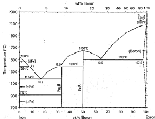
Figure 3-14: Diagramme de phases du système Fe – B [3.48]
