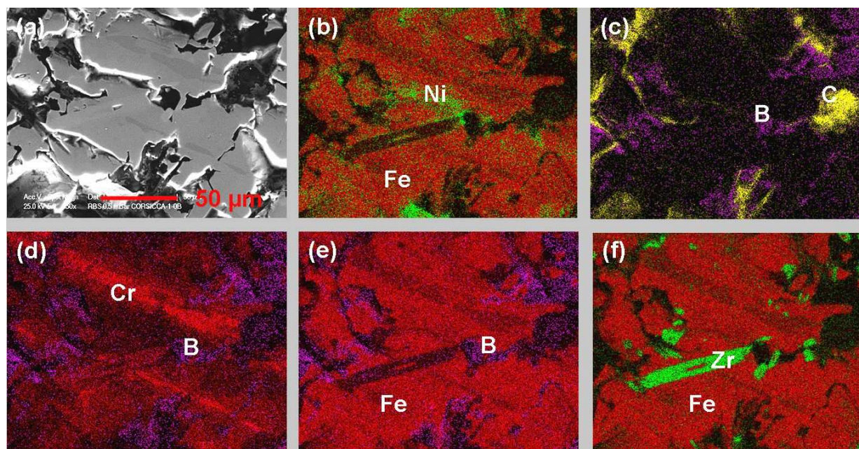
Figure 6-6 : Cartographie EDX de la charge fondue Acier inoxydable – \text{B}_4\text{C} après le refroidissement, effectuée à l'Institut de Chimie Inorganique à Rez, République Tchèque. (a) micrographie MEB de l'échantillon, (b) Fe en rouge, Ni en vert, (c) B en violet, C en jaune, (d) Cr en rouge, B en violet, (e) Fe en rouge, B en violet, (f) Fe en rouge, Zr en vert
