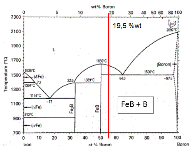
Figure 6-7 : Diagramme de phases Fe – B avec l'indication de la composition du mélange expérimental lors de l'essai d'interaction Acier inoxydable – \text{B}_4\text{C} (en assimilant l'acier au fer)
