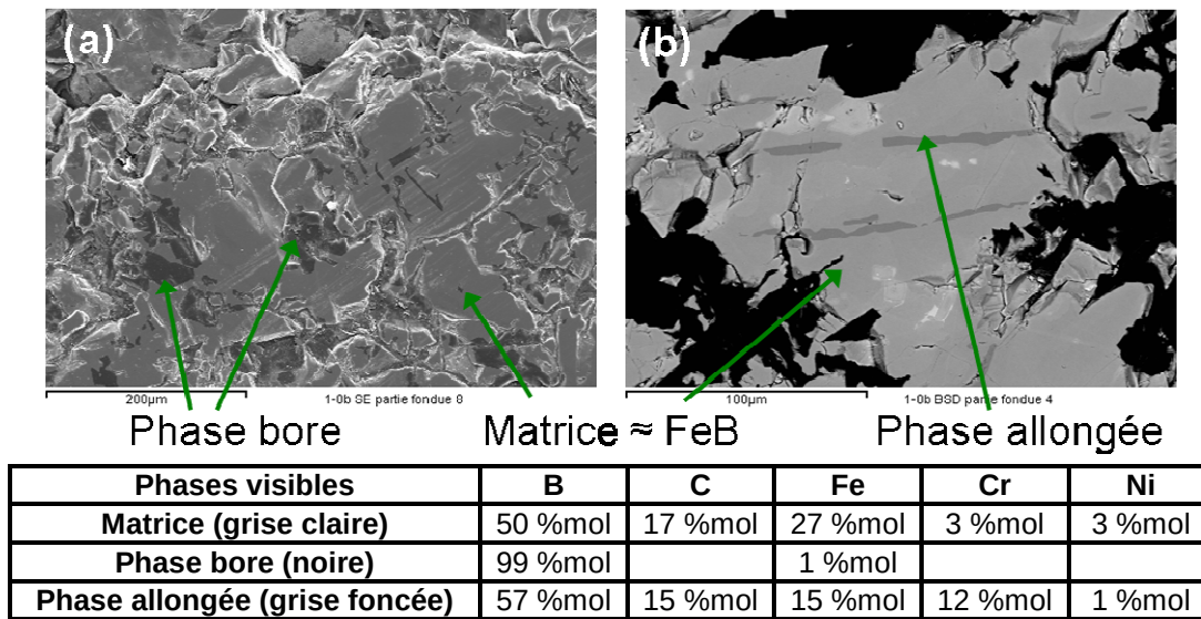
Figure 6-5 : Photos MEB de la charge fondue Acier inoxydable – \text{B}_4\text{C} après le refroidissement avec l'analyse chimique EDX. Trois phases ont été révélées : la matrice contenant majoritairement du fer, du bore et du carbone (en gris clair), la phase bore pure (en noir sur l'image (a)) et la phase allongée enrichie en chrome, contenant du fer, du chrome, du bore et du carbone (en gris foncé sur l'image (b) en électrons rétrodiffusés)
