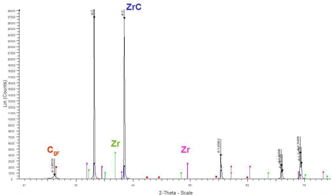
Figure 5-18 : Spectre DRX du revêtement en carbure de zirconium. Le revêtement est du \text{ZrC} pur. Il n'y a plus de trace de zirconium : tout le zirconium a réagi.
