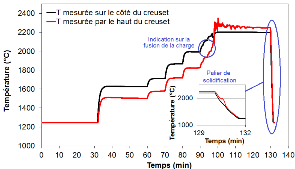
Figure 6-10 : Courbe de températures (température en fonction de la durée de l'essai) enregistrée au cours de l'essai CORSICCA 1_2b relatif à l'interaction \text{UO}_2 – \text{B}_4\text{C} dans un creuset en graphite. Le palier de solidification est visible au refroidissement.
