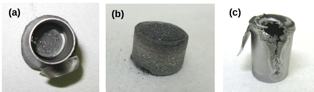
Figure 6-17 : (a) Vue du creuset en tungstène contenant la charge \text{UO}_2 - \text{B}_4\text{C} après le chauffage jusqu'à 2400^\circ\text{C} et le refroidissement (b) Charge \text{UO}_2 - \text{B}_4\text{C} correspondante (c) Creuset à l'envers – le fond du creuset a commencé à fondre. Le diamètre externe du creuset est de 20 mm.
