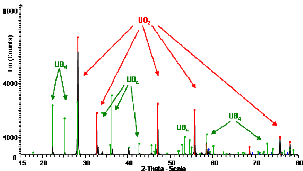
Figure 6-18 : Spectre DRX de la charge \text{UO}_2 - \text{B}_4\text{C} chauffée jusqu'à 2400^\circ\text{C} (palier à 2400^\circ\text{C} pendant 30 min) dans un creuset en tungstène, après le refroidissement
