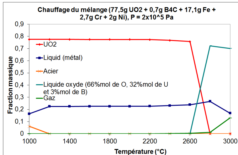
Figure 4-12: L'évolution des fractions massiques du système (0,7% B 11 C 3 – 77,5% UO 2 – 17,1% Fe – 2,7% Cr – 2% Ni) à l'équilibre, à 2·10 5 Pa, en fonction de la température du milieu
