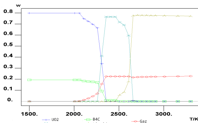
Figure A8-2 : L'évolution des fractions massiques du système (20%wt B_{11}C_3 – 80%wt UO_2 ) à l'équilibre, à 2 \cdot 10^5 Pa, en fonction de la température du milieu (en K). Lors de ce calcul, les gaz produits ont été conservés dans le système.
