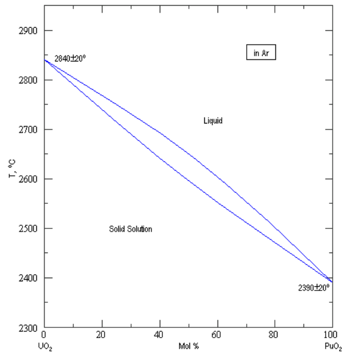
Figure A2-7 : Diagramme de phase \text{UO}_2 - \text{PuO}_2 [3.18]
