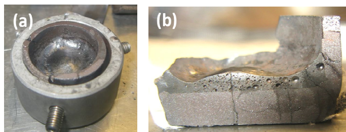
Figure 6-32 : Le mélange 70% \text{Eu}_2\text{O}_3 + 30% \text{UO}_2 en proportions massiques après le chauffage jusqu'à 2200^\circ\text{C} et le refroidissement dans un creuset en \text{UO}_2 . Le diamètre externe du creuset est de 27,9 mm. (a) Vue de toute la charge (b) Section longitudinale de la charge.
