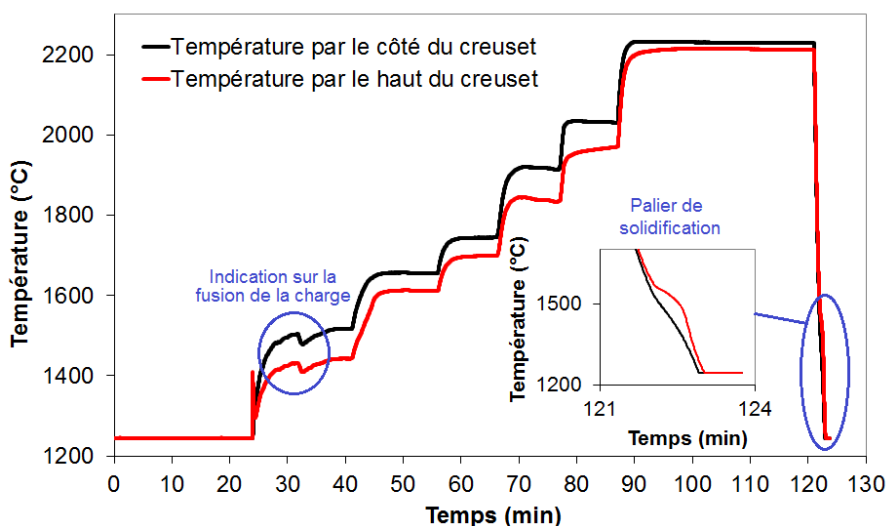
Figure 6-2 : Courbe de températures (température en fonction de la durée de l'essai) enregistrée au cours de l'essai CORSICCA 1_0. Le palier de solidification est visible au refroidissement.
