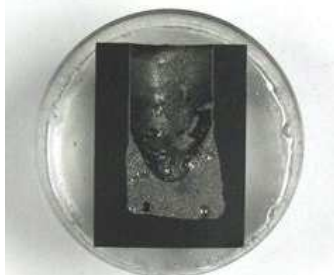
Figure 6-3 : Section longitudinale du creuset en graphite après refroidissement avec la charge fondue Acier inoxydable – \text{B}_4\text{C} . Le diamètre externe du creuset est de 25 \text{ mm} .
