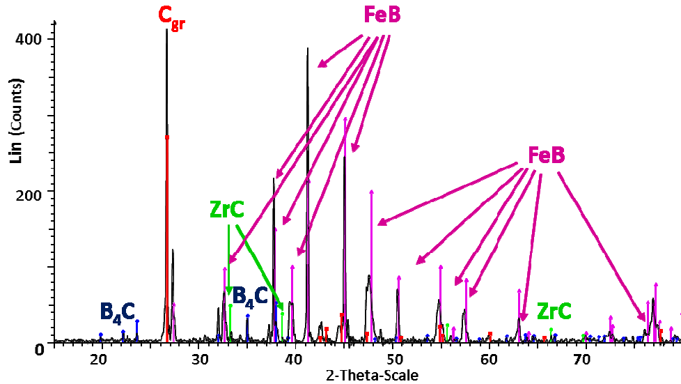
Figure 6-4 : Spectre DRX de la charge fondue Acier inoxydable – \text{B}_4\text{C} après le refroidissement
