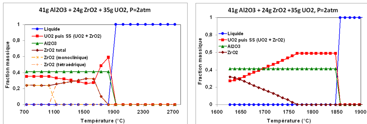
Figure 4-15 : L'évolution des fractions massiques du système (35% \text{UO}_2 + 41\%\text{Al}_2\text{O}_3 + 24\%\text{ZrO}_2 ) à l'équilibre, à 2 \cdot 10^5 Pa, en fonction de la température du milieu (a) pas de température = 100°C, (b) pas de température = 10°C
