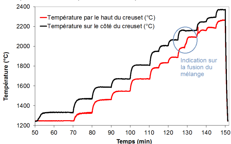
Figure 6-28 : Courbe de températures (température en fonction de la durée de l'essai) enregistrée au cours de l'essai CORSICCA 2_Eu_1e relatif à l'interaction 25% \text{UO}_2 – 75% \text{Eu}_2\text{O}_3 (composition massique) dans un creuset en tungstène, dans le but de retrouver l'eutectique reporté par L.N. Grossman et al. La température maximale de l'essai était de 2370 \pm 35^\circ\text{C} . Aucun palier de solidification n'est visible au refroidissement.
