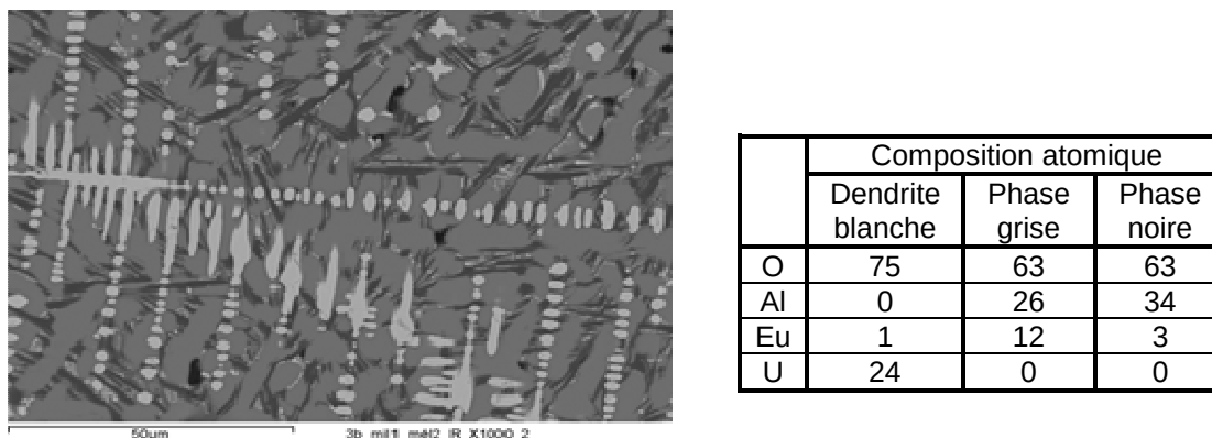
Figure 6-43 : Micrographie MEB accompagnée de l'analyse par EDX du mélange 30% \text{UO}_2 – 33% \text{Al}_2\text{O}_3 – 37% \text{Eu}_2\text{O}_3 en proportions massiques après le chauffage jusqu'à 1870°C et refroidissement dans un creuset en \text{UO}_2
