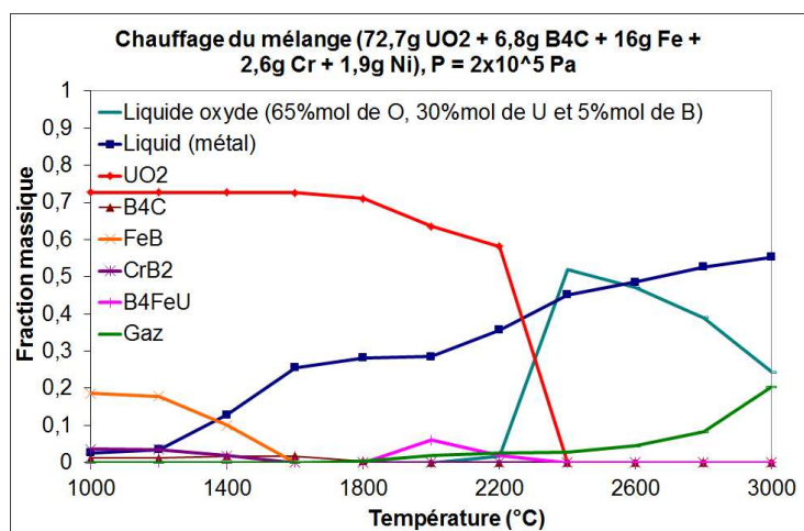
Figure 4-9: L'évolution des fractions massiques du système (6,8% \text{B}_{11}\text{C}_3 – 72,7% \text{mUO}_2 – 16% \text{mFe} – 2,6% \text{mCr} – 1,9% \text{mNi} ) à l'équilibre, à 2 \cdot 10^5 Pa, en fonction de la température du milieu
