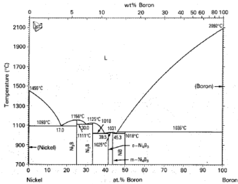
Figure 3-16: Diagramme de phases du système Ni – B [3.48]
