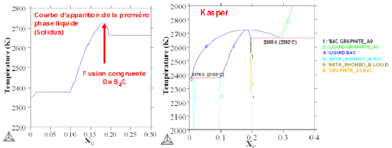
Figure 3-10: Diagramme de phases du système B – C selon Kasper (en mol) [3.37]
