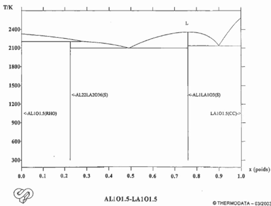
Figure A4-8 : Diagramme de phases \text{Al}_2\text{O}_3 – \text{La}_2\text{O}_3 contenu dans la base de données Nuclea – Critère de qualité = parfait
