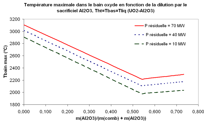
Figure 4-28 : Température maximale dans le bain oxyde en fonction de la dilution par le sacrificiel \text{Al}_2\text{O}_3 , dans le cas où une croûte se formerait à la surface supérieure du bain
