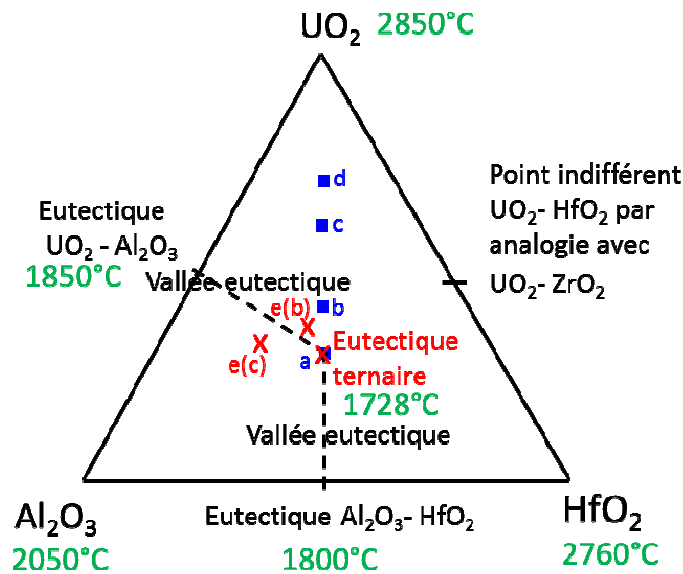
Figure 6-52: Triangle de compositions (compositions massiques) relatif au système ternaire \text{UO}_2 - \text{Al}_2\text{O}_3 - \text{HfO}_2 montrant l'eutectique ternaire et les vallées eutectiques. Les compositions initiales des mélanges initiaux CORSICCA 2_Al_x sont représentées par des carrés bleus. Les compositions eutectiques correspondant à ces essais sont représentées par des croix rouges. L'eutectique relatif à l'essai d n'a pas pu être mesuré.
