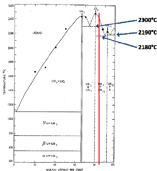
Figure 6-12 : Diagramme de phases U – B avec l'indication de la composition du mélange expérimental lors de l'essai d'interaction \text{UO}_2 – \text{B}_4\text{C} (en considérant que C et O ne sont plus présents dans le mélange car volatilisés sous forme de CO)
