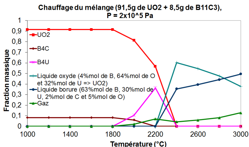
Figure 4-3: L'évolution des fractions massiques du système (8,5% B_{11}C_3 – 91,5% UO_2 ) à l'équilibre, à 2 \cdot 10^5 Pa, en fonction de la température du milieu
