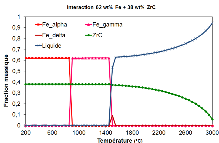
Figure A16-4 : Calcul GEMINI2 + NUCLEA_08 simulant l'interaction 62 wt% Fe + 38 wt% ZrC. Sur la courbe sont tracées les fractions massiques des produits présents en fonction de la température.
