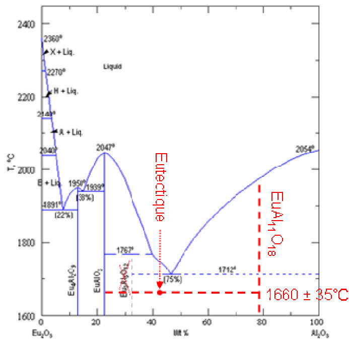
Figure 6-56 : Diagramme de phases binaire \text{Eu}_2\text{O}_3 – \text{Al}_2\text{O}_3 modifié à partir des essais CORSICCA 2_Eu_2
