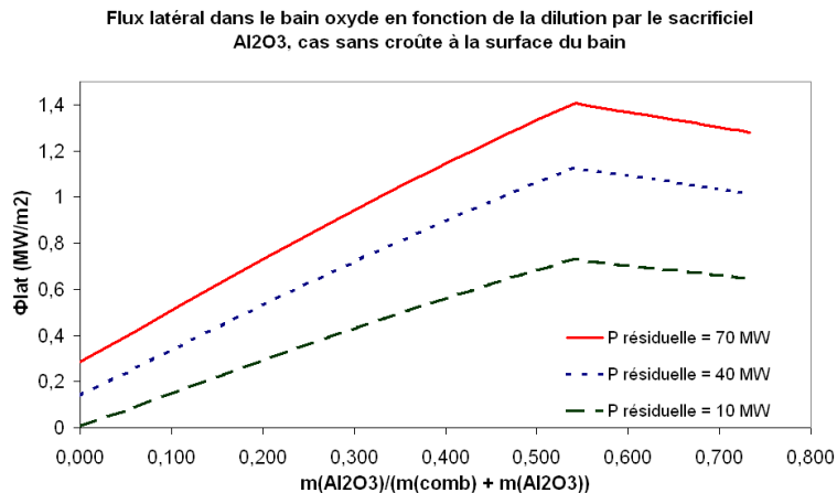
Figure A12-2 : Flux latéral dans le bain oxyde en fonction de la dilution par le sacrificiel \text{Al}_2\text{O}_3 dans le cas de la non formation d'une croûte stable à la surface du bain
