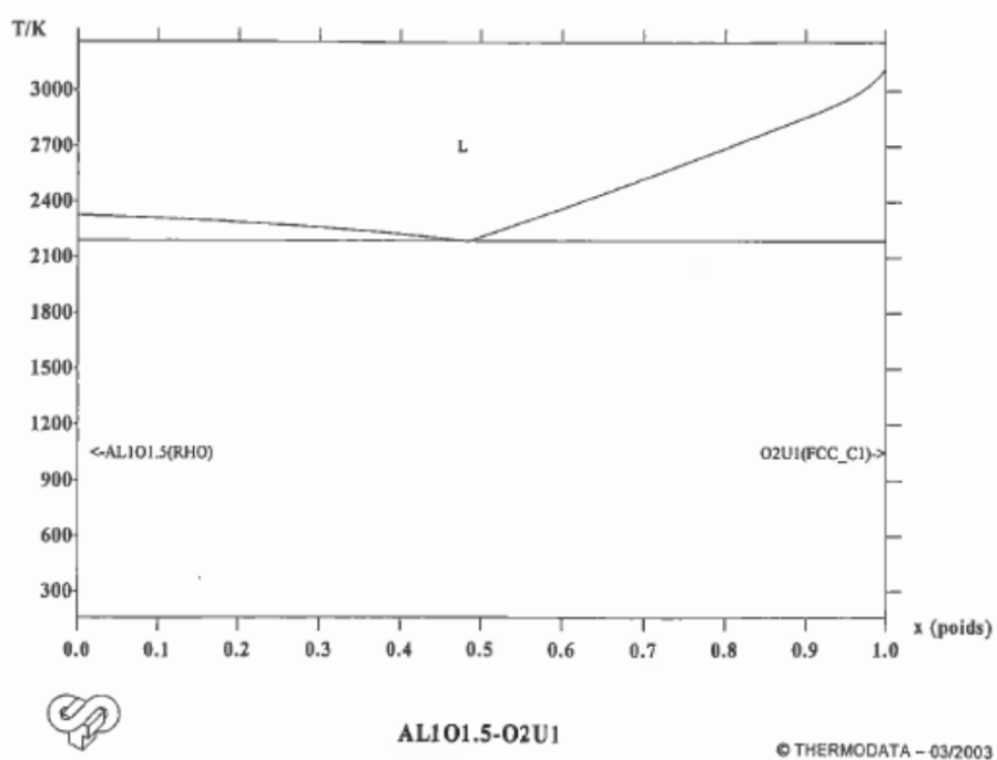
Figure A4-6 : Diagramme de phases \text{Al}_2\text{O}_3 – \text{UO}_2 contenu dans la base de données Nuclea – Critère de qualité = acceptable
