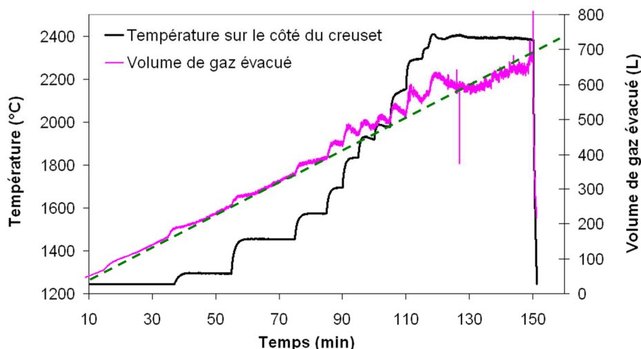
Figure 6-19 : Courbe de température (température en fonction de la durée de l'essai) enregistrée au cours de l'essai CORSICCA 1_2e relatif à l'interaction \text{UO}_2 – \text{B}_4\text{C} dans un creuset en tungstène. A ce tracé de température est superposé le volume des gaz évacués du four VITI. Un dégagement gazeux plus important est observé à partir de 1700^\circ\text{C} environ. Ceci peut être attribué au dégagement gazeux dû à l'interaction \text{UO}_2 – \text{B}_4\text{C} .
