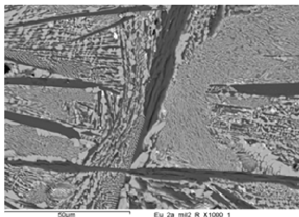
Figure 6-36 : Micrographie MEB accompagnée de l'analyse par EDX du mélange initial 53% \text{Eu}_2\text{O}_3 + 47% \text{Al}_2\text{O}_3 en proportions massiques après le chauffage jusqu'à 2200°C et refroidissement dans un creuset en tungstène
