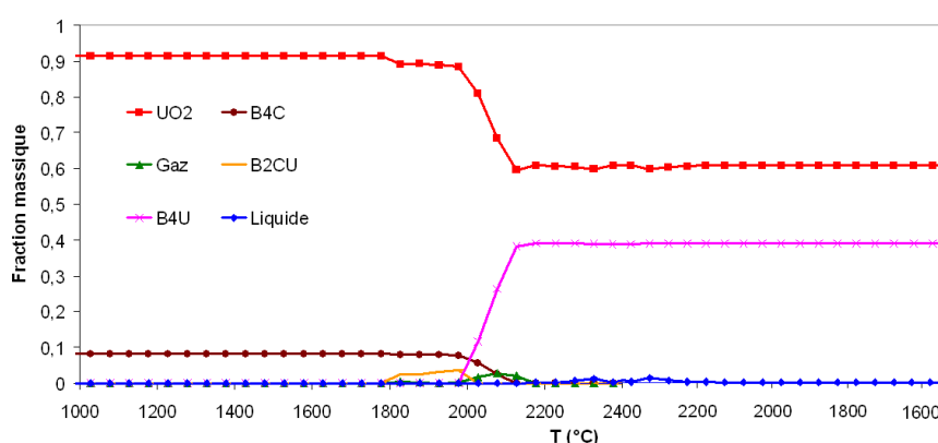
Figure 6-9 : Calcul GEMINI2 + NUCLEA_08 reproduisant l'essai d'interaction de composition massique 91,5% \text{UO}_2 + 8,5% \text{B}_4\text{C} qui simule la fusion d'un assemblage avec un SAC sans acier. Sur la courbe sont tracées les fractions massiques des produits présents en fonction de la température, au cours du chauffage jusqu'à 2400°C puis du refroidissement.
