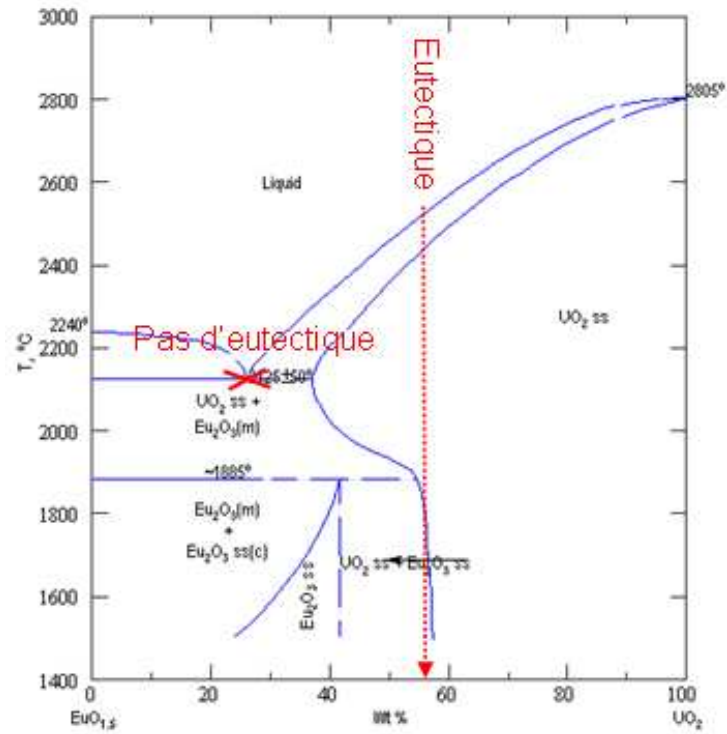
Figure 6-55 : Diagramme de phases \text{Eu}_2\text{O}_3 – \text{UO}_2 modifié après les essais CORSICCA 2_Eu_1
