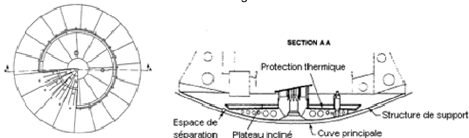
Figure 2-9: Schéma intégral du récupérateur du Superphénix en fond de cuve
