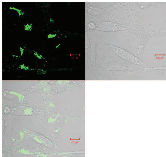
Glycolyl
