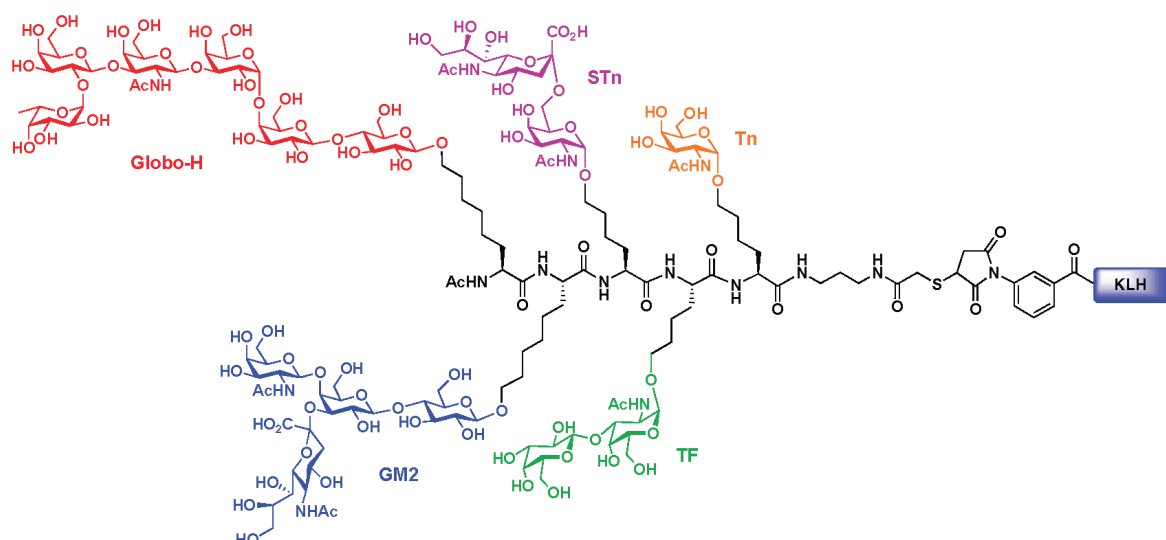
Figure 16. Exemple de structure d'un vaccin multi-antigénique (Zhu et al., 2009).
