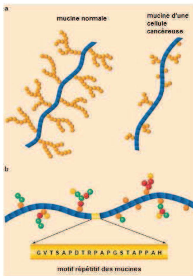
Figure 9. a Comparaison de la glycosylation de MUC1 d'une cellule normale (à gauche) avec celle d'une cellule tumorale (à droite) b Représentation de MUC1 et de sa séquence répétitive d'acides aminés (Agrawal et al. , 1998).
