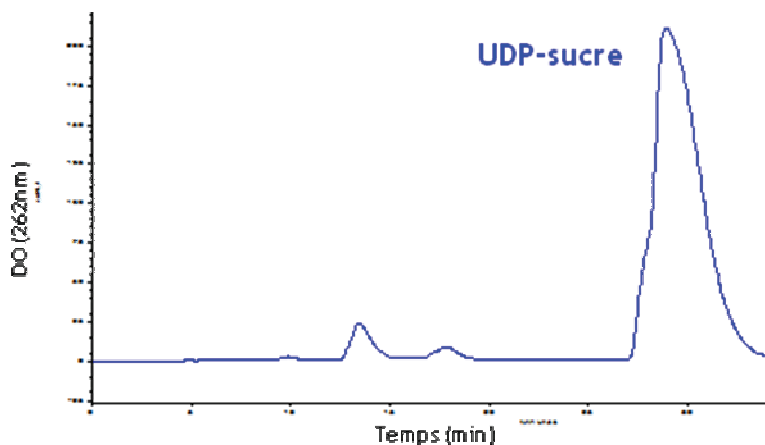
Figure 35. Profil HPLC de sortie des UDP-sucre (DO à 262 nm).
