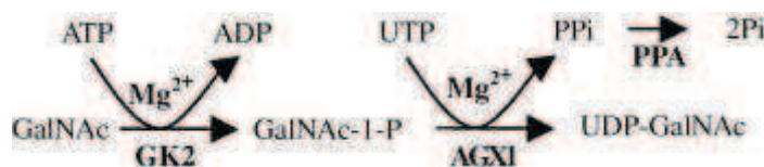
Figure 25. Schéma de la synthèse enzymatique d'UDP-GalNAc.
