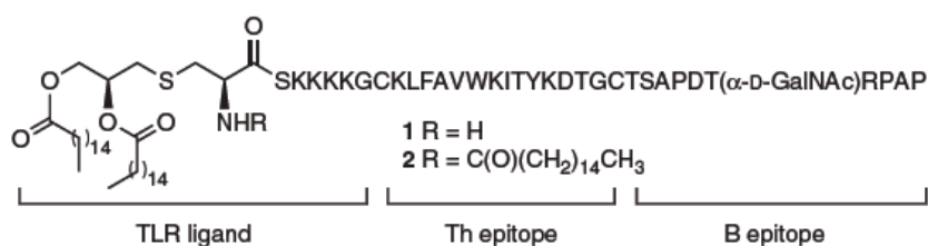
Figure 17. Structure du vaccin synthétique (Ingale et al. , 2007).
