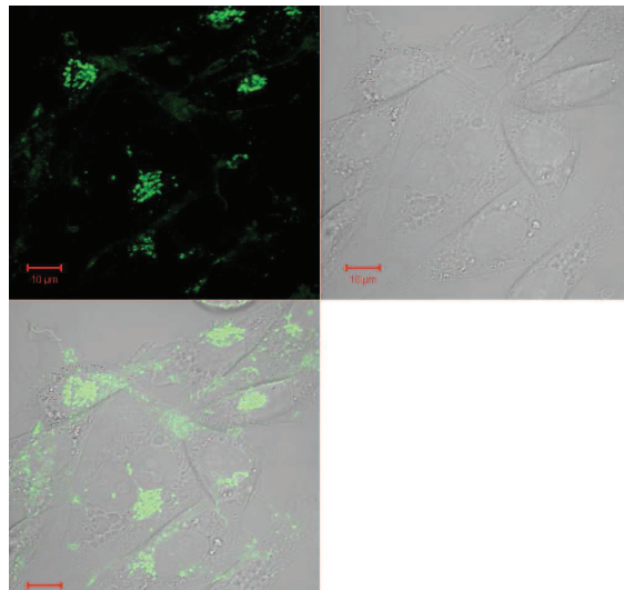
GalNAc
