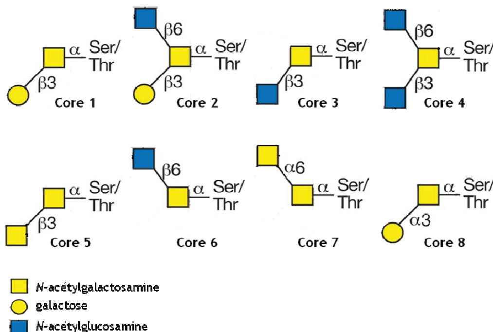
Figure 4. Représentation des différentes structures core des O-glycanes de type mucine (Varki et al., 2009).
