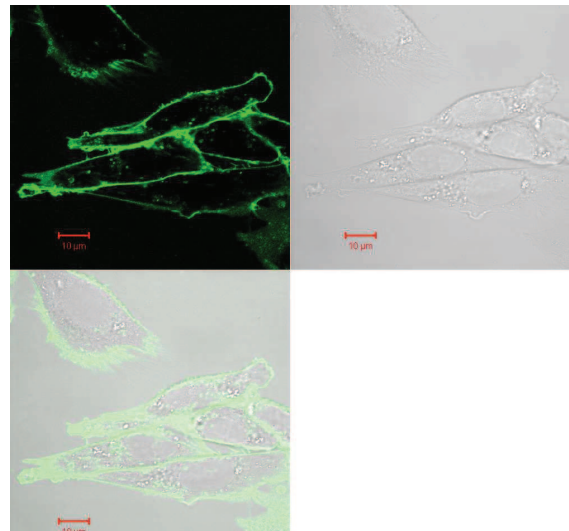
GalNAc
