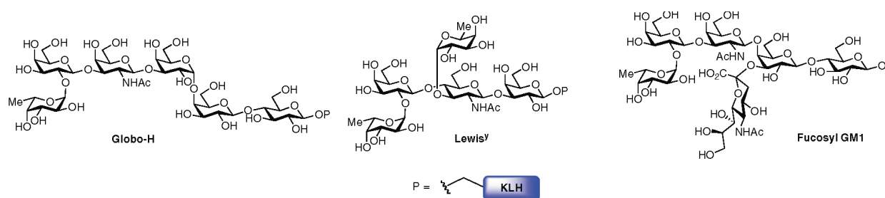
Figure 15. Représentation des antigènes tumoraux utilisés par Danishefsky et son équipe (Zhu et al. , 2009).
