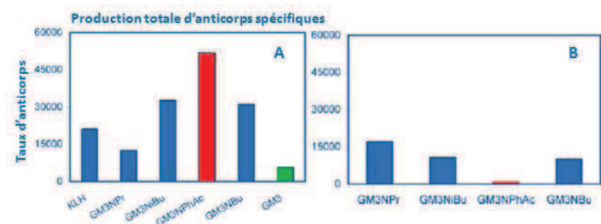
Figure 19. Analyse des titres d'anticorps présents dans les anti-sérums après immunisation par ELISA contre les GM3 modifiés respectifs (A) et contre le GM3 naturel (B).
