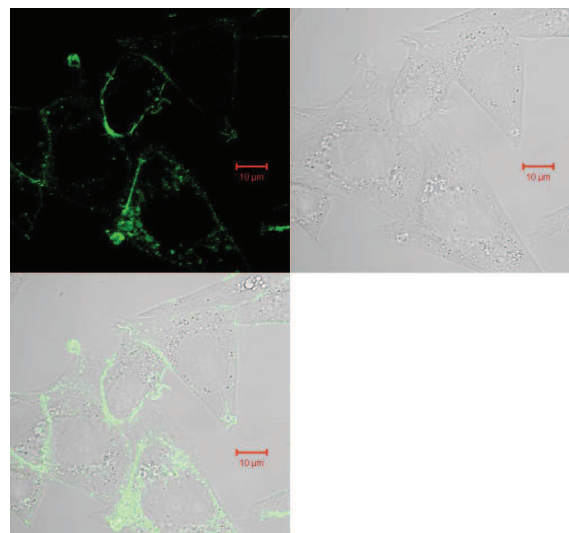
Glycolyl
