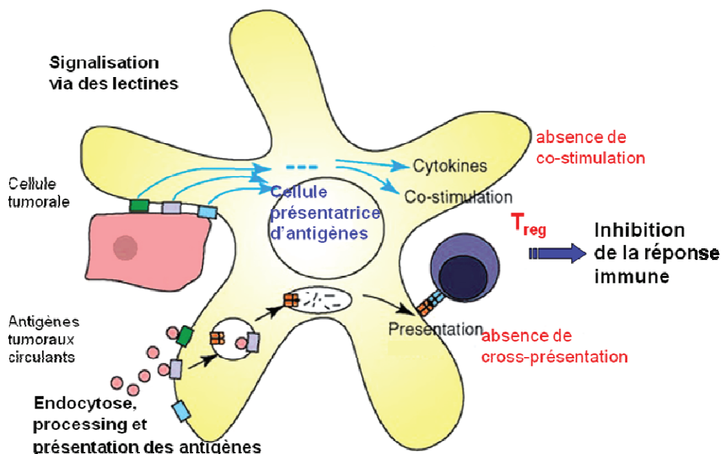
Figure 22. Représentation schématique de la reconnaissance d'une tumeur par une cellule dendritique via des lectines (schéma d'après Aarnoudse et al. , 2006).
