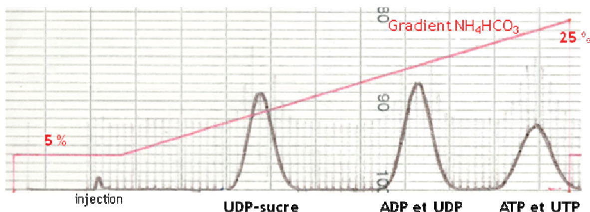
Figure 34. Profil de purification des UDP-sucres par gel échangeur d'anions (DO à 254 nm).
