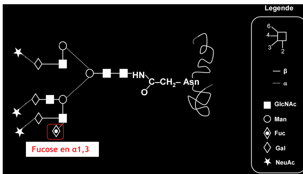
Figure 8. Représentation d'une forme tri-antennée présentant l'épitope sLe x .
