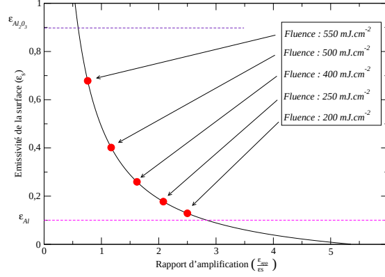
FIG. 3.10: Évolution de l'émissivité de la surface d'un échantillon d'aluminium en fonction de la fluence laser pour l'échantillon d'aluminium
