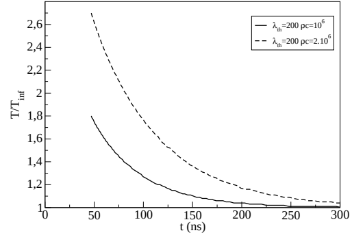
(b) Influence de la capacité calorifique volumique
