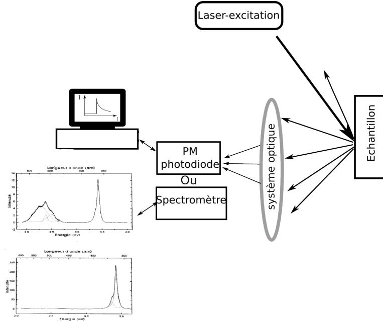
FIG. 2.1: Schéma représentant des systèmes de détection du signal de photoluminescence
