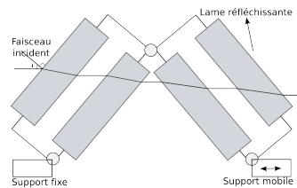
FIG. 3.3: Schéma de l'atténuateur
