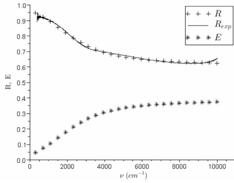
(a) Mesure expérimentale de la réflectivité de l'échantillon Ti/Si mésoporeux comparée aux valeurs théoriques attendues
