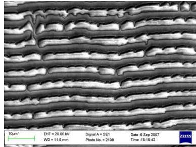
FIG. 1.5: Image MEB des ripples de surface d'après Gedvilas et al. [1]
