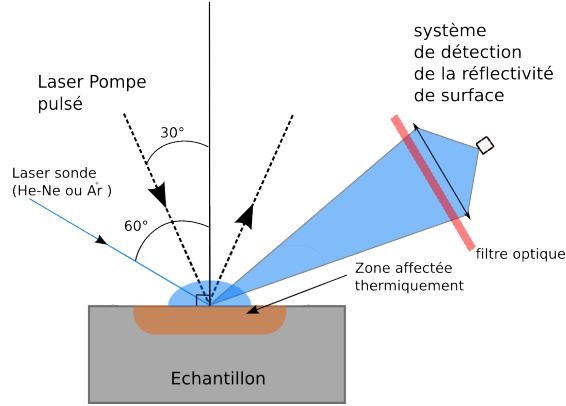
FIG. 3.19: Configuration schématique pour la méthode RRT
