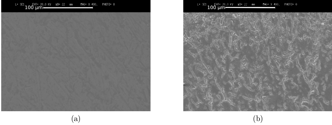
FIG. 3.11: Images MEB de l'échantillon d'aluminium avant (a) et après irradiation par laser (b)
