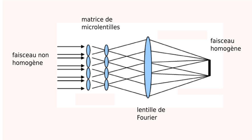
FIG. 3.1: Configuration optique de l'homogénéiseur
