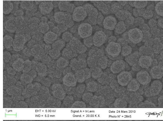
FIG. 5.12: Image MEB d'un dépôt de Ti de 600 nm d'épaisseur sur un tapis de NTC, vue de dessus
