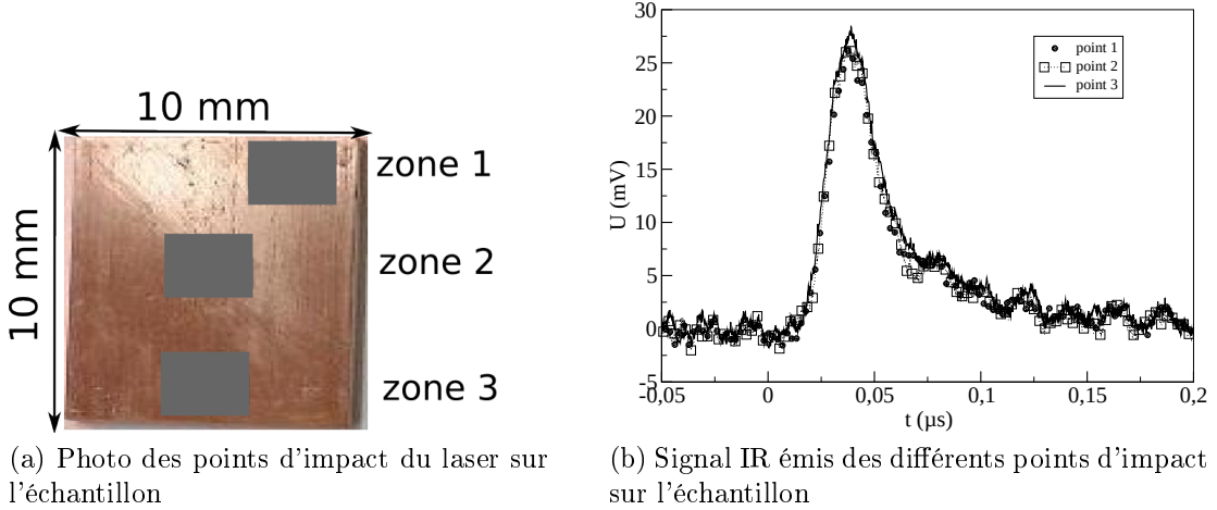
FIG. 3.18: Test de sensibilité de la méthode PIR à la position de l'impact laser
