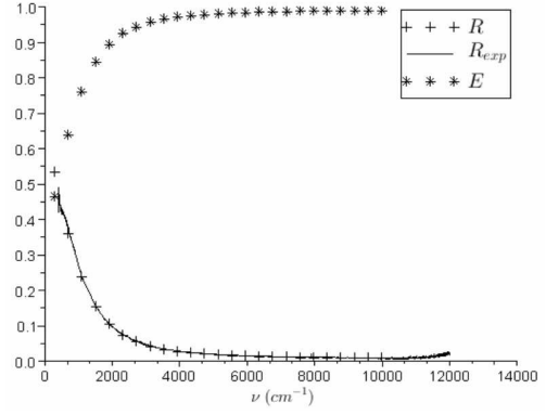
(b) Mesure expérimentale de la réflectivité de l'échantillon Ti/NTC comparée aux valeurs théoriques attendues
