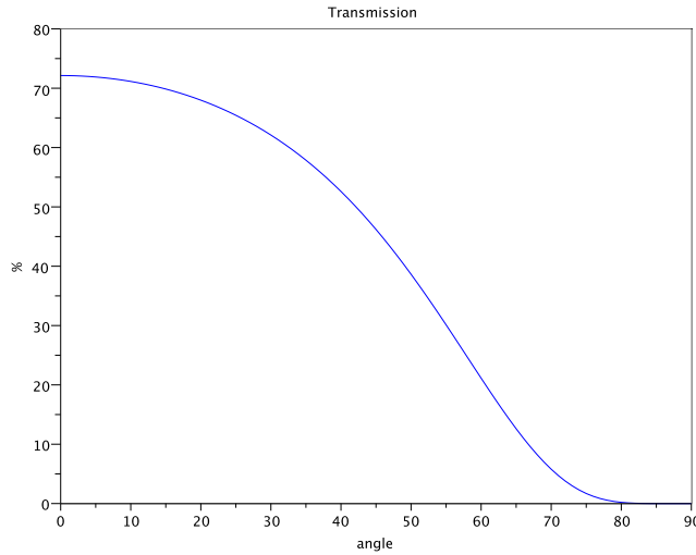
FIG. 3.4: Transmission du faisceau laser UV à travers l'atténuateur en fonction de l'angle d'incidence
