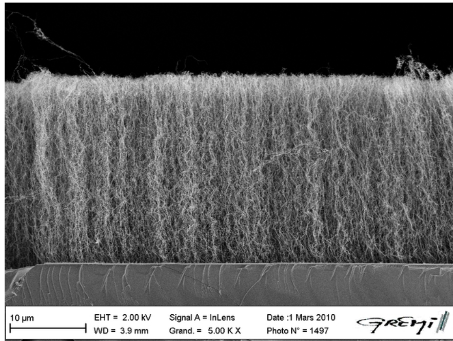
FIG. 5.8: Image MEB d'un tapis de NTC
