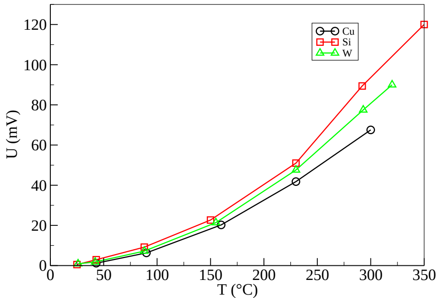
FIG. 3.15: Courbes d'étalonnage pour des échantillons massifs
