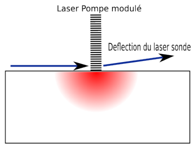
FIG. 2.7: Schéma simplifié de la méthode mirage
