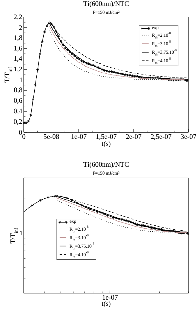
FIG. 5.21: Simulations de la relaxation temporelle du signal thermique normalisé ( T/T_{\text{inf}} ) pour différentes valeurs de R_{th} confrontées aux mesures expérimentales ( R_{th} en K \cdot m^2 \cdot W^{-1} )
