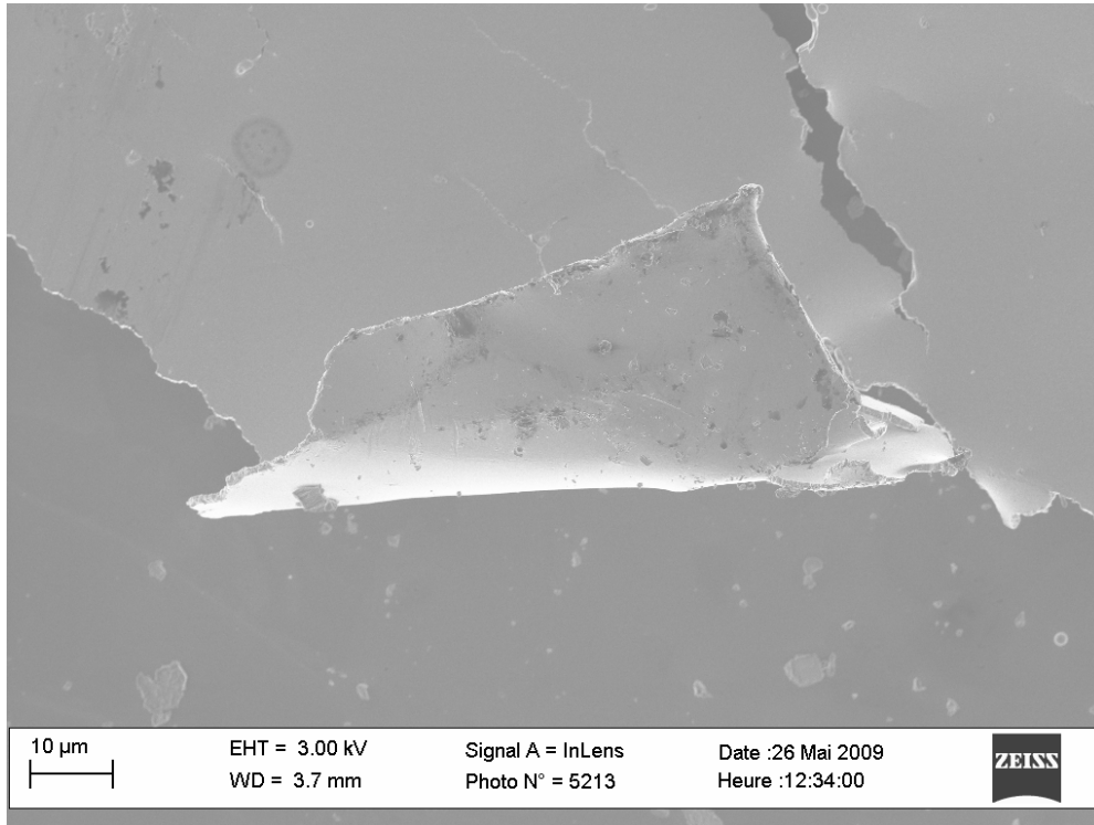
FIG. 4.2: Image MEB d'une couche mince de cuivre décollée du substrat de verre
