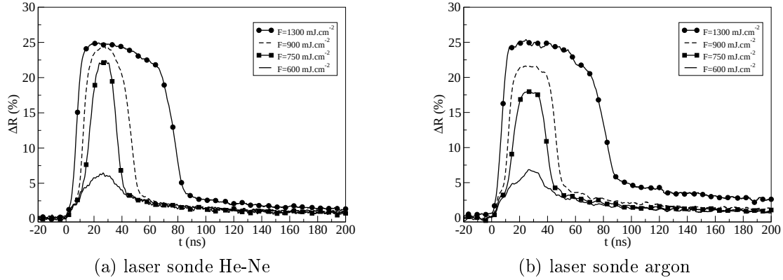
FIG. 4.11: Variations de la réflectivité de surface du silicium soumis à différentes fluences laser
