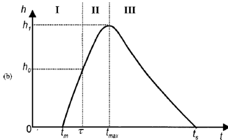
FIG. 1.4: Les variations de la profondeur de fusion en fonction du temps.
