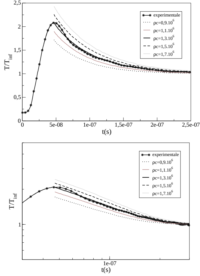
FIG. 5.20: Simulations de la relaxation temporelle du signal thermique normalisée ( T/T_{\text{inf}} ) confrontées au modèle analytique pour différentes valeurs de \rho c ( J \cdot K^{-1} \cdot m^{-3} )
