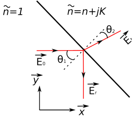
FIG. 1.1: Schéma simplifié de la propagation d'une onde électromagnétique à l'interface entre deux milieux
