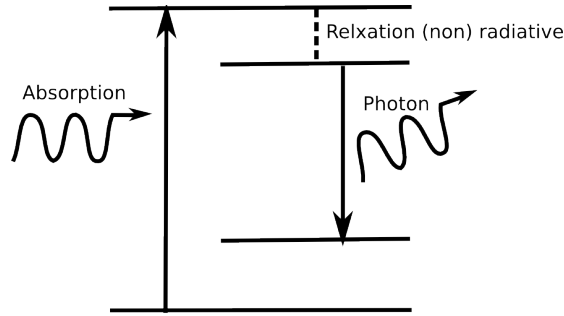
FIG. 1.3: Principe de la photoluminescence
