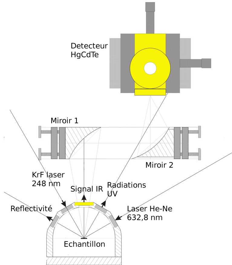
FIG. 3.13: Illustration de la configuration de la méthode PIR
