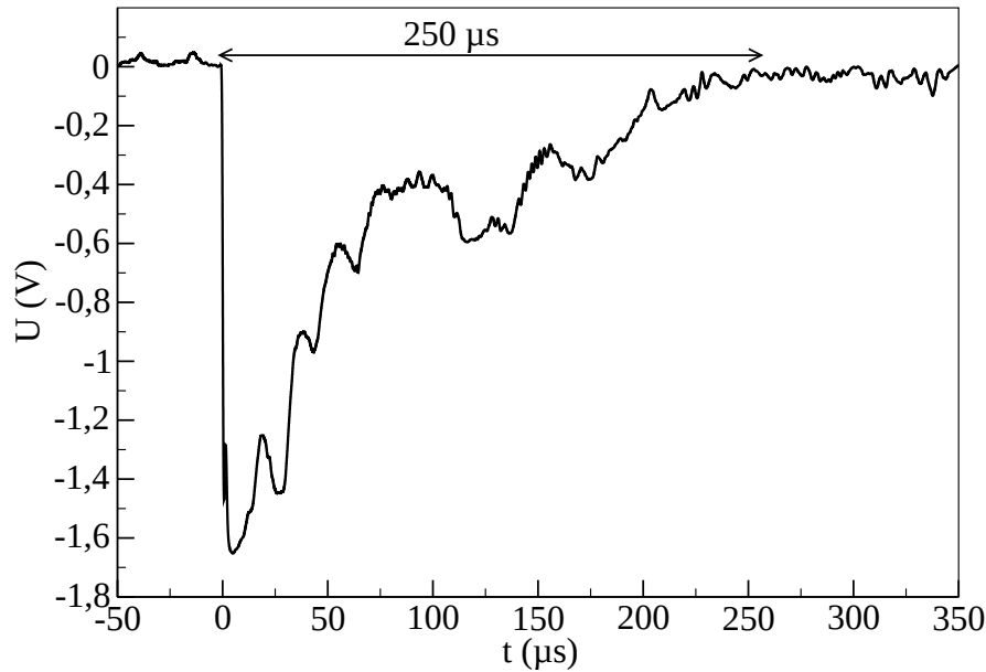
FIG. 4.14: Variations temporelles de la réflectivité de surface du titane après un tir laser dont la fluence est supérieure à 1500 \text{ mJ.cm}^{-2}
