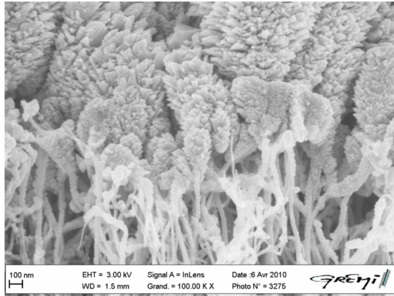
FIG. 5.19: Image MEB de l'interface entre le dépôt de Ti et le tapis de NTC
