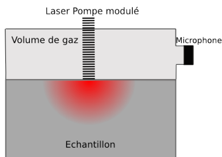
FIG. 2.8: Schéma simplifié de la spectroscopie photo-acoustique
