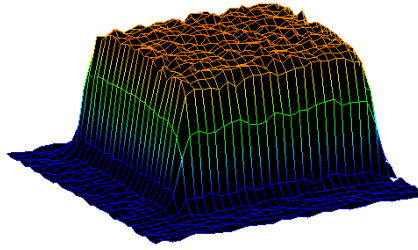
FIG. 3.2: Distribution spatiale de l'énergie laser après homogénéisation
