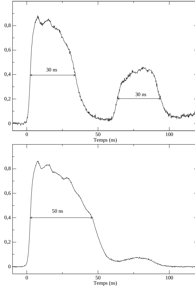
FIG. 5.28: Superposition temporelle des deux impulsions laser (KrF) décalées
