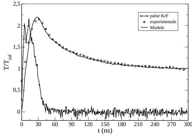
FIG. 5.3: Variations temporelles expérimentales et modélisées de la température de surface pour une impulsion laser KrF
