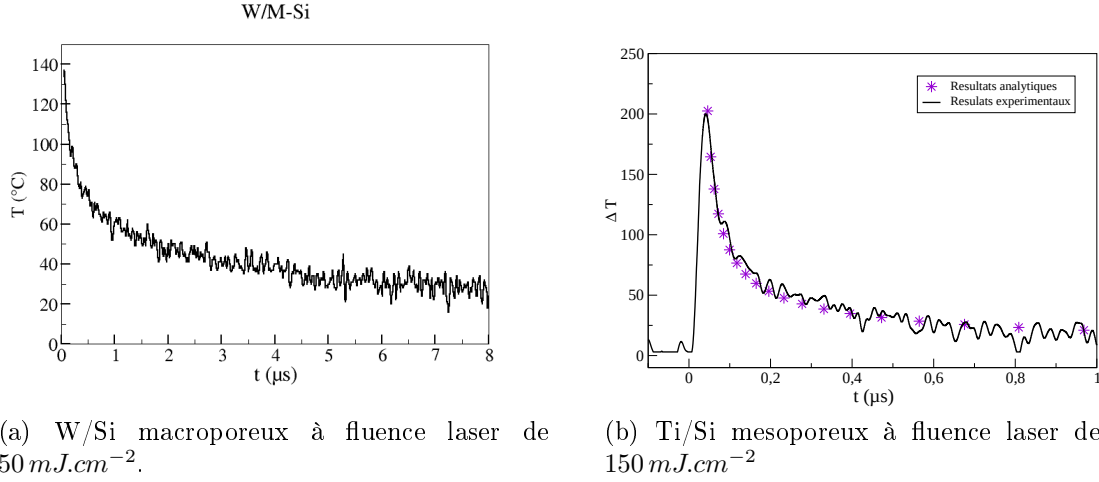
FIG. 5.25: Variations temporelles de la température de surface
