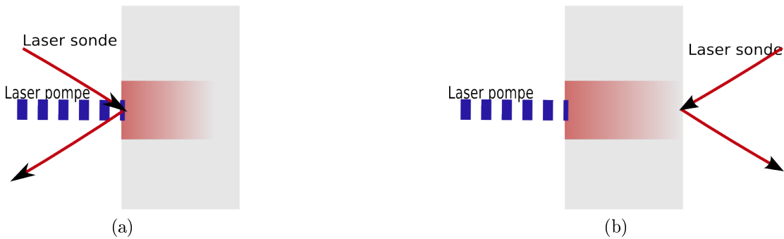
FIG. 2.6: Représentations schématiques de la méthode de mesure de la réflectivité résolue en temps en face avant (a) et en face arrière (b)
