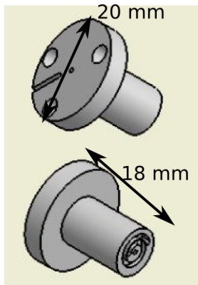
(a) vue schématique de l'élément chauffant
