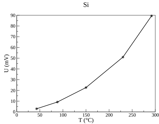
FIG. 5.4: Courbe d'étalonnage du détecteur IR pour un échantillon de silicium cristallin
