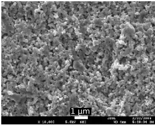
(a) Images MEB de la surface du silicium macroporeux
