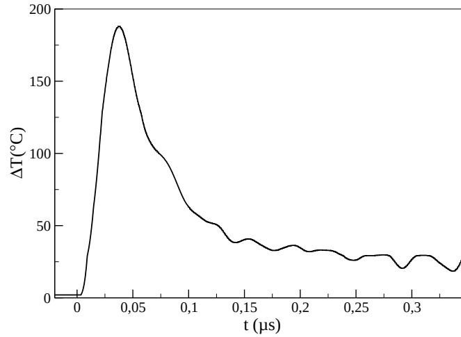
FIG. 5.6: Relaxation temporelle de la température de surface de l'échantillon Ti/Si après irradiation laser
