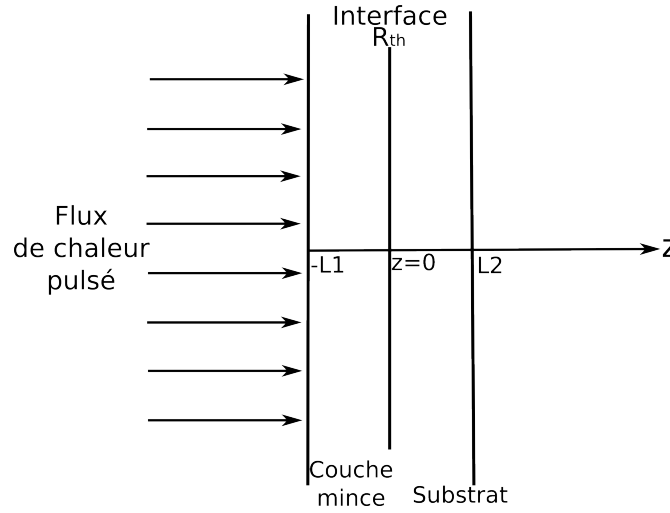
FIG. 5.1: Schéma du modèle de diffusion thermique à deux couches
