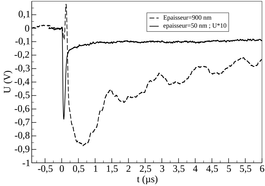
FIG. 4.6: Variations temporelles de la réflectivité de surface pour un dépôt de cuivre de 50 nm et 900 nm sur silicium pour une fluence laser de 400 \text{ mJ.cm}^{-2}
