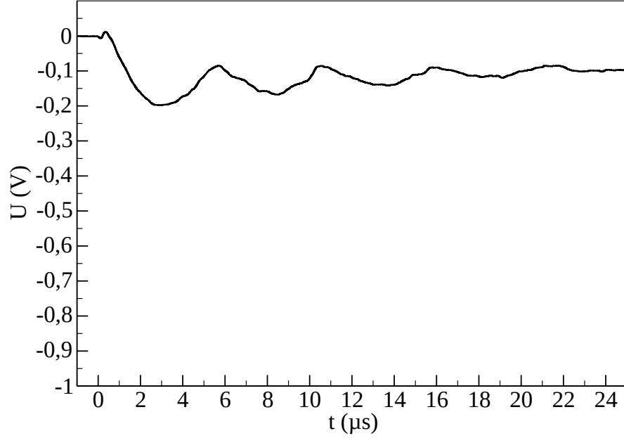
FIG. 4.5: Variations temporelles de la réflectivité de surface pour un dépôt de cuivre de 5 \mu m d'épaisseur sur verre irradié avec une fluence laser de 250 mJ.cm^{-2}
