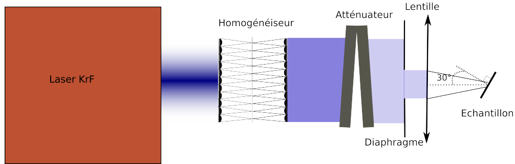
FIG. 3.6: Schéma représentant le trajet du faisceau laser KrF depuis la sortie du laser jusqu'à l'échantillon
