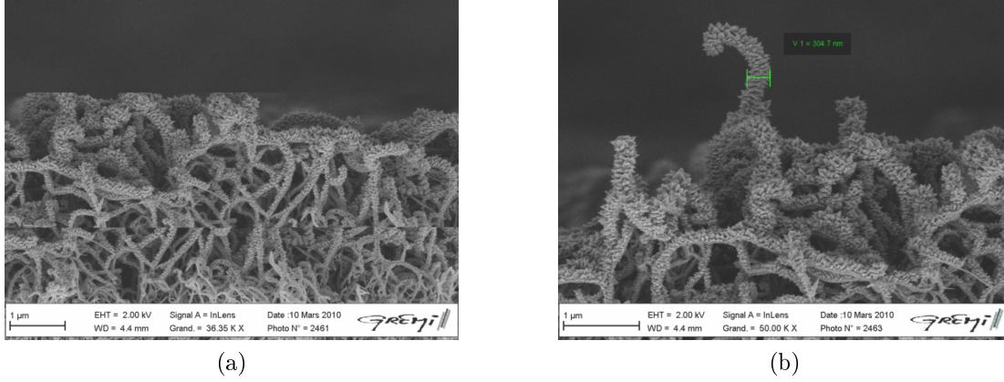
FIG. 5.11: Images MEB d'un dépôt de Ti de 300 nm sur un tapis de NTC
