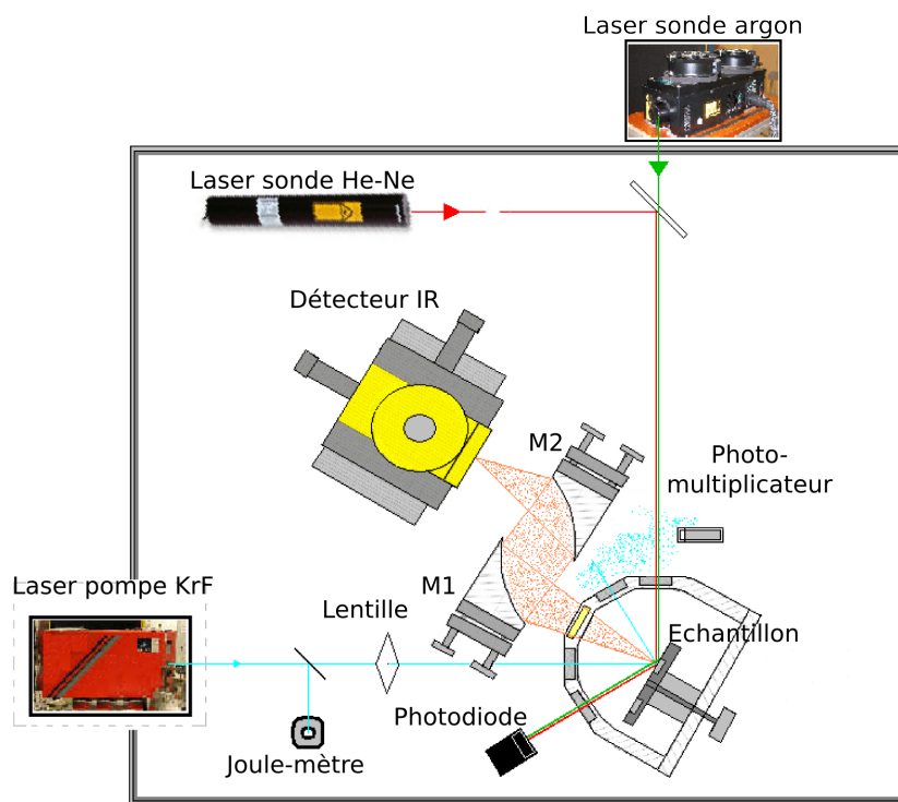
FIG. 3.20: Représentation schématique du système expérimental complet : RRT et PIR
