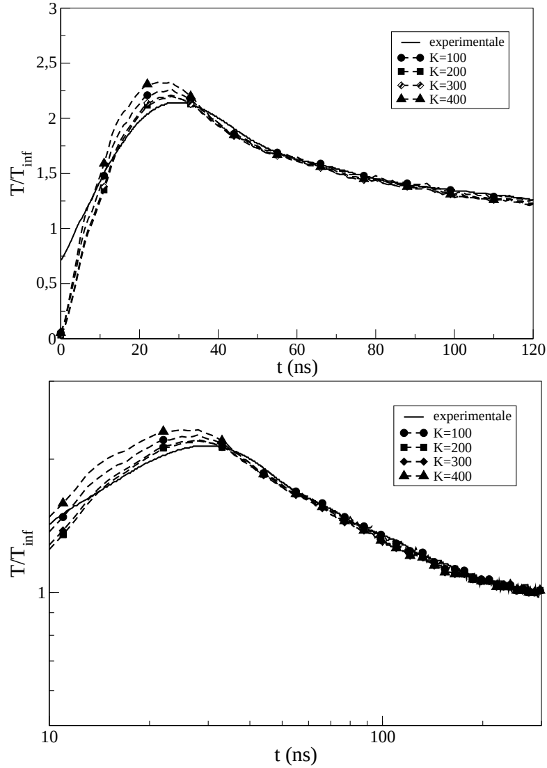
FIG. 5.23: Simulations de l'évolution temporelle du signal thermique normalisé ( T/T_{\text{inf}} ) pour différentes valeurs de la conductivité thermique du tapis de NTCs confrontés aux mesures expérimentales pour une distribution temporelle d'énergie correspondant à celle du laser KrF. ( \lambda_{th} en W.m^{-1}.K^{-1} , \rho c_p = 10^6 J \cdot K^{-1} \cdot m^{-3} et R_{th} = 3,75.10^{-8} K.m^2.W^{-1} )
