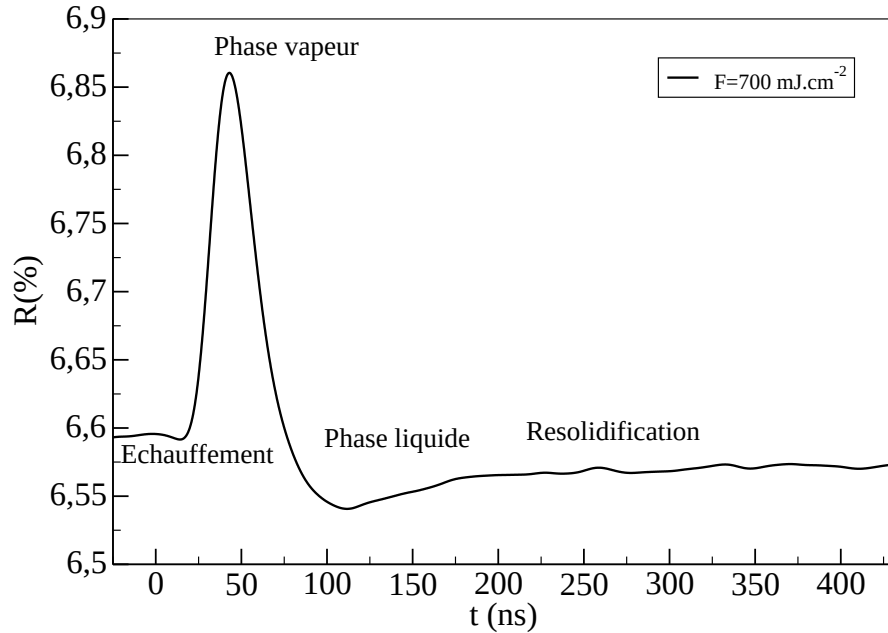
FIG. 4.12: Variations temporelles de la réflectivité de surface du titane à fluence laser 700 \text{ mJ.cm}^{-2}
