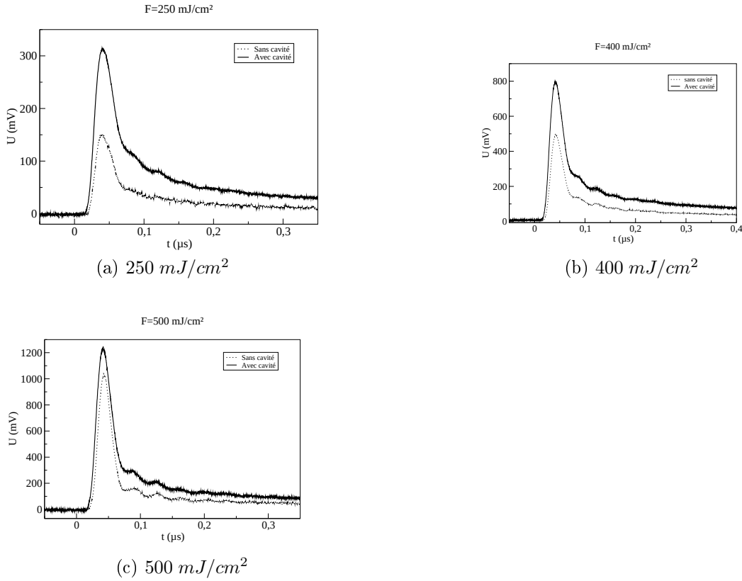
FIG. 3.9: Effet de la sphère sur le signal IR
