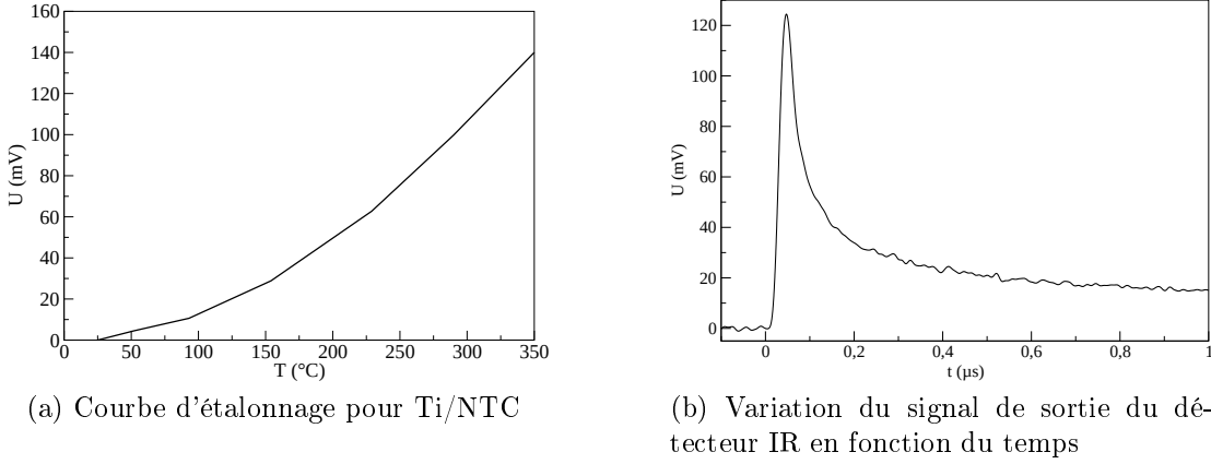
FIG. 5.17: courbe d'étalonnage (a) et signal IR émis (b) de l'échantillon Ti/NTC
