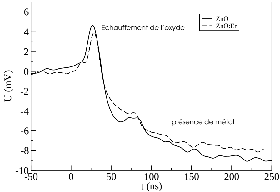
FIG. 4.9: Signal de réflectivité émis d'un échantillon de ZnO et ZnO :Er
