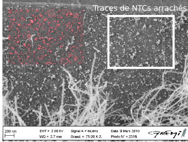
FIG. 5.26: Image MEB d'un tapis de NTCs arrachés sur un substrat de Si_3N_4
