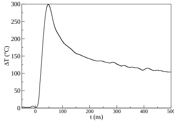
FIG. 5.18: Variation de la température de surface du Ti/NTC après un tir laser à 150 \text{ mJ.cm}^{-2}
