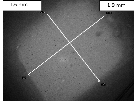
FIG. 3.5: Observation MEB de l'impact laser sur un échantillon de silicium
