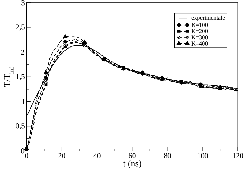
FIG. 5.22: Comparaison entre le signal expérimental de T/T_{inf} en fonction du temps et le modèle à différentes valeurs de \lambda_{th} en W.m^{-1}.K^{-1}
