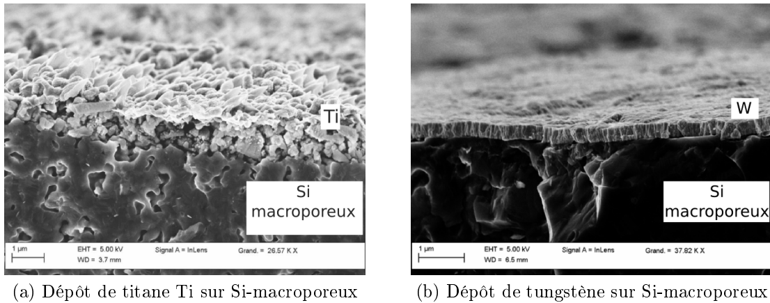
FIG. 5.15: Dépôt PVD sur substrat de Si macroporeux
