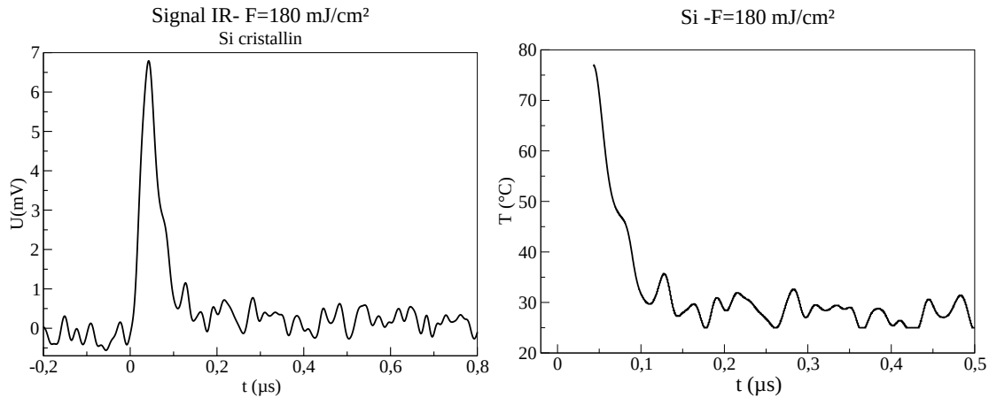
FIG. 5.5: A gauche : Signal IR émis de la surface du Si après irradiation par laser à fluence de 180 \text{ mJ} \cdot \text{cm}^{-2} . A droite : Relaxation temporelle de la température de surface du Si
