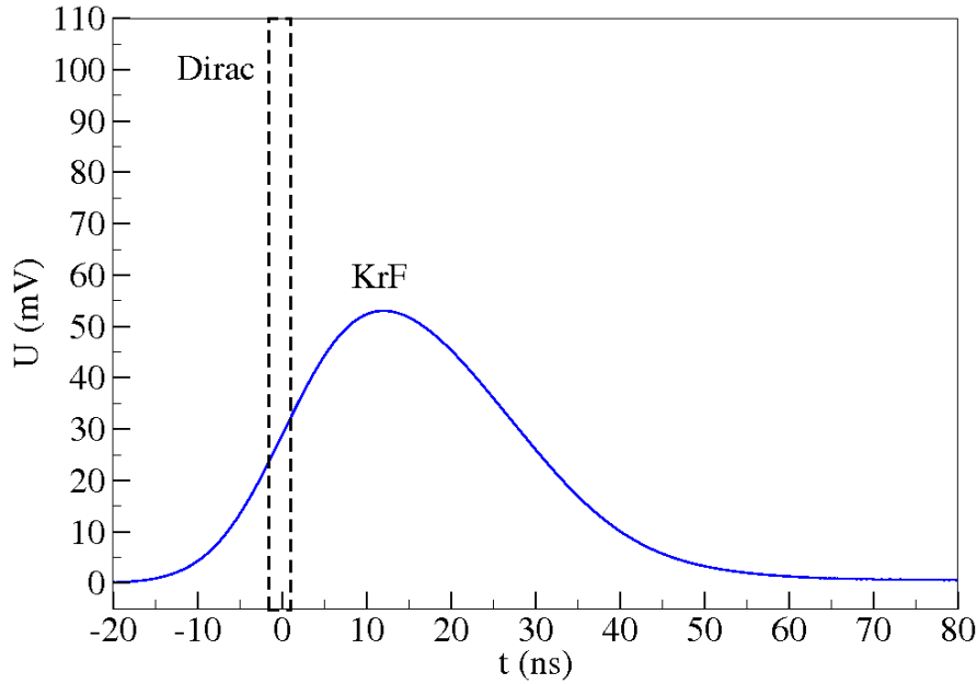
FIG. 5.2: Évolution temporelle de l'impulsion laser comparée à une impulsion de Dirac
