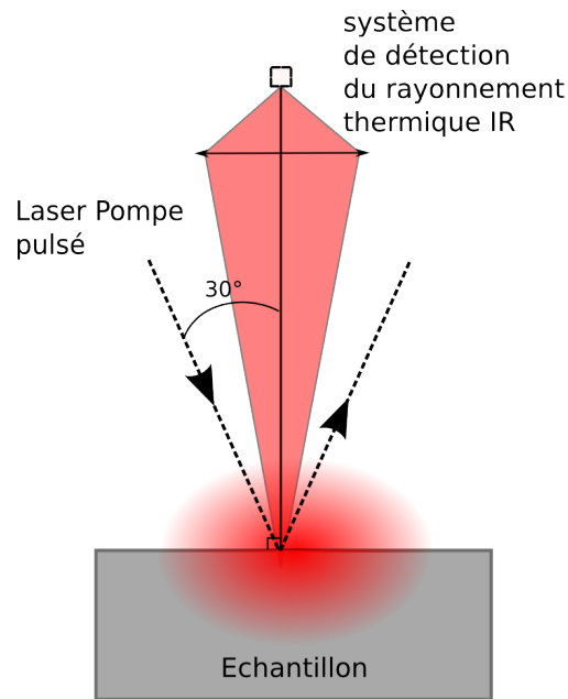
FIG. 2.4: Schéma simplifié de la méthode de radiométrie photothermique
