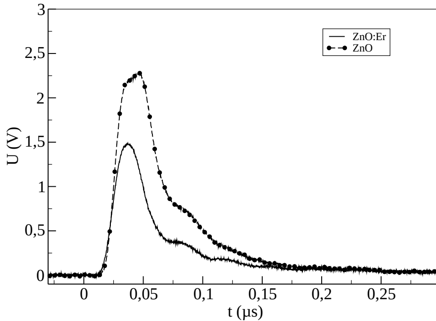
FIG. 4.8: Comparaison des signaux IR émis des échantillons de ZnO et ZnO :Er
