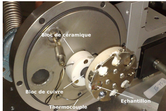
(b) photo de la résistance électrique, du thermocouple et de la position de l'échantillon par rapport à l'élément chauffant
