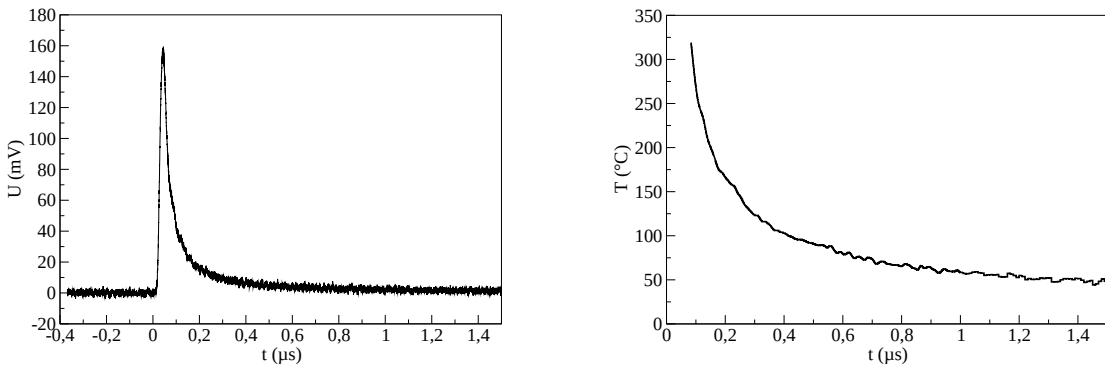
(a) Variation temporelle de la tension de sortie du détecteur U(t) pour un échantillon de tungstène exposé à une fluence laser de 150\text{ mJ/cm}^2
