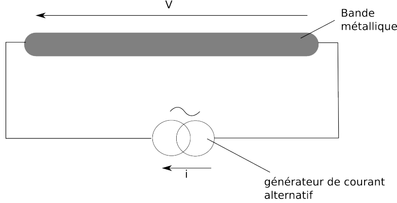
FIG. 2.3: Schéma de la bande métallique utilisée pour la méthode 3\omega . Généralement, la largeur est de quelques dizaines de micromètres, la hauteur de quelques centaines de nanomètres et la longueur fait plusieurs millimètres
