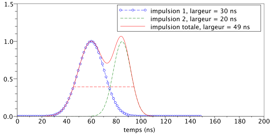
FIG. 5.27: Signal théorique de superposition temporelle des deux impulsions laser (KrF)
