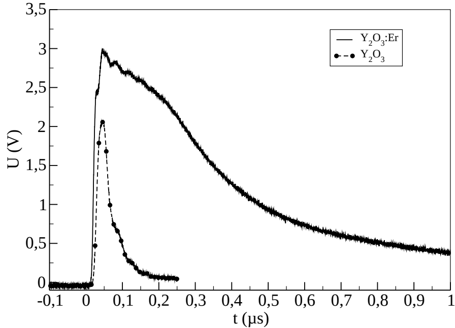
FIG. 4.7: Signaux IR émis de deux échantillons : Y_2O_3 et Y_2O_3 :Er pour une fluence laser KrF de 400 mJ.cm^2
