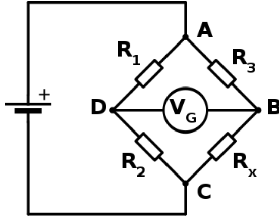
FIG. 2.2: Pont de Wheatstone ( R_x représente la résistance de la bande métallique)
