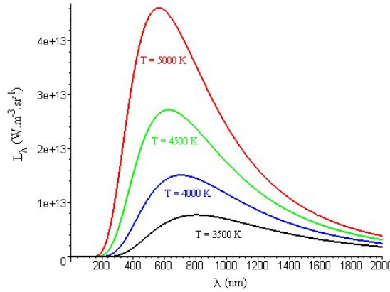
FIG. 1.2: Illustration de la loi de Wien et Planck à différentes températures
