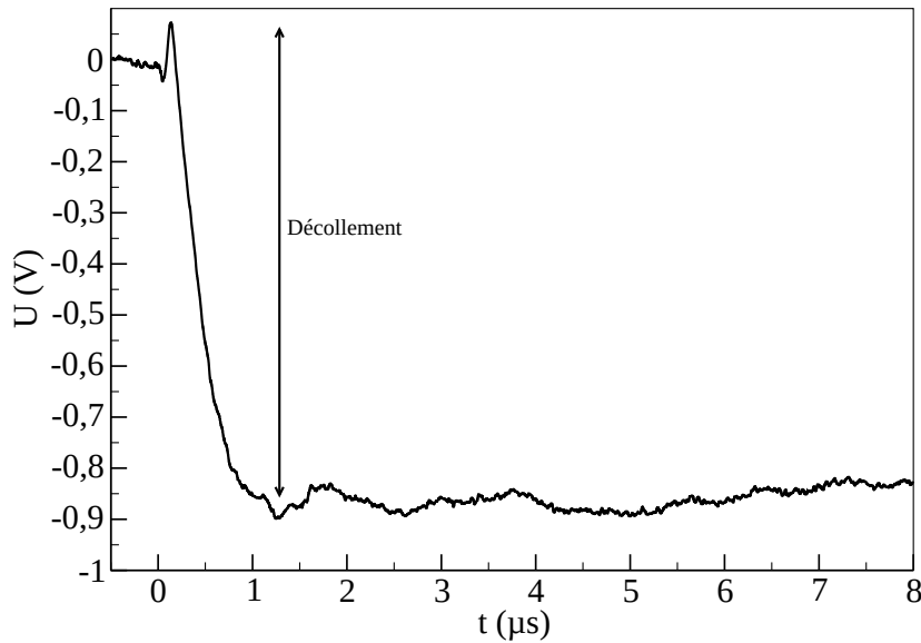
FIG. 4.1: Signal de réflectivité associé au décollement de la couche de cuivre sur un substrat de verre
