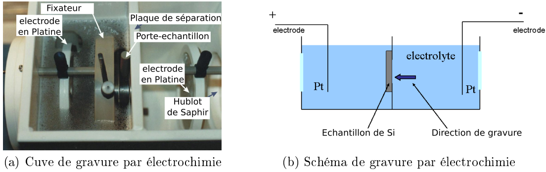
FIG. 5.10: Système et schéma expérimental pour la gravure par électrochimie
