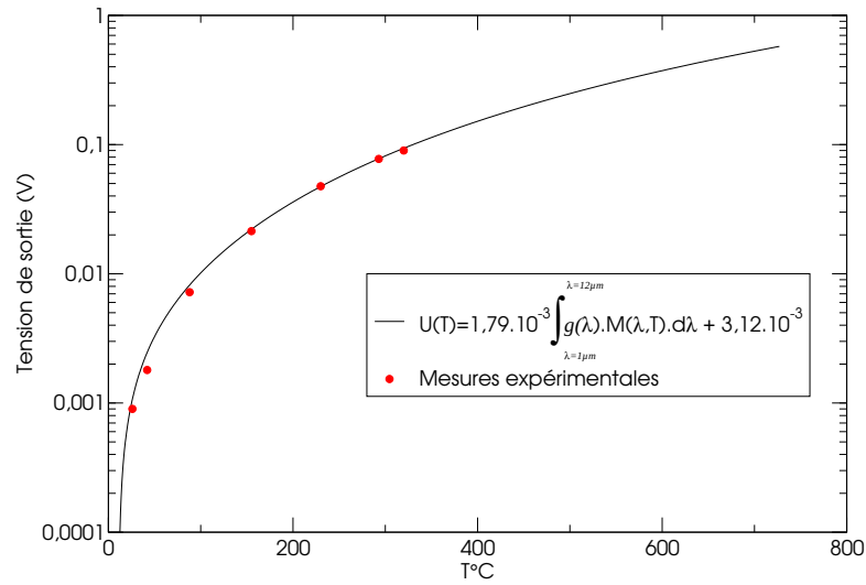
FIG. 3.17: Extrapolation jusqu'à 800°C de l'étalonnage dans le cas du tungstène
