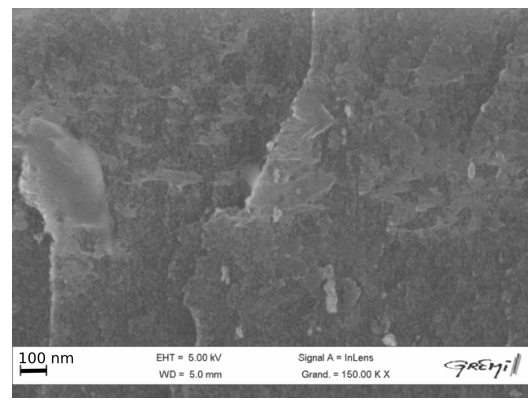
(b) Images MEB transverse du silicium mésoporeux
