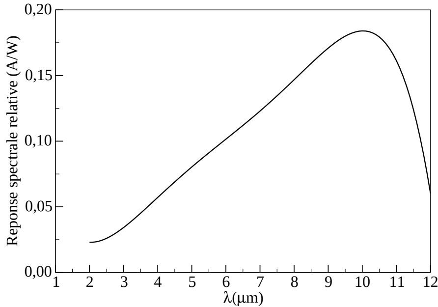
FIG. 3.12: Courbe de réponse spectrale du détecteur IR
