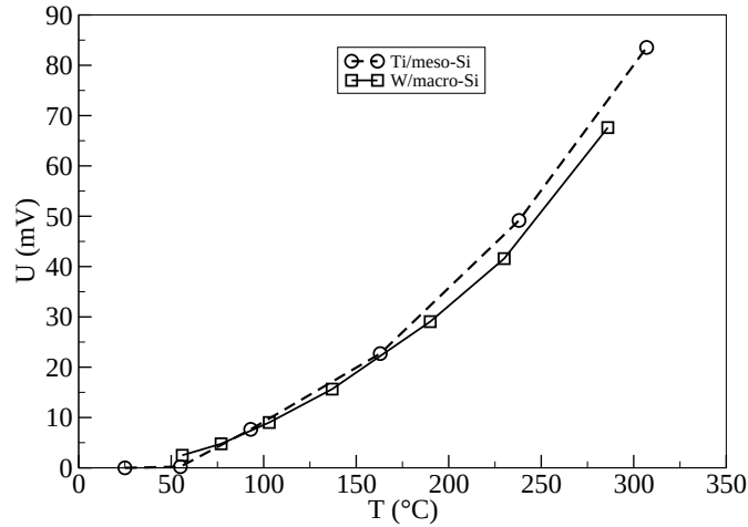
FIG. 5.24: Courbes d'étalonnage en température des dépôts de Ti sur Si mésoporeux et macroporeux
