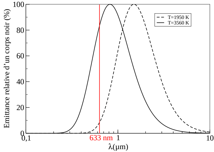
FIG. 4.13: Emittance normalisée d'un corps noir chauffé à la température d'évaporation du titane
