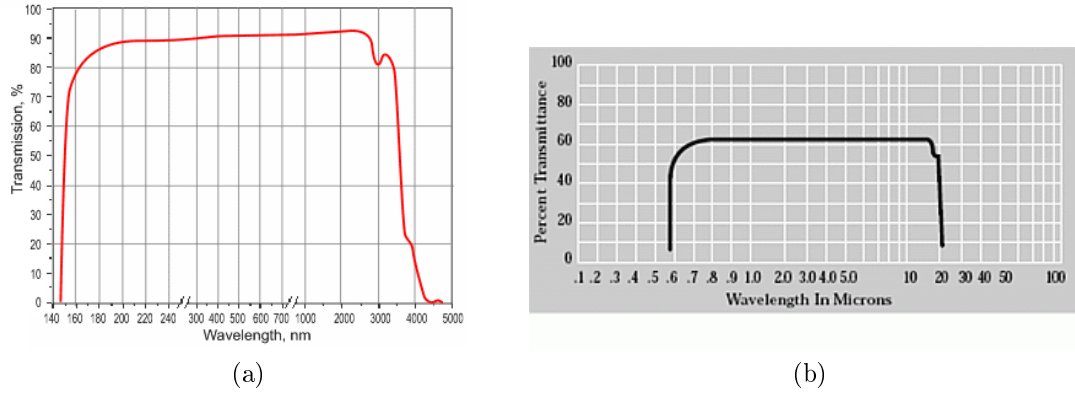
FIG. 3.8: Coefficients de transmission des hublots en quartz (a) et en ZnSe (b)
