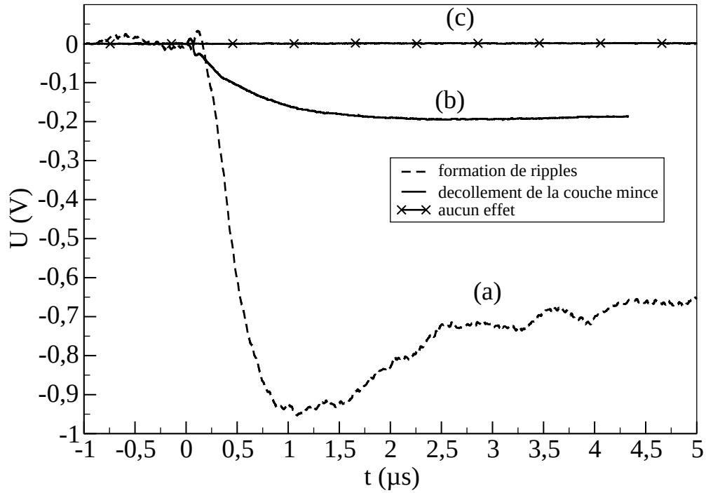
FIG. 4.3: Variations de la réflectivité de surface pour un dépôt de cuivre de 250 nm d'épaisseur sur verre, dans le cas d'apparition des ripples (a), de décollement de la couche de cuivre (b) et dans la cas où la surface n'est pas modifiée (c)
