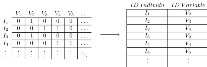
FIGURE 4.8 – Jeu de données binaire de faible densité : depuis la matrice creuse ( individus-variables ) au tableau bivarié dense
