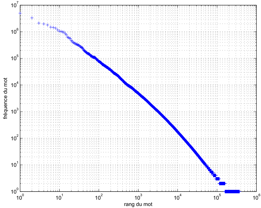
FIGURE 5.1 – Graphique log/log de la fréquence des mots par leur rang dans le Corpus Flixster
