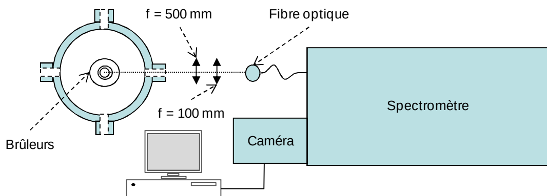
Figure V.6. Dispositif expérimental pour la mesure de l'émission de \text{OH}^* , \text{CH}^* et \text{C}_2^*
