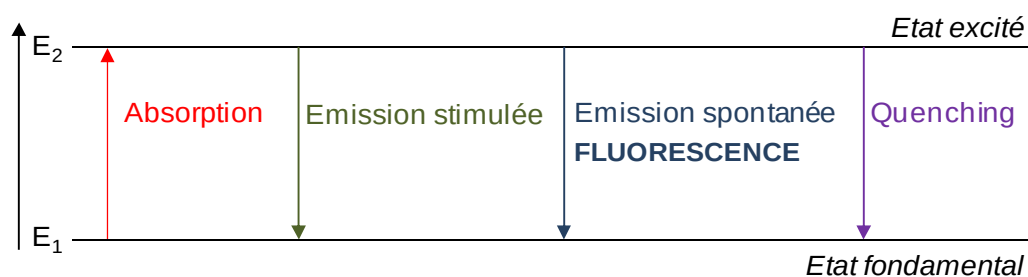
Figure II.14. Schéma de principe de la Fluorescence Induite par Laser
