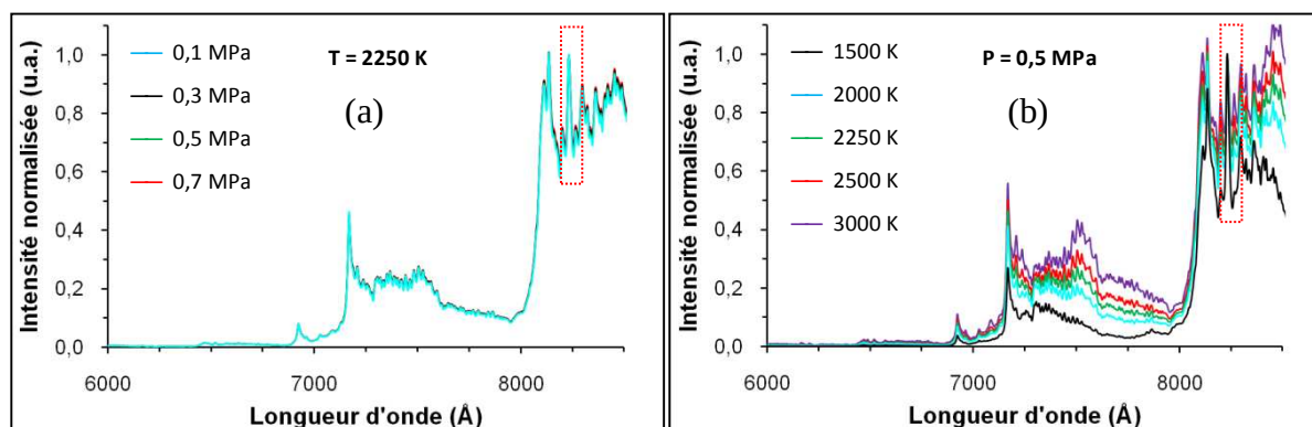
Figure V.14. Spectres de \text{H}_2\text{O}^* simulés à différentes pressions (a) et différentes températures (b)
