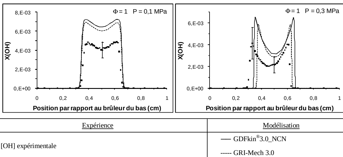
Figure V.26. Comparaison entre les profils de OH expérimentaux et modélisés pour la flamme \text{CH}_4/\text{air} de richesse 1 à 0,1 MPa et 0,3 MPa
