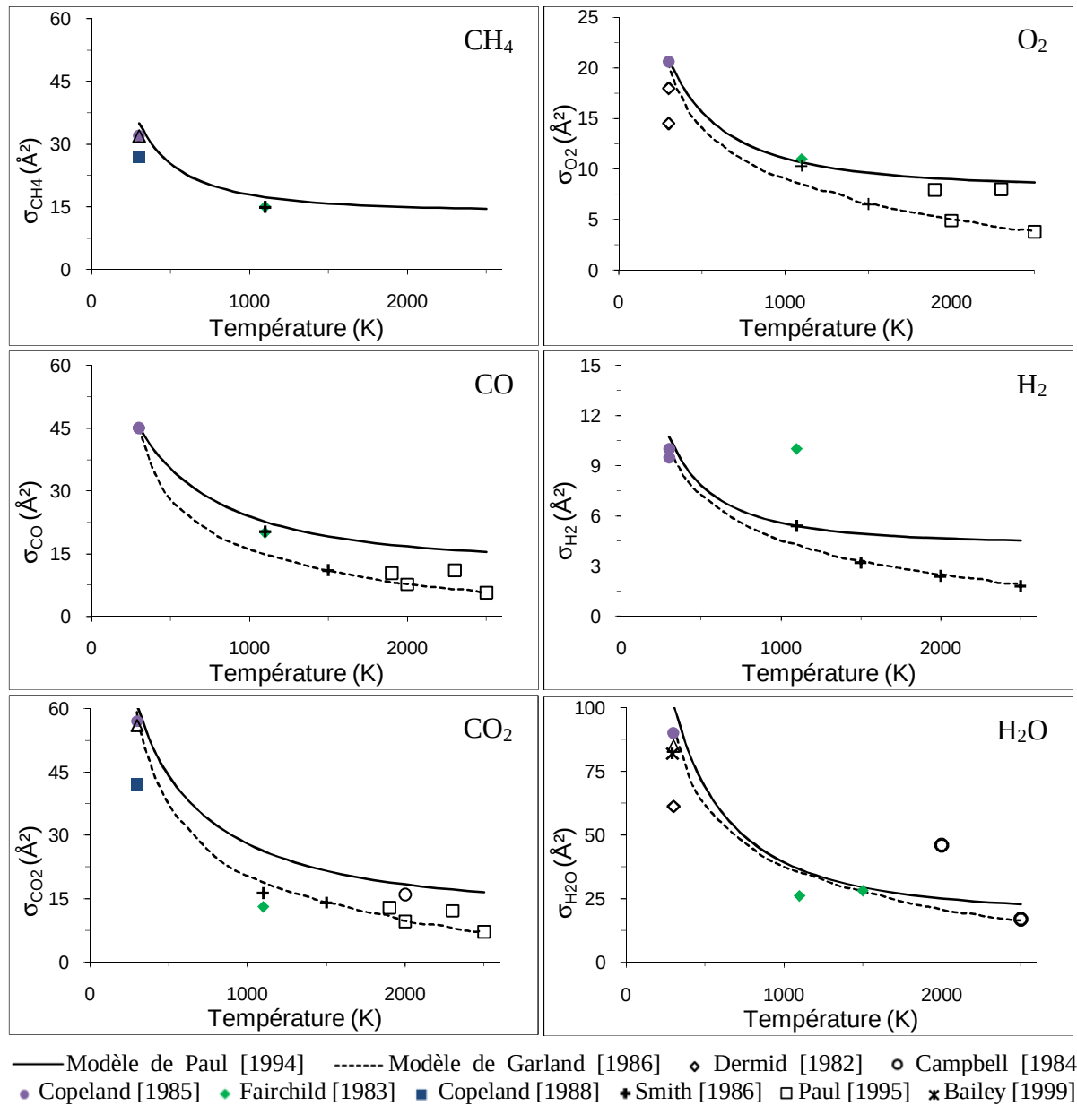
Figure IV.8. Sections efficaces de collision pour OH calculées avec les modèles de Paul (1994) et de Garland et Crosley (1986) comparées avec les données expérimentales de la littérature
