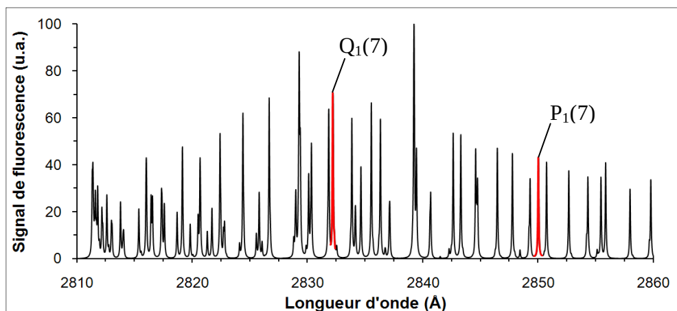
Figure IV.2. Spectre d'excitation de OH de la bande A^2\Sigma^+ \leftarrow X^2\Pi(1,0) modélisé par Lifbase [Luque et Crosley (1999)]
