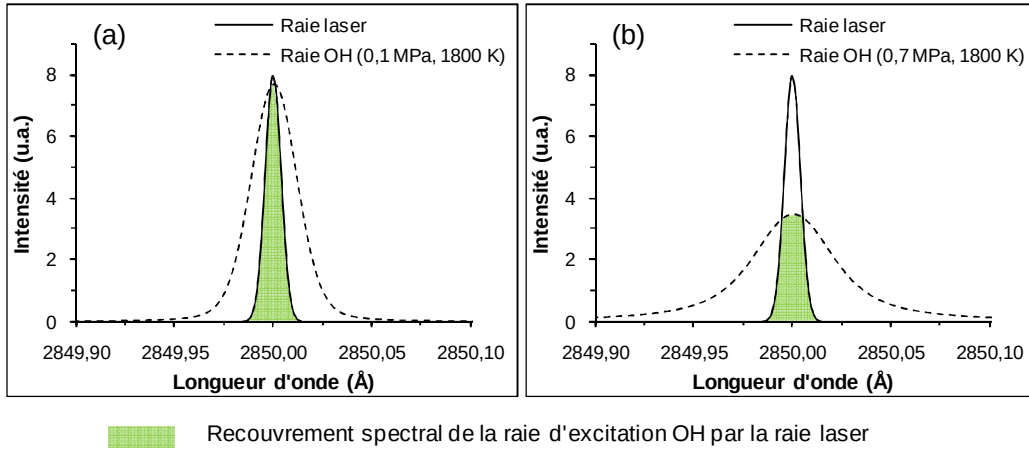
Figure IV.4. Formes de la raie laser et de la raie d'absorption de OH à pression atmosphérique et haute pression et représentation de la variation du recouvrement spectral dans chacun des cas.
