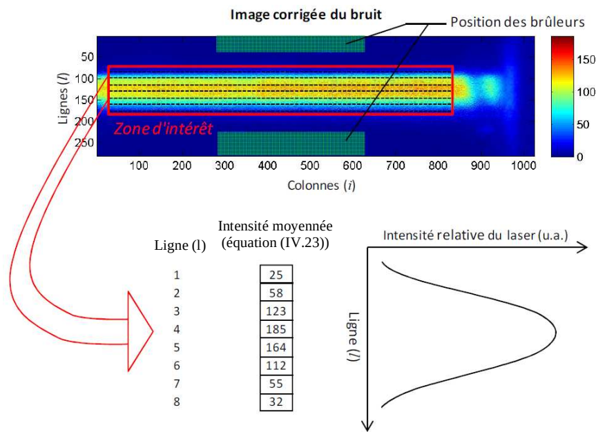
Figure IV.28. Schéma du calcul pour la répartition de l'énergie laser
