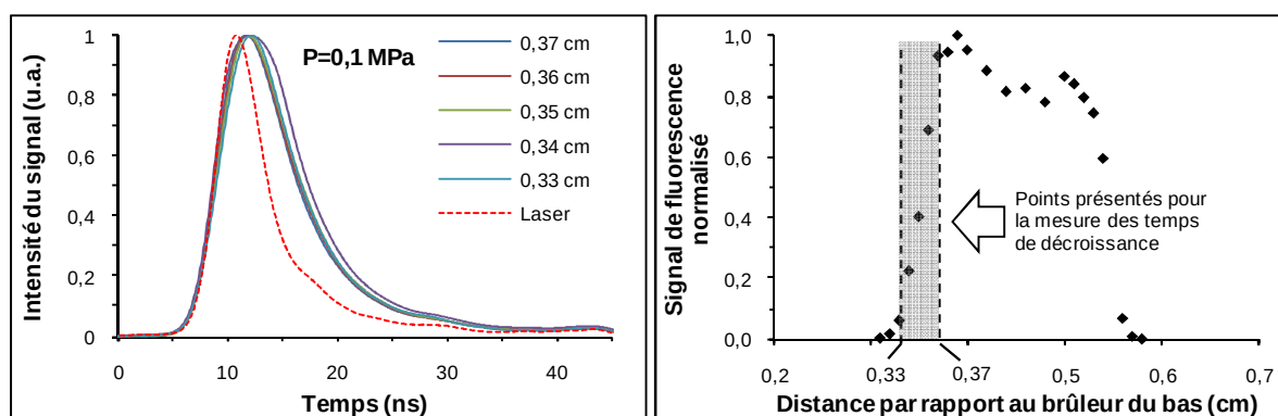
Figure V.18. Evolution temporelle du signal de fluorescence mesurée dans la flamme \text{CH}_4/\text{air} ( \Phi=0,7 ) à P=0,1 MPa à différentes positions dans le front de la flamme du bas
