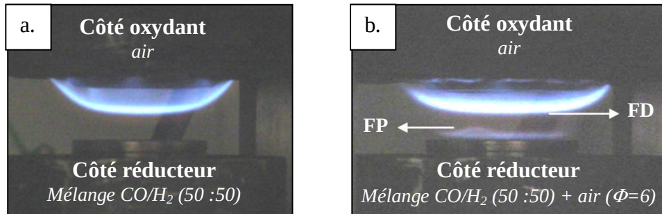
Figure II.4. Photographies de flammes à contre-courants [Som et al. (2008)]
