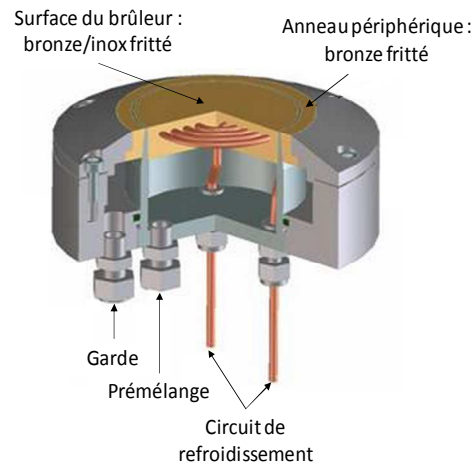
Figure II.5. Schéma d'un brûleur McKenna.
