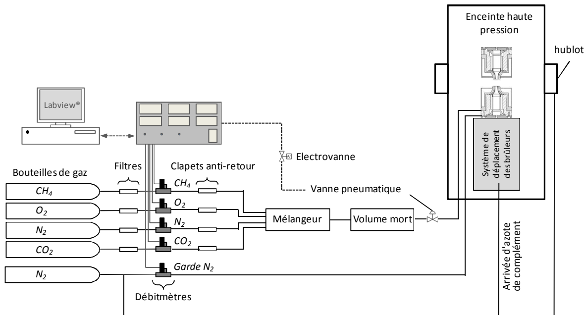
Figure III.10. Schéma du système d'alimentation en gaz pour un brûleur
