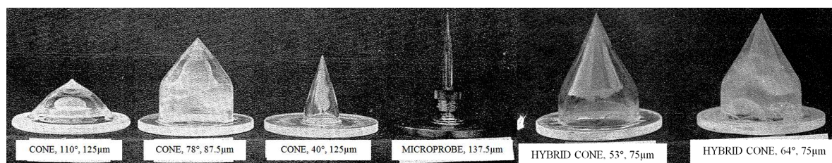
Figure II.11. Photographies de différents types de sondes de prélèvement.
