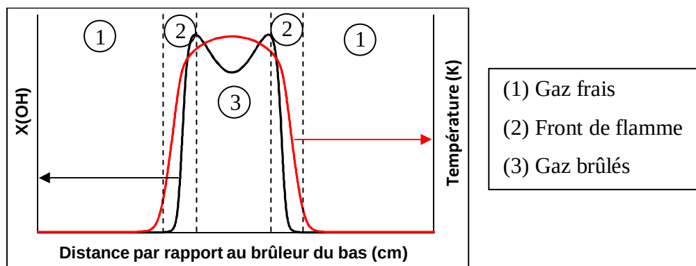
Figure IV.15. Représentation schématisée d'un profil de OH et d'un profil de température typiquement observés dans une flamme à contre-courants \text{CH}_4/\text{air} et des zones d'intérêt pour décrire les variations de la fraction de Boltzmann, du rendement quantique de fluorescence et du recouvrement spectral dans le cadre d'une mesure de OH par FIL.
