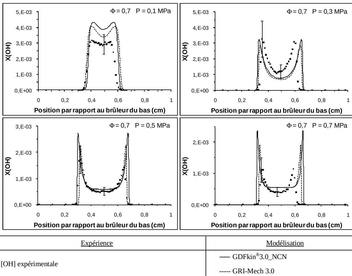
Figure V.25. Comparaison entre les profils de OH expérimentaux et modélisés pour la flamme \text{CH}_4/\text{air} de richesse 0,7 de 0,1 MPa à 0,7 MPa
