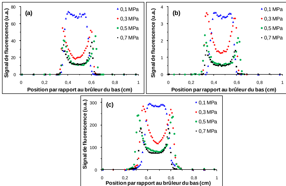
Figure V.15. Signal de fluorescence de OH mesuré dans les flammes \text{CH}_4/\text{air} \Phi=0,7 à différentes pressions ( P=0,1 à 0,7 MPa) avec différents schémas d'excitation/détection :
