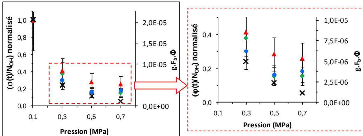
Figure V.16. Rapports des signaux de fluorescence sur la densité de population de OH mesurés dans les gaz brûlés des flammes CH_4/air \Phi=0,7 à différentes pressions
