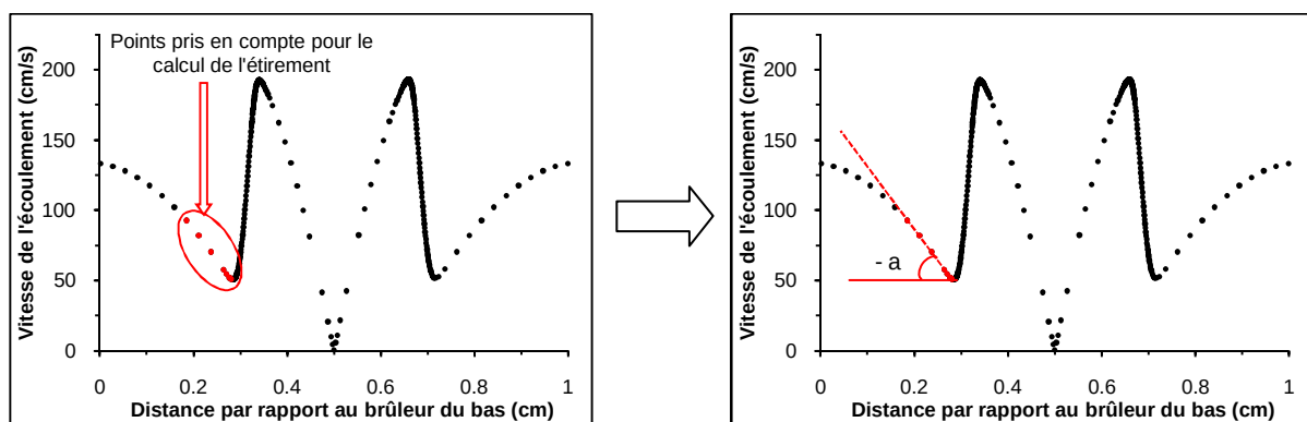
Figure V.1. Représentation du calcul de l'étirement pour la flamme CH 4 /air, \Phi=1 , P=0,1 MPa
