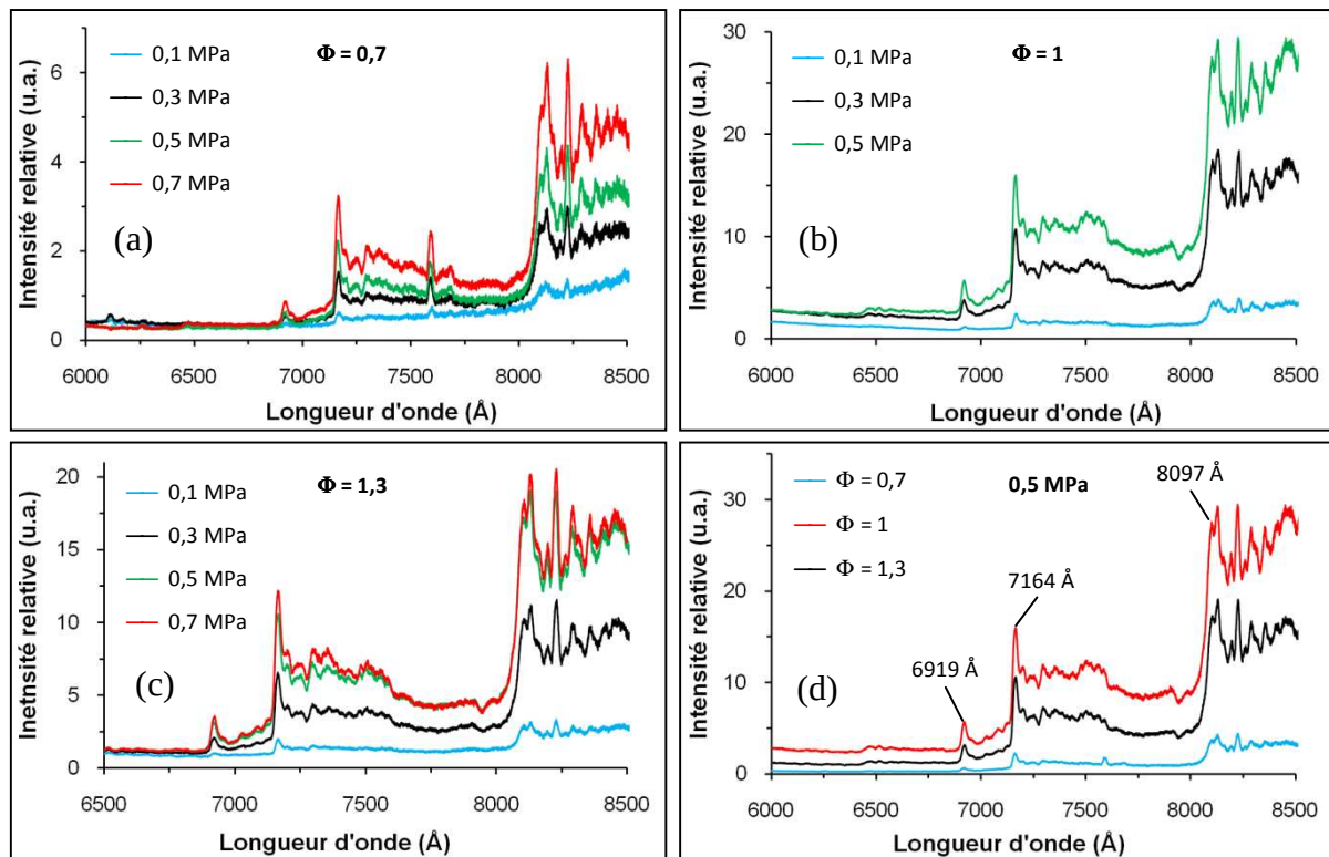
Figure V.11. Spectres d'émission de 6000 à 8500 Å des flammes \text{CH}_4/\text{air} à différentes richesses et à différentes pressions
