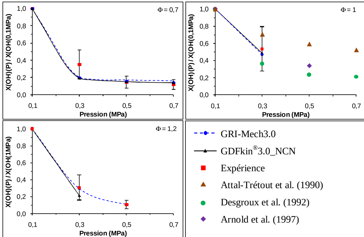
Figure V.28. Evolution en fonction de la pression du rapport des concentrations de OH haute pression / pression atmosphérique dans le cas de l'expérience et de la simulation.
