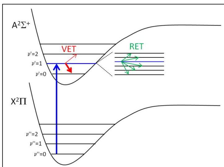
Figure A.4. Schéma de principe des Transferts d'Energie Vibrationnels (VET) et Rotationnels (RET)
