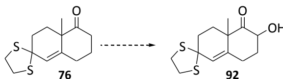
Schéma 83
