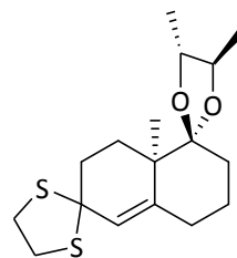
(-)110
