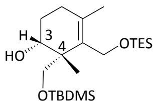
Figure 62 : composé 37
