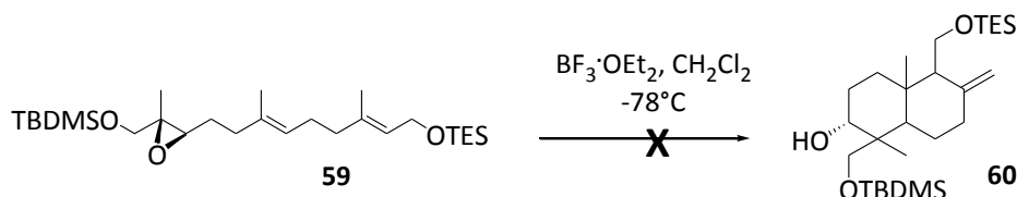
Schéma 49
