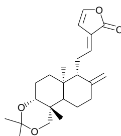
Composé 5
