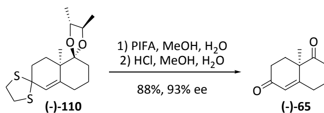
Schéma 107
