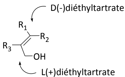
Figure 58 : Différenciation diastéréofaciale
