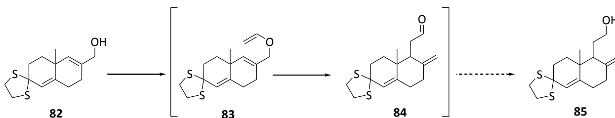
Schéma 77
