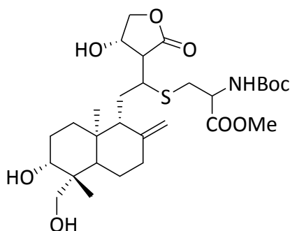
Composé 10
