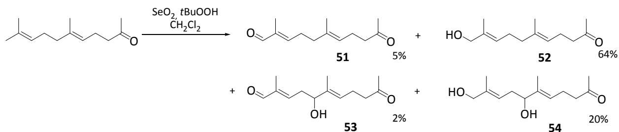
Schéma 47
