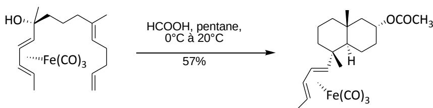
Schéma 11
