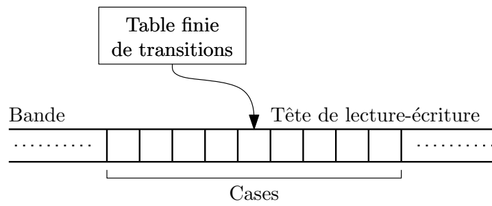
FIGURE 1.1 — Schéma représentant une machine de TURING déterministe à une bande.
