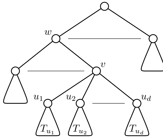
FIGURE 4.5 — Arbre T contenant un noeud v , de père w et avec d fils u_1, u_2, \dots, u_d .
