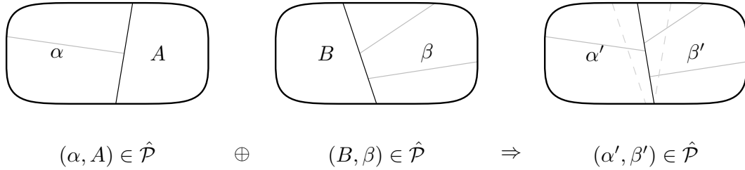
FIGURE 2.5 — Schéma de deux partitions (\alpha, A), (B, \beta) \in \hat{\mathcal{P}} , et d'une partition \mu = (\alpha', \beta') \in \hat{\mathcal{P}} plus fine que (\alpha, \beta) .
