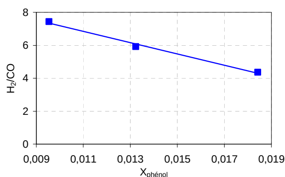
Figure 4.56 : Rapport H_2/CO en fonction de la fraction molaire du phénol dans le liquide injecté ( D_{inj} = 75,3\text{mL/h} ).
