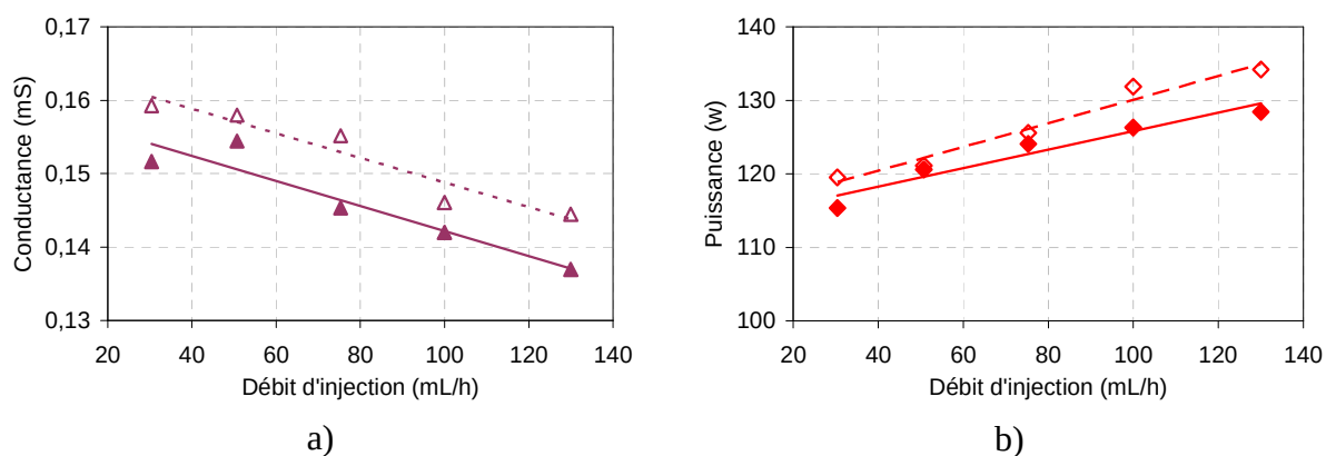
Figure 4.21 : Evolution a) la conductance (mS) ; b) la puissance électrique (W) en fonction du débit d'injection. ( X_{\text{CH}_3\text{OH}} = 0,09 symboles pleins) et ( X_{\text{CH}_3\text{OH}} = 0,21 symboles vides).
