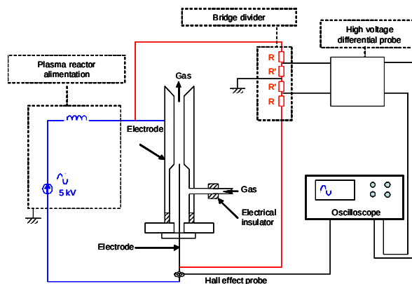
Figure 1.13 : Schéma de fonctionnement du réacteur plasma et son alimentation électrique.
