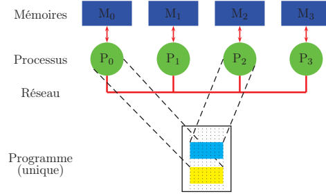
FIGURE 1.6 – Modèle de programmation de SPMD
