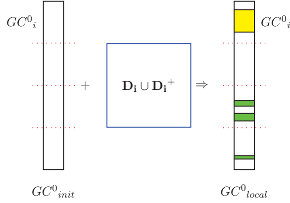
FIGURE 6.4 – Calcul de GC^0_i dans un sous-domaine D_i
