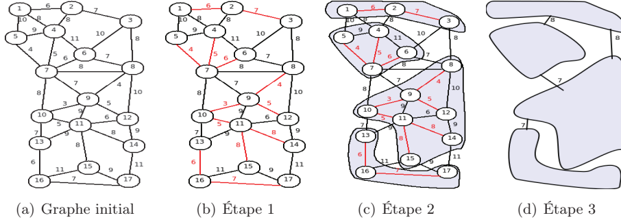
FIGURE 5.2 – Illustration de l'algorithme de Borůvka
