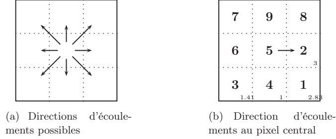
FIGURE 2.3 – Modèle D8 (Deterministic Eight-neighbor en anglais)
