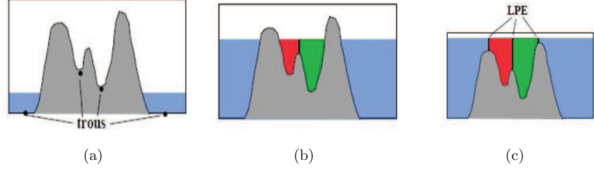
FIGURE 3.2 – Simulation d'immersion dans la LPE
