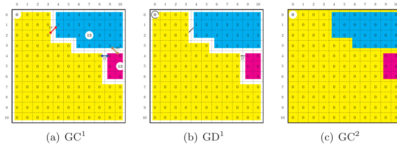
FIGURE 5.5 – Calcul de la hiérarchie : deuxième niveau
