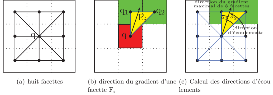
FIGURE 2.4 – Modèle D_\infty pour le calcul des directions d'écoulements
