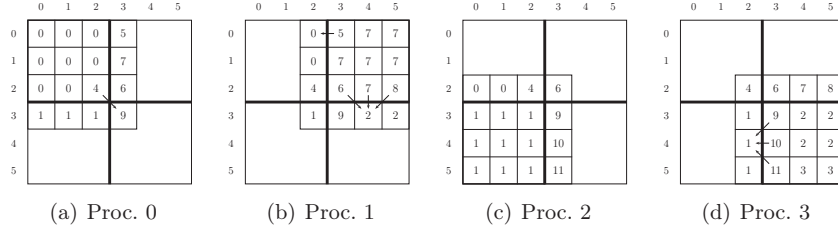
FIGURE 6.2 – Calcul parallèle local des bassins versants aux Proc. i
