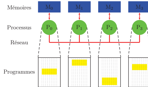
FIGURE 1.9 – Modèle de programmation à passage de messages
