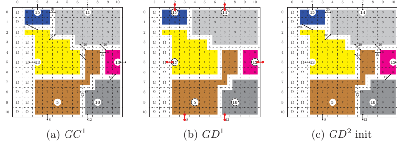
FIGURE 5.8 – Hiérarchie avec règle \Omega : Deuxième étape
