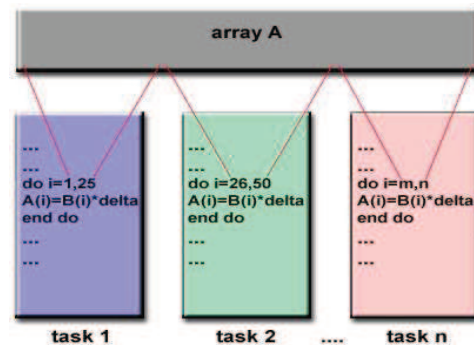
FIGURE 1.7 – Modèle de programmation de “Data-Parallel”
