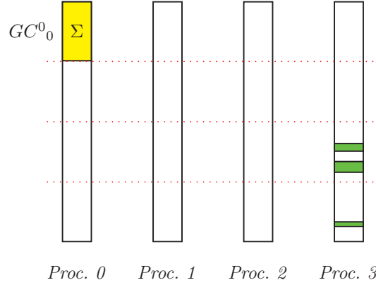
FIGURE 6.5 – Finalisation GC^0_0 correspondant au Proc. 0
