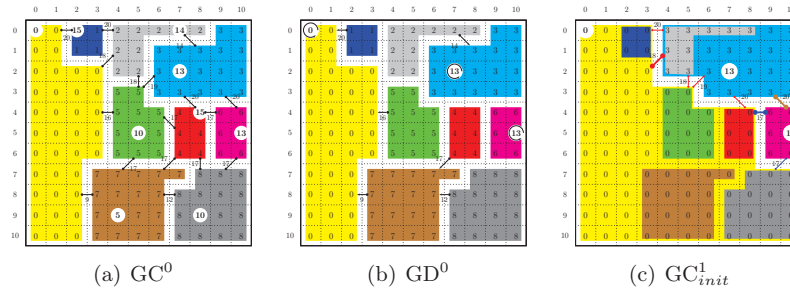
FIGURE 5.4 – Calcul de la hiérarchie : Premier niveau
