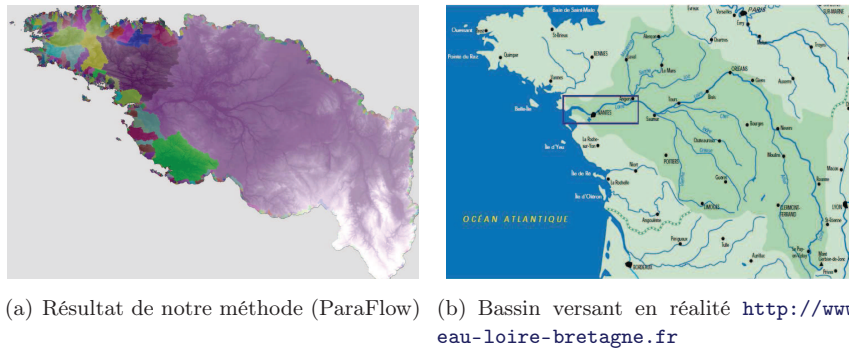
FIGURE 7.4 – Bassin versant de la Loire en France
