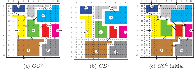
FIGURE 5.7 – Hiérarchie avec règle \Omega : Première étape
