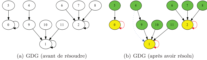
FIGURE 6.3 – Graphe de dépendances GDG global
