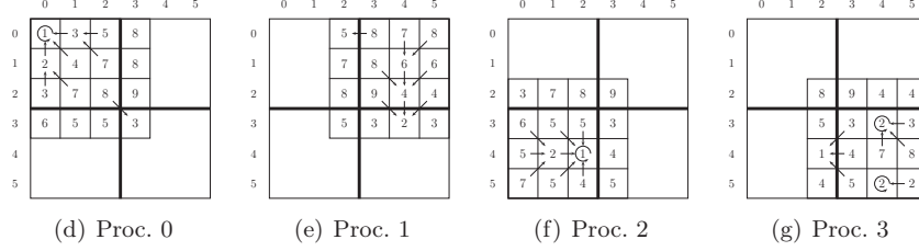
FIGURE 6.1 – Calcul parallèle des directions d'écoulements
