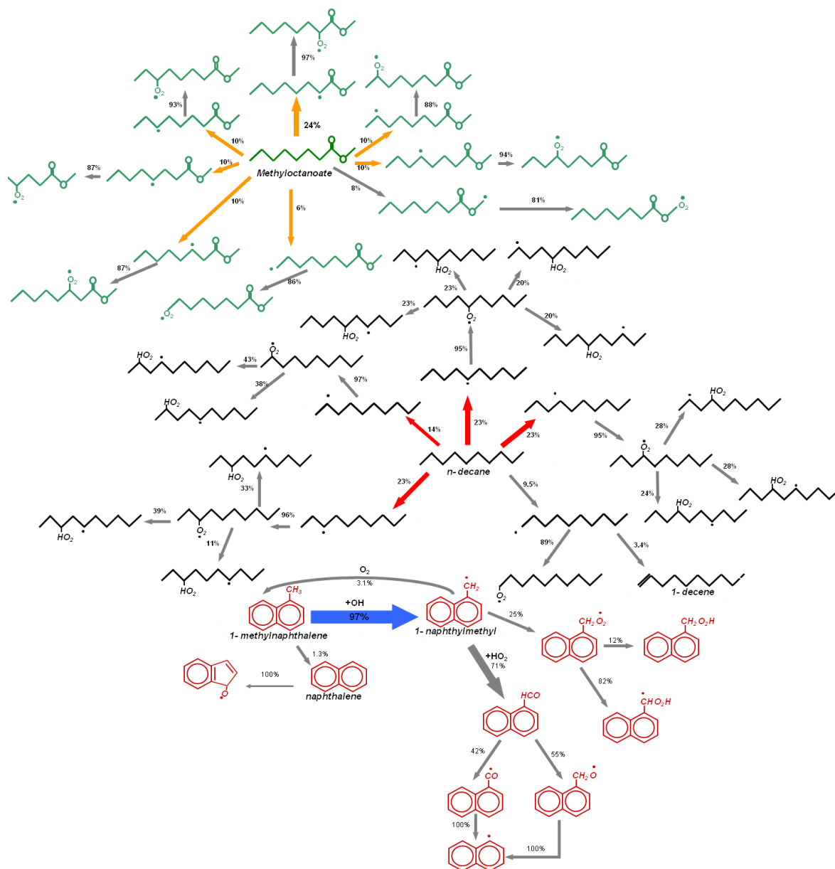
Figure 96. Analyse des principales voies réactionnelles pour l'oxydation du B30 modèle à 910 K, 20 bar, \phi=1 et pour une consommation de 21,69% du 1-méthyl-naphtalène, de 76,09% du n -décane et 64,14% de l'octanoate de méthyle.
