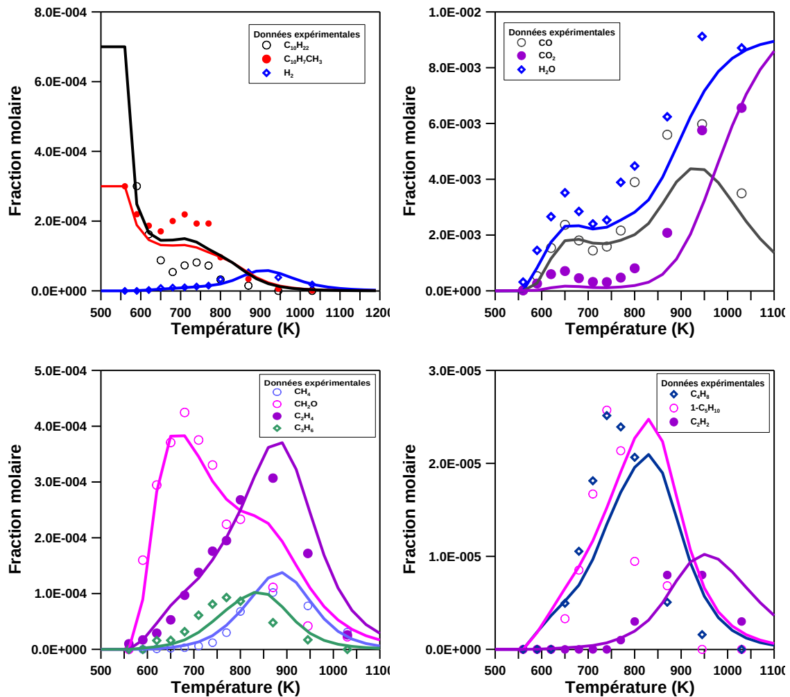
Figure 64. Confrontation du modèle (lignes) avec les expériences (symboles) lors de l'oxydation d'un carburant réel type gazole en JSR : \phi=0.25 , 10 bar et \tau=1 s. Les incertitudes estimées sont de l'ordre de \pm 10\% .
