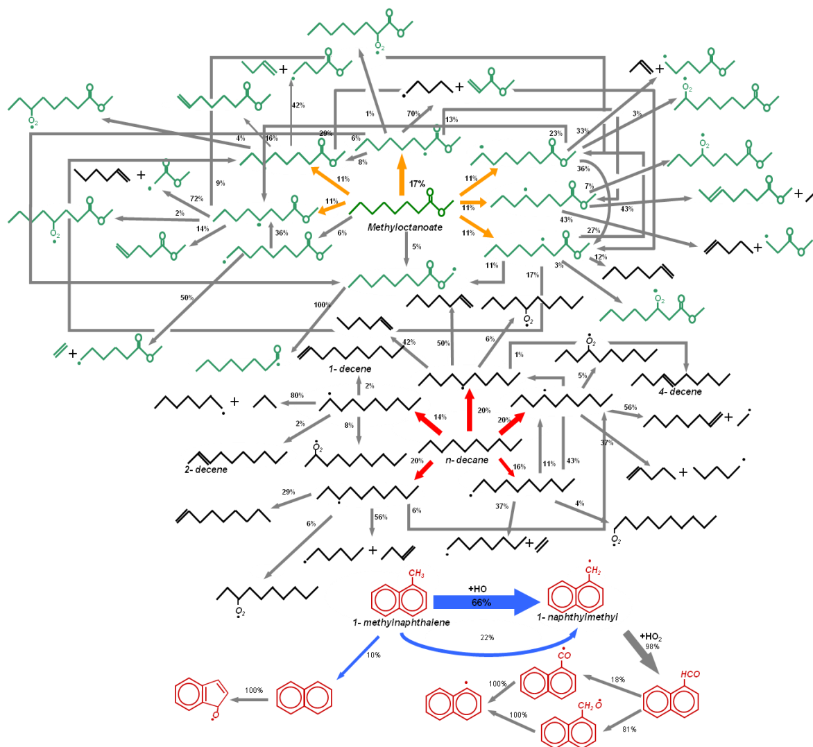
Figure 98. Analyse des principales voies réactionnelles lors de l'oxydation du B30 modèle à 1210 K, 20 bar, \phi=1 et pour une consommation de 19,08% du 1-méthyl-naphtalène, de 45,74% du n -décane et de 60,71% de l'octanoate de méthyle.
