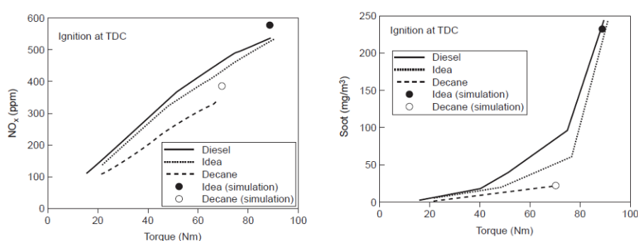
Figure 30. Concentration dans les gaz d'échappement de a) NO x et b) Suie pour différents carburants. Barths et al. 1999.
