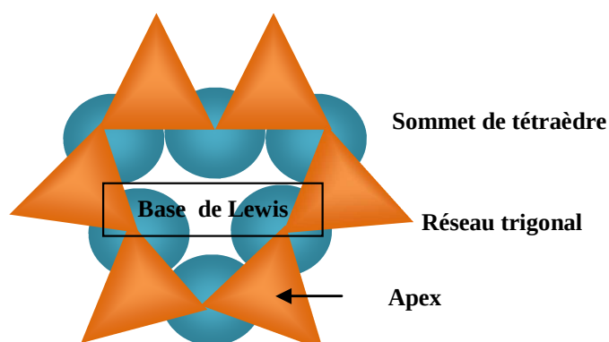
Figure 6 Schéma d'une cavité hexagonale selon le plan a-b se comportant comme un site de base faible (Lewis)
