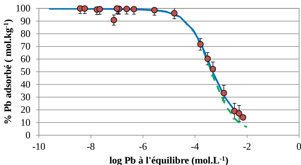
Figure 45 Isotherme d'adsorption du plomb dans une montmorillonite calcique à pH 7 (MOPS à 10 -3 M) et r_{S/L} = 10 \text{ g L}^{-1} . • : points expérimentaux ; courbe verte en trait interrompu obtenue en utilisant le modèle de Bradbury and Baeyens (1999) et nos données thermodynamiques déterminées à pH 5 (Ghayaza et al. , 2011) ; courbe bleue en trait continu : meilleure corrélation obtenue pour \log K_c(\text{Ca-Pb})=1
