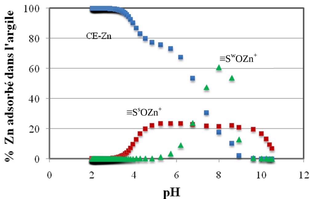
Figure 55 Contribution des différents mécanismes d'adsorption du zinc en fonction du pH dans la montmorillonite Na-SWy2 ; ■ : % du Zn adsorbé par échange cationique (CE-Zn), ▲ % du Zn adsorbé par les sites faibles ( \equiv S^wOZn^+ ) ; ■ : % du Zn adsorbé par les sites forts ( \equiv S^sOZn^+ );
