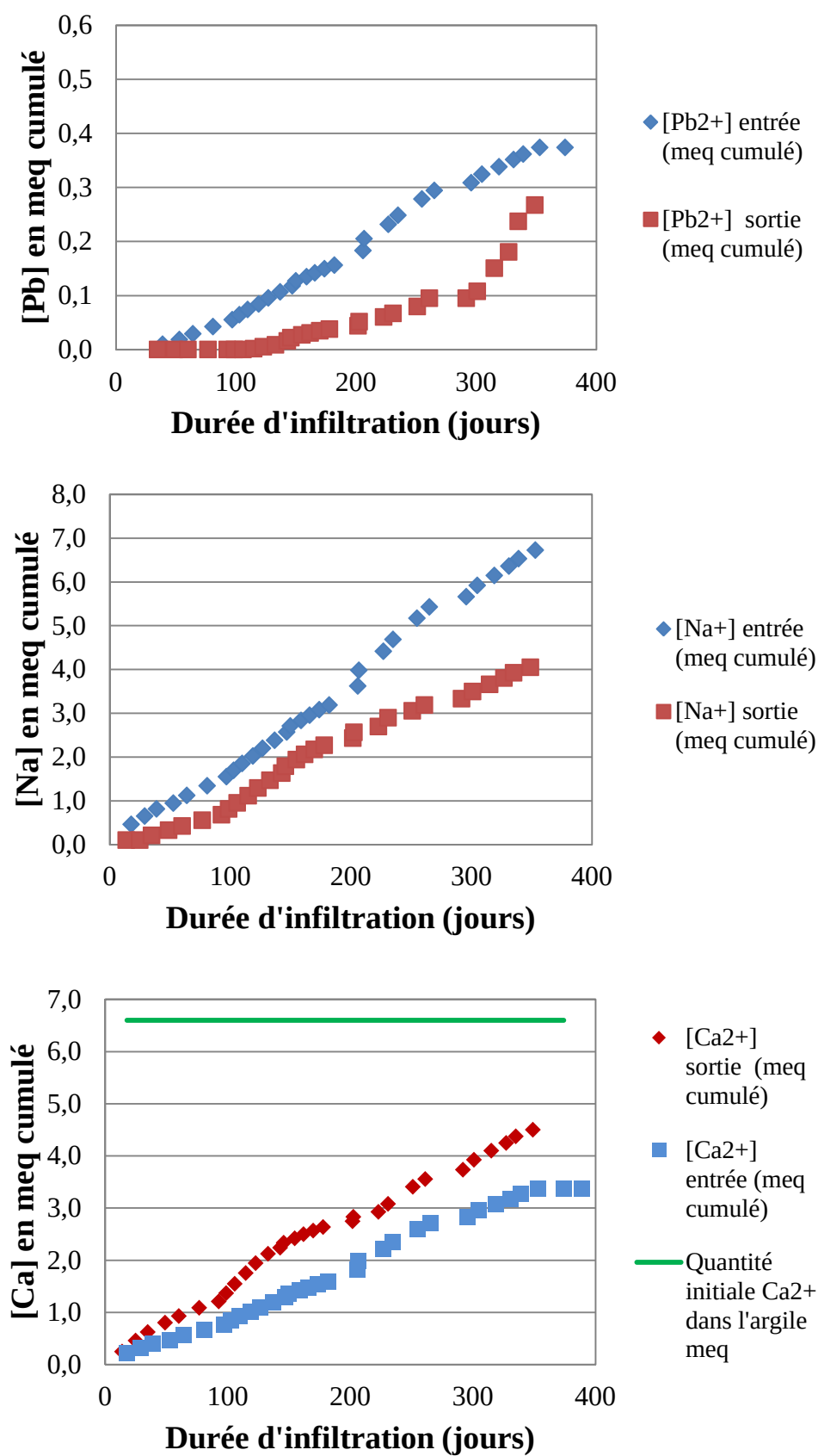
Figure 106 Concentrations des cations Pb 2+ , Na + et Ca 2+ dosés en solution (en meq cumulé) en entrée et à la sortie des cellules œdométriques Le trait vert continu correspond à la quantité initiale de Ca dans la galette d'argile
