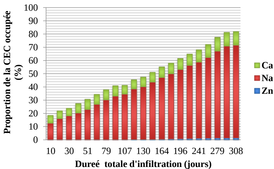
Figure 105 : Proportion (%) de la CEC occupée par les cations \text{Ca}^{2+} , \text{Na}^+ et \text{Zn}^{2+} en fonction de la durée totale d'infiltration
