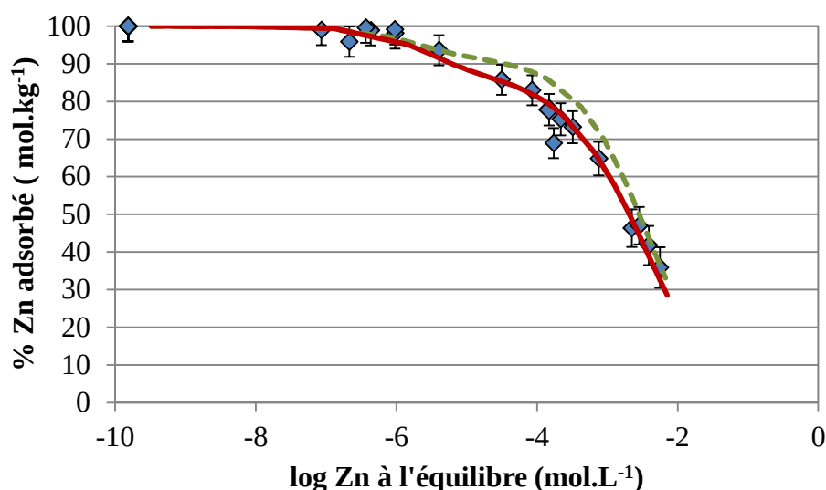
Figure 39. Isotherme d'adsorption du zinc dans une montmorillonite sodique à pH 7 (MOPS à 10^{-3} M) et r_{S/L} = 10 \text{ g L}^{-1} . ♦ : points expérimentaux ; courbe verte en trait interrompu obtenue en utilisant le modèle et les constantes de Bradbury and Baeyens (1997) ; courbe rouge en trait continu: meilleure corrélation obtenue pour \log K_c(\text{Na-Zn}) = 0,2
