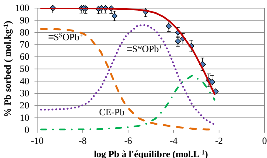
Figure 44 Isotherme d'adsorption du plomb dans une montmorillonite sodique à pH 7 et contribution des différents sites d'échange de surface. ♦: données expérimentales. La courbe rouge en trait continu représente la courbe modélisée avec les paramètres suivants: \log K_c(\text{Pb-Na}) = -0,7 ; \log {}^S K_{\text{int}}(\text{Pb}) = 1,5 et \log {}^W K_{\text{int}}(\text{Pb}) = -0,5 . Courbe verte: échange cationique (CE-Pb); courbe orange avec trait interrompu: complexation sur les sites forts ( \equiv S^S \text{OPb}^+ ); courbe violette en pointillés: complexation sur les sites faibles ( \equiv S^W \text{OPb}^+ ).
