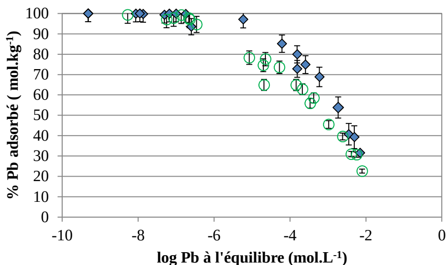
Figure 35 Isotherme d'adsorption du plomb dans la montmorillonite sodique Na-SWy2, respectivement à pH 5 (tampon d'acide acétique / acétate de sodium) et pH 7 (tampon MOPS à 10^{-3} M) avec I = 0,04 M, et r_{S/L} = 10 \text{ g L}^{-1} . ♦ : % du Pb adsorbé à pH 7 et ○ : % du Pb adsorbé à pH 5
