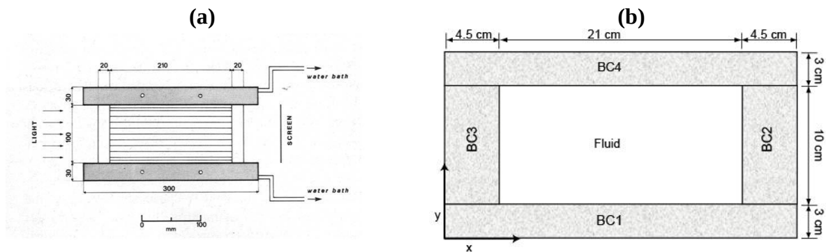
Figure 14. Détail des dimensions de la cuve de plexiglas : (a) expérience analogue [Brandeis, 1983]. Dans l'expérience analogue on peut noter que les parois ont 2 cm d'épaisseur, les dimensions horizontales sont de 25 x 25 cm et 10 cm de haut. Les limites supérieure et inférieure sont composées de plaques de cuivre de 3 cm d'épaisseur à travers lesquelles circule de l'eau maintenue à température constante, (b) expérience numérique. BC signifie conditions limites.
