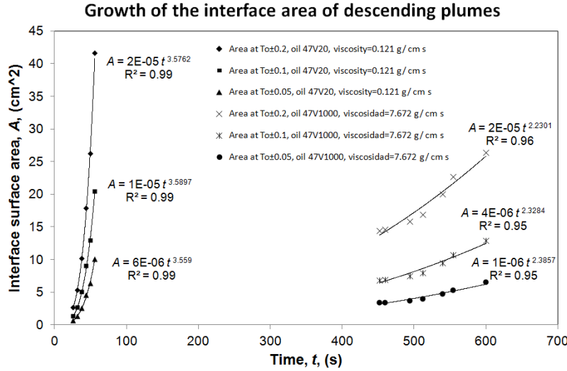
Figure 21. Évolution de l'aire d'interface des instabilités en fonction du temps : comparaison entre l'expérience avec l'huile 47V20 (moins visqueuse) et celle avec l'huile 47V1000 (plus visqueuse). Les différentes courbes (du haut vers le bas) correspondent à une précision du facteur de croissance égale à la température initiale du système T_o \pm 0.2 , T_o \pm 0.1 et T_o \pm 0.05 pour chaque expérience.
