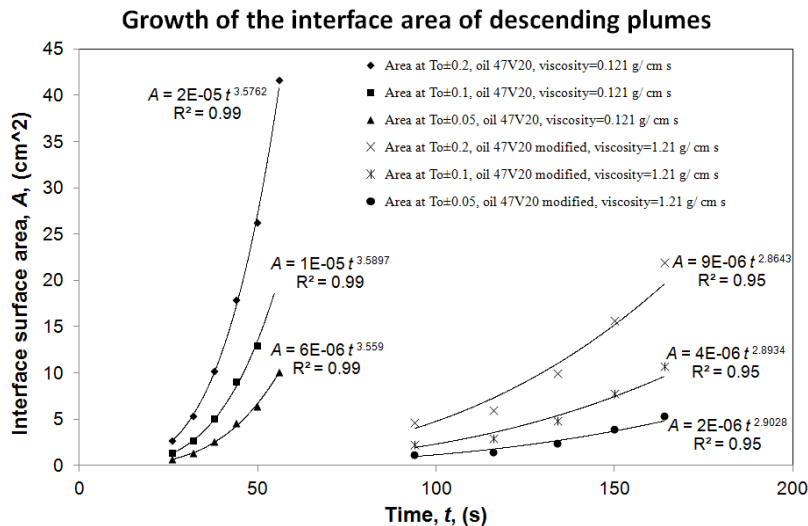
Figure 22. Comparaison de l'évolution de l'aire d'interface des instabilités en fonction du temps pour l'huile 47V20 et la même huile dont la valeur de viscosité est décuplée. Les différentes courbes (du haut vers le bas) correspondent à une précision du facteur de croissance égale à la température initiale du système T_o \pm 0.2 , T_o \pm 0.1 et T_o \pm 0.05 pour chaque expérience.
