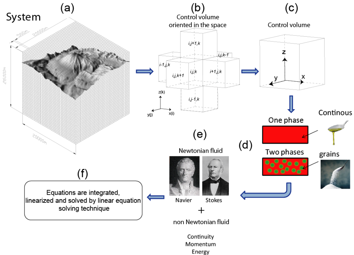
Figure 1. Représentation des principales étapes dans le calcul multiphasique.
