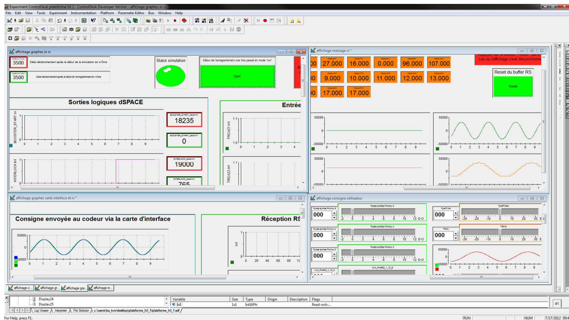
Figure V.20 : Interface de pilotage et d'observation du boîtier dSPACE
