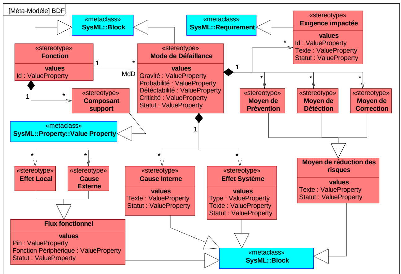
Figure III.10 : Méta-Modèle de la BDF
