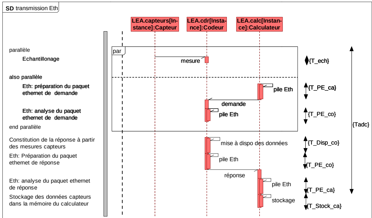
Figure V.13 : SD de la transmission Ethernet des données capteurs
