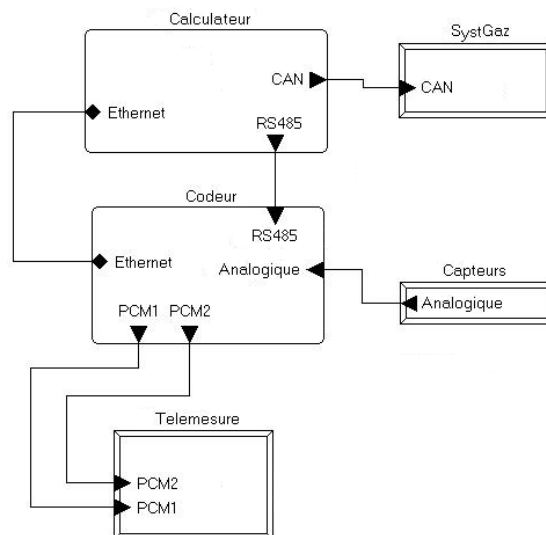
Figure V.14 : Modèle AADL du véhicule LEA
