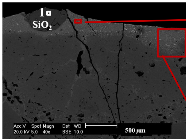
Figure IV-116 Microstructure MEB (mode électron rétrodiffusés) de l'interphase de corrosion (A1) du post mortem
