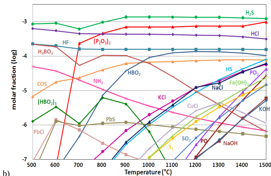
Figure III-27 Evolution de la fraction molaire des gaz minoritaires en fonction de la température pour la composition T [17].
