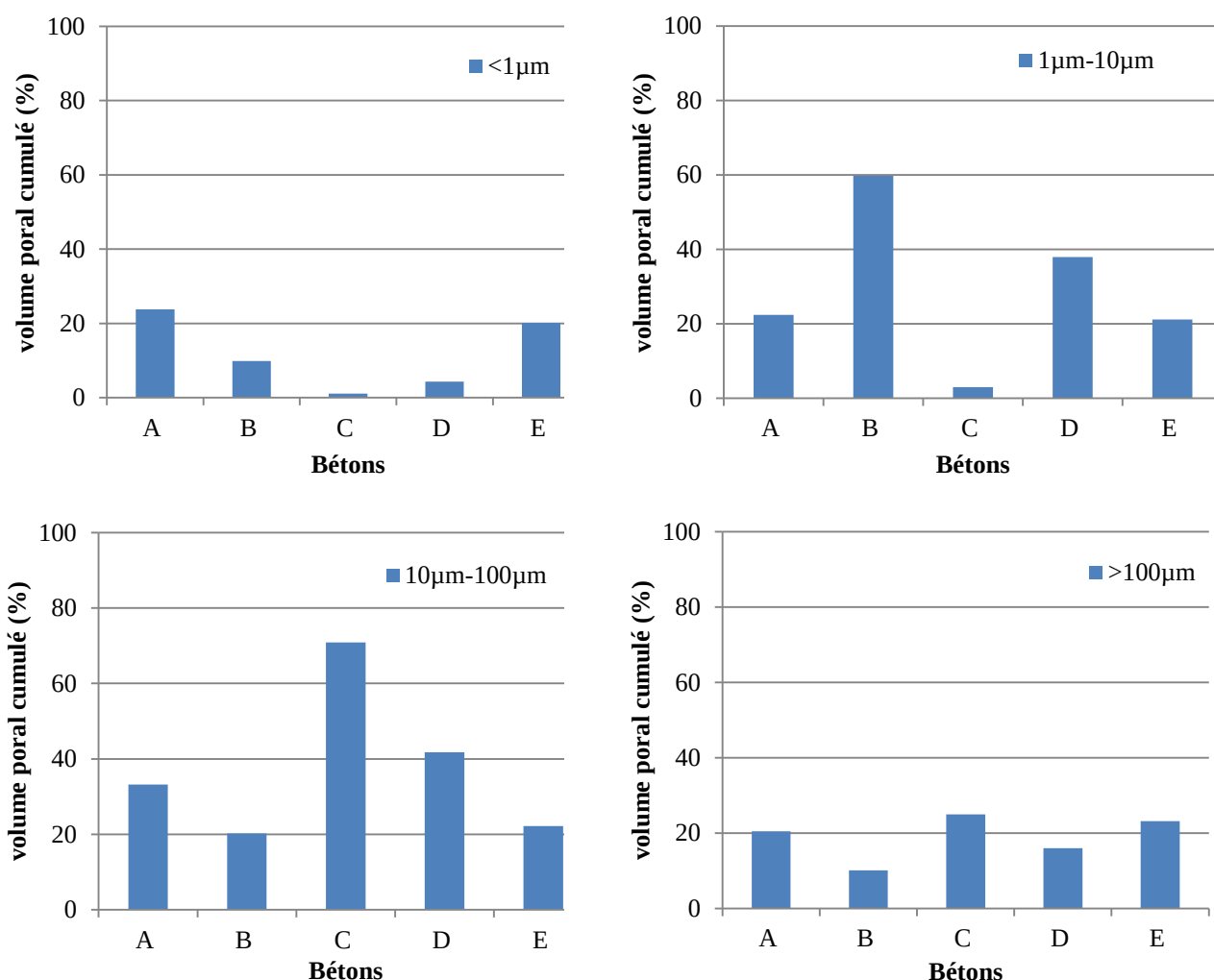
Figure IV-6 Distribution des volumes cumulés de la porosité selon la classe des pores
