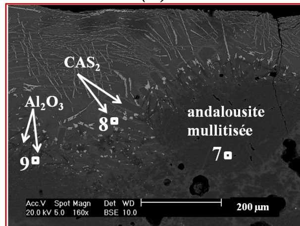
Figure IV-118 Agrandissement (mode électron rétrodiffusés) de l'interphase de corrosion (A1)
