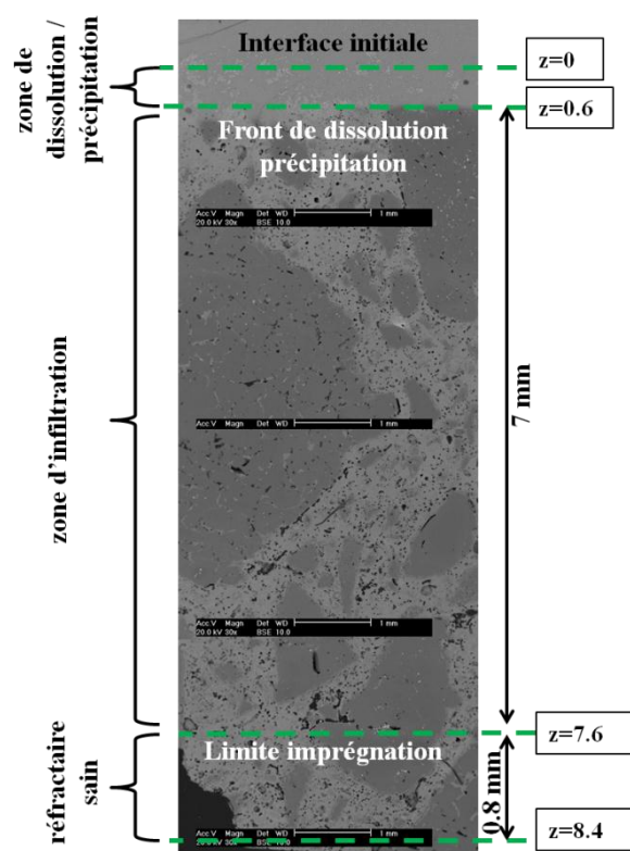
Figure IV-68 Interphase de corrosion du béton E
