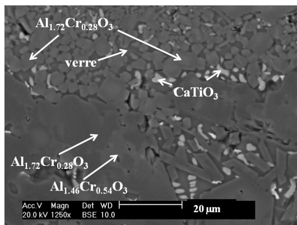
Figure IV-20 Cliché MEB (mode électrons rétrodiffusés) de la phase cimentaire du béton E
