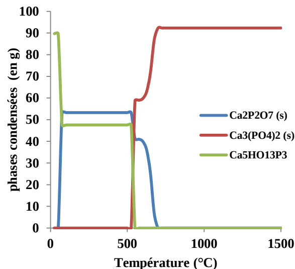
Figure III-7 Phases condensées et liquides en fonction de la température en absence d'oxygène pour 50% CaO-50% P_2O_5
