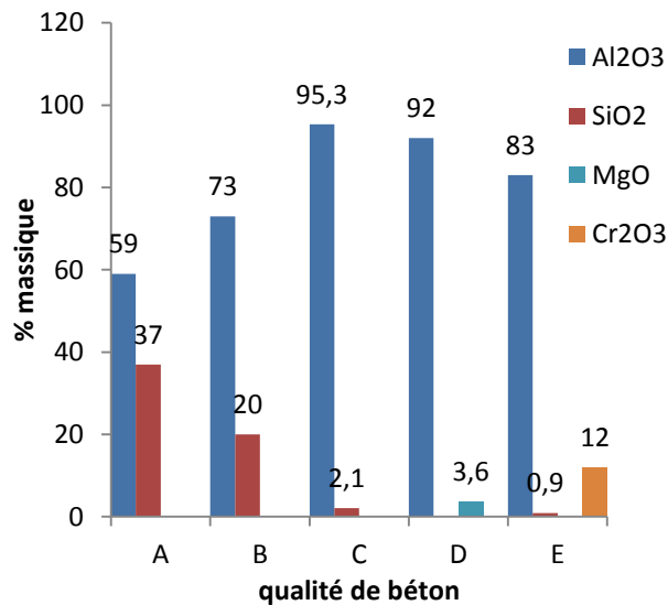
Figure IV-4 Composition (oxydes majeurs) des bétons utilisés
