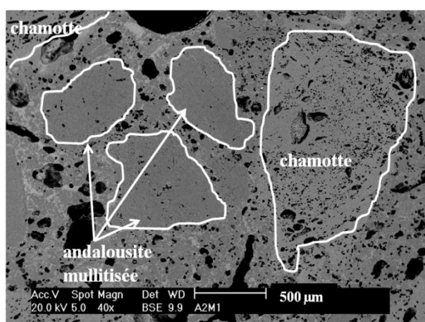
Figure IV-7 Cliché MEB (mode électrons rétrodiffusés) des agrégats constituant le béton A
