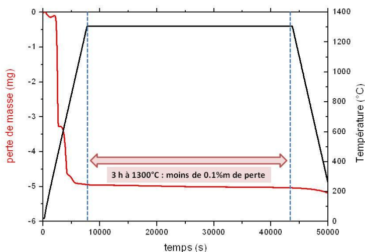
Figure III-19 ATG (courbe rouge) et température (courbe noire) pour le binaire 50% CaO -50% P_2O_5 en fonction du temps.
