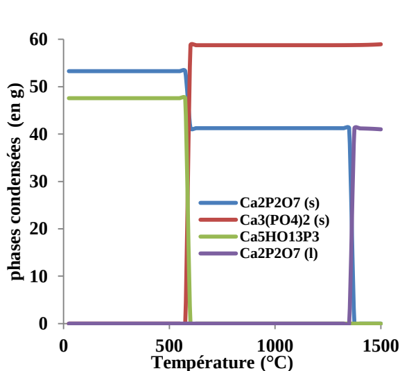
Figure III-6 Phases condensées en fonction de la température sous atmosphère oxydante pour 50% CaO-50% P_2O_5
