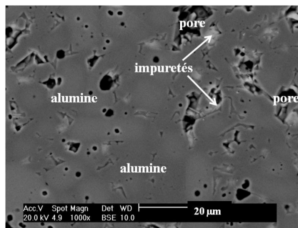
Figure IV-14 Agrandissement d'un grain d'alumine (mode électrons rétrodiffusés) contenu dans le béton C
