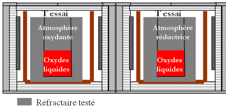
Figure IV-23 Schéma de l'essai comparatif sous différentes atmosphères
