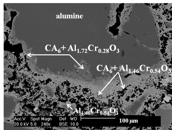
Figure IV-19 Cliché MEB (mode électrons rétrodiffusés) d'un grain d'alumine réagissant avec le \text{Cr}_2\text{O}_3
