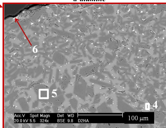
Figure IV-60 changements structuraux de la phase cimentaire du béton C après essai
