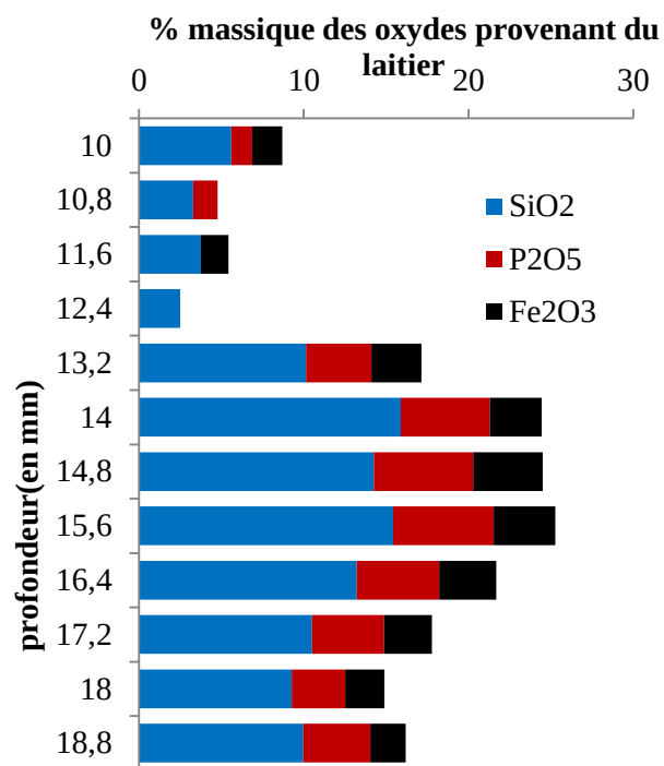
Figure IV-57 Profil chimique (par EDS) des oxydes provenant du laitier en fonction de la profondeur
