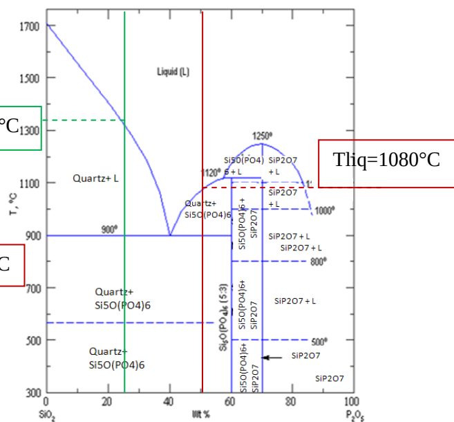
Figure II-10 Compositions replacées dans le diagramme établi par Mal'shikov et Bondar
