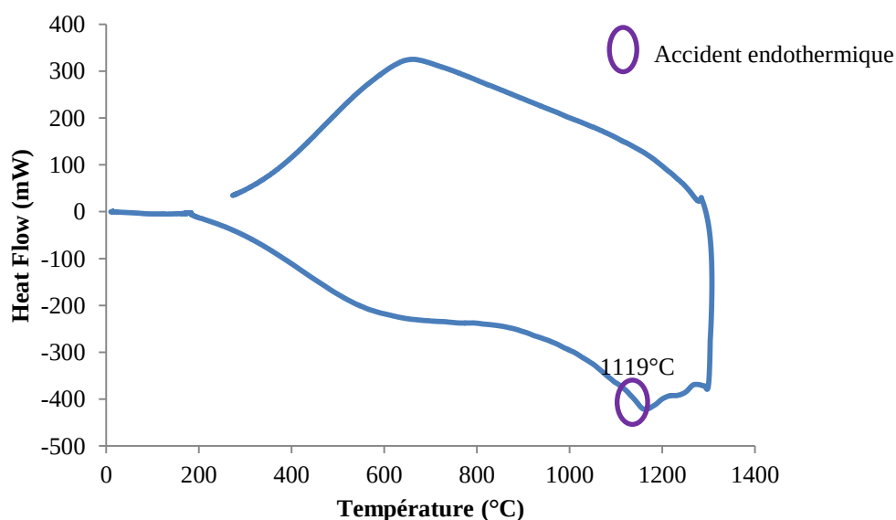
Figure II-16 DSC sur l'échantillon 50% \text{m SiO}_2 et 50% \text{m P}_2\text{O}_5
