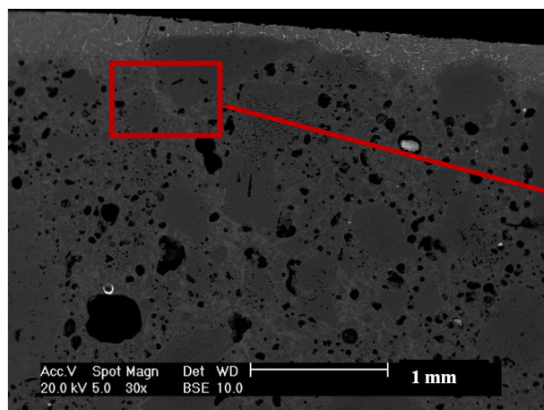
Figure IV-119 Cliché MEB (mode électron rétrodiffusés) de l'interphase de corrosion (A1) du post mortem
