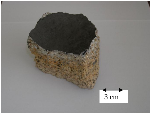
Figure IV-113 Réfractaire post mortem
