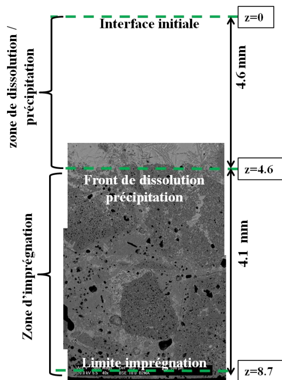
Figure IV-50 Interphase de corrosion du béton B
