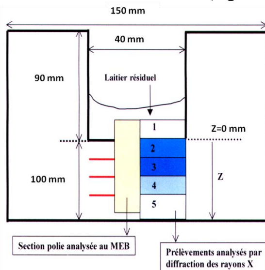
Figure IV-26 Localisation des prélèvements analysés sur un creuset corrodé
