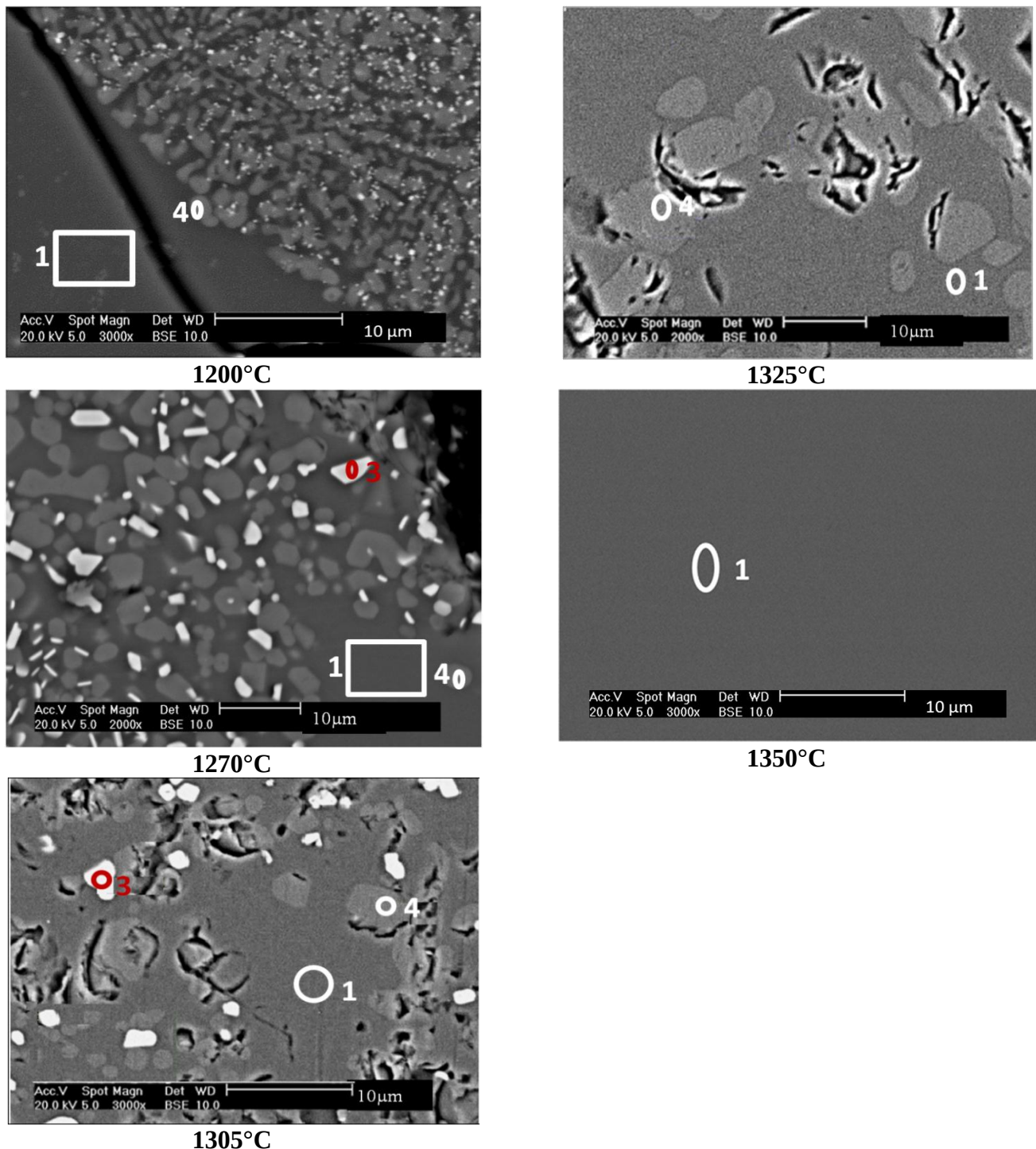
Figure II-40 Microstructures (mode électrons rétrodiffusés) de l'échantillon T en fonction de la température de recuit.
