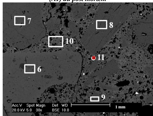
Figure IV-121 Agrandissement (mode électron rétrodiffusés) de l'échantillon A2
