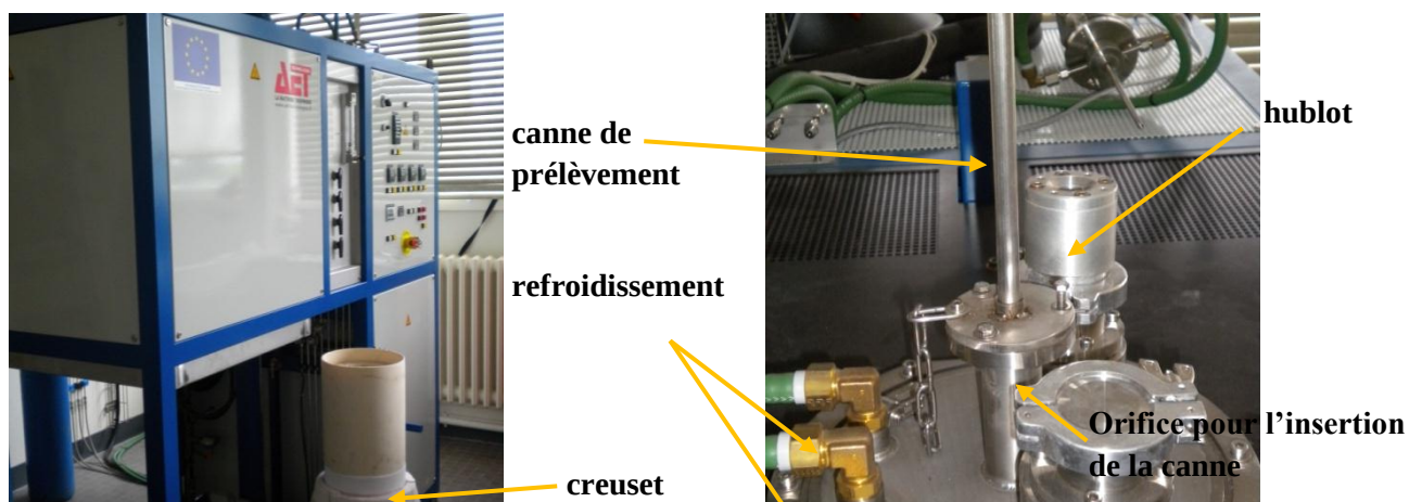
Figure IV-124 Four utilisé pour les essais de cinétique
