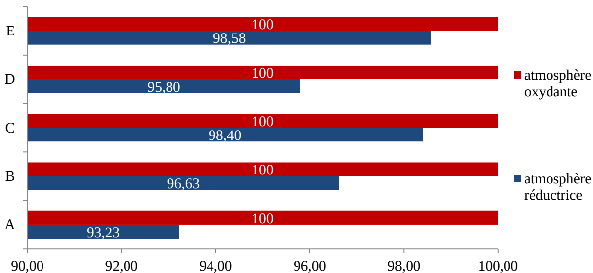
Figure IV-92 Comparaison des taux d'oxygène mesurés sur les interphases de corrosion par EDS après l'essai en atmosphère oxydante et réductrice
