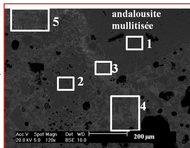
Figure IV-120 Agrandissement (mode électron rétrodiffusés) de l'interphase de corrosion (A1) du post mortem
