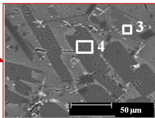
Figure IV-53 cristallisation d'anorthite à l'interphase laitier réfractaire
