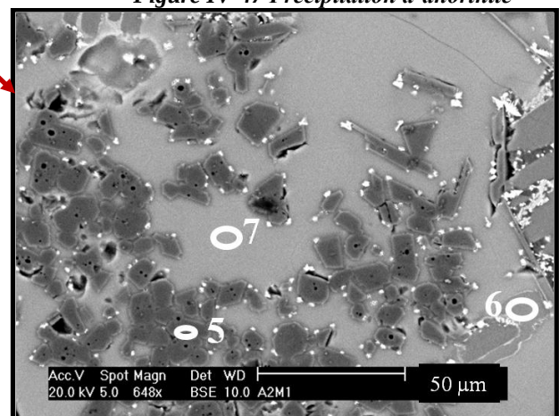
Figure IV-48 Précipitation de mullite
