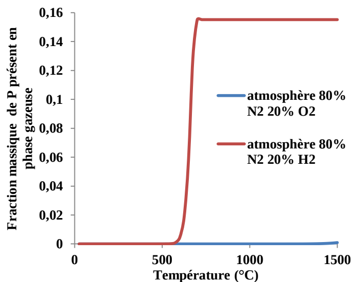
Figure III-5 Fraction massique du phosphore en phase gazeuse en fonction de la température pour le binaire 50% massique CaO - 50% massique P_2O_5
