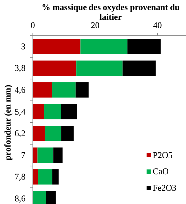
Figure IV-51 Profil chimique (par EDS) des oxydes provenant du laitier en fonction de la profondeur
