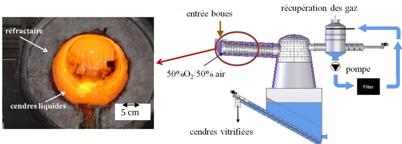
Figure IV-109 Schéma du réacteur de TKEnergy
