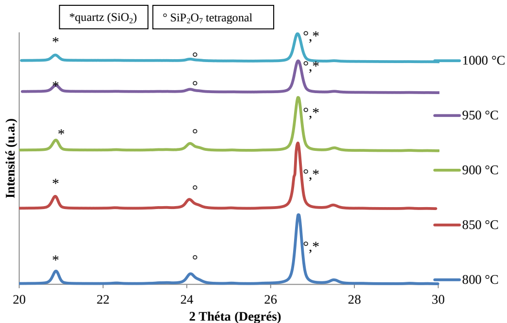
Figure II-20 Cristallisation de l'échantillon 75% \text{SiO}_2 -25% \text{P}_2\text{O}_5 entre 800°C et 1000°C
