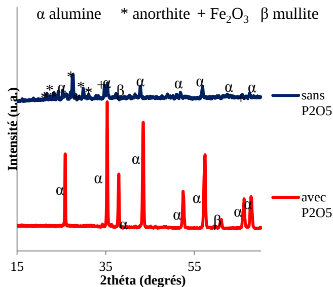
Figure IV-75 Phases cristallisées dans la zone de corrosion du béton B
