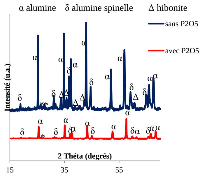
Figure IV-77 Phases cristallisées dans la zone de corrosion du béton D
