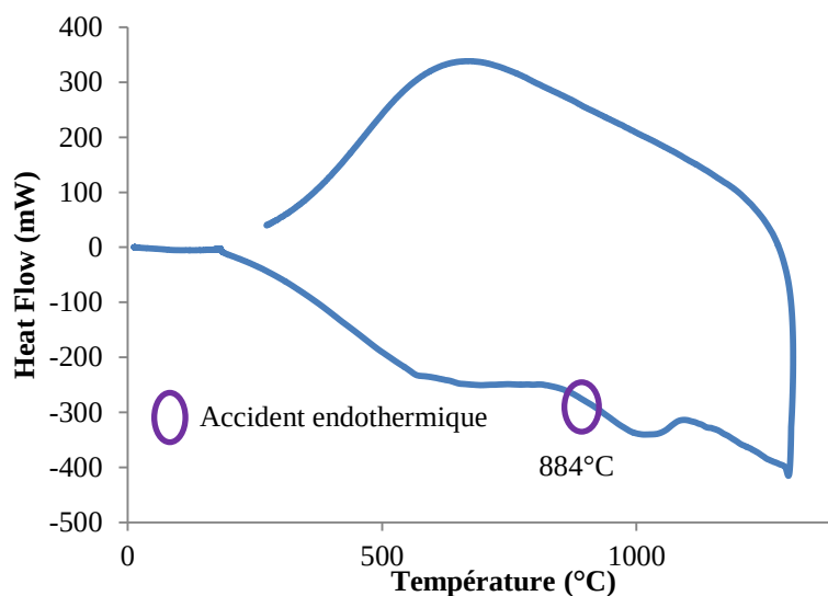
Figure II- 22 analyse thermique différentielle sur l'échantillon 75 % \text{m} \text{SiO}_2 25% \text{m} \text{P}_2\text{O}_5
