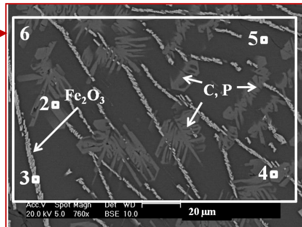
Figure IV-117 Agrandissement (mode électron rétrodiffusés) de l'interphase de corrosion (A1)
