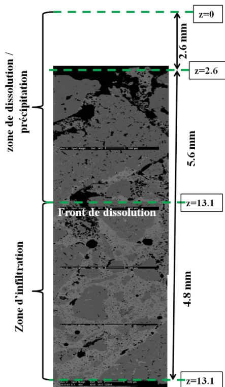
Figure IV-62 Interphase de corrosion du béton D
