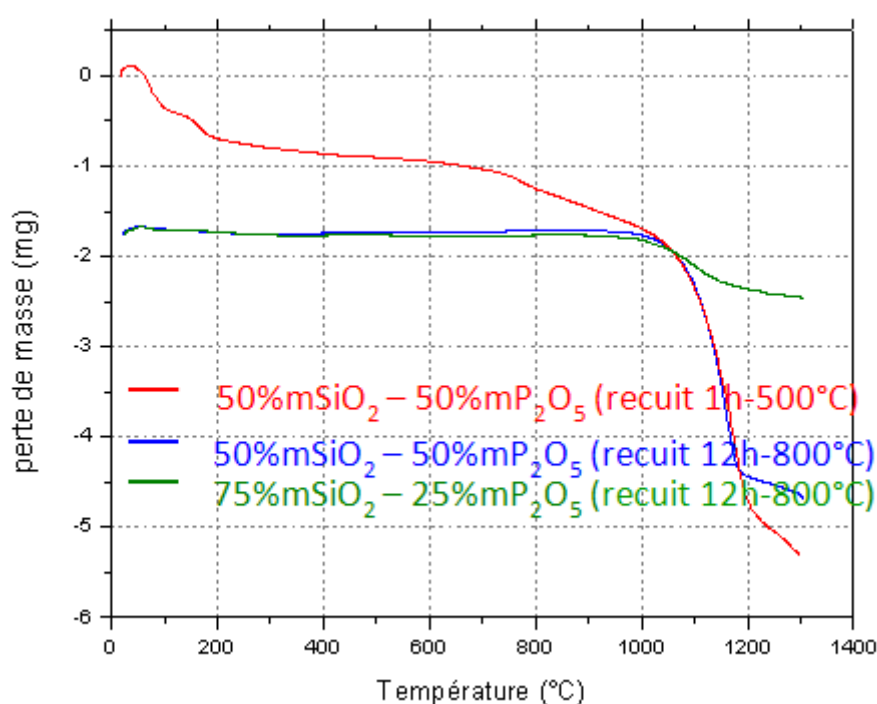
Figure III-10 Courbes ATG pour le binaire 50% SiO_2 -50% P_2O_5 (courbes rouge et bleue) et 75% SiO_2 -25% P_2O_5 (courbe verte) suivant des traitements thermiques différents en fonction de la température.
