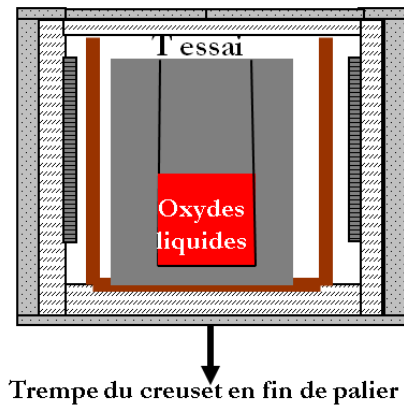
Figure IV- 21 Schéma de l'essai de corrosion statique
