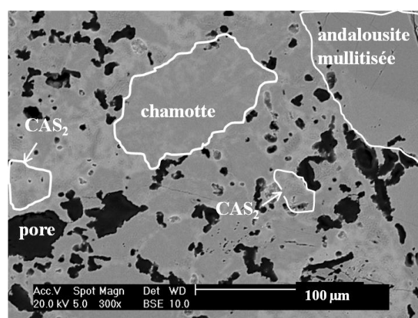
Figure IV-8 Cliché MEB (mode électrons rétrodiffusés) de la partie matricielle du béton A
