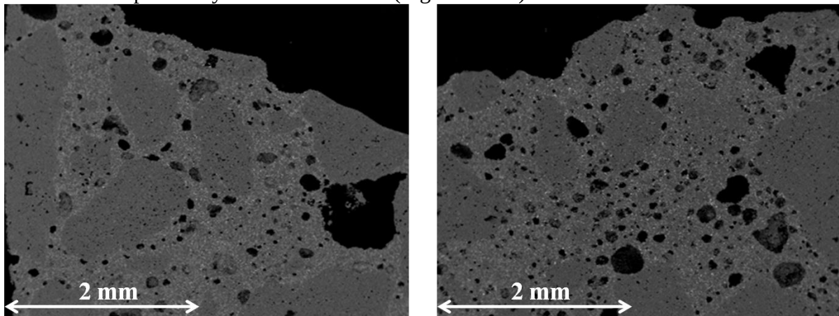
Figure IV-91 Interphases de corrosion du béton C. en atm. oxydante (à gauche) et réductrice (à droite)
