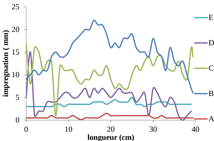
Figure IV-107 profondeur d'imprégnation en fonction de la longueur du claveau
