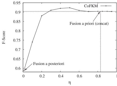
FIGURE 2.6 — CoFKM sur mfeat pour différentes valeurs de \eta . On remarque que l'heuristique de mfeat .
