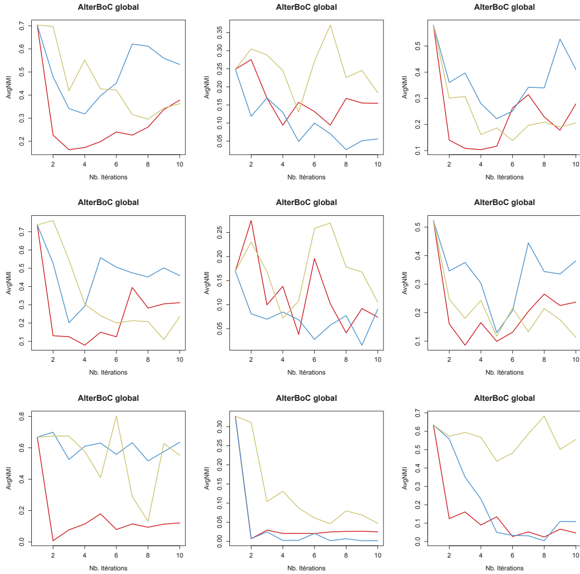
FIGURE 4.7 — Évolution de l' AvgNMI pour la combinaison de modèle et l'heuristique globale. Dans l'ordre, les données iris , parkinson et wine . Les trois lignes correspondent (1) à l'application de deux algorithmes : KM et CLINK, (2) à l'application de quatre algorithmes : KM, SC, SLINK et CLINK, (3) à l'application de six algorithmes : KM, FKM, SC, SLINK, ALINK et CLINK.
