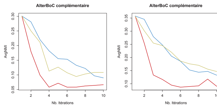
FIGURE 4.10 — Évolution de l' AvgNMI pour le clustering multi-vues et l'heuristique complémentaire. Dans l'ordre, les données mfeat avec le même algorithme pour toutes les six vues, et mfeat avec des algorithmes différents pour chaque vue.
