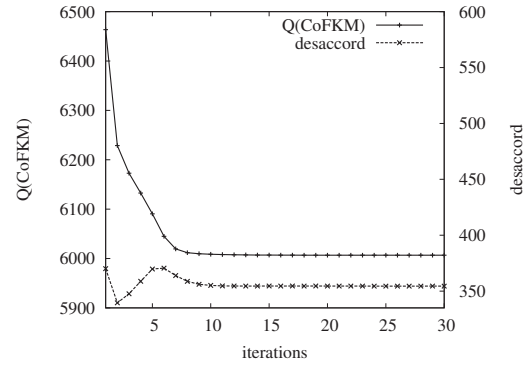
FIGURE 2.7 — Évolution du critère CoFKM sur
