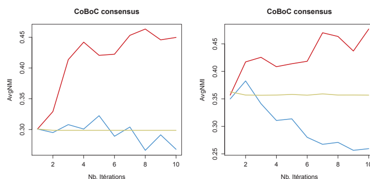
FIGURE 4.5 — Évolution de l' AvgNMI pour le clustering multi-vues et l'heuristique consensus. Dans l'ordre, les données mfeat avec le même algorithme pour toutes les six vues, et mfeat avec des algorithmes différents pour chaque vue.
