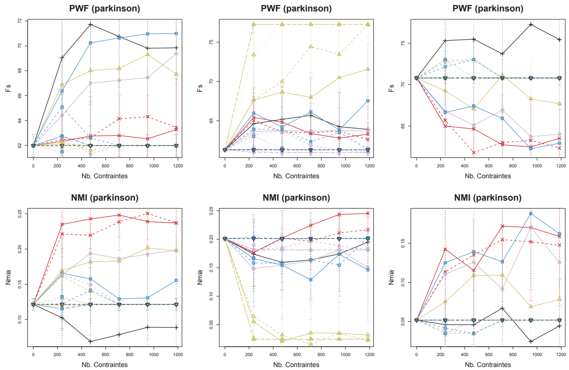
FIGURE 3.16 — Comparaison des approches BOC, UzABOC, ADAUzABOC et BC sur Parkinson centré et réduit.
