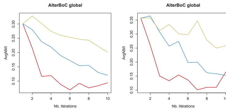
FIGURE 4.9 — Évolution de l' AvgNMI pour le clustering multi-vues et l'heuristique global. Dans l'ordre, les données mfeat avec le même algorithme pour toutes les six vues, et mfeat avec des algorithmes différents pour chaque vue.
