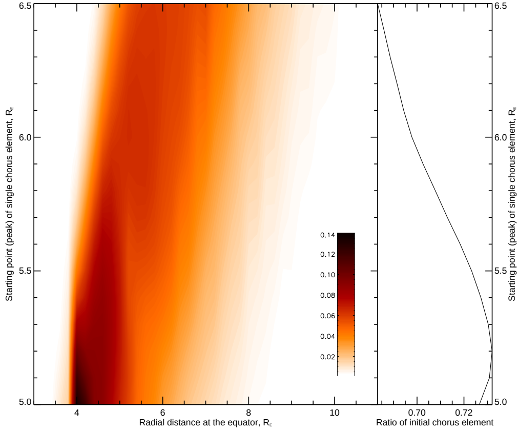
Fig. 5.5: La fonction de densité de probabilité de la distribution de puissance d'onde d'un élément de chœur dans le plan équatorial en fonction de sa distance initiale L_m (axe x), pour différentes valeurs de L_m (axe y). Chaque distribution (ligne) est obtenue d'un élément de chœur généré à l'équateur, centré à L_m et pondéré par l'Equ.(5.1). A l'image de la figure précédente, chaque élément est unidimensionnel, mais la distribution de puissance d'onde réfléchiée est considérée unidimensionnelle ici aussi, i.e. on néglige ses variations selon Y . Sur le panneau de droite est montré, en fonction de L_m , le ratio du nombre de rayons réfléchis atteignant l'équateur par rapport au nombre total de rayons présents dans le SCE initial.
