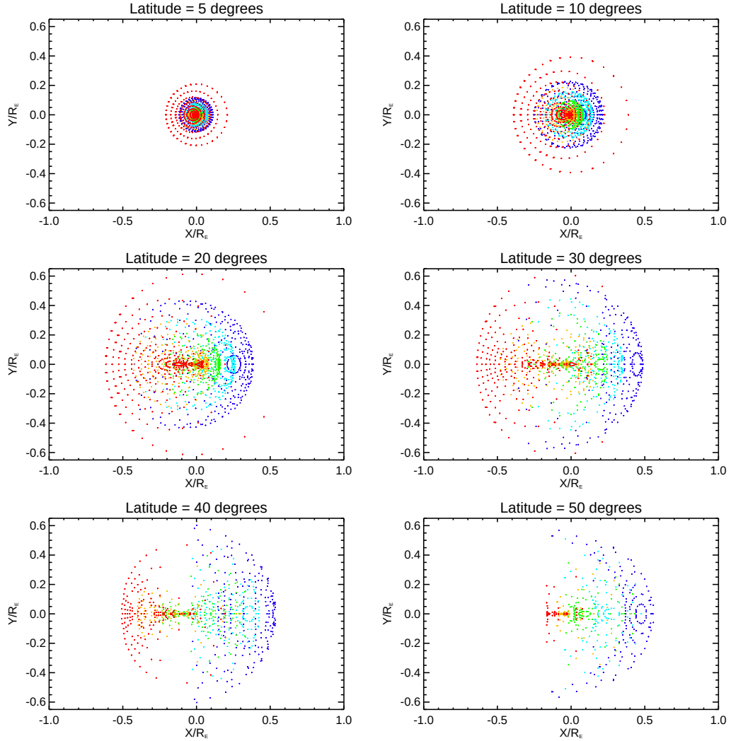
Fig. 4.5: Divergence spatiale (X/R_E, Y/R_E) le long de la coquille magnétique L = 5 d'un paquet d'ondes choeur depuis l'équateur vers l'hémisphère nord, dans différents plans de latitude (ces plans sont décrits dans la Fig.4.6). Les couleurs représentent les différentes fréquences, ce paquet d'ondes étant aussi constitué de rayons de différents angles latitudinaux 5^\circ \leq \theta_0 \leq \theta_{res} et azimutaux -180^\circ \leq \varphi_0 \leq 180^\circ . Cette divergence est donc incluse dans les statistiques réalisées à l'aide du code numérique.
