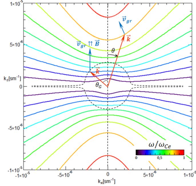
Fig. 4.7: Surfaces d'indice de réfraction calculées pour des paramètres typiques d'ondes de type chœur dans la magnétosphère interne ( L = 6 ), à l'équateur magnétique. Les différentes couleurs indiquent les différentes fréquences, normalisées par rapport à la gyrofréquence équatoriale.
