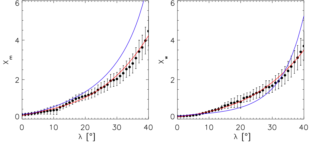
Fig. 4.14: Valeur moyenne X_m (panneau de gauche) et variance X_w (panneau de droite) de la distribution de \tan \theta , en fonction de la latitude magnétique. Cette figure montre la comparaison quantitative entre les valeurs obtenues par les données statistiques de CLUSTER STAFF-SA (cercles), leur ajustement (ligne rouge) et nos simulations numériques (ligne bleue) pour les ondes de type choeur.
