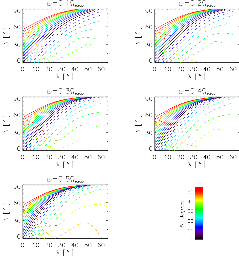
Fig. 4.10: Variation de \theta en fonction de la latitude pour des rayons, lancés depuis l'équateur ( L = 6 ), de différentes fréquences et de différents angles \theta_0 (en couleur). Les tirets représentent les rayons lancés initialement vers la Terre ( \varphi_0 = 180^\circ ) et les lignes solides représentent les rayons initialement lancés dans la direction opposée ( \varphi_0 = 0^\circ ).
