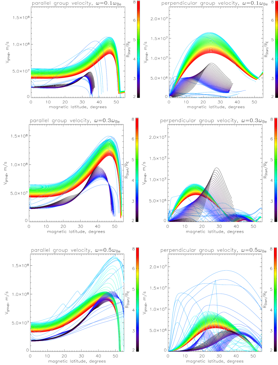
Fig. 4.4: Illustration de la vitesse groupe de différents rayons en fonction de la latitude \lambda pour des points de génération différents (couleur) et des fréquences de choeur de basse-bande différentes (lignes). La colonne de gauche représente la composante parallèle de la vitesse de groupe et la colonne de droite représente la composante perpendiculaire. Les rayons présentés dans cette figure sont générés parallèlement au champ magnétique ( \theta_0 = 0^\circ ).
