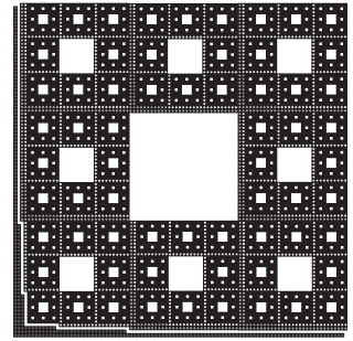
(c) Un tapis de Sierpiński auto-assemblant [Patitz et Summers 2010, Fig. 14].
