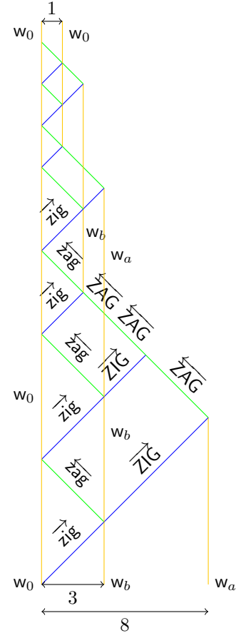
FIGURE 4.6 – La machine \mathfrak{M}_{pgcd} : algorithme d'Euclide géométrique.
