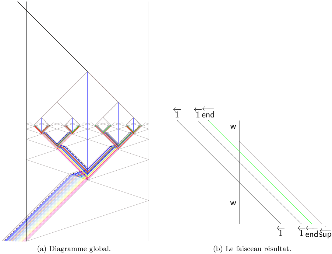
FIGURE 9.3 – Résolution de \#SAT pour l'instance \varphi = x_1 \wedge (\neg x_2 \vee x_3) . Le faisceau sortant en haut à gauche représente le nombre 3 en binaire, qui correspond au nombre d'assignments satisfaisant \varphi .
