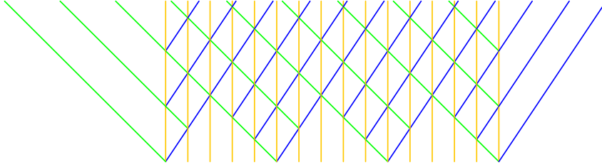
FIGURE 4.12 – Une (\frac{2}{3}, 5, 0, 1, 3) – multi-bande : elle est constituée de trois (\frac{2}{3}, 5, 0, 1) – Bandes, c'est-à-dire 3 bandes, toutes de largeur 1, ayant chacune 5 sous-divisions, et dont la première bande commence en position 0.
