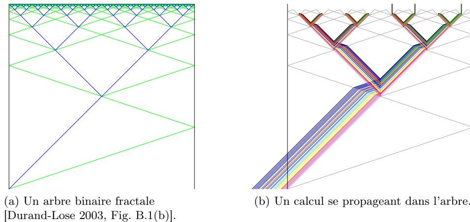
FIGURE 3 – Distribuer un calcul grâce à une structure fractale.
