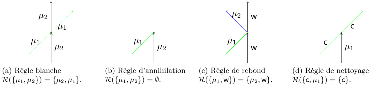
FIGURE 2.2 – Quelques formes utiles de règles de collisions.
