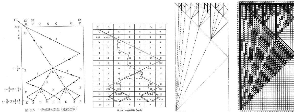
(a) La solution continue de Goto et sa version discrétisée [Goto 1966, Fig. 3].
