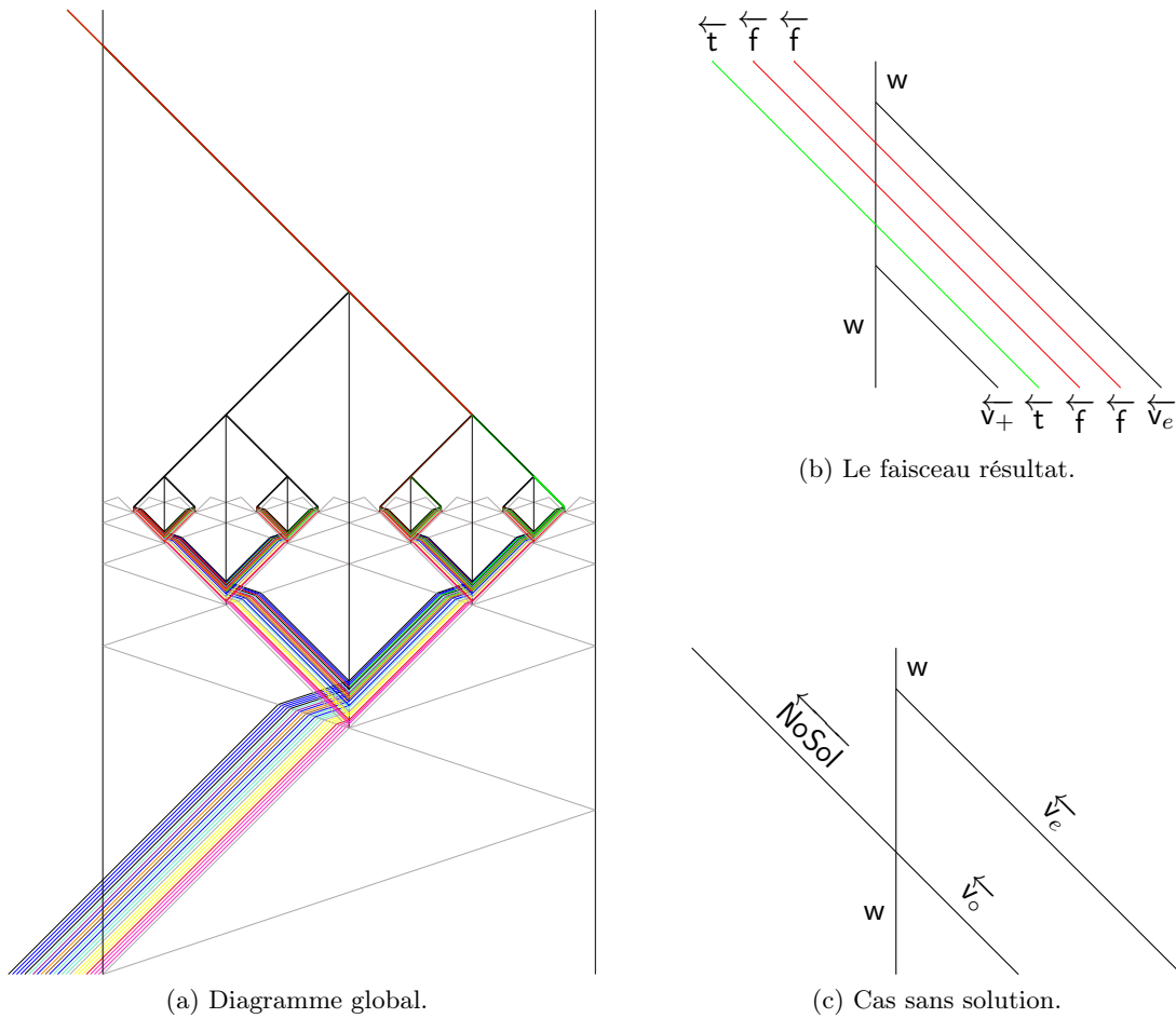
FIGURE 9.6 – Résolution de ONE-SAT pour l'instance \varphi = x_1 \wedge (\neg x_2 \vee x_3) . L'assignation (x_1, x_2, x_3) = (vrai, faux, faux) est une solution (la première dans l'ordre lexicographique), donnée sous forme de faisceau sortant en haut à gauche de la construction.
