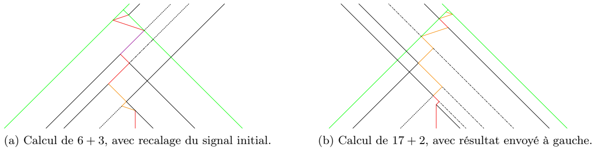
FIGURE 3.5 – Autres exemples d'additions binaires géométriques.
