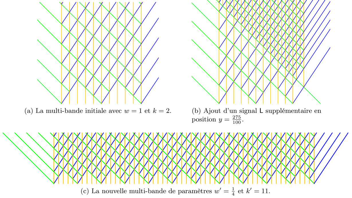
FIGURE 4.14 – Exemple d'ajout d'un signal \mathbf{L} en position y = \frac{275}{100} à une (\frac{2}{3}, 5, 0, 1, 2) – multi-bande. Les nouveaux paramètres obtenus sont w' = \text{pgcd}(w, y) = \text{pgcd}(1, \frac{275}{100}) = \frac{1}{4} et k' = \frac{y}{w'} = \frac{275/100}{1/4} = 11 , et la nouvelle multi-bande est donc une (\frac{2}{3}, 5, 0, \frac{1}{4}, 11) – multi-bande.
