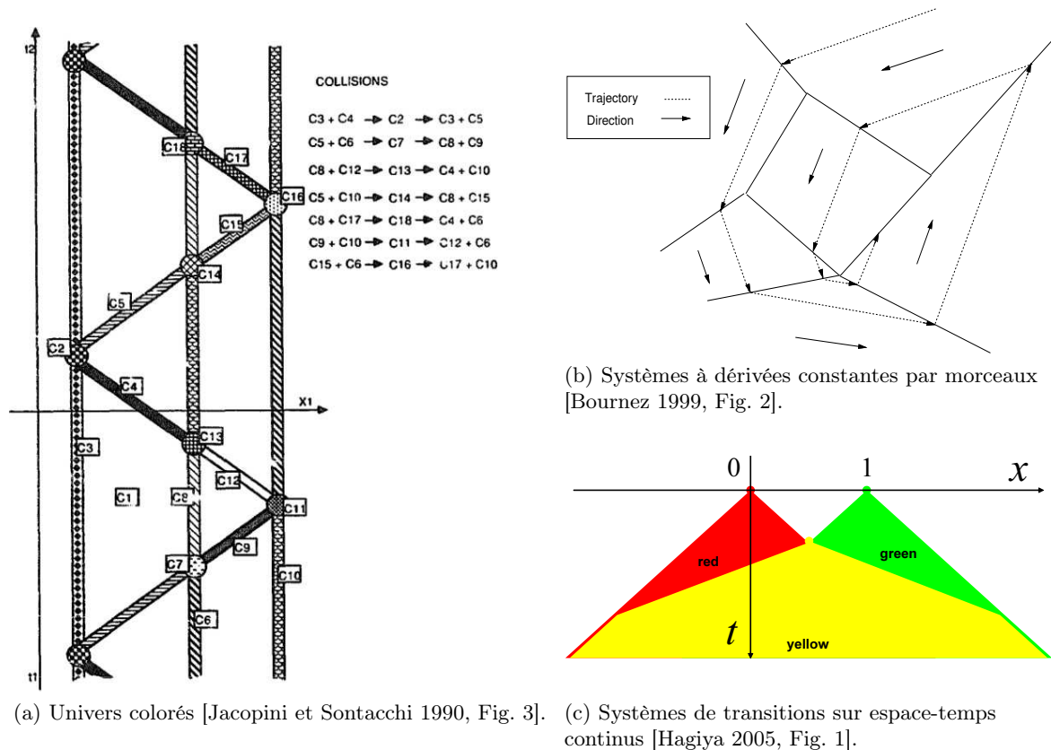
FIGURE 1.1 – Exemples de modèles géométriques de calcul.
