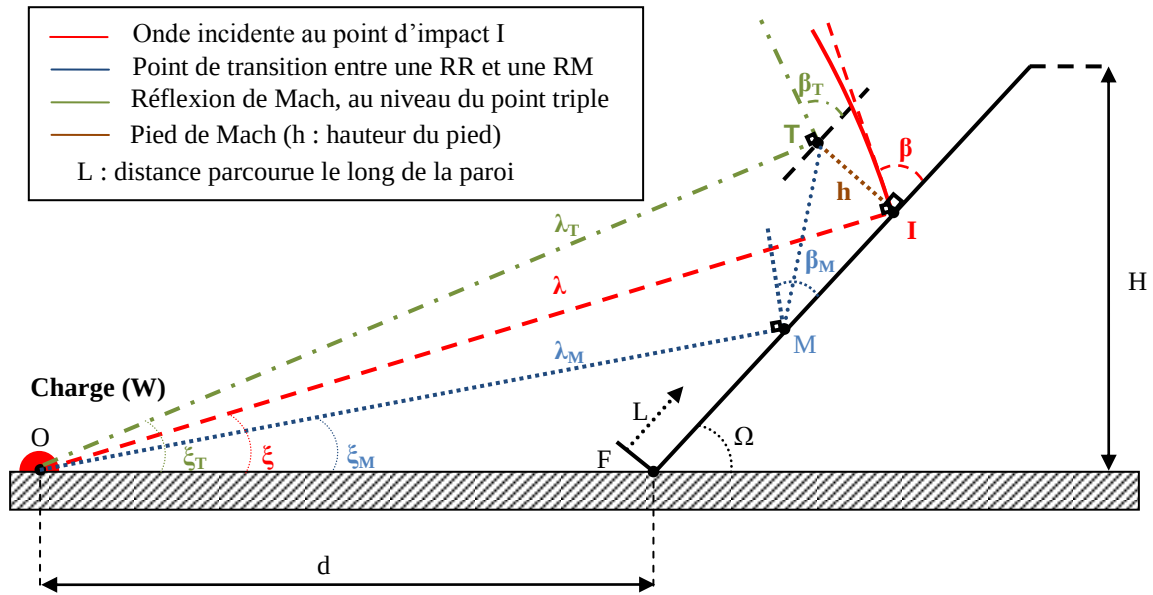
Figure 19 : Représentation schématique de l'onde incidente et de l'onde réfléchi pour une surface plane
