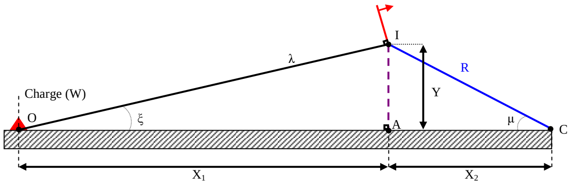
Figure A14 : Représentation du triangle OCI
