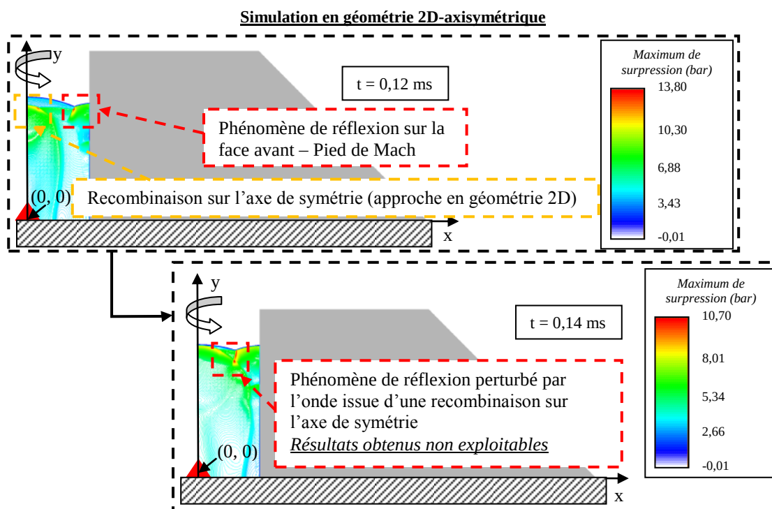
Figure 132 : Visualisation sur les champs de pression pour le merlon 2B en géométrie 2D-axisymétrique (configuration 2B C6 d7)
