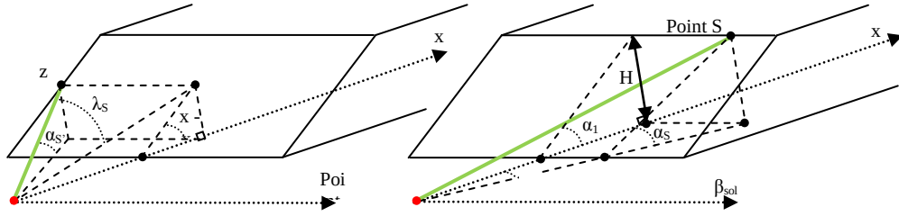
Figure A31 : Représentation des points de sortie S' et S sur la face avant de la barrière
