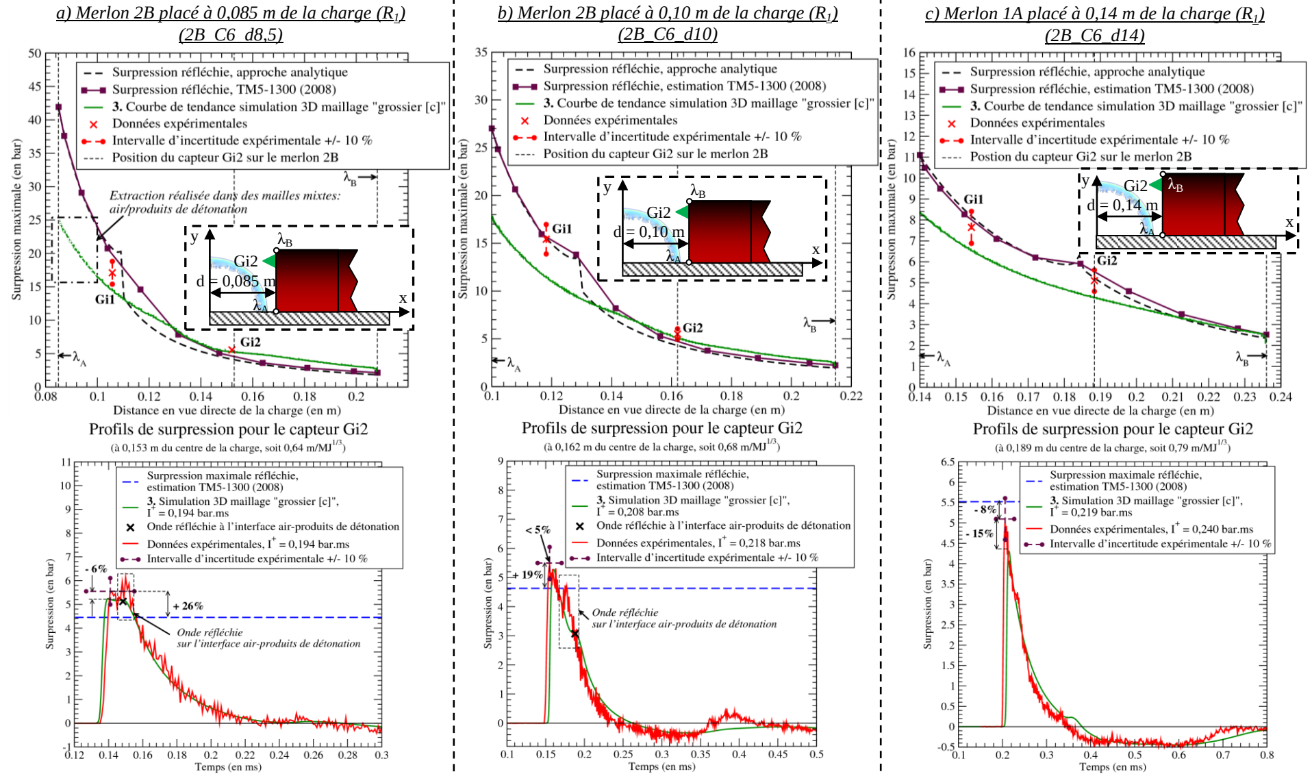
Figure 137 : Evolution du maximum de surpression réfléchi sur la face avant du merlon 2B
