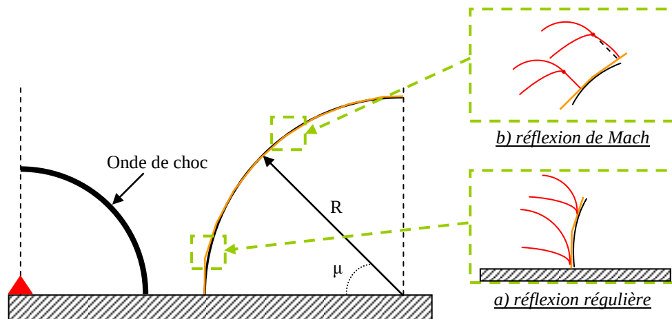
Figure A24 : Représentation schématisée de l'interaction d'une onde de choc avec une paroi convexe
