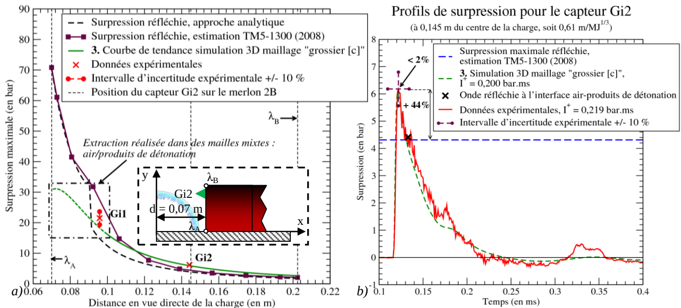
Figure 133 : Evolution du maximum de surpression réfléchie sur la face avant du merlon 2B placé à 0,07 m d'une charge gazeuse de rayon ( R_1 ) (2B C6 d7, soit 0,29 m/MJ 1/3 )
