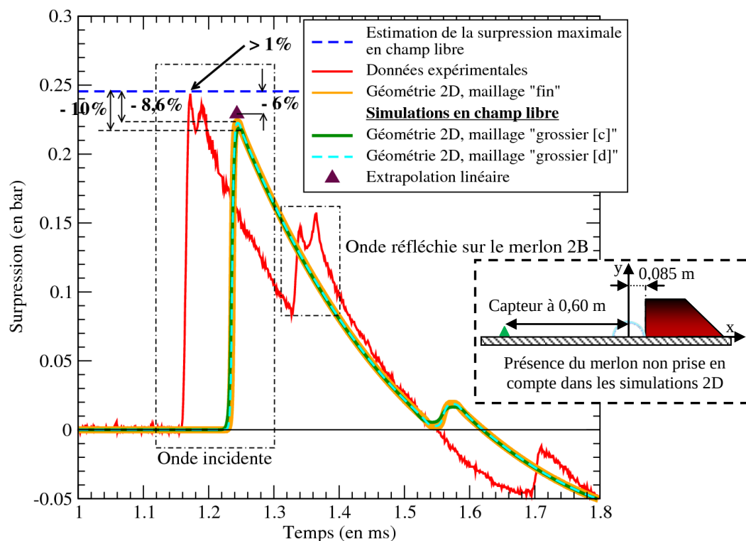
Figure 164 : Profils de surpression pour un capteur de référence du merlon « court » 2B
