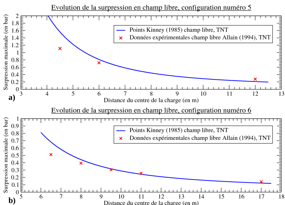
Figure 34 : Analyse des écarts expérimentaux / bibliographiques pour une charge sphérique de 8 kg de TNT
