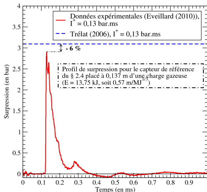
Figure 69 : Profil de surpression de l'étude préliminaire du projet ANR BARPPRO (Eveillard (2010))
