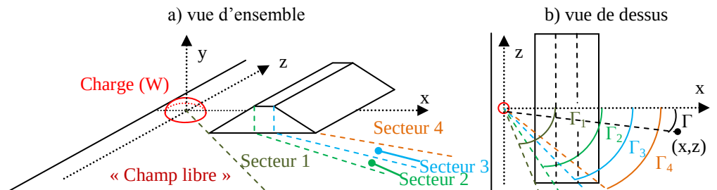
Figure 156 : Définition des secteurs géométriques autour de la barrière
