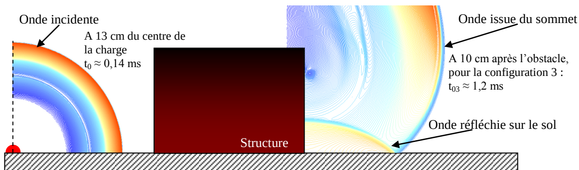
Figure 83 : Représentation schématique de la détente et de la réflexion sur le sol après l'obstacle de la configuration 3
