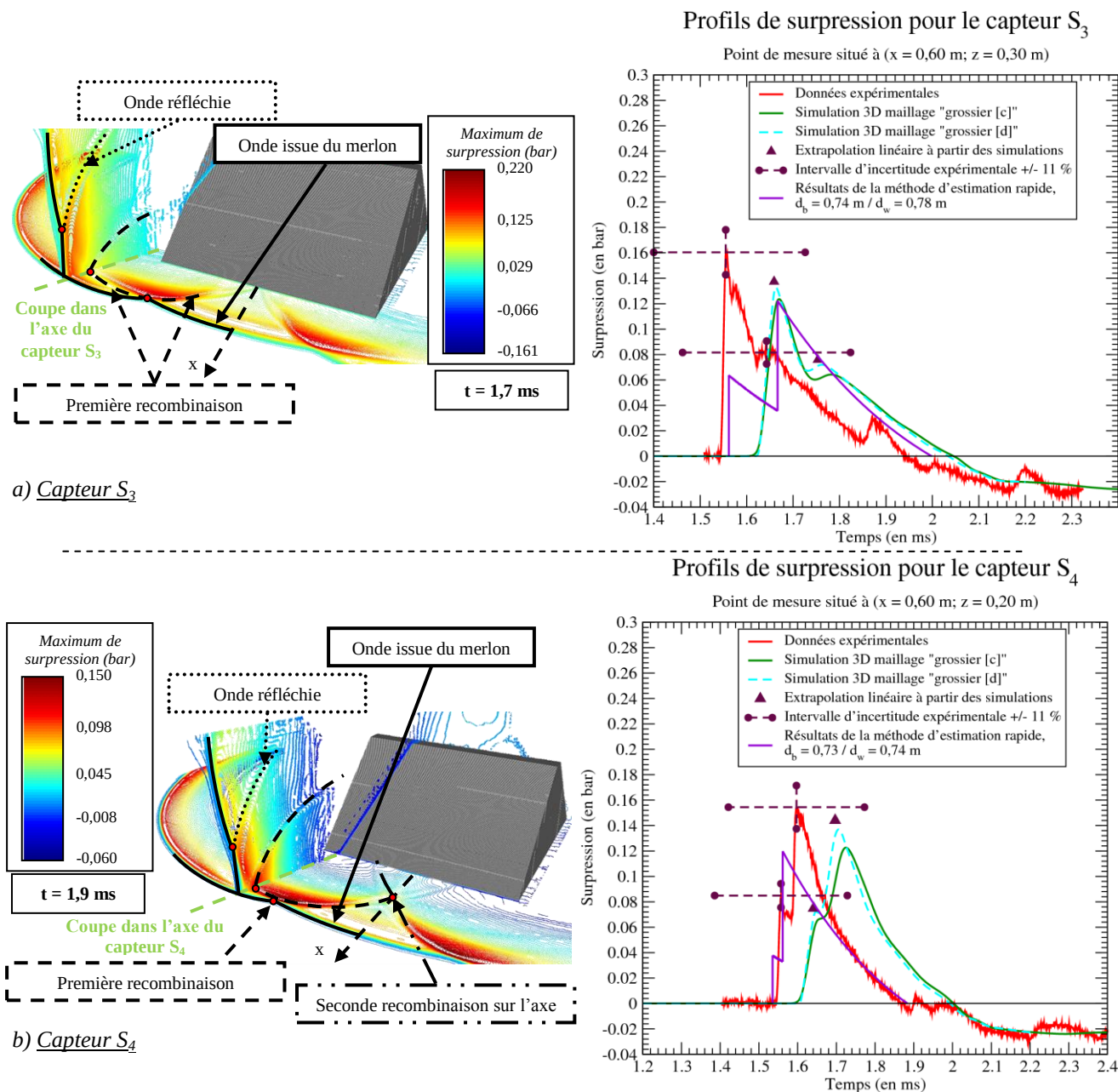
Figure 168 : Visualisations des champs et des profils de surpression pour les capteurs S_3 et S_4 du merlon 1A « court »
