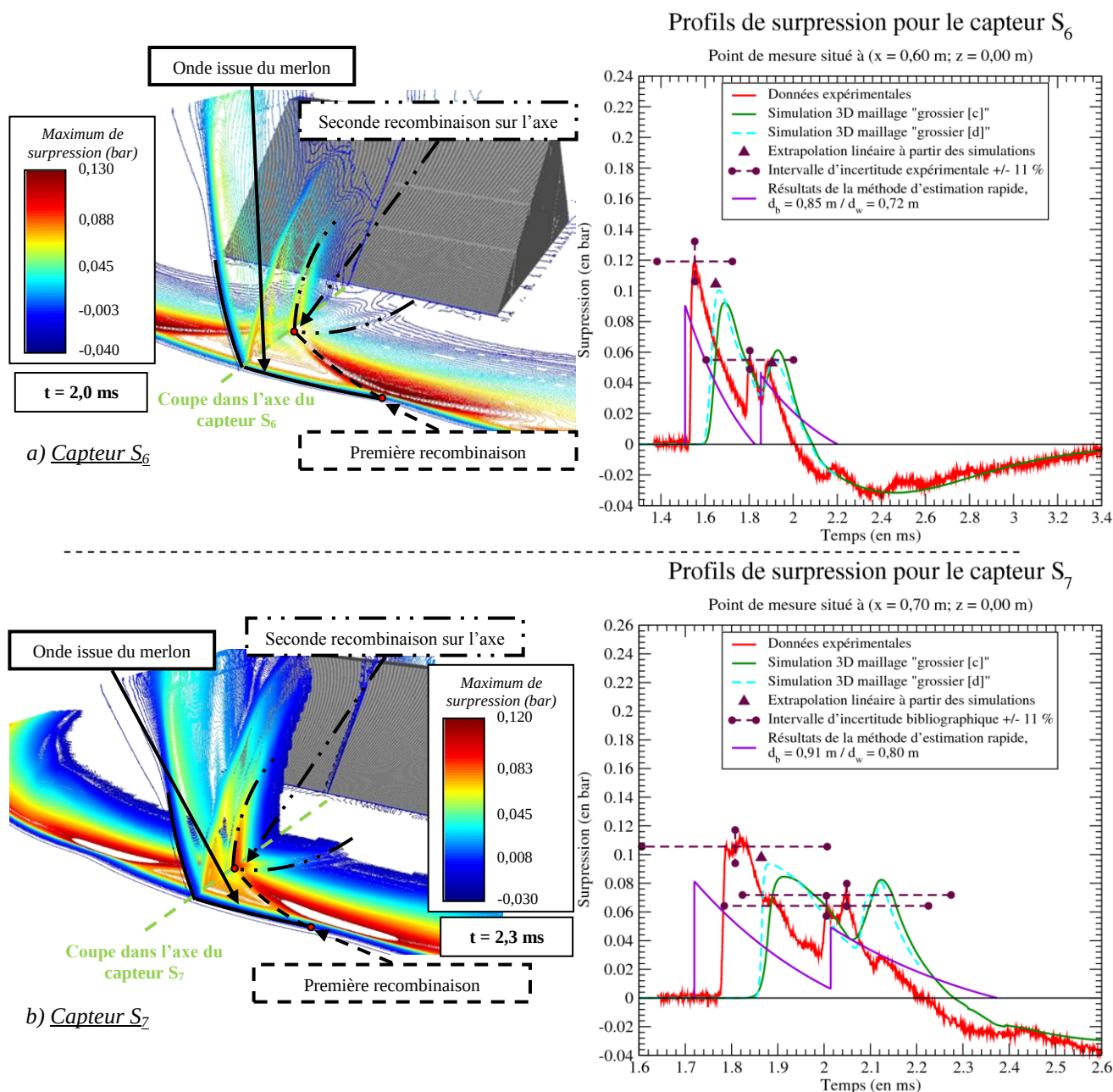
Figure 170 : Visualisations des champs et des profils de surpression pour les capteurs S_6 et S_7 du merlon 1A « court »
