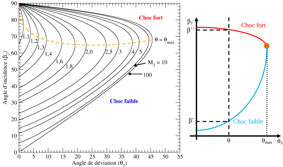
Figure 16 : Evolution de l'angle d'incidence de l'onde réfléchi en fonction du nombre de Mach et de l'angle de déviation de l'état 2
