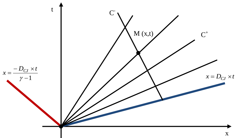
Figure 8 : Droites caractéristiques C^+ et C^- lors de la détonation de la charge explosive
