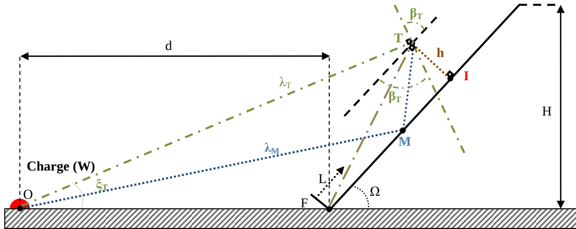
Figure 22 : Représentation schématique d'une réflexion de Mach au point d'impact I
