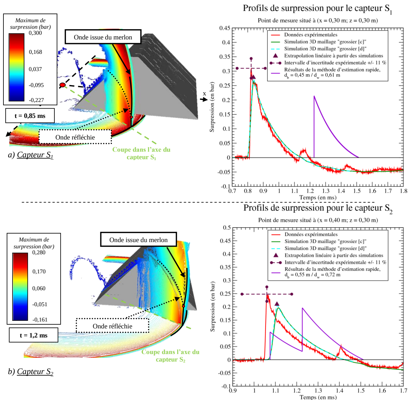
Figure 167 : Visualisations des champs et des profils de surpression pour les capteurs S_1 et S_2 du merlon 1A « court »
