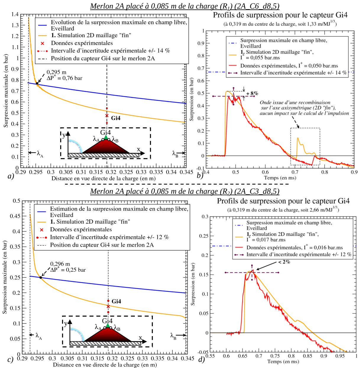
Figure 118 : Evolution du maximum de surpression au sommet du merlon 2A
