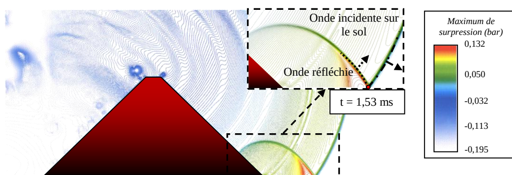
Figure 124 : Visualisation sur les champs de pression pour le phénomène de réflexion en aval de la barrière de protection (configuration 1A_C6_d7)
