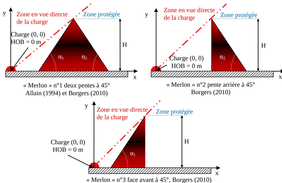
Figure 32 : Représentation schématisée des configurations étudiées par Borgers (2010) et Allain (1994)
