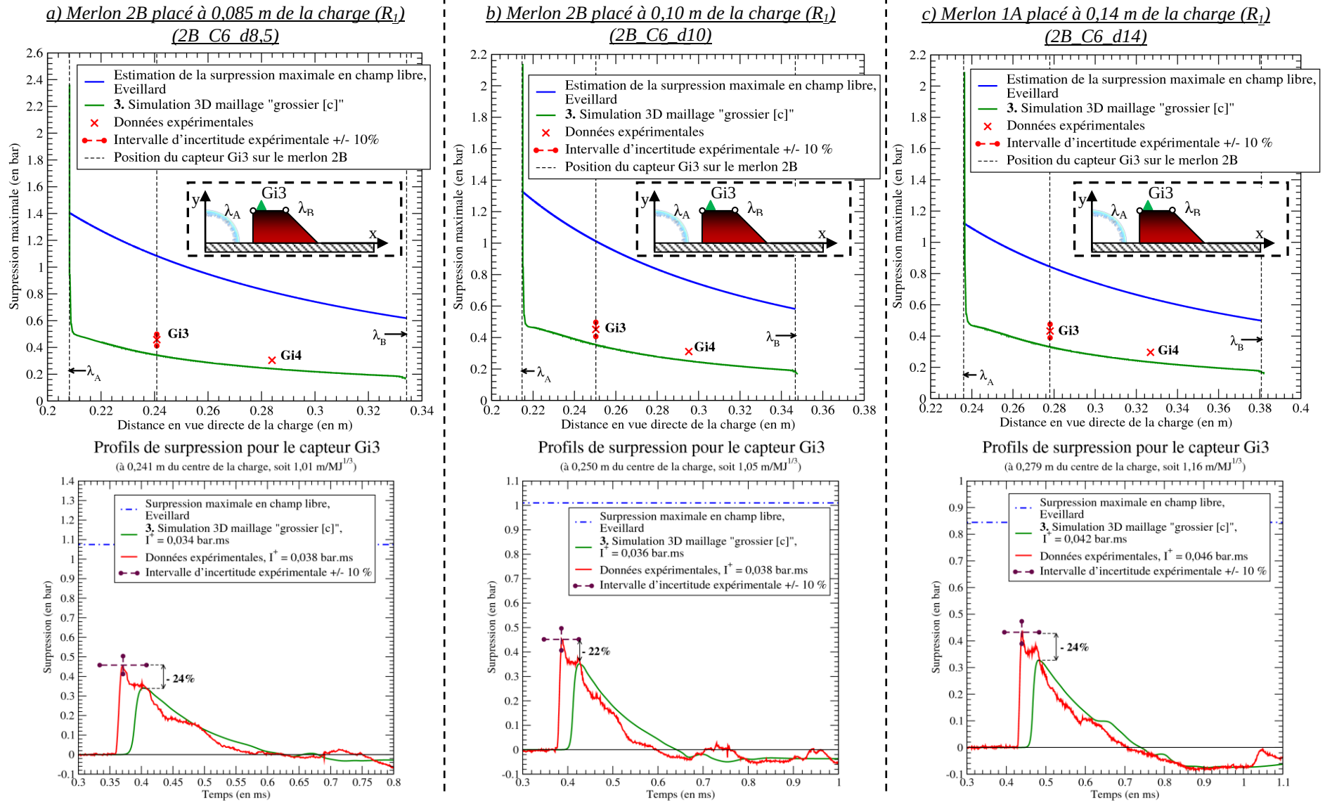
Figure 142 : Evolution du maximum de surpression au sommet du merlon 2B
