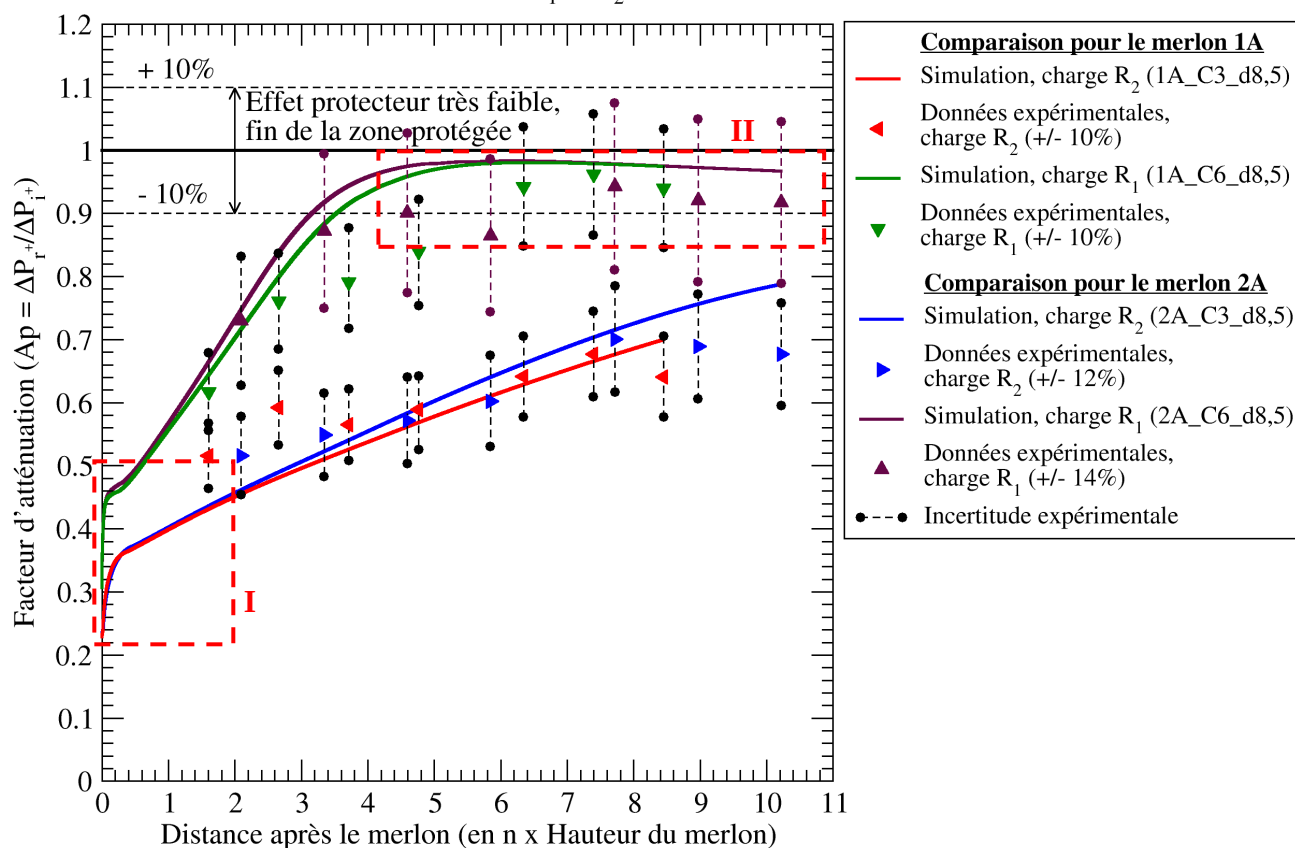
Figure 127 : Evolution du facteur d'atténuation en aval du merlon pour les deux charges gazeuses étudiées
