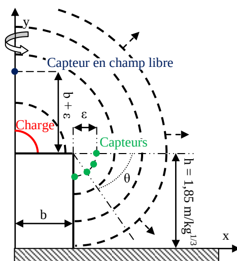
Figure 154 : Représentation schématisée de la configuration étudiée pour le phénomène de détente
