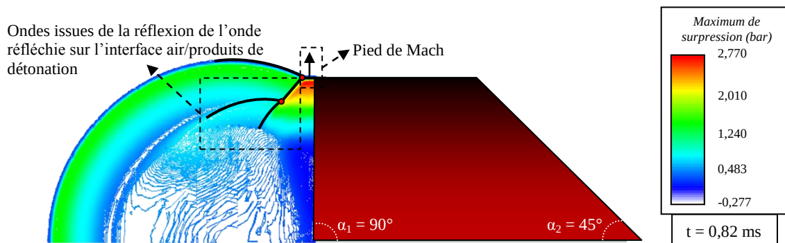
Figure 138 : Visualisation sur les champs de pression lors du phénomène de réflexion sur la face avant de la barrière de protection (configuration 2B C6 d10)
