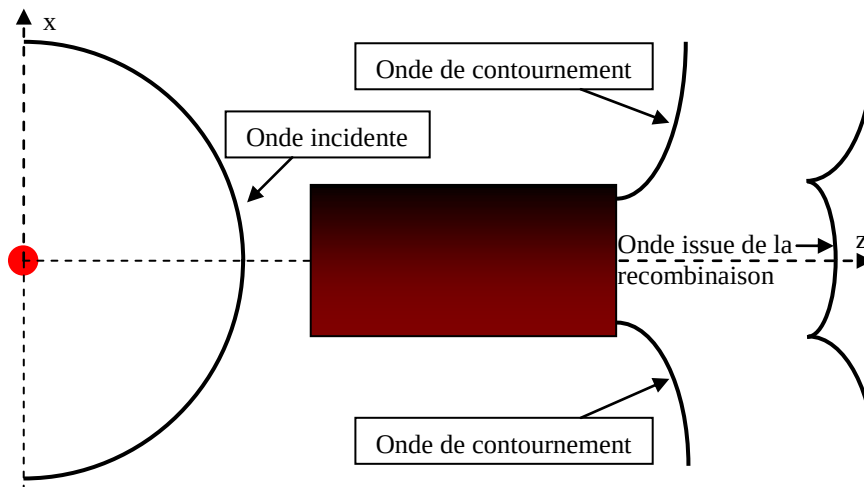
Figure 86 : Représentation schématisée du contournement de l'onde de choc pour la configuration 2, vue du dessus
