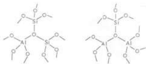
Figure 74. Représentation des triclusters 1\text{AlO}_4 , 2\text{SiO}_4 et 1\text{SiO}_4 , 2\text{AlO}_4 selon le modèle de Lacy [37].
