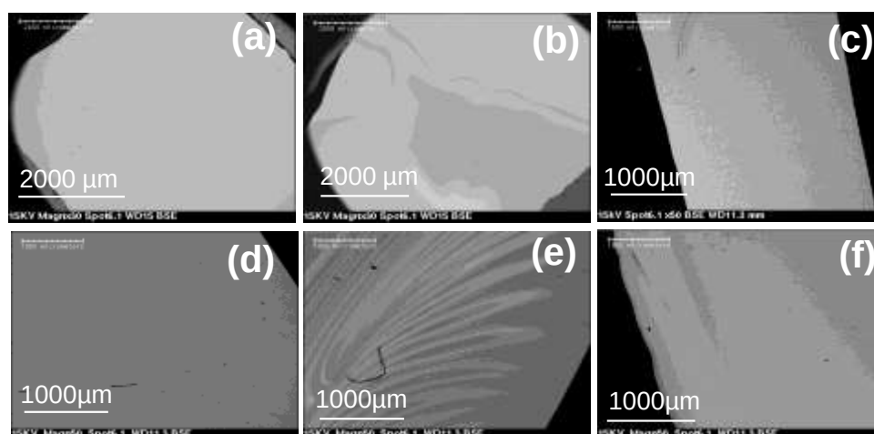
Figure 86. Clichés MEB en électrons rétrodiffusés des verres étalons (a) SiAlLa (b) BAiLa (c) B20TR0 (d) B20La4Na (e) B20La4Ca (f) B20La14-(0NaCa).
