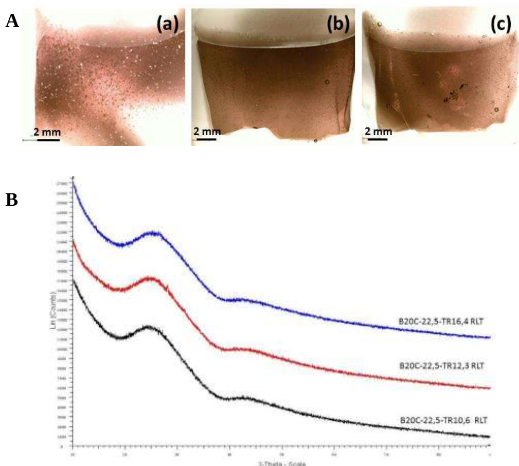
Figure 28. (A) Observations au microscope optique des verres refroidis en température à 1^\circ\text{C}/\text{min} de la série B20C à teneur en terres rares croissantes (a) B20C-22,5-TR10,6 RLT (b) B20C-22,5-TR12,3 RLT et (c) B20C-22,5-TR16,4 RLT. (B) Diffractogrammes de rayons X correspondants aux différents verres.
