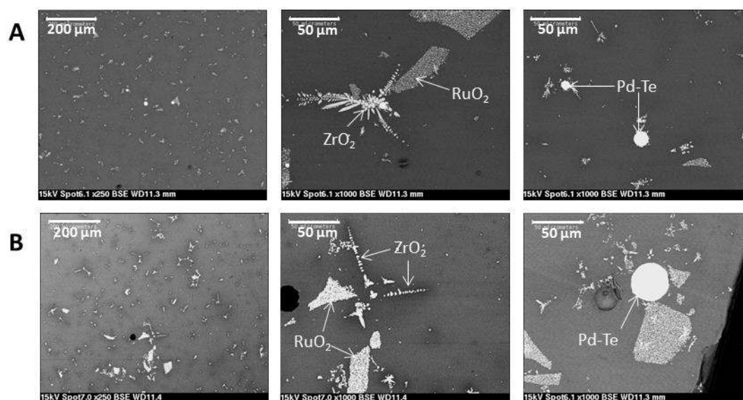
Figure 26. Clichés MEB en électrons rétrodiffusés des verres contenant des platinoïdes après refroidissement en température à 1^\circ\text{C}/\text{min} (RLT) (A) B20C-22,5(P) RLT et (B) B20C-22,5(P+F) RLT.
