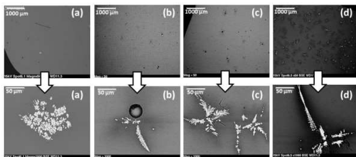
Figure 22. Clichés MEB en électrons rétrodiffusés des verres de la série B20C à teneur en PFA variable et refroidis à 1°C/min (a) B20C-18,5 RLT (b) B20C-22,5 RLT (c) B20C-25 RLT et (d) B20C-32 RLT.
