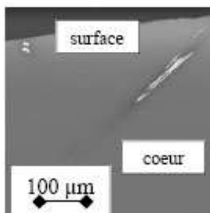
Figure 5. Cliché MEB en électrons rétrodiffusés du verre A ayant subi une descente en température à 1°C/min, et présentant quelques rares cristaux d'apatite \text{Ca}_2\text{Nd}_8(\text{SiO}_4)_6\text{O}_2 en surface de l'échantillon (en blanc sur la figure) [23].
