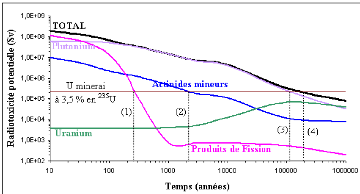
Figure 1. Evolution au cours du temps de l'inventaire radiotoxique pour un combustible utilisé "UOX1" (enrichi à 3,5 % d' 235 U), exprimé en sievert/tonne de métal lourd initial (Sv/tmli). Les repères (1), (2), (3) et (4) précisent le temps nécessaire pour que la radiotoxicité potentielle respectivement des produits de fission, des actinides mineurs, du plutonium et de la totalité du colis devienne inférieure à celle du minerai d'uranium initial enrichi à 3,5 % en 235 U.
