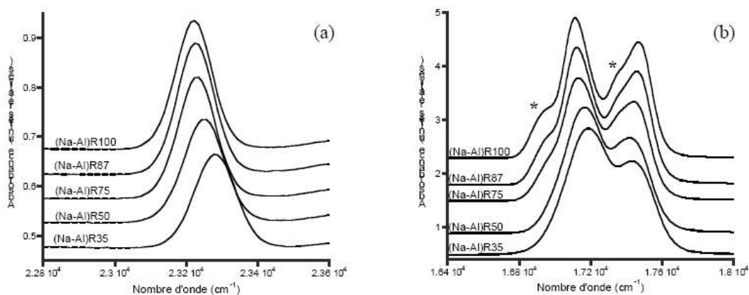
Figure 83. Spectres d'absorption optique présentant les bandes correspondant aux transitions (a) ^4I_{9/2} \rightarrow ^2P_{1/2} et (b) ^4I_{9/2} \rightarrow ^2G_{7/2} , ^4G_{5/2} pour les verres présentant un rapport peralcalin/peralumineux variable [99,100].
