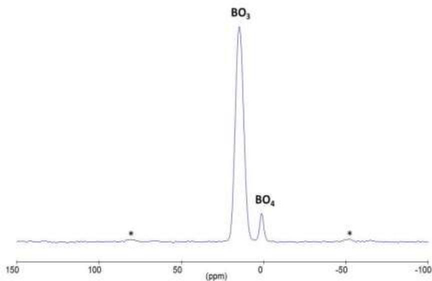
Figure 146. Spectre ^{11}\text{B} MAS ( B_0=18,8 T, \nu_r=22 kHz). * : bandes de rotation de la transition satellite.
