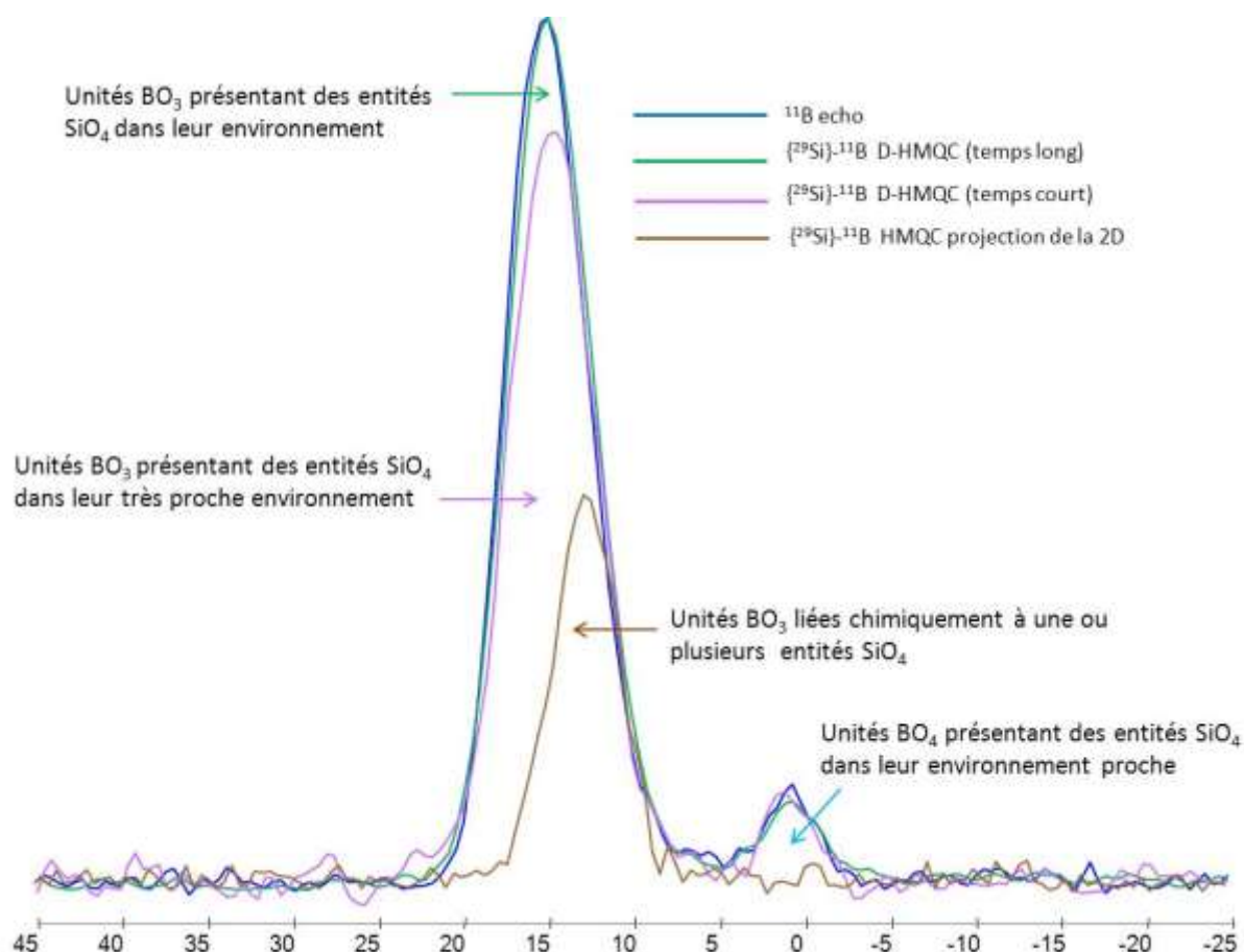
Figure 132. Comparaison de la projection dans la dimension directe ( ^{11}\text{B} ) des spectres ^{29}\text{Si}/^{11}\text{B} 2D HMQC et DHMQC avec le spectre ^{11}\text{B} MAS correspondant pour le verre B14La10-E.
