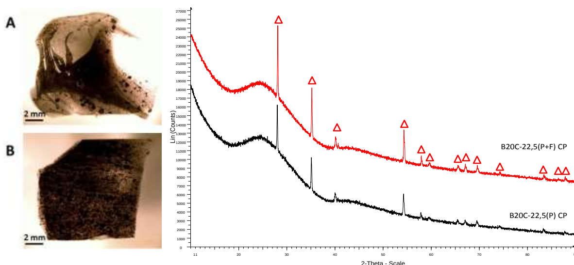
Figure 12. Observations au microscope optique des verres (A) B20C-22,5(P) CP (avec platinoïdes) et (B) B20C-22,5(P+F) CP (avec fines et platinoïdes) et diffractogrammes de rayons X des verres correspondants. ( \Delta ) : \text{RuO}_2 (JCPDS 40-1290).
