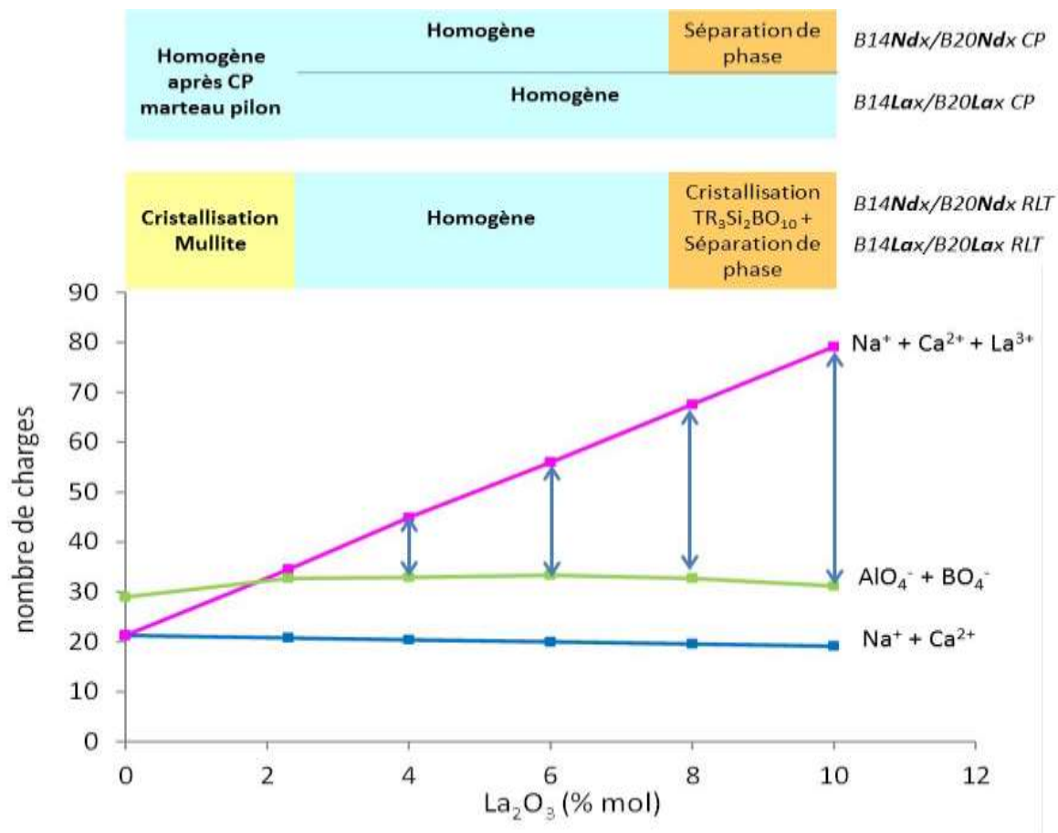
Figure 138. Schéma récapitulatif des résultats microstructuraux et structuraux obtenus sur les verres des séries B14TRx et B20TRx. Les flèches bleues représentent l'excès de charges \text{Na}^+ + \text{Ca}^{2+} + \text{TR}^{3+} vis-à-vis de la compensation de charge des entités \text{AlO}_4 et \text{BO}_4 . CP : coulée sur plaque, RLT : refroidissement à 1°C/min.
