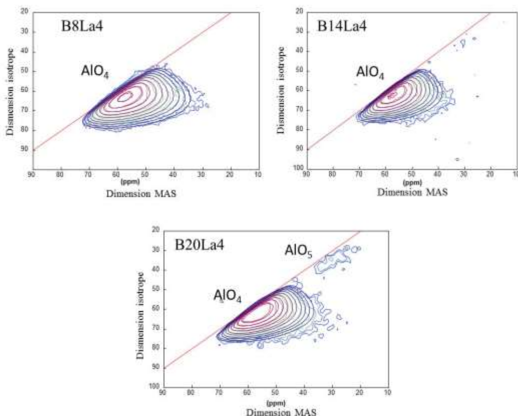
Figure 100. Spectres RMN ^{27}\text{Al} MQMAS expérimentaux (en couleur) et simulés (tracé violet) des verres B8La4, B14La4 et B20La4 coulés sur plaque ( B_0=17,6 T, \nu_r=30 kHz).
