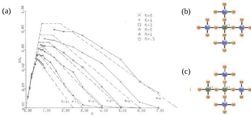
Figure 79. (a) Variation de N_4 mesurée par RMN en fonction du rapport R = [\text{Na}_2\text{O}]/[\text{B}_2\text{O}_3] et K = [\text{SiO}_2]/[\text{B}_2\text{O}_3] . Les traits hachurés correspondent au modèle décrit ci-dessus [79]. (b) Représentation structurale d'une unité reedmergnerite (1 \text{BO}_4 pour 4 \text{SiO}_4 ) et (c) Représentation structurale d'une unité danburite (1 \text{BO}_4 pour 3 \text{SiO}_4 et 1 \text{BO}_4 ).
