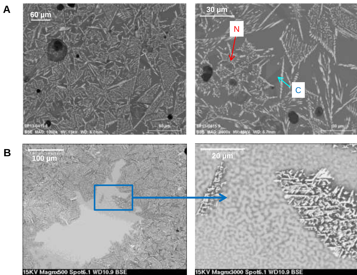
Figure 56. Clichés MEB obtenus en électrons rétrodiffusés des échantillons (A) B14Nd8 TT et (B) B14Nd10 TT. N : phase de type \text{Nd}_3\text{Si}_2\text{BO}_{10} prédominante, C : phase inconnue.
