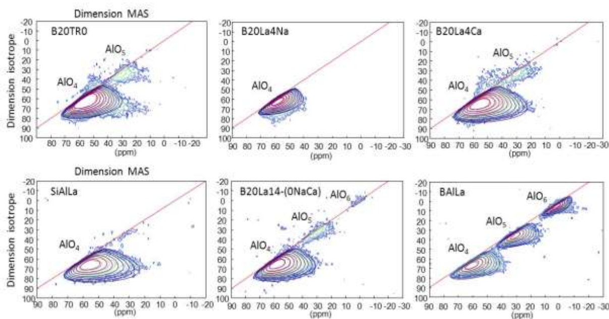
Figure 90. Spectres ^{27}\text{Al} MQMAS des verres B20TR0, B20La4Na, B20La4Ca, SiAlLa, B20La14-(0NaCa) et BAlLa ( B_0=17,6 T, \nu_r=30 kHz).
