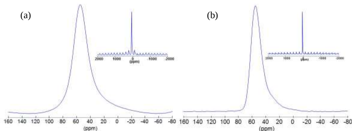
Figure 98. Spectres RMN ^{27}\text{Al} MAS des verres (a) B14Nd4 et (b) B14La4 ( B_0=17,6 T, \nu_r=30 kHz)).
