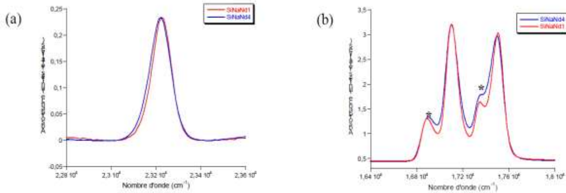
Figure 97. Spectres d'absorption optique du néodyme des verres (A) SiAlNd, BAlNd et 3B1Nd et (B) SiNaNd1 et SiNaNd4 [1] pour les transitions (a) ^4I_{9/2} \rightarrow ^2P_{1/2} et (b) ^4I_{9/2} \rightarrow ^4G_{5/2}, ^4G_{7/2} .
