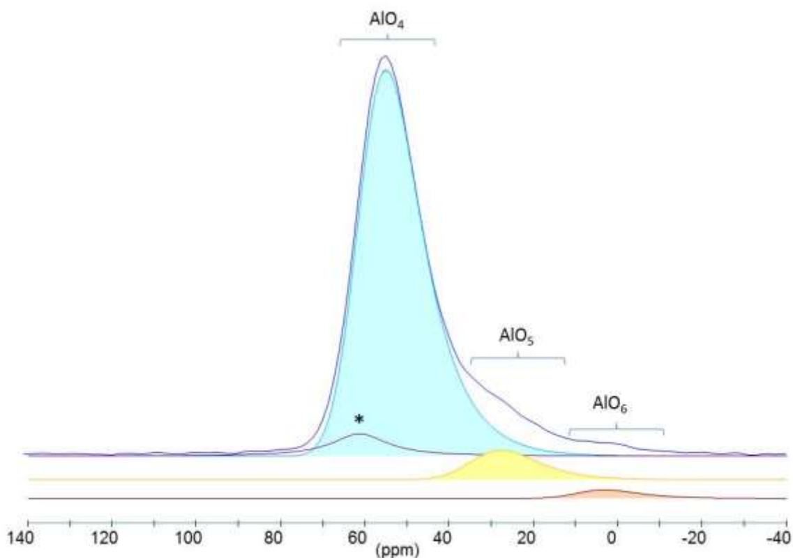
Figure 101. Simulation des différentes contributions \text{AlO}_4 , \text{AlO}_5 , et \text{AlO}_6 présentes sur le spectre ^{27}\text{Al} MAS du verre B20La4. * : bande de rotation.
