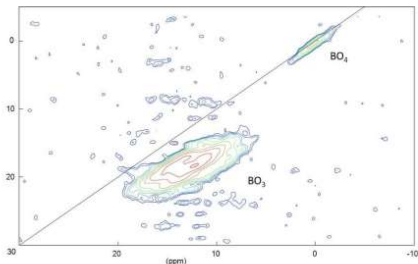
Figure 150. Spectre RMN ^{11}B MQMAS du verre B14La4 CP ( B_0=17,6 T, \nu_r=33 kHz).
