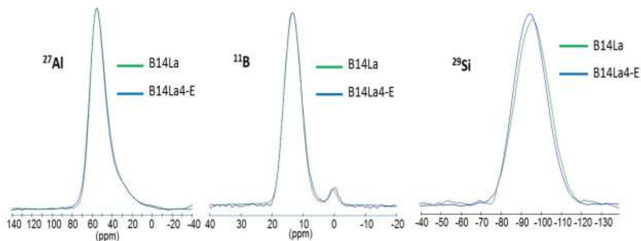
Figure 118. Comparaison des spectres RMN ^{27}\text{Al} MAS ( B_0=17,6\text{ T} , \nu_r=30\text{kHz} ), ^{11}\text{B} MAS ( B_0=19,9\text{ T} , \nu_r=22\text{kHz} ) et ^{29}\text{Si} MAS ( B_0=9,4\text{ T} , \nu_r=10\text{kHz} ) entre les verres B14La4 (en vert) et B14La4-E (en bleu).
