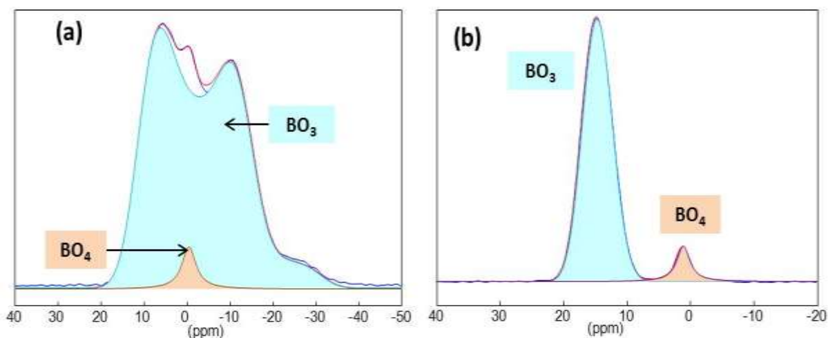
Figure 105. Spectres ^{11}\text{B} MAS expérimentaux (en bleu) et simulés (en rouge) du verre B14La4 réalisés à (a) 7 T et (b) 19,9 T. Les différentes contributions des espèces \text{BO}_3 et \text{BO}_4 sont indiquées en ne prenant en compte qu'une seule contribution pour simuler la raie des entités \text{BO}_3 .
