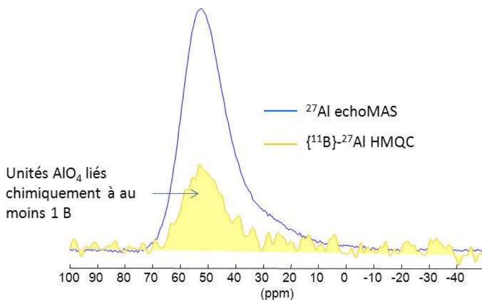
Figure 125. Spectre ^{27}\text{Al}/^{11}\text{B} HMQC (en jaune) du verre B14La4-E et comparaison avec le spectre ^{27}\text{Al} MAS correspondant (en bleu) ( B_0=17,6 T, \nu_r=33\text{kHz} ).
