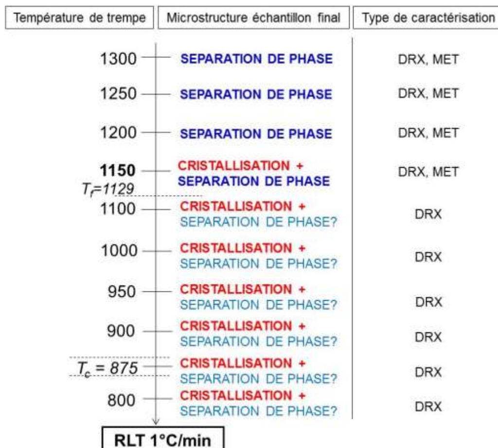
Figure 64. Schéma récapitulatif des domaines de température pour lesquels des phénomènes de séparation de phase et/ou cristallisation ont été observés (DRX, MET) au cours d'un refroidissement en température de 1^{\circ}\text{C}/\text{min} . T_f : température de fusion et T_c : température de cristallisation déterminées par DSC.
