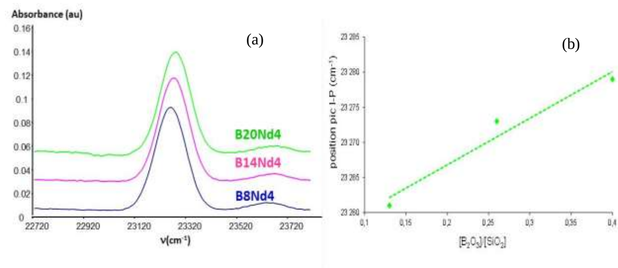
Figure 108. (a) Spectres d'absorption optique correspondants à la transition ^4I_{9/2} \rightarrow ^2P_{1/2} du néodyme ( T=10\text{K} ) des verres B8Nd4, B14Nd4 et B20Nd4 et (b) Evolution de la position en nombre d'onde de la transition ^4I_{9/2} \rightarrow ^2P_{1/2} des verres en fonction du rapport [\text{B}_2\text{O}_3]/[\text{SiO}_2] .
