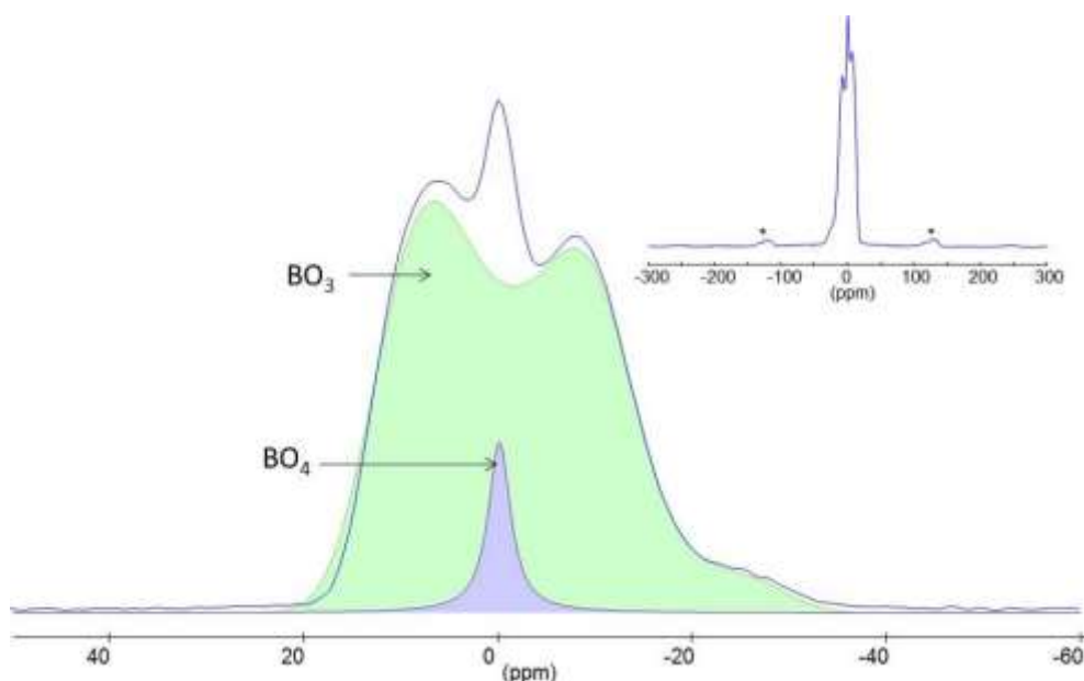
Figure 145. Spectre ^{11}\text{B} MAS ( B_0=7 T, \nu_r=12 kHz) global et représentant uniquement la transition centrale \langle +1/2 ; -1/2 \rangle . Les contributions des entités \text{BO}_3 et \text{BO}_4 sont indiquées. * : bandes de rotation dues à la transition centrale.
