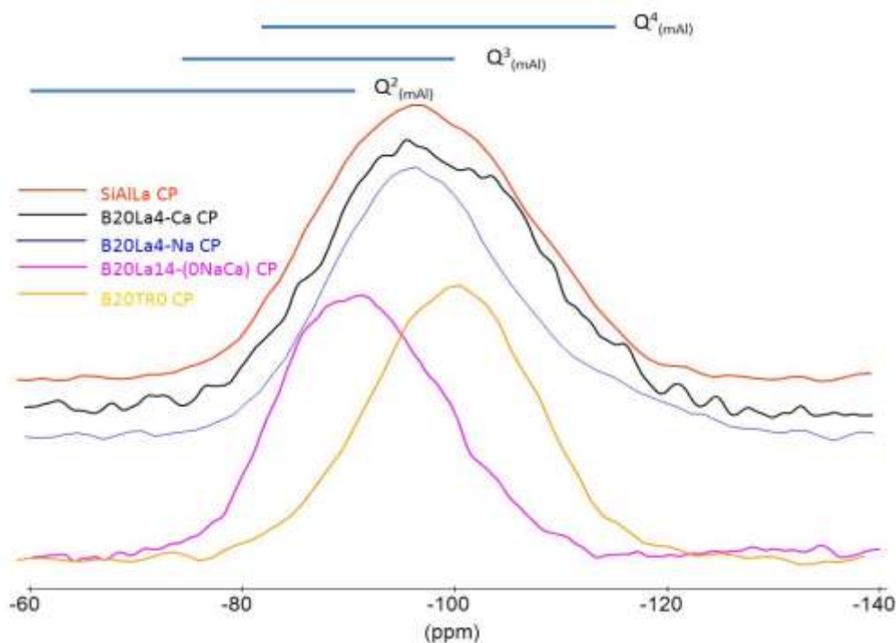
Figure 96. Spectres ^{29}\text{Si} MAS des verres SiAlLa, B20La4Ca, B20La4Na, B20La14-(0NaCa) et B20TR0, ( B_0=11,6 T, \nu_r=10 kHz). Les gammes de déplacements chimiques Q_m^n sont représentées en haut.
