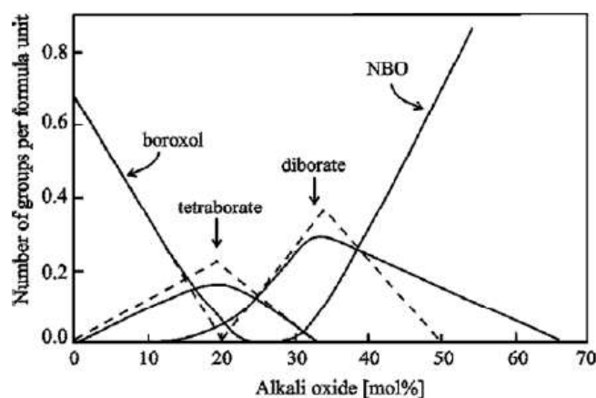
Figure 76. (a) Les différentes entités boratées présentes dans le réseau B_2O_3 - M_2O [56], (b) Evolution de leurs concentrations en fonction de la teneur en M_2O [60].
