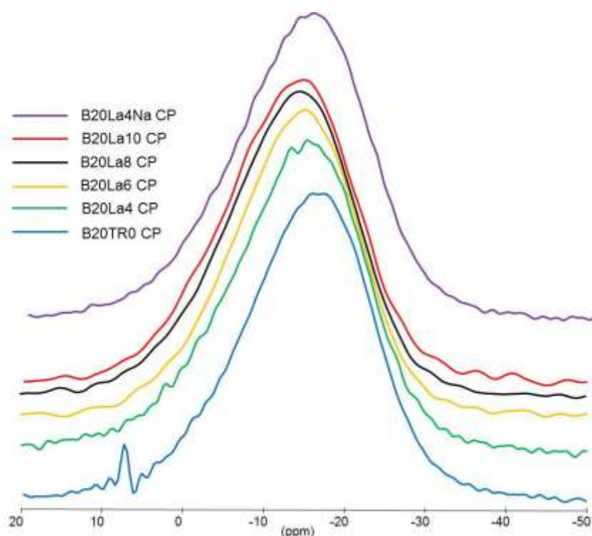
Figure 111. Spectre RMN MAS ^{23}\text{Na} ( B_0 = 17,6 \text{ T} , \nu_r = 30 \text{ kHz} ) correspondants aux verres coulés sur plaque B20TR0, B20La4, B20La6, B20La8 et B20La10. Pour comparaison, le spectre du verre B20La4Na est également présenté sur la figure.
