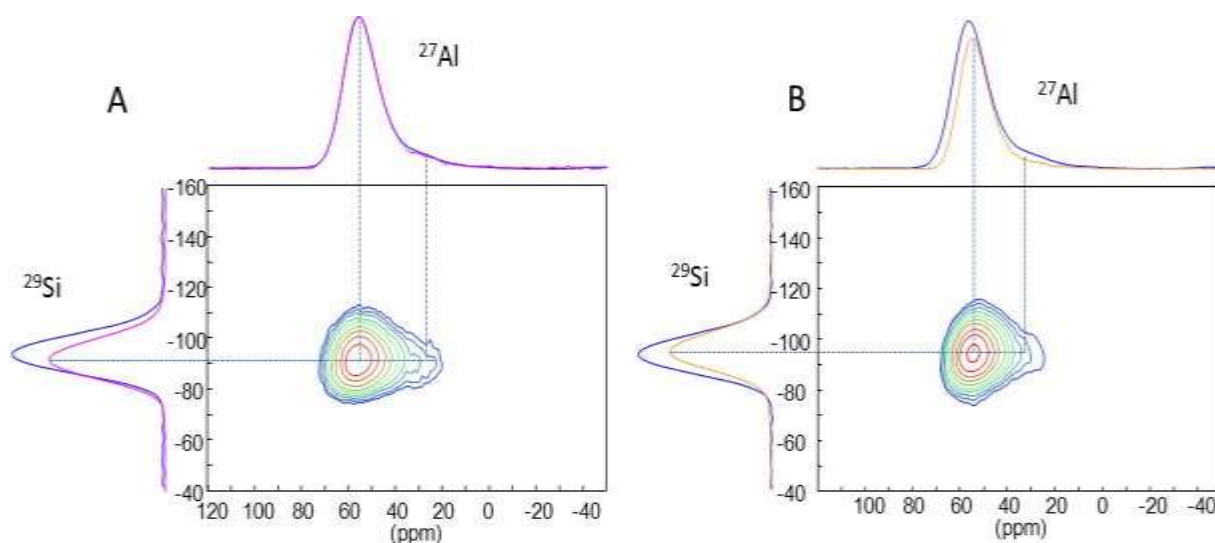
Figure 119. Spectres de corrélation 2D ^{29}\text{Si}/^{27}\text{Al} (A) DHMQC et (B) HMQC pour le verre B14La4-E. Les projections des signaux dans les dimensions directe ( ^{27}\text{Al} ) et indirecte ( ^{29}\text{Si} ) sont représentées et comparées aux spectres MAS correspondant(en bleu foncé).
