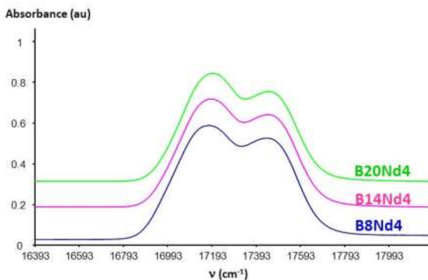
Figure 109. Spectres d'absorption optique correspondants à la transition hypersensible ^4I_{9/2} \rightarrow ^4G_{5/2}, ^4G_{7/2} du néodyme ( T=10K ) des verres B8Nd4, B14Nd4 et B20Nd4 coulés sur plaque.
