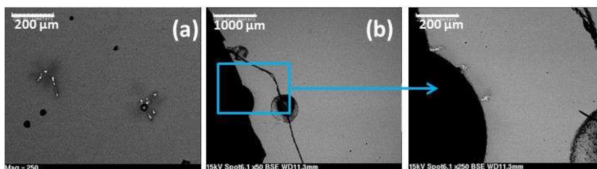
Figure 27. Clichés MEB en électrons rétrodiffusés du verre B20C-22,5 RLT ayant subi un refroidissement en température à 1^\circ\text{C}/\text{min} (a) après 5h d'affinage à 1350^\circ\text{C} (élaboration classique en four à moufle) et (b) après 5h + 4h = 9h d'affinage à 1350^\circ\text{C} .
