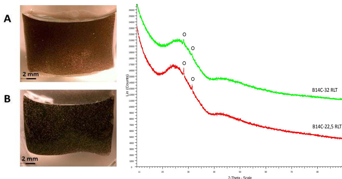
Figure 23. Observations au microscope optique (à gauche) des verres de la série B14C refroidis en température (A) B14C-22,5 RLT et (B) B14C-32 RLT et diffractogrammes de rayons X correspondants. ○ : \text{ZrO}_2 baddeleyite (JCPDS : 37-1484).
