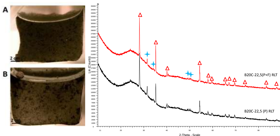
Figure 25. Observations au microscope optique (à gauche) des verres refroidis en température à 1^\circ\text{C}/\text{min} (A) B20-22,5(P) RLT et (B) B20C-22,5(P+F) RLT, et diffractogrammes des rayons X correspondants. \Delta : \text{RuO}_2 (JCPDS 40-1290) et \star : \text{ZrO}_2 Baddeleyite (JCPDS 37-1484).
