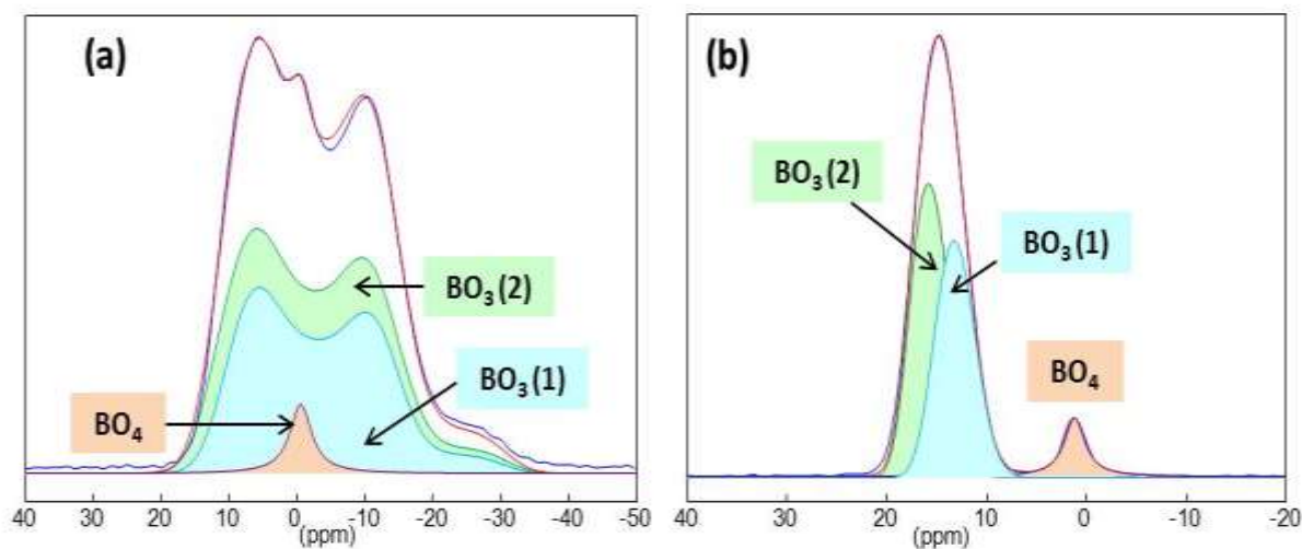
Figure 106. Spectres ^{11}\text{B} MAS expérimentaux (en bleu) et simulés (en rouge) du verre B14La4 réalisés à (a) 7 T et (b) 19,9 T. Les différentes contributions des espèces \text{BO}_3 et \text{BO}_4 sont indiquées en prenant en compte deux contributions \text{BO}_3(1) et \text{BO}_3(2) pour simuler la raie des entités \text{BO}_3 .
