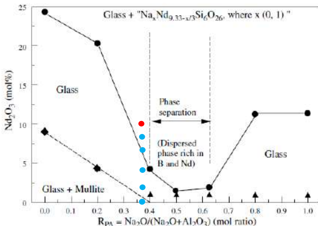
Figure 48. Représentation des verres homogènes (points bleus, contenant 0, 2,3, 4, 6 et 8 % molaires \text{Nd}_2\text{O}_3 ) ou démixés (point rouge, contenant 10 % molaires \text{Nd}_2\text{O}_3 ) reportés sur le schéma de Li et al. indiquant la limite de solubilité de l'oxyde de néodyme en fonction du caractère peralcalin ou peralumineux du verre (verre de base 60\text{SiO}_2\text{-}15\text{B}_2\text{O}_3\text{-}5\text{Al}_2\text{O}_3\text{-}20\text{Na}_2\text{O} (% molaires)) [11]. Rappelons que l'homogénéité des verres B14TR0 et B20TR0 est due à la méthode de trempe utilisée, au marteau pilon qui permet d'accélérer la vitesse de trempe et de figer au mieux un état non cristallisé.
