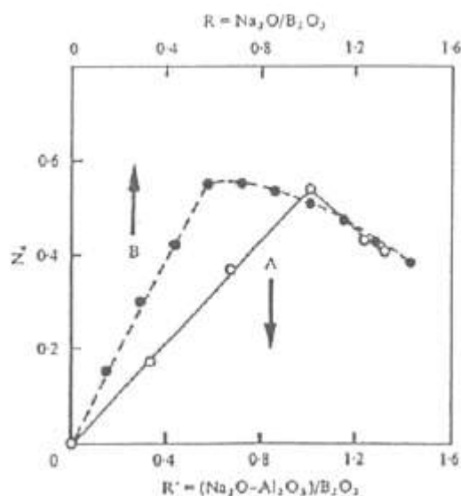
Figure 80. Variation de N_4 en fonction du rapport R' = ([\text{Na}_2\text{O}] - [\text{Al}_2\text{O}_3]) / [\text{B}_2\text{O}_3] (courbe A) ou du rapport R = [\text{Na}_2\text{O}] / [\text{B}_2\text{O}_3] (courbe B) des verres de compositions 30\text{SiO}_2 - 30\text{B}_2\text{O}_3 - [0-25]\text{Al}_2\text{O}_3 - [40-15]\text{Na}_2\text{O} [83].
