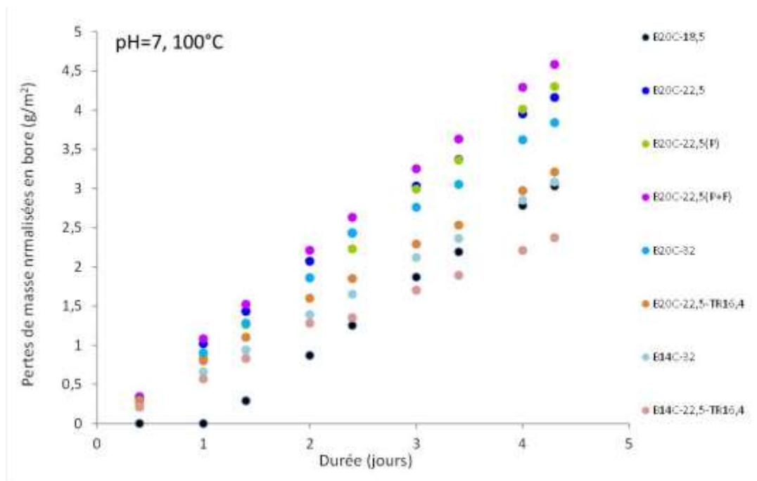
Figure 33. Evolution des pertes de masse normalisées en bore (g/m 2 ) pour les différentes compositions de verres étudiées lors de la mesure des vitesses initiales de dissolution.
