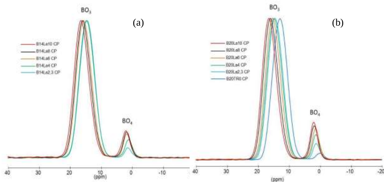
Figure 112. Spectres RMN MAS ^{11}\text{B} ( B_0=18,8 T, \nu_r=20 kHz) des séries de verres (a) B14Lax avec x variant de 2,3 à 10 % molaires \text{La}_2\text{O}_3 et (b) B20Lax avec x variant de 0 à 10 % molaires \text{La}_2\text{O}_3 .
