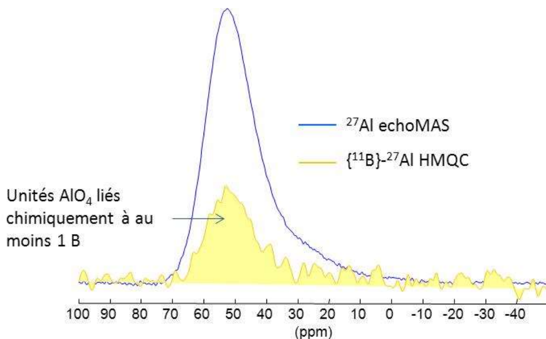
Figure 153. Spectre ^{27}\text{Al}/^{11}\text{B} HMQC (en jaune) du verre B14La4-E et comparaison avec le spectre ^{27}\text{Al} MAS correspondant (en bleu).
