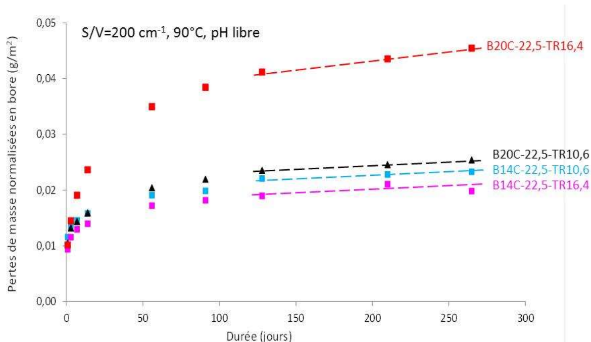
Figure 34. Evolution des pertes de masse normalisées du bore pour les verres des séries B14C et B20C à teneur en PFA fixe (22,5% massiques) et teneur en terres rares variables (10,6 ou 16,4 % massiques).
