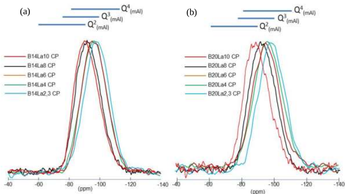
Figure 115. Spectres RMN ^{29}\text{Si} MAS ( B_0=11,6 T, \nu_r=10 kHz) des séries de verres des séries (a) B14Lax et (b) B20Lax avec x variant de 2,3 à 10 % molaires \text{La}_2\text{O}_3 . Les gammes de déplacements chimiques correspondant aux unités Q^n_{m(\text{Al})} ( 2 < n < 4 ) sont représentées en haut des spectres.
