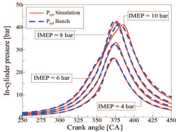
Figure 4-9a. \phi=1 , 15% O 2
