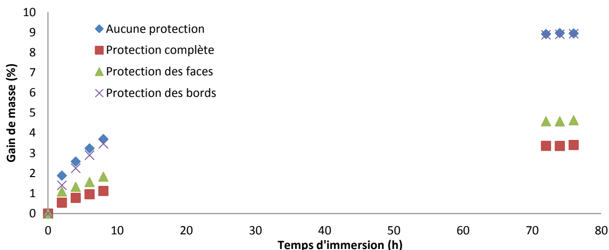
Figure 5-14: Comparaison des courbes d'absorption entre des éprouvettes non protégées et des éprouvettes protégées.
