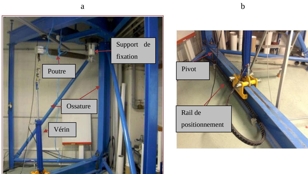
Figure 4-1 : Banc d'essai MAQUET
