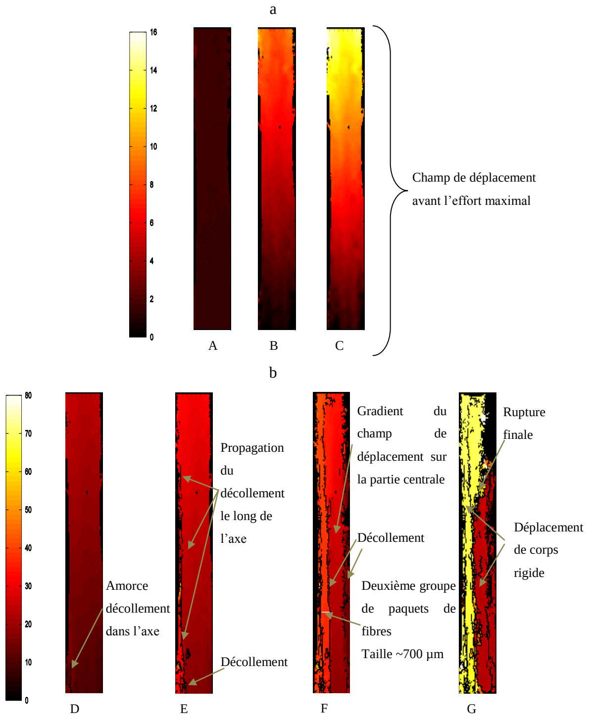
Figure 3-22: Champ de déplacement a) avant l'effort maximal, b) après l'effort maximal.
