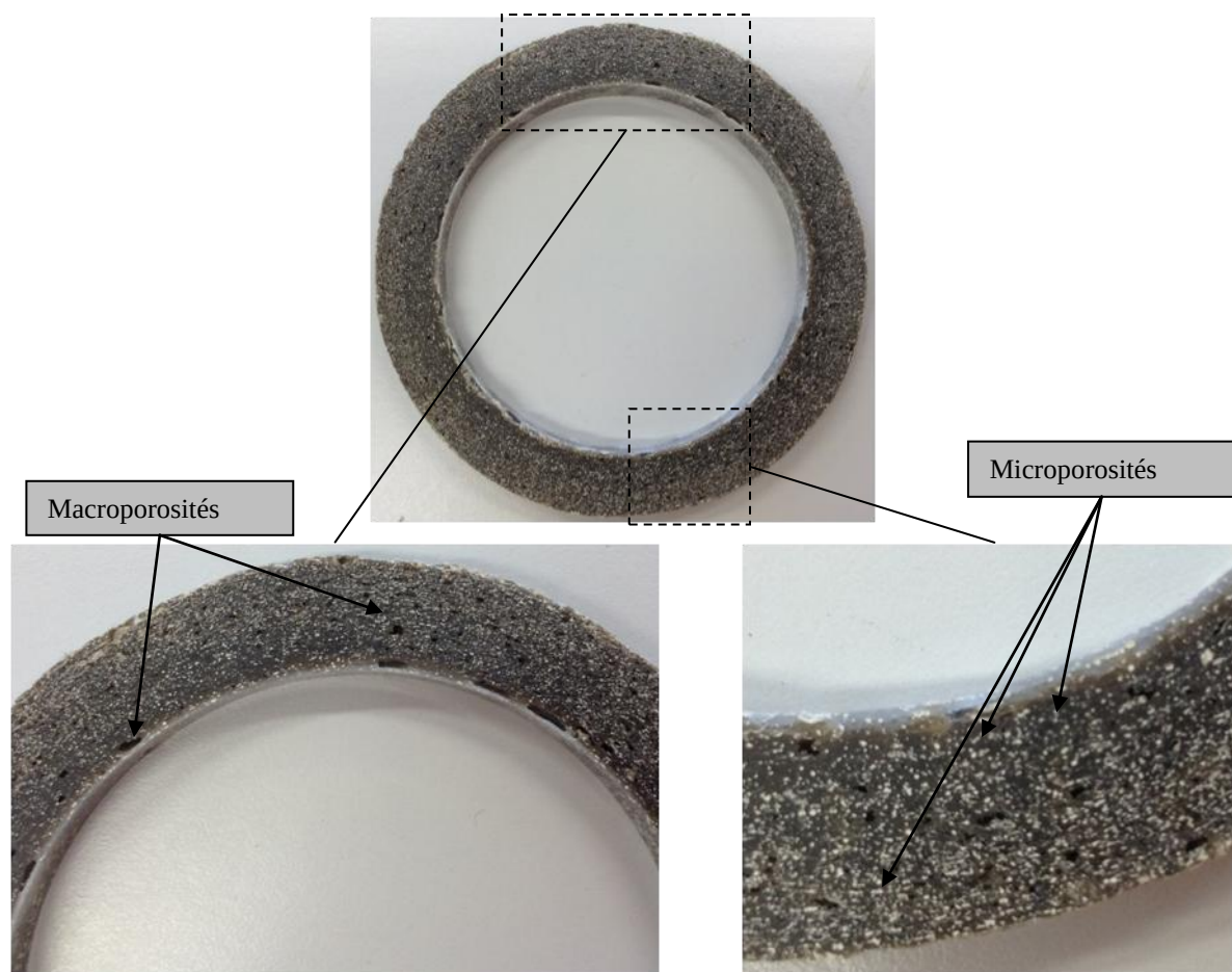
Figure 4-30 : Section transversale du prototype 3.
