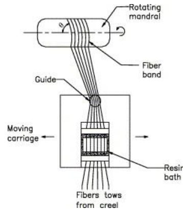
Figure 2-15: Schéma des étapes de l'enroulement [112]
