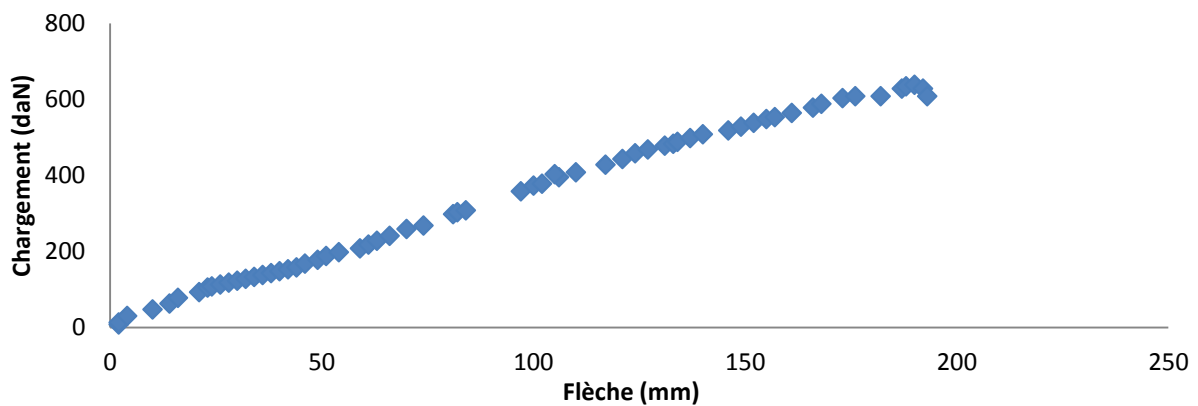
Figure 4-18: Essai de flexion jusqu'à la rupture, prototype 2.
