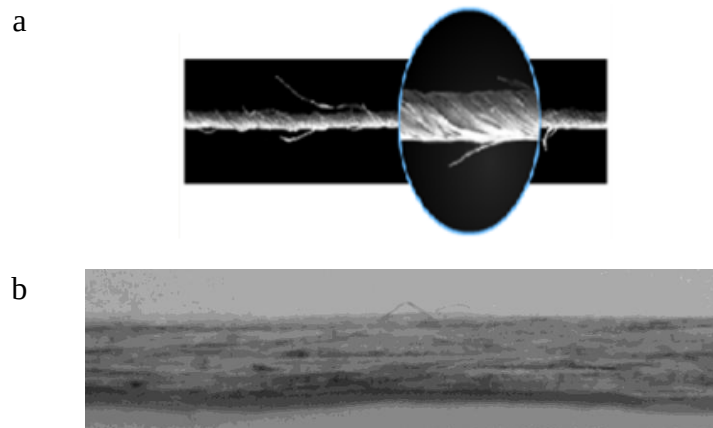
Figure 3-3: Architectures des mèches de lin, a) twistée, b) non-twistée.
