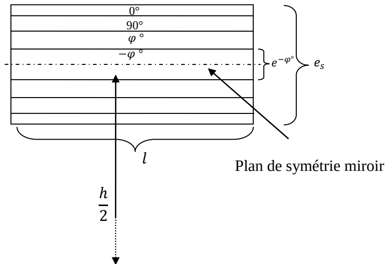
Figure 2-9: Représentation de la stratification d'une semelle
