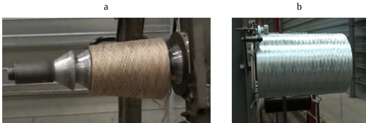
Figure 4-26: Bobines sur cantre pour l'enroulement filamentaire, a) bobines coniques, b) bobines cylindriques
