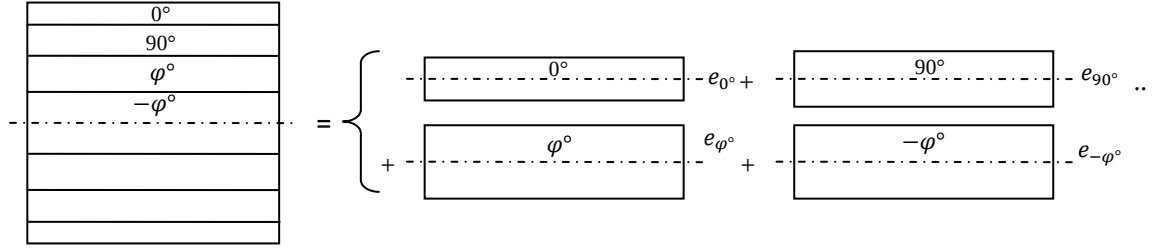
Figure 2-10: Approximation de la stratification pour le pré-dimensionnement en flexion.
