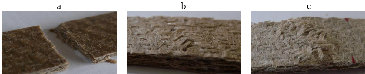
Figure 5-11: Zones de rupture des éprouvettes de traction de Lin/PLA-B a) non-vieilli, b) 2 semaines-humide, c) 2 semaines-sec.
