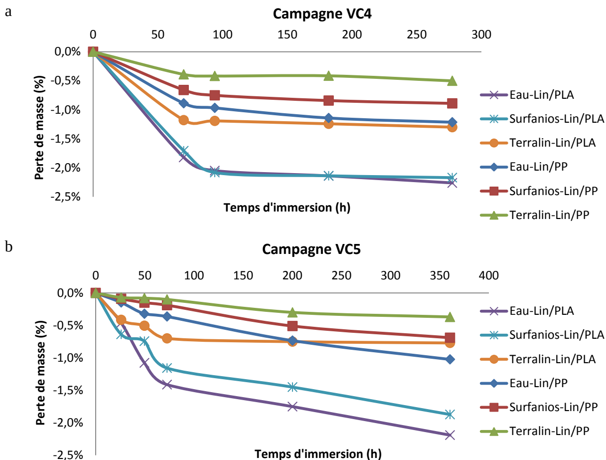
Figure 5-9: Courbes de pertes de masse, a) campagne VC4, b) campagne VC5.
