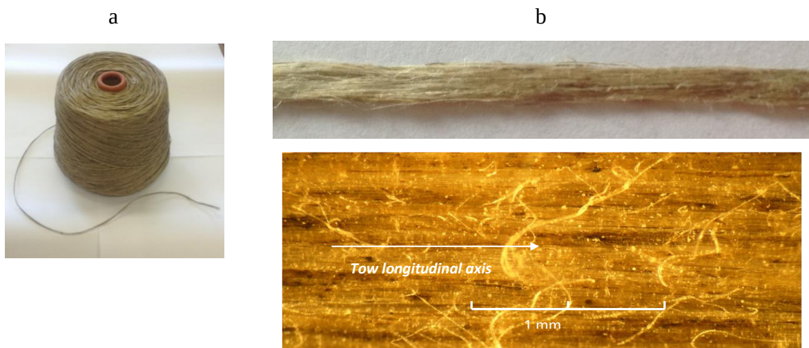
Figure 3-5: Matériau, a) bobines, b) Vues de dessus de la mèche BR.
