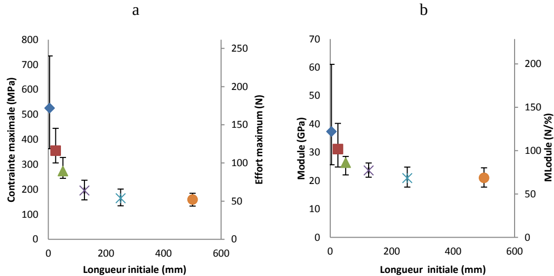
Figure 3-11: Effet de la longueur sur la contrainte max. et sur le module longitudinal.
