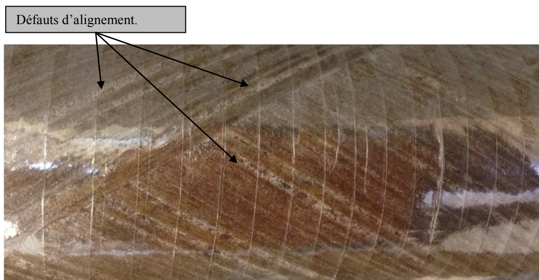
Figure 4-28 : Défauts d'alignement des mèches.
