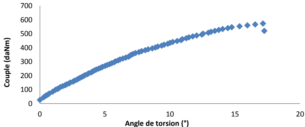
Figure 4-23: Essai de torsion jusqu'à la rupture, prototype 2.
