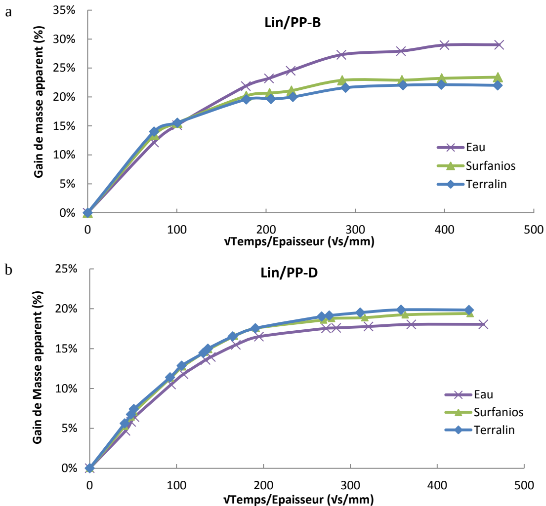
Figure 5-8: Courbes d'absorption pour le lin/PP a) Campagne VC4, b) Campagne VC5.
