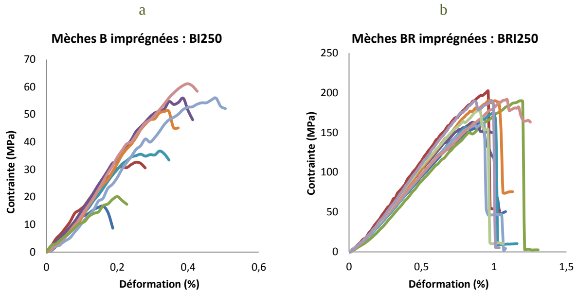
Figure 3-18: Courbes de traction sur mèches imprégnées-humides, a) mèches B, b) mèches BR.
