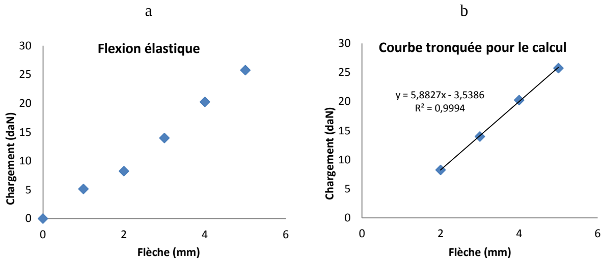
Figure 4-17: Courbe de l'essai de flexion, prototype 2.
