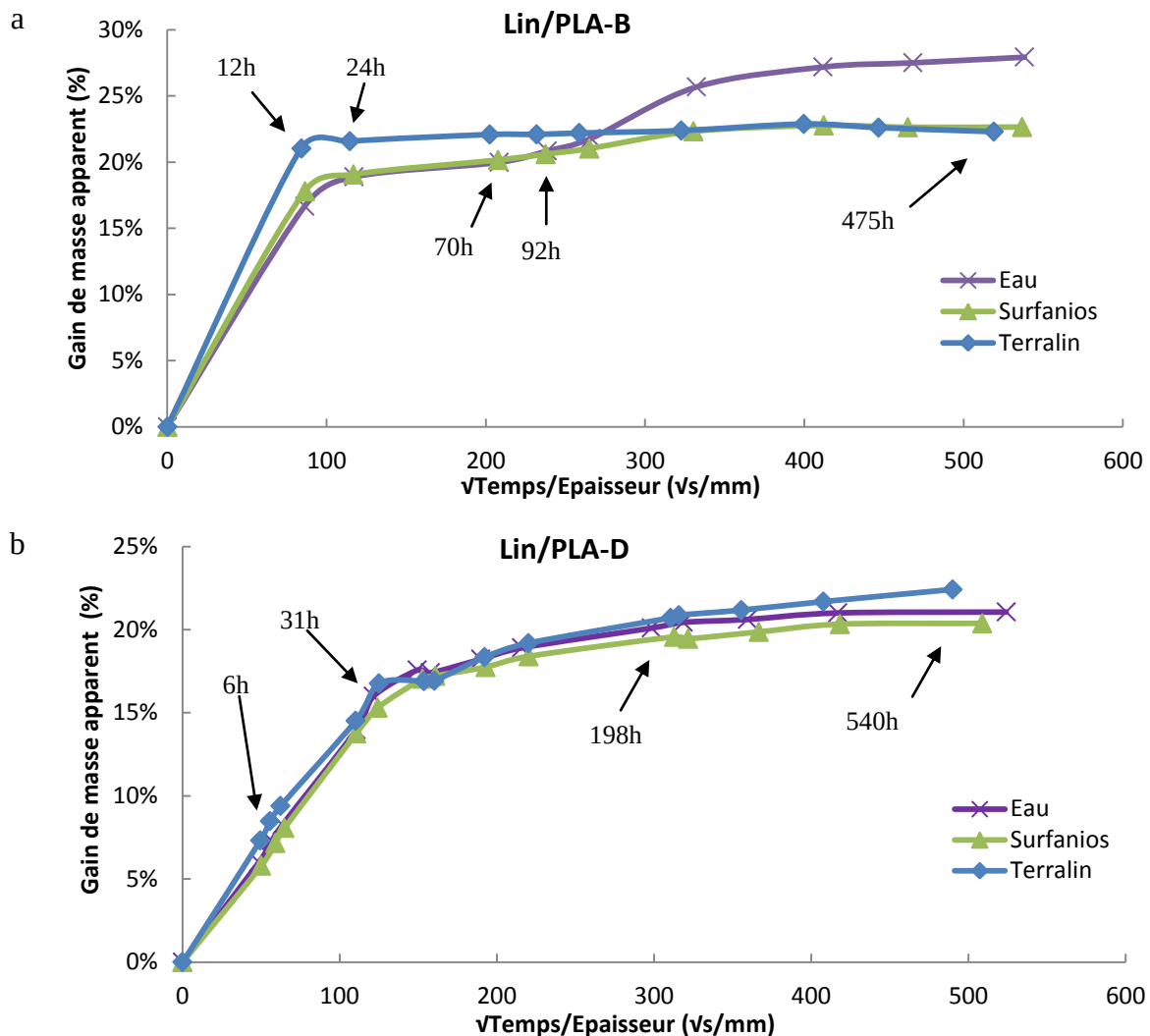
Figure 5-7: Courbes d'absorption pour le Lin/PLA a) Campagne VC4, b) Campagne VC5.
