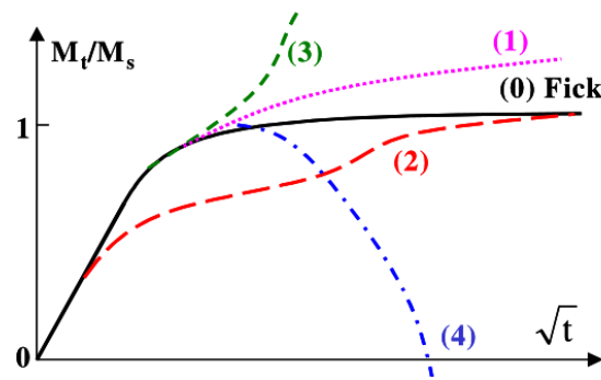
Figure 5-2: Courbes d'absorption [163].
