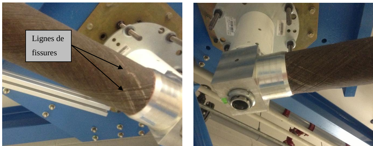
Figure 4-24: Localisation de la rupture en torsion
