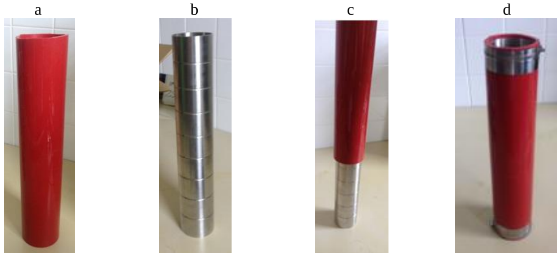
Figure 2-17: Assemblage de la membrane sur mandrin
