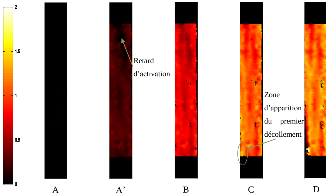
Figure 3-24: Champs de déformation longitudinale \epsilon_{xx} .
