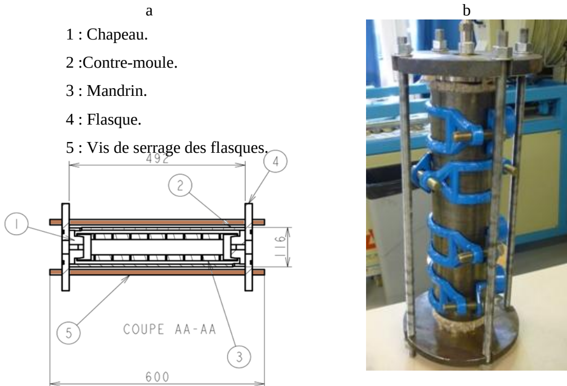
Figure 2-16: Ensemble du montage de moulage à la vessie a) vue en coupe b) montage réel
