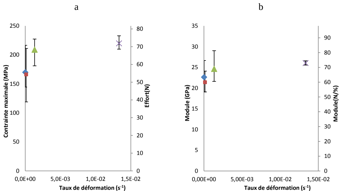
Figure 3-15: Effet du taux de déformation pour une longueur d'éprouvette de 250 mm a) contrainte maximale, b) module.
