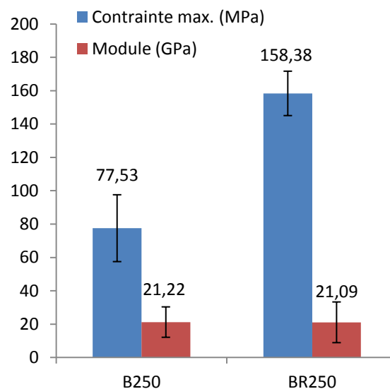
Figure 3-17: Propriétés mécaniques des mèches sèches.
