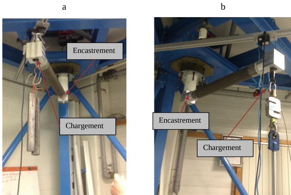
Figure 4-4 : Montage et chargement en flexion.
