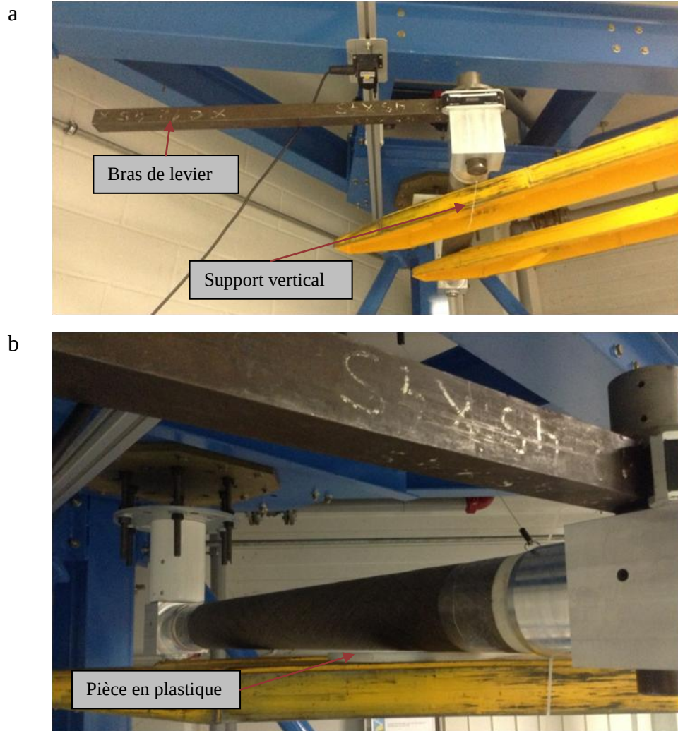
Figure 4-5 : Montage en torsion.
