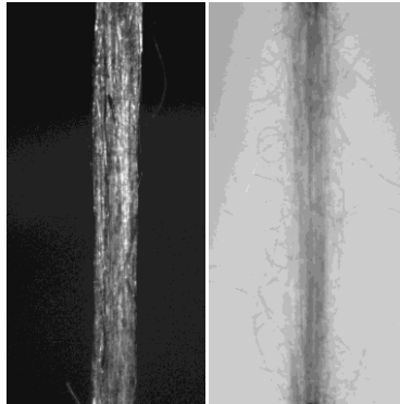
Figure 3-23: Comparaison entre une mèche de lin (gauche) et une mèche de verre (droite) après rupture.
