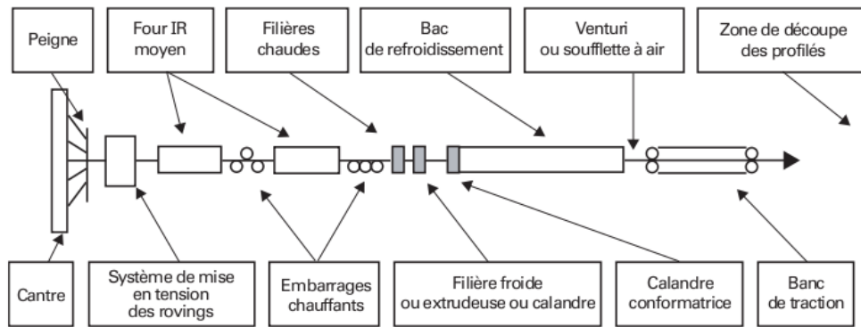
Figure 2-13: Schéma de la pultrusion des thermoplastiques [107].
