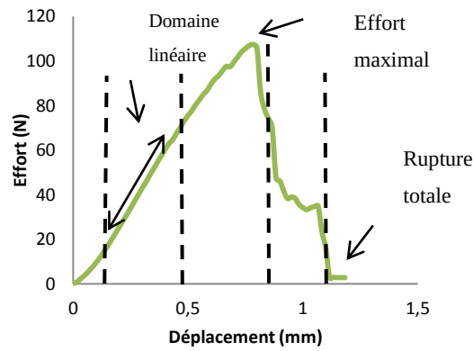
Figure 3-10: Comportement en traction typique d'une mèche de lin.
