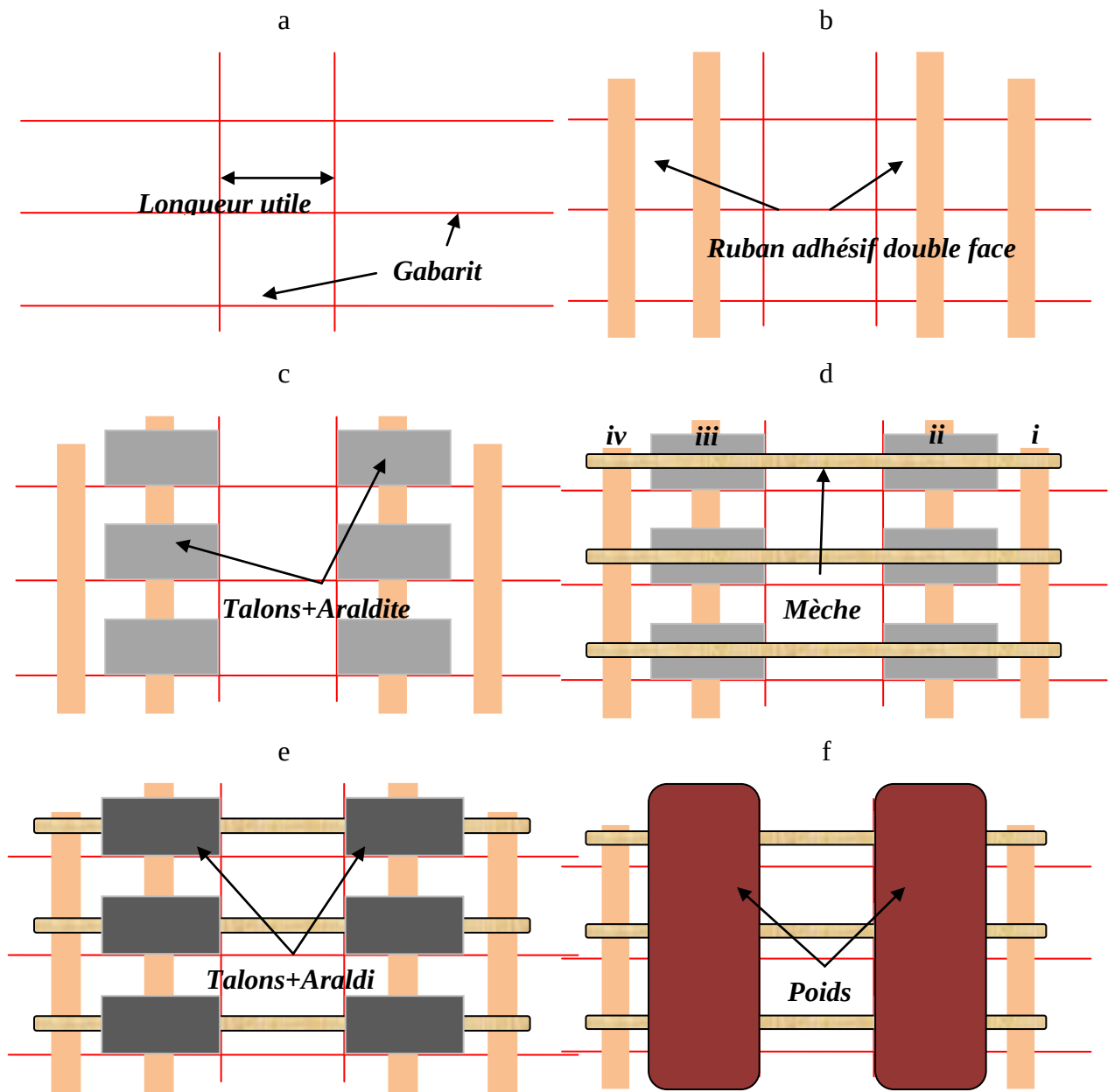
Figure 3-7: Etapes de préparation des éprouvettes de traction.
