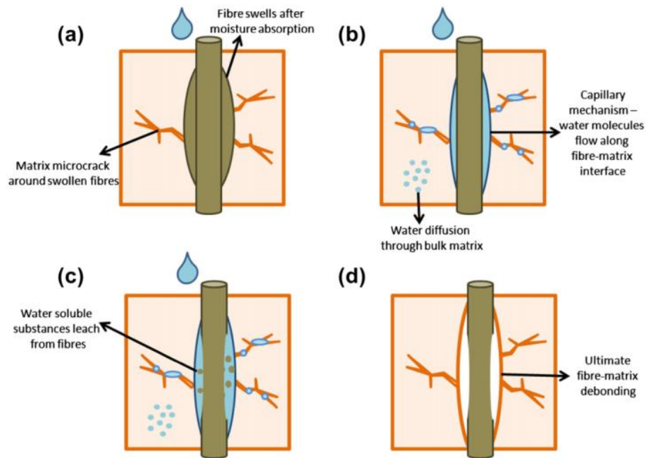
Figure 5-4: Effet de l'absorption sur l'interface fibre matrice [14].
