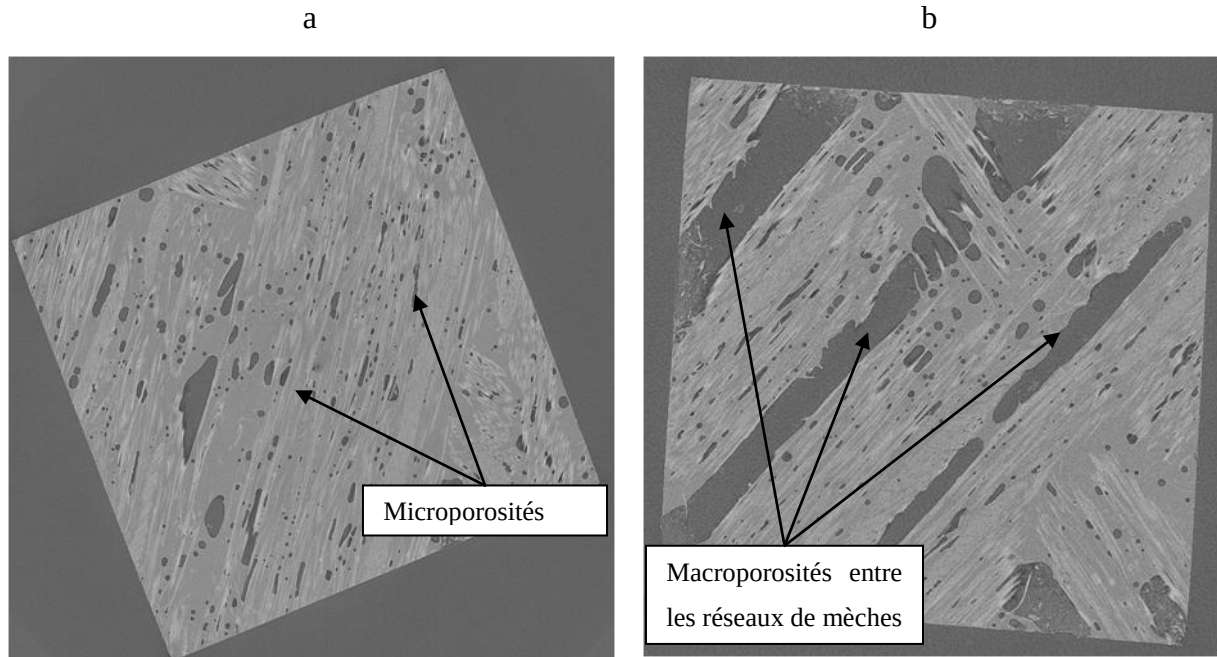
Figure 4-16: Images de tomographie d'échantillons.
