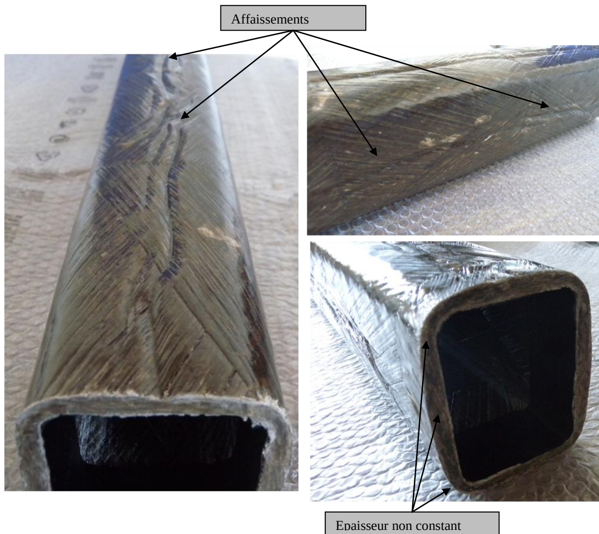
Figure 4-8: Vues en perspective du prototype 1
