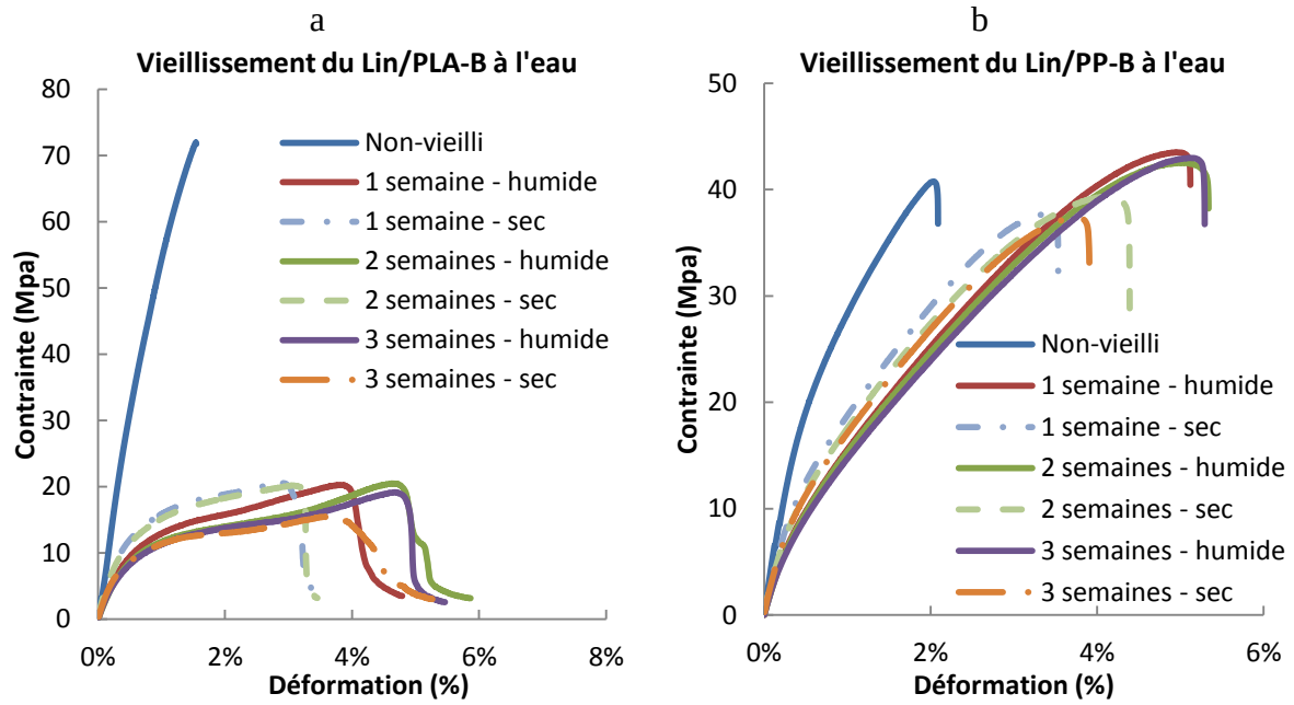
Figure 5-10: Evolution du comportement mécaniques des composites de la campagne VC4 pour une immersion à l'eau, a) Lin/PLA-B, b) Lin/PP-B.
