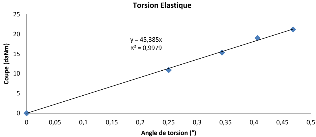
Figure 4-22: Courbe de l'essai de torsion, prototype 2.
