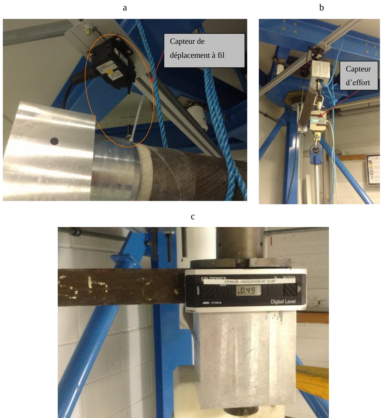
Figure 4-7 : Moyens d'acquisition des déplacements et efforts
