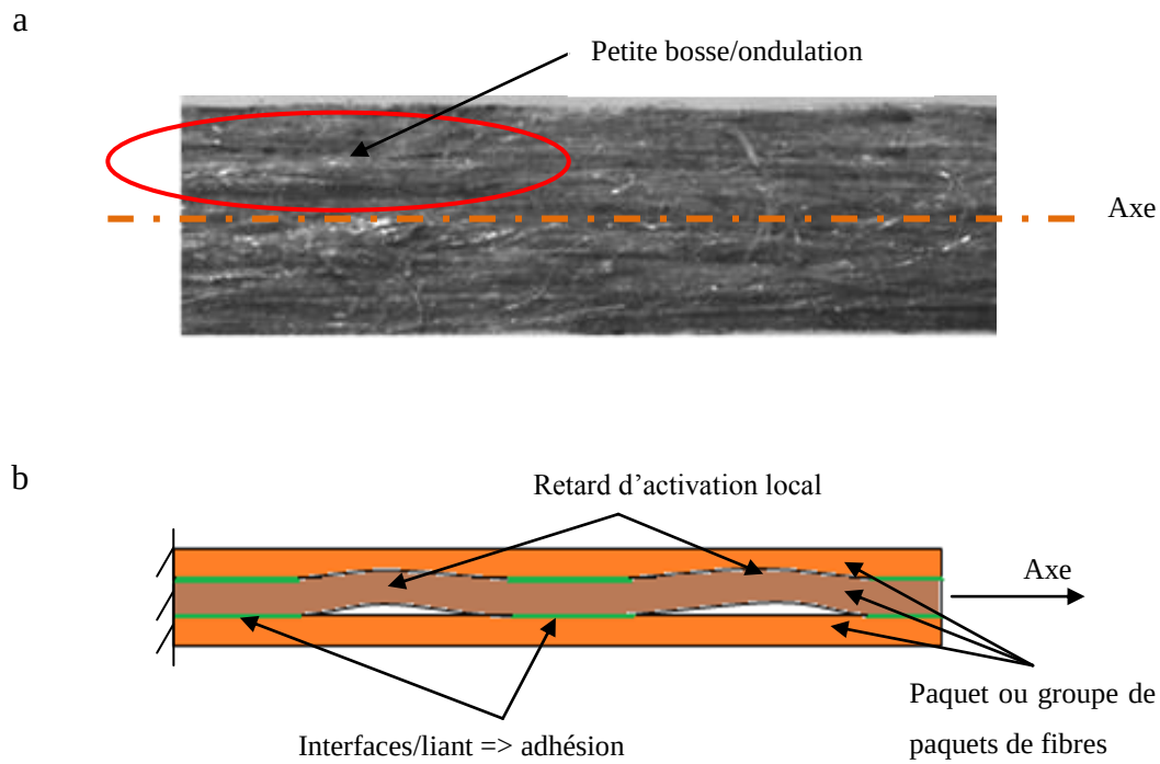
Figure 3-25: Irrégularités le long de la mèche.
