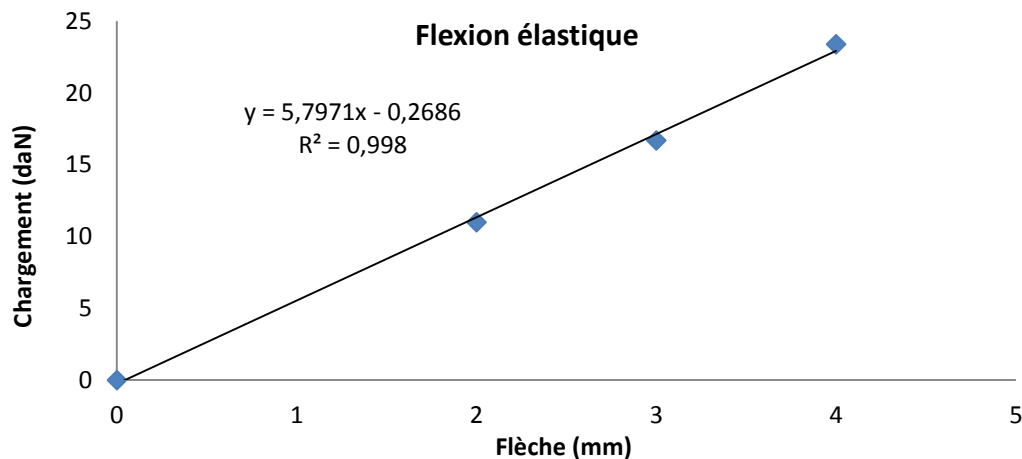
Figure 4-10: Courbe de l'essai de flexion, prototype 1
