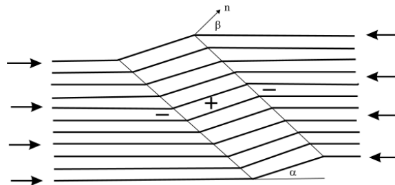
Figure 4-21: Formation d'un « kink band » dans une strate en compression [143].
