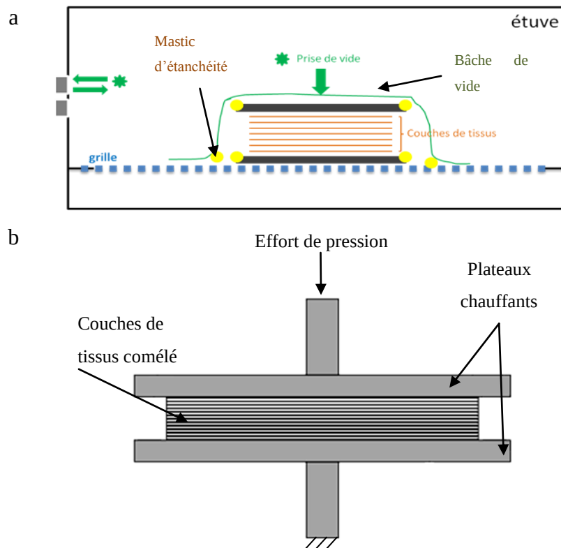
Figure 5-5: Consolidation des plaques bio-composites a) moulage sous vide en étuve, b) moulage à la presse à plateaux chauffants (schéma adapté de [171]).
