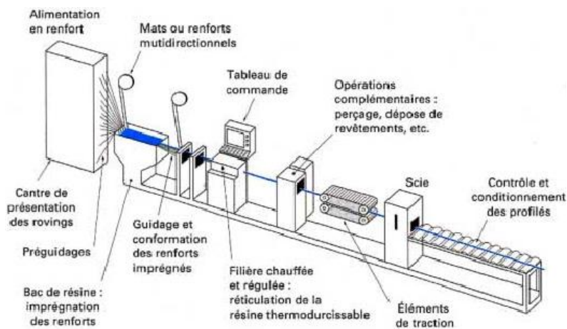
Figure 2-14: Schéma de la pultrusion des thermodurcissables [109].
