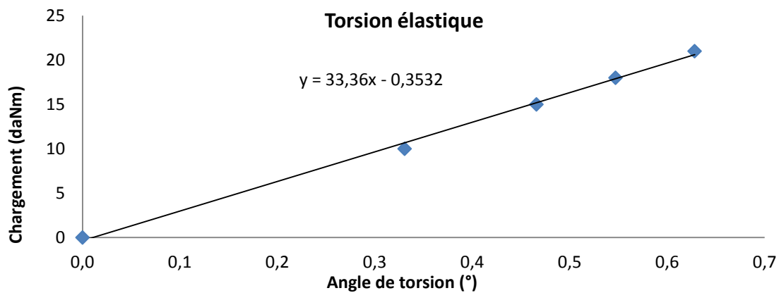
Figure 4-11: Courbe de l'essai de torsion, prototype 1
