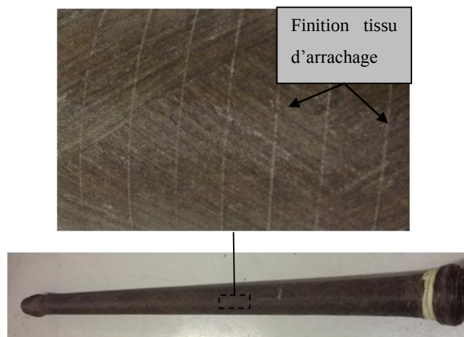
Figure 4-13: Réception du prototype 2.
