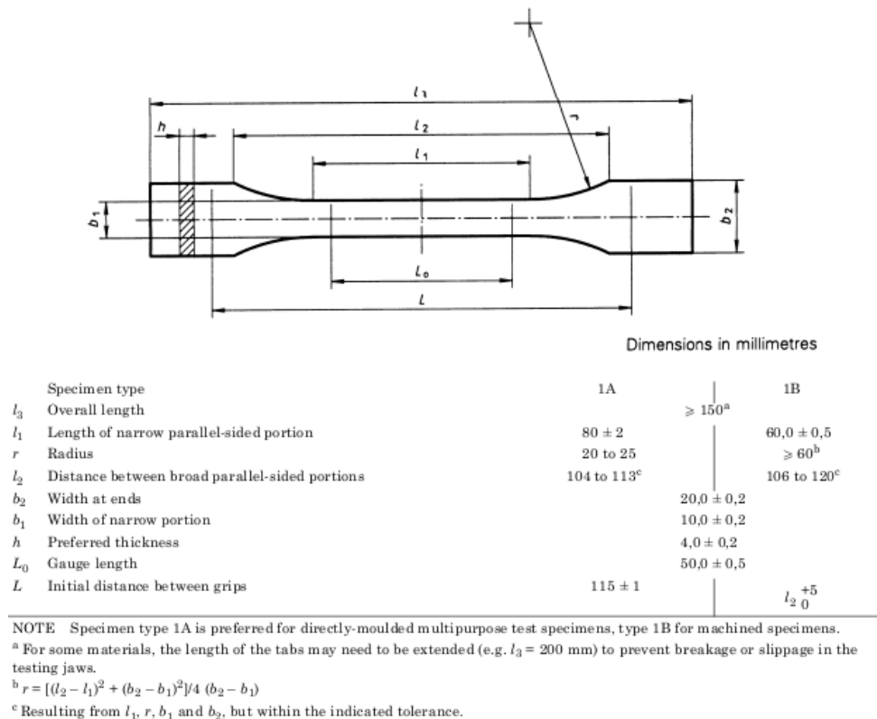
Figure 5-6: Eprouvette de traction selon l'ISO 527 [172].
