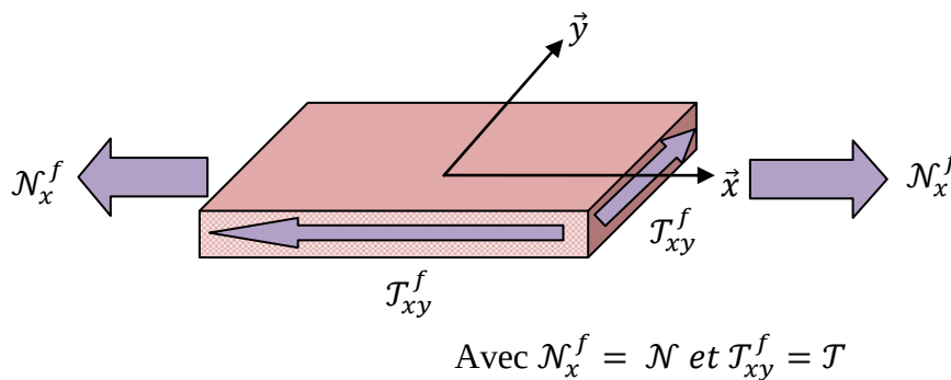
Figure 2-7: Stratifié sous sollicitation
