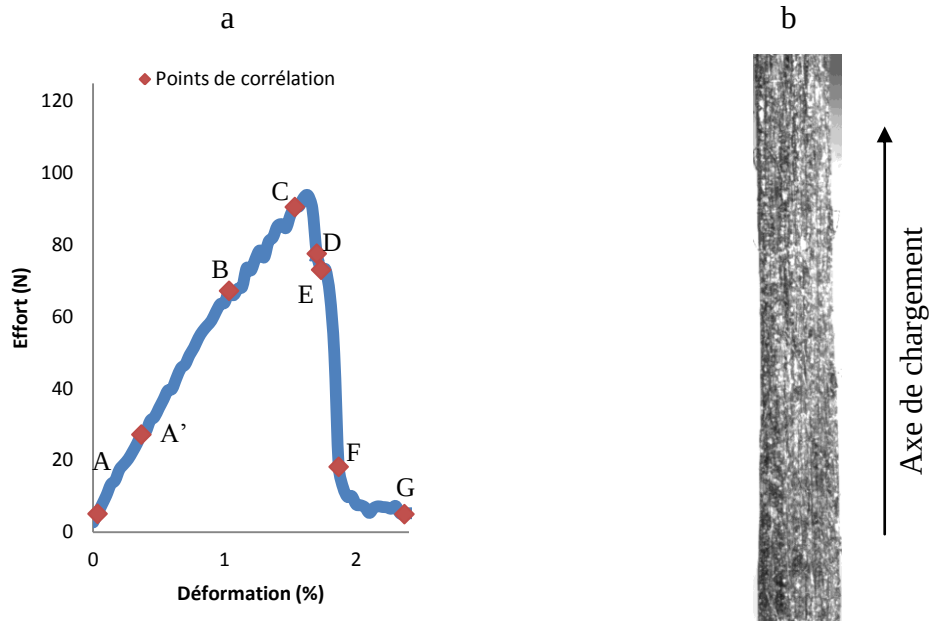
Figure 3-21: a) Courbe de traction et les états correspondant à la corrélation, b) l'éprouvette et son mouchetis.
