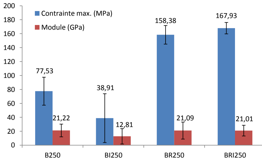
Figure 3-19 : Comparaison des propriétés mécaniques avant et après imprégnation.
