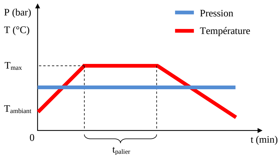
Figure 4-33: Cycle de température et pression.
