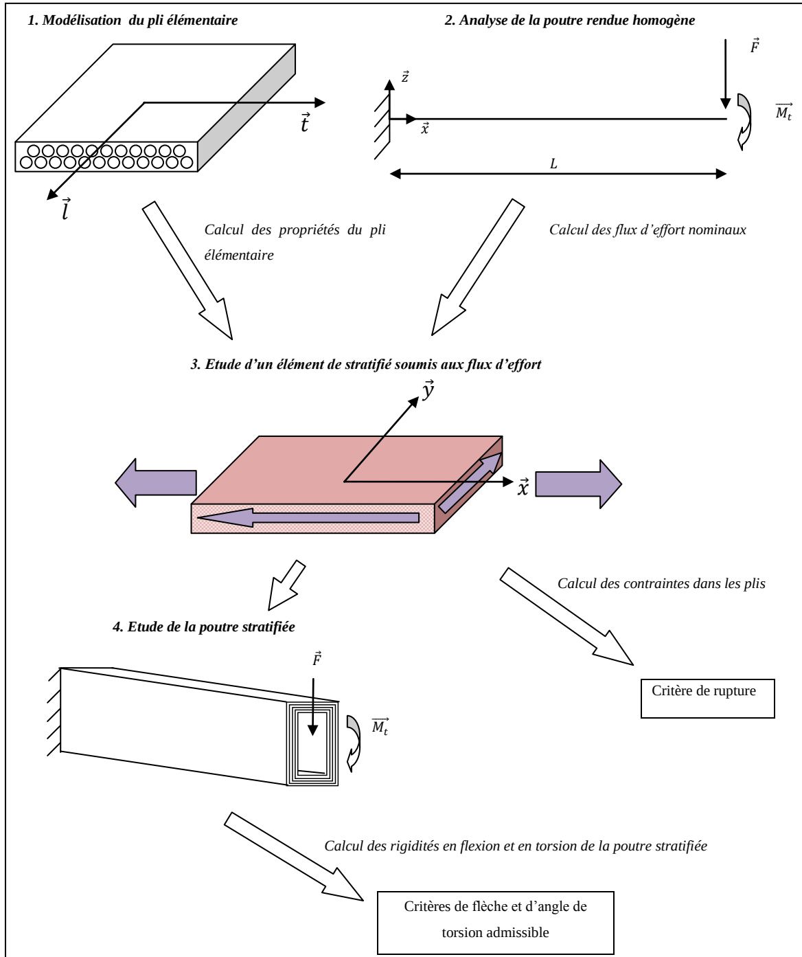
Figure 2-5: Illustration de la démarche pour l'expression des critères de dimensionnement.
