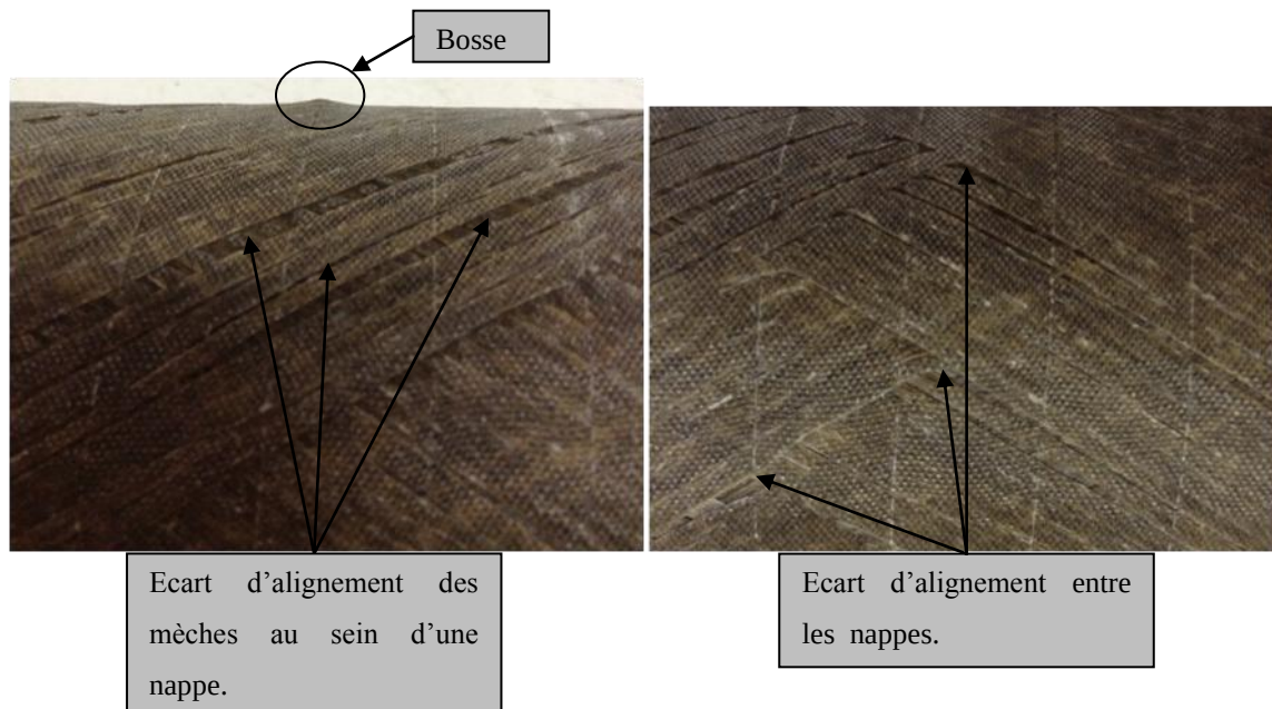
Figure 4-14: Défauts en surface.
