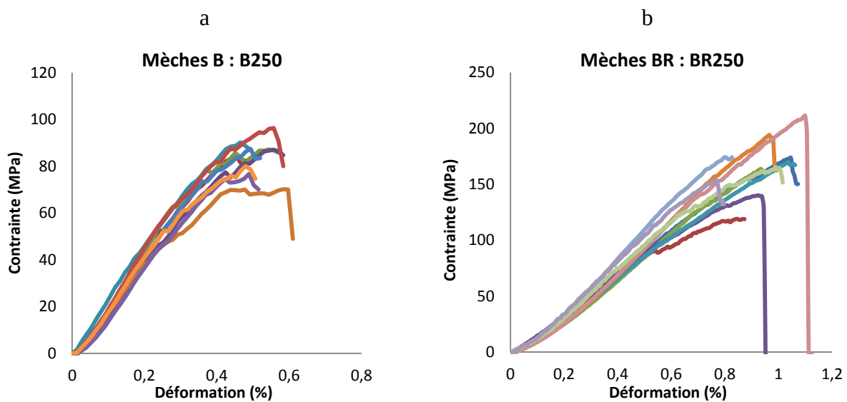
Figure 3-16: Courbes de traction sur mèches sèches, a) mèches B, b) mèches BR.
