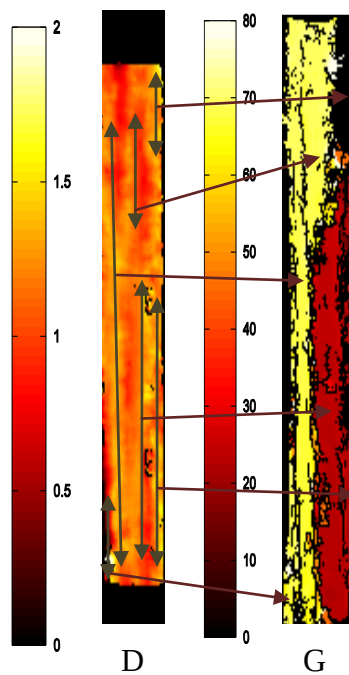
Figure 3-26: Correspondance entre l'état d'activation des groupes de paquets avec l'état de rupture.
