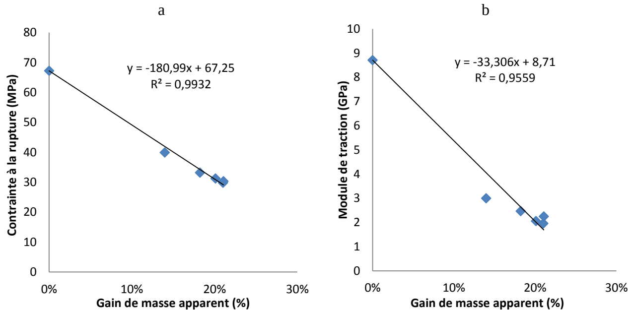
Figure 5-15: Evolution des propriétés mécaniques en fonction du gain de masse, Lin/PLA-D.
