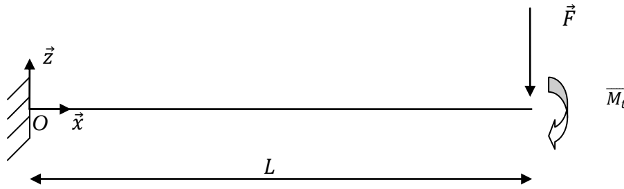
Figure 2-2: Cas de charge de la pièce
