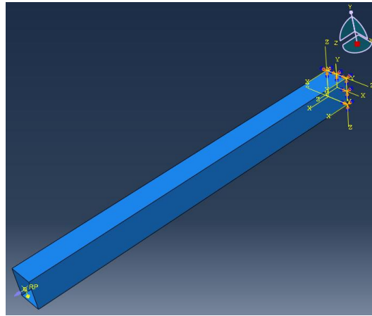
Figure 2-12: Vues du modèle numérique (Abaqus®)
