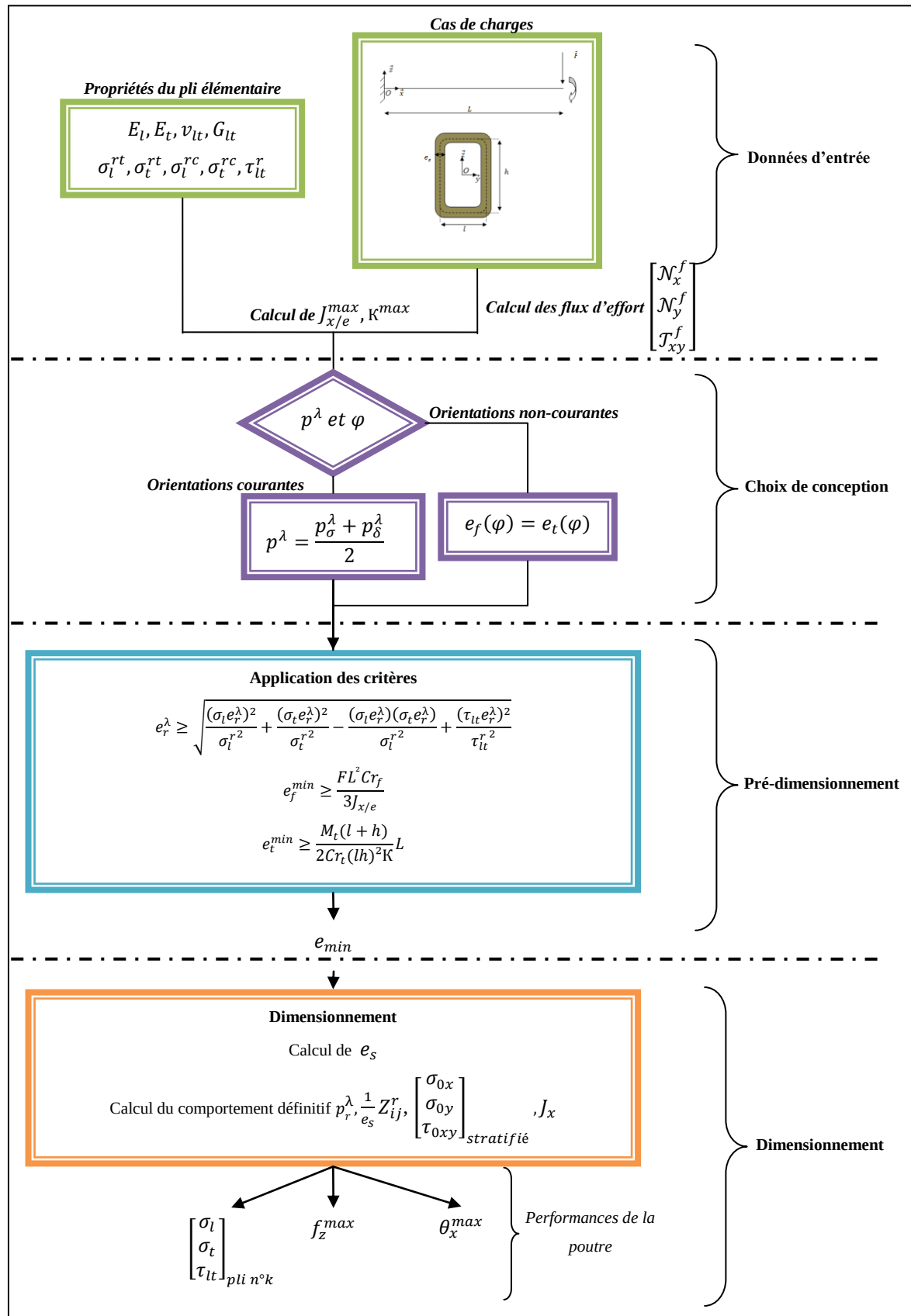
Figure 2-11: Chaine de calculs analytiques
