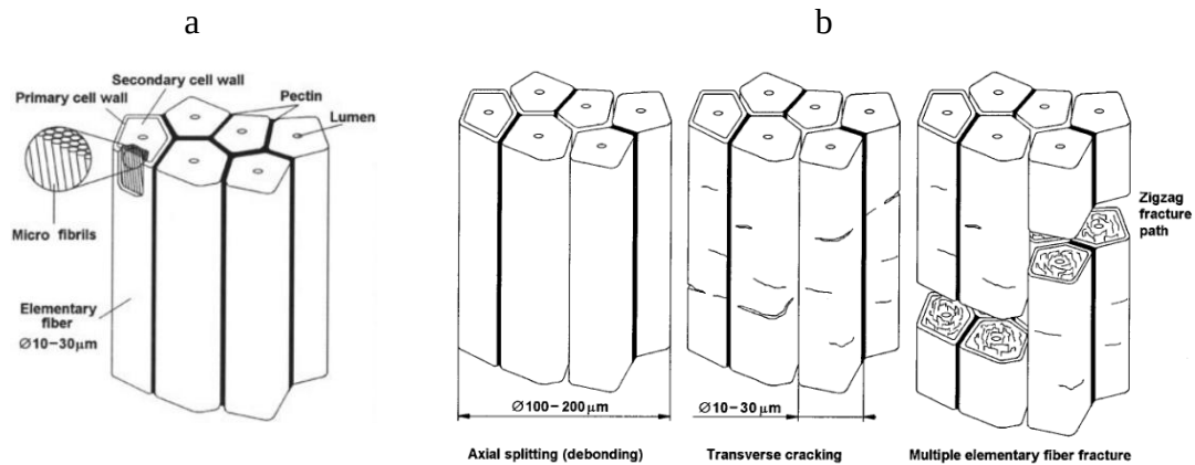
Figure 3-2: a) Paquet de fibres b) Modes de rupture des paquets de fibres.
