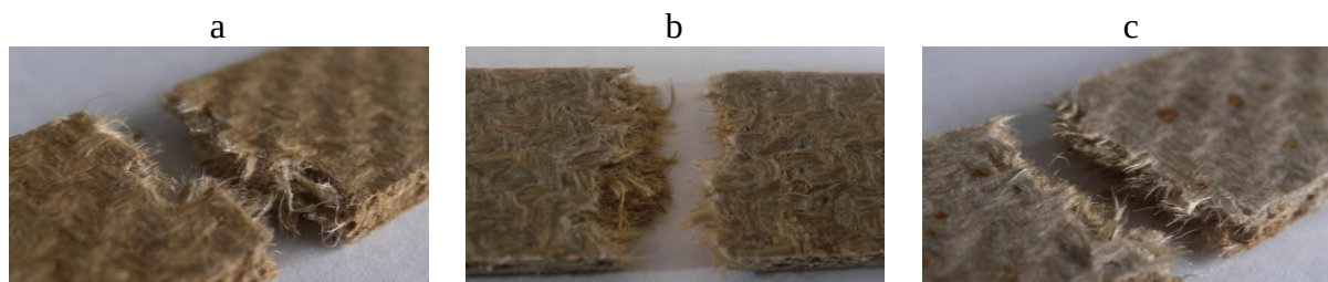
Figure 5-12: Zones de rupture des éprouvettes de traction de Lin/PP-B a) non-vieilli, b) 2 semaines-humide, c) 2 semaines-sec.
