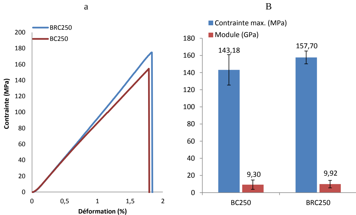
Figure 3-20: Mèches imprégnées-durcies a) comportement, b) propriétés mécaniques.
