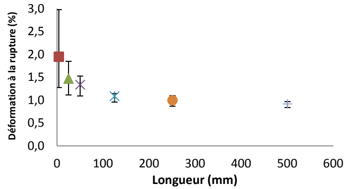
Figure 3-13: Evolution de la déformation à la rupture en fonction de la longueur.
