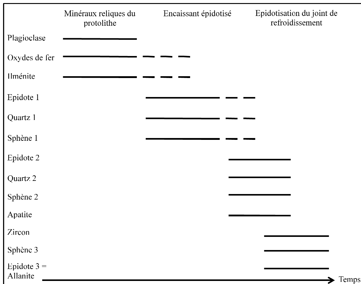
Figure 2.25 : Séquence paragénétique des épidotes de joint de refroidissement.
