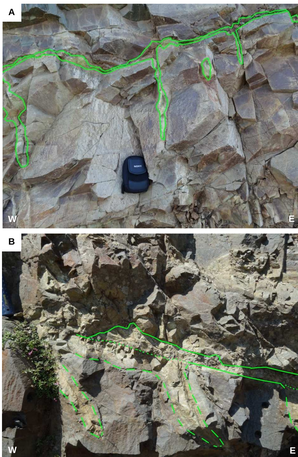
Figure 2.22 : Epidote entre les dykes et dans les joints de refroidissement. (A) Affleurement localisé sur la route d'Oikos-Gerakies. (B) Affleurement localisé juste au nord du village de Lemithou.
