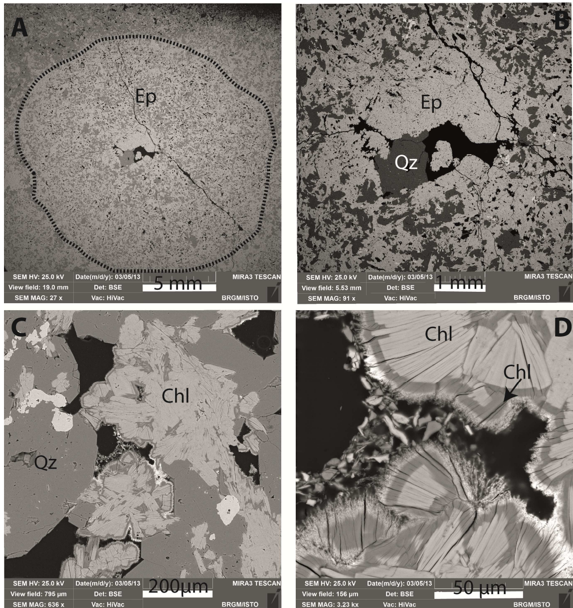
Figure 2.34 : (A) Image MEB d'une sphérulite d'épidote et quartz (éch. 65). (B) Zoom sur le cœur de cette sphérulite. (C&D) Chlorite zonée dans la porosité (Mokni-Leconte, 2013). Abréviations : Chl = Chlorite ; Ep = Epidote ; Qz = Quartz.
