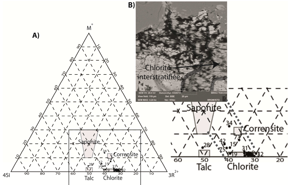
Figure 2.39 : A) Diagramme ternaire M^+-4Si-3R^{2+} présentant la composition des argiles ( M^+=2Ca+Na+K ; 4Si=Si/4 ; 3R^{2+}=(Fe^{2+}+Mg+Mn)/3 ) (figure modifiée d'après Meunier et al., 2012) et B) Image MEB de chlorites interstratifiées dans l'échantillon de métadiabase en cours d'épidotisation (éch. V23B) (Mokni-Leconte, 2013).
