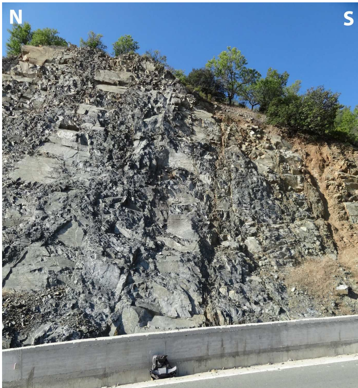
Figure 2.14 : Photographie présentant l'affleurement de métadiabase le moins altéré rencontré lors de notre première mission de terrain. Affleurement localisé sur la route d'Alona-Askas.
