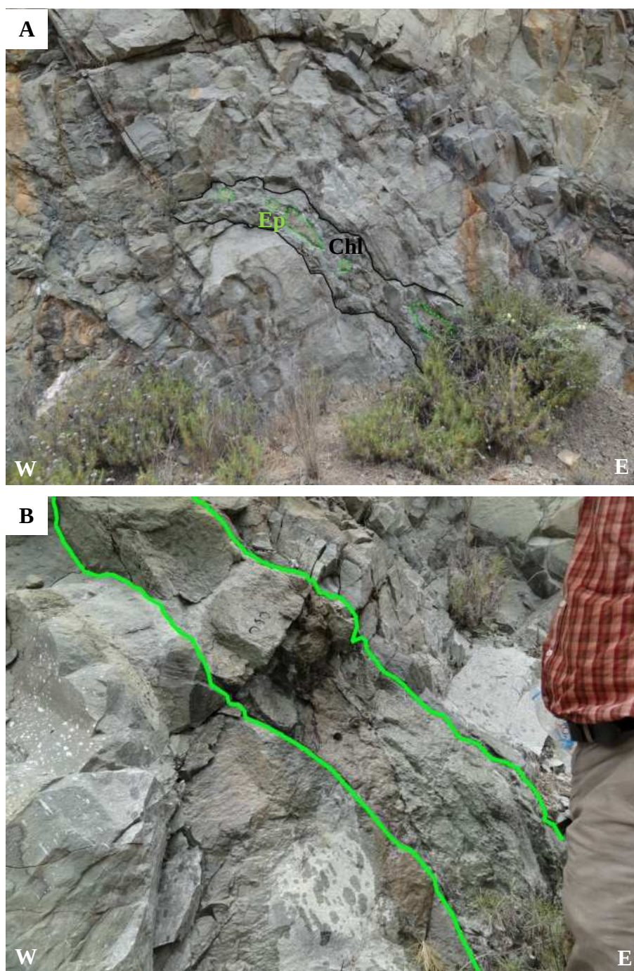
Figure 2.26 : Affleurements présentant des dykes fins à épidosite à sulfures. Affleurements localisés sur la route de Platanistasa-Mitsero. Abréviations : Chl = Chlorite ; Ep = Epidote.
