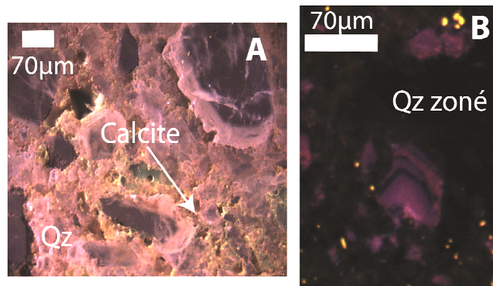
Figure B.2 : Images de cathodoluminescence présentant de la calcite interstitielle dans le quartz cataclaté issu de la fracture à épidote et quartz géodique (éch. 53) (A) et des microcristaux de quartz zonés au niveau de la veine à allanite-sphène remplissant le joint de refroidissement épidotisé (éch. 62) (B) (Mokni-Leconte, 2013). Abréviations : Qz = quartz.
