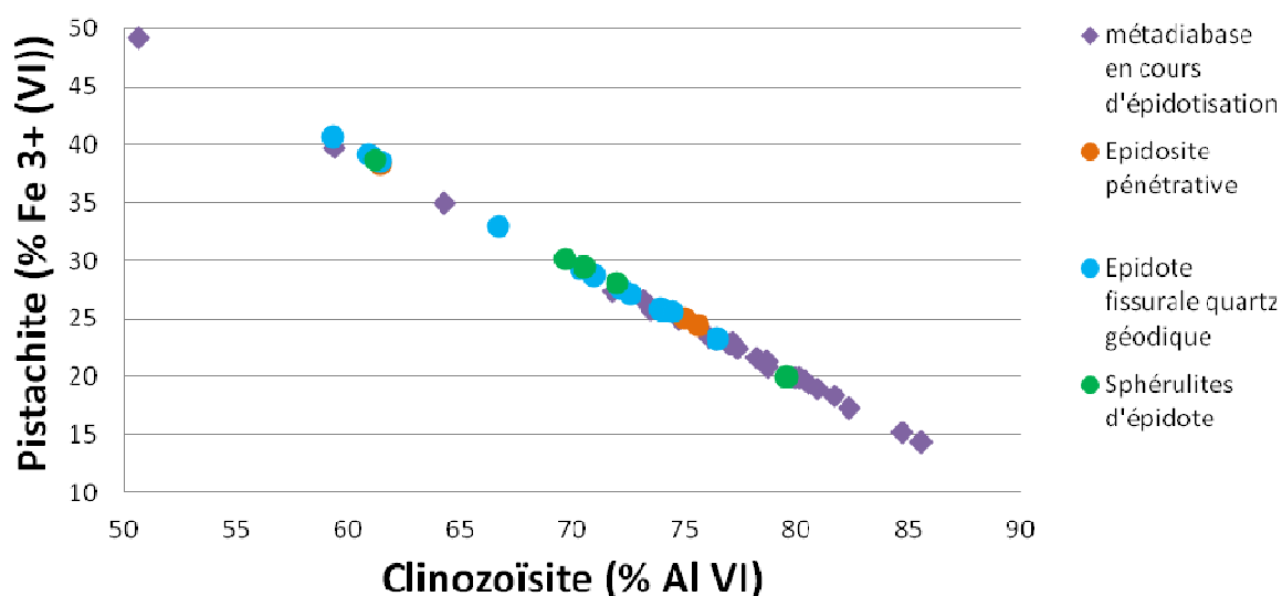
Figure 2.41 : Graphique représentant la distribution de l'ensemble des épidotes analysées suivant les pôles Clinozoïsité (Al) et Pistachite ( Fe^{3+} ) du site VI (Mokni-Leconte, 2013).
