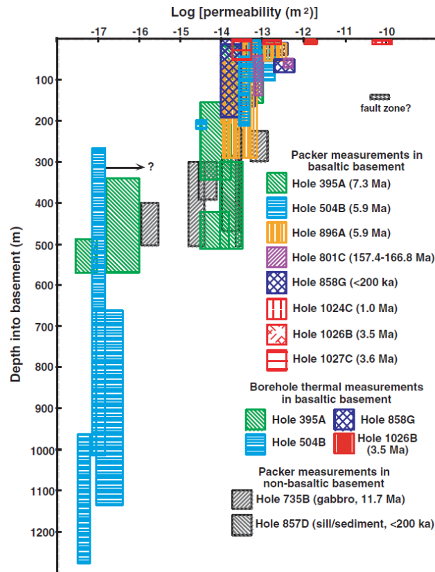
Figure 1.6 : Compilation de mesures in situ de perméabilité dans la croûte océanique actuelle (Fisher, 1998 ; Becker et Fisher, 2000). Diagramme illustré par Fisher (2002).
