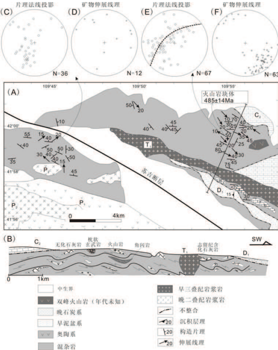
图 3-1-8 红旗牧场地区混杂带地质简图 (A)、剖面 (B)、和构造数据分析 (D-F)
