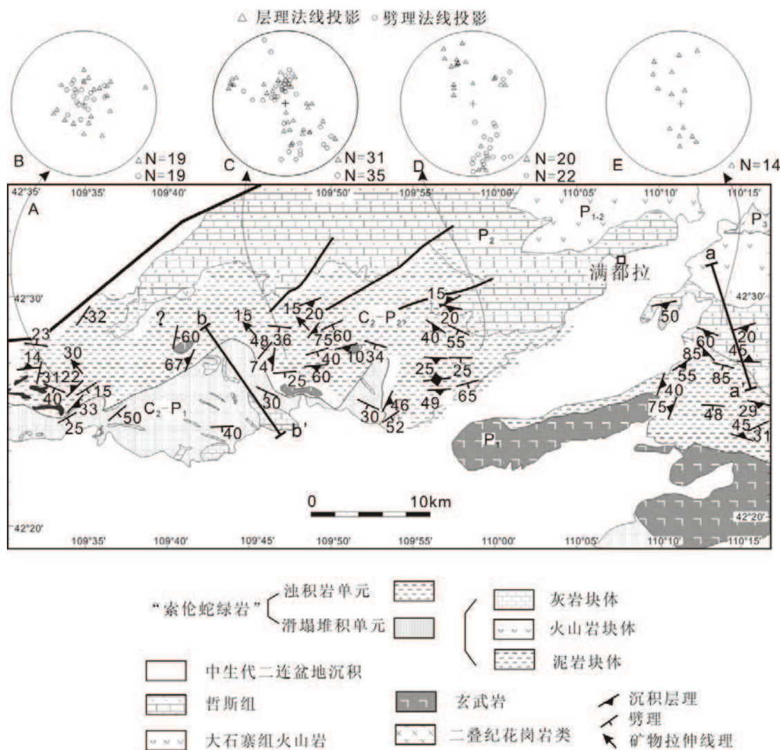
图 4-2-1 满都拉地区构造变形特征简图
