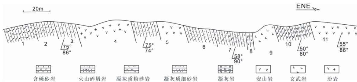
图 3-1-2 格少庙地区布龙山组实测剖面 I
