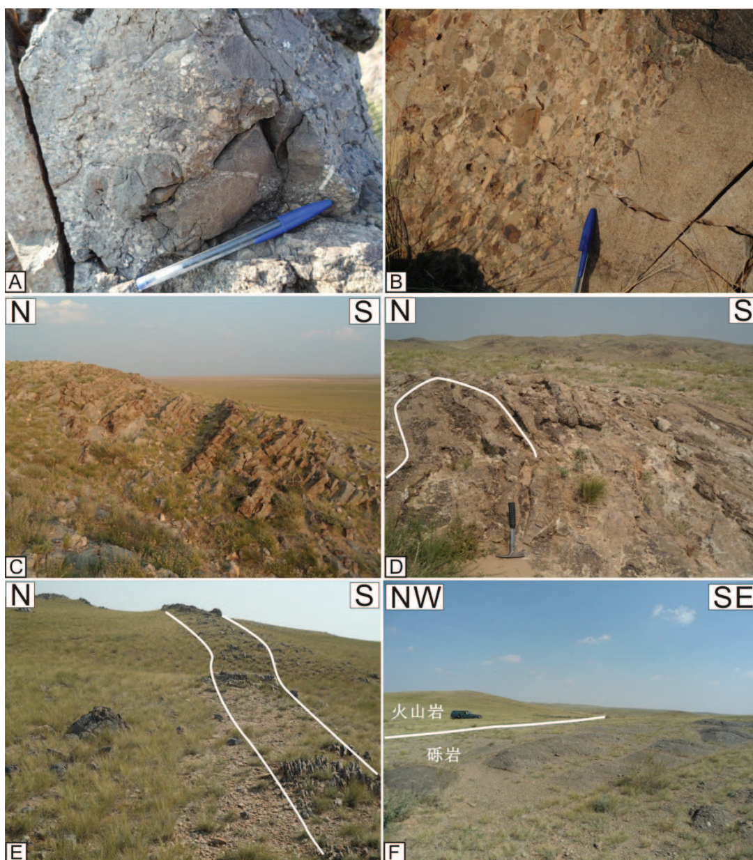
图 4-1-12 满都拉地区哲斯组沉积特征露头图片
