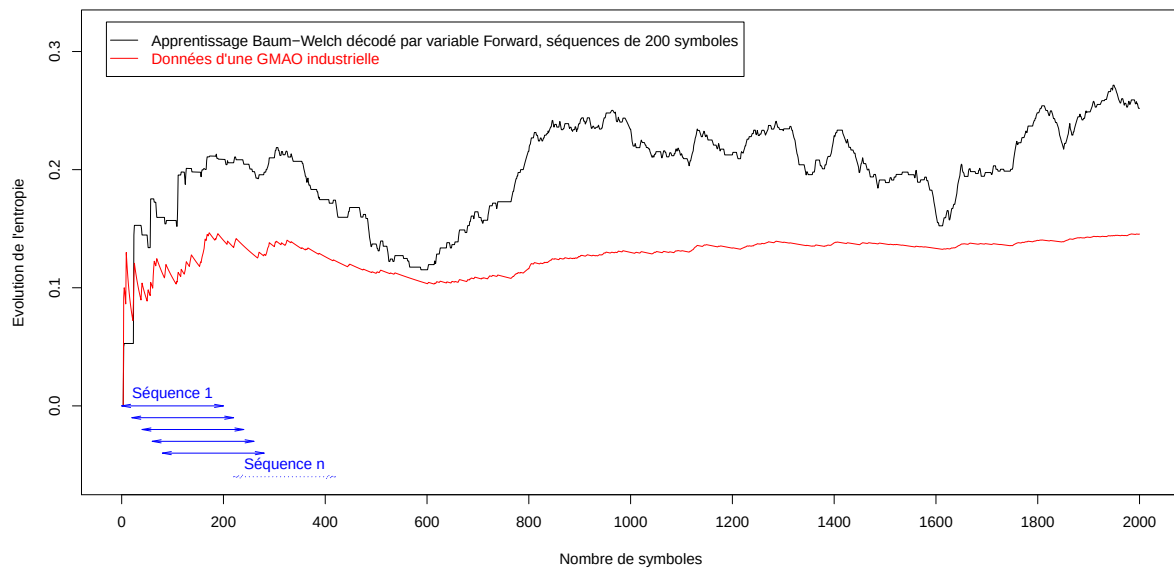
Fig 4.22 – Évolution de l'entropie évaluée avec une fenêtre glissante normée (200 symboles). Les données d'apprentissage sont issues d'une GMAO industrielle.
