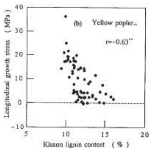
Figure 20. Rapport entre le stress de croissance longitudinal et le contenu de lignines Klason en 3 tronc de tulipier de virginie inclinés (d'après Okuyama et al., 1994).
