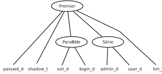
FIGURE 3.4 – L'arbre de décomposition modulaire généré à partir du graphe symétrisé
