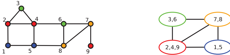
FIGURE 2.1 – Graphe G et le graphe quotient G_{\mathcal{P}}
