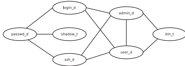
FIGURE 3.3 – Le graphe de flux symétrisé
