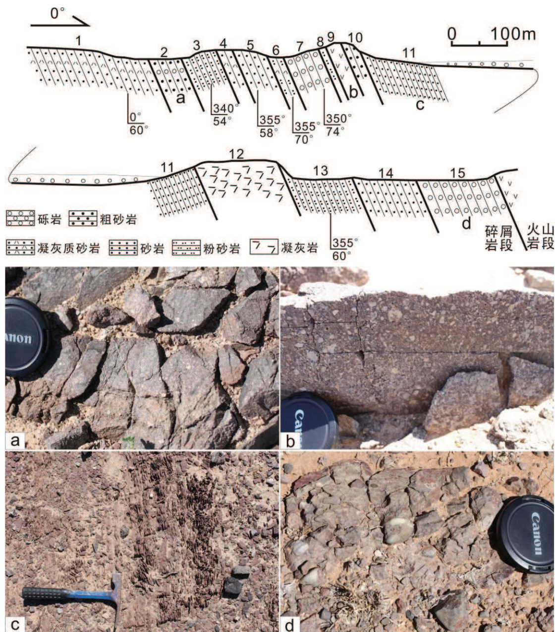
图4-2 查干敖包地区上石炭统一下二叠统宝力高庙组碎屑岩段实测地层剖面: a, 下部含砾粗砂岩; b, 火山角砾岩夹层; c, 红色粉砂岩, 风化为薄片状; d, 上部砾岩
