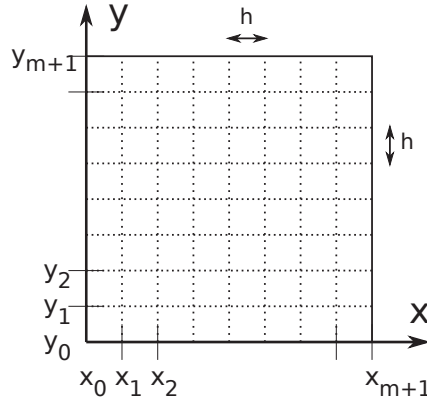
FIGURE 2.4 – Discrétisation régulière de \Omega = \{(x, y) : (x, y) \in [0, 1]^2\} .
