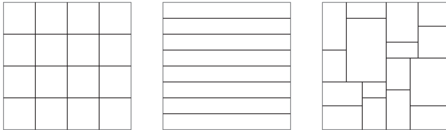
FIGURE 2.10 – De gauche à droite : partitionnement en blocs, en blocs-lignes et bisection récursive orthogonale
