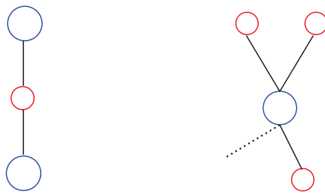
(a) Étape de communication 1, des nœuds rouges vers les nœuds bleus de G' .
