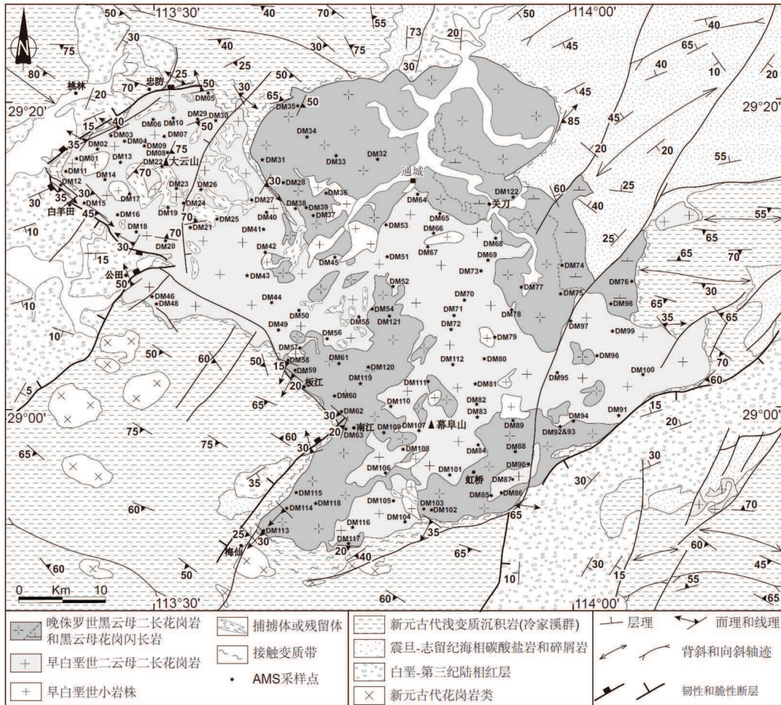
图4-10 大云山-幕阜山岩基磁组构采样位置分布图
