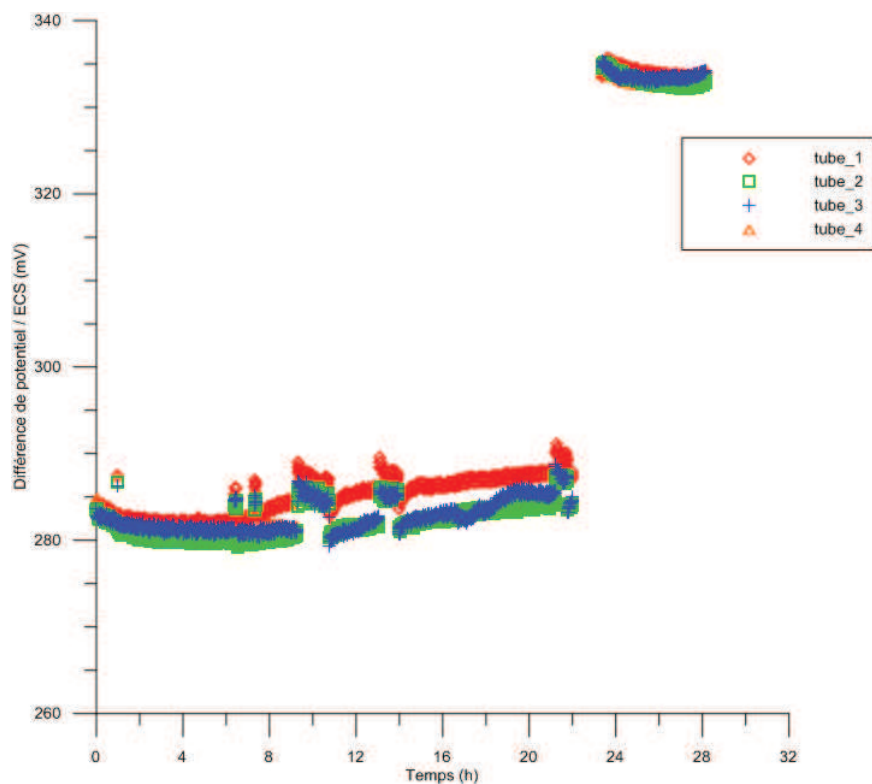
FIGURE 0-5 : EVOLUTION DE LA DIFFÉRENCE DE POTENTIEL DE QUATRE ÉLECTRODES \text{Cu/CuSO}_4 DE TYPE TUBE PAR RAPPORT À UNE ÉLECTRODE DE RÉFÉRENCE ECS, DANS UNE SOLUTION DE KCL, AU COURS DU TEMPS. A 24H, L'ÉLECTRODE DE RÉFÉRENCE A ÉTÉ RÉGÉNÉRÉE CE QUI EXPLIQUE LE « SAUT » DES DDP.
