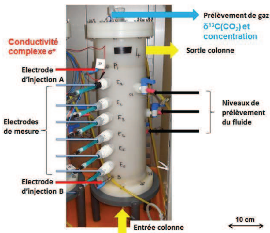
FIGURE V-1 : PHOTO ANNOTÉE D'UNE COLONNE BIOPHY. À GAUCHE, ON RETROUVE L'ÉQUIPEMENT NÉCESSAIRE AUX MESURES DE RÉSISTIVITÉ ÉLECTRIQUE COMPLEXE : DEUX ÉLECTRODES D'INJECTION (A ET B) SONT SITUÉES À CHAQUE EXTRÉMITÉ DE LA COLONNE ; SIX ÉLECTRODES DE POTENTIEL SONT RÉPARTIES SUR LA HAUTEUR DE LA COLONNE. EN HAUT DE LA COLONNE, UN ROBINET PERMET DE PRÉLEVER DU GAZ EN TÊTE DE COLONNE AFIN DE POUVOIR ANALYSER LA QUANTITÉ DE CO 2 AINSI QUE SA SIGNATURE ISOTOPIQUE. SUR LA DROITE, IL Y A TROIS ROBINETS (S1, S2 ET S3) POUR DES PRÉLÈVEMENTS DE FLUIDE EN VUE D'ANALYSES CHIMIQUES ET MICROBIOLOGIQUES COMPLÉMENTAIRES.
