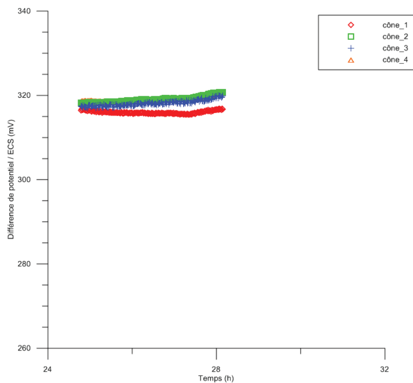
FIGURE 0-4 : EVOLUTION DE LA DIFFÉRENCE DE POTENTIEL DE QUATRE ÉLECTRODES \text{Cu/CuSO}_4 DE TYPE CÔNE PAR RAPPORT À UNE ÉLECTRODE DE RÉFÉRENCE ECS, DANS UNE SOLUTION DE KCL, AU COURS DU TEMPS. UNE FOIS L'ÉLECTRODE DE RÉFÉRENCE RÉGÉNÉRÉE ( T=24\text{H} ), LA DDP DES QUATRE ÉLECTRODES \text{Cu/CuSO}_4 EST STABLE.
