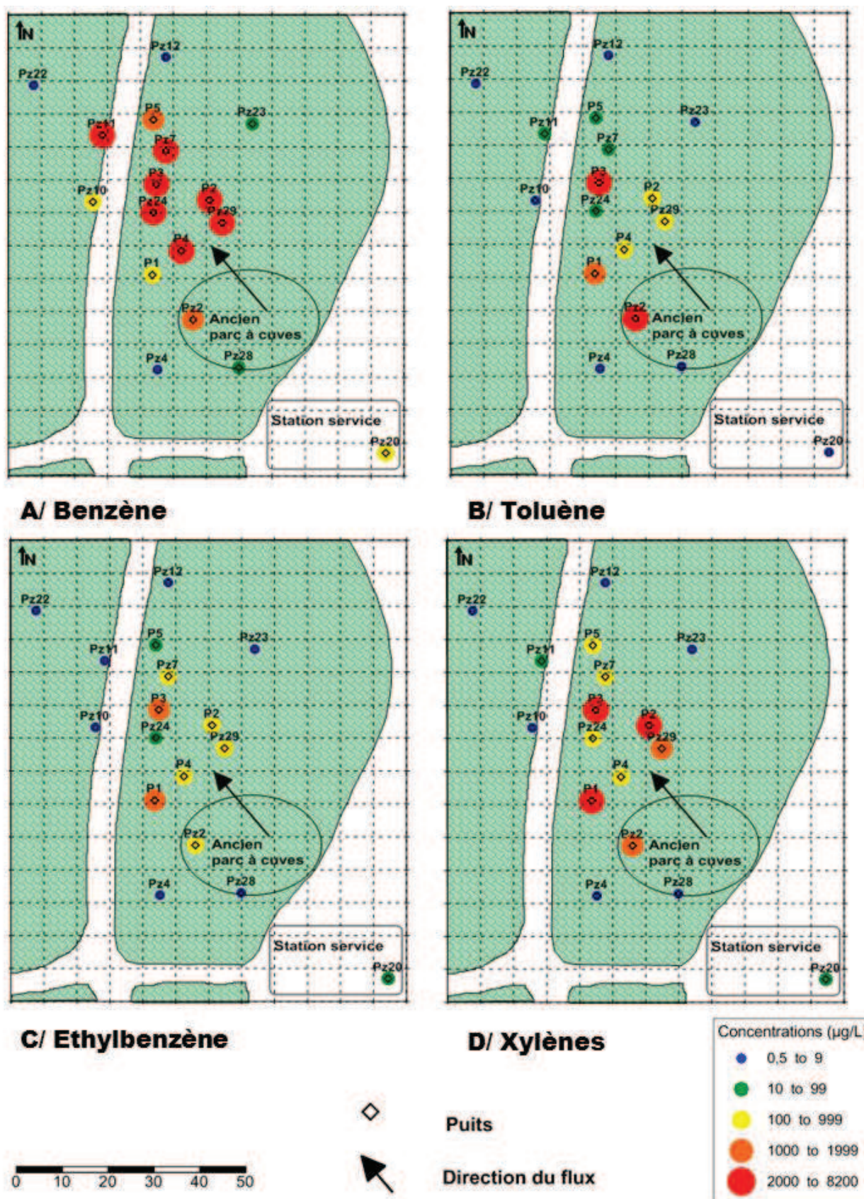
FIGURE VI-2 : CARTES DES CONCENTRATIONS EN BTEX MESURÉES DANS LES PUIITS DE SURVEILLANCE (SEPTEMBRE 2013) : A/ BENZÈNE, B/ TOLUÈNE, C/ ETHYLE-BENZÈNE ET D/ XYLÈNES. L'ANCIEN PARC À CUVES CORRESPOND À LA ZONE SOURCE DE LA POLLUTION, ET LA FLÈCHE INDIQUE LE FLUX DE DIRECTION NORD-OUEST DE LA NAPPE.
