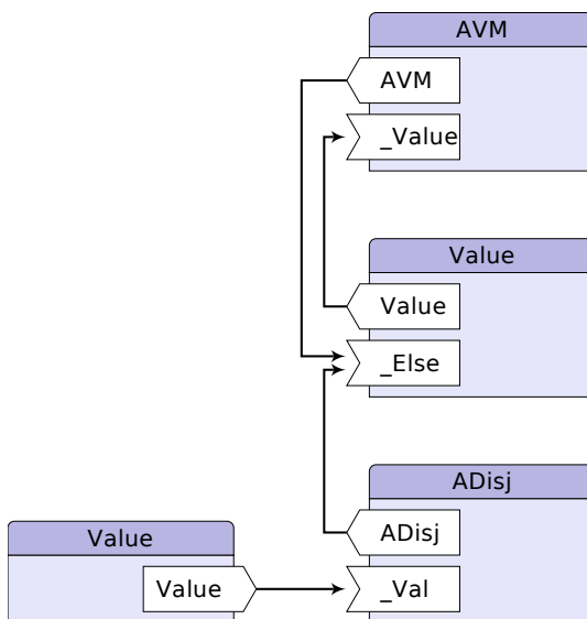
FIGURE 6.6 — Connexion de briques pour des structures récursives
