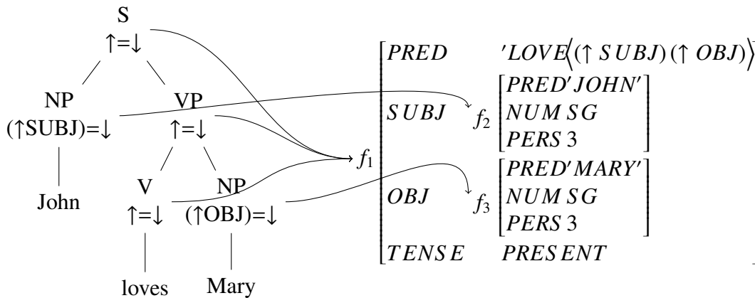
FIGURE 3.3 — Grammaire LFG, c-structure et f-structure pour la phrase "John loves Mary"
