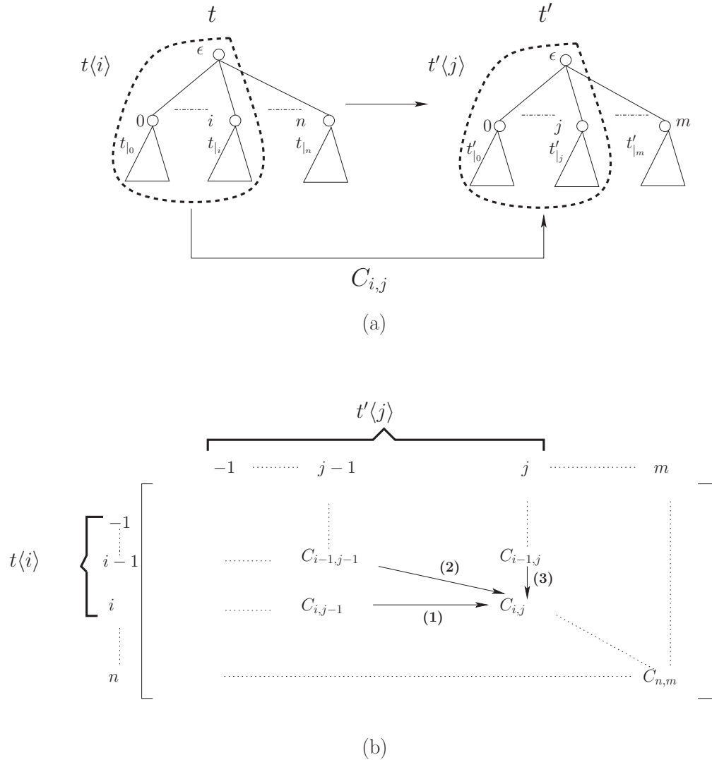
FIGURE 5.6 – (a) Deux arbres partiels t\langle i \rangle et t'\langle j \rangle . (b) Matrice pour la distance d'édition : calcul de la case H[i, j] = C_{i,j} .
