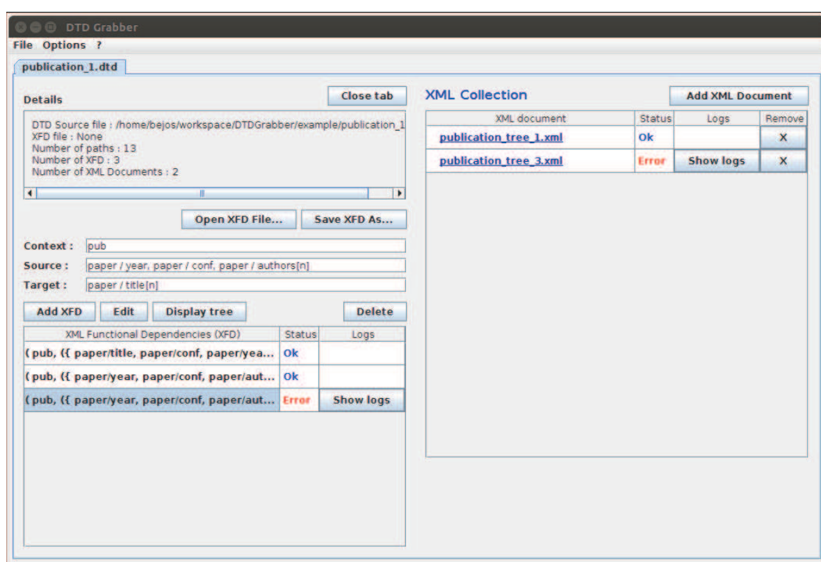
FIGURE 7.5 – Fenêtre principale de DTDGrabber.
