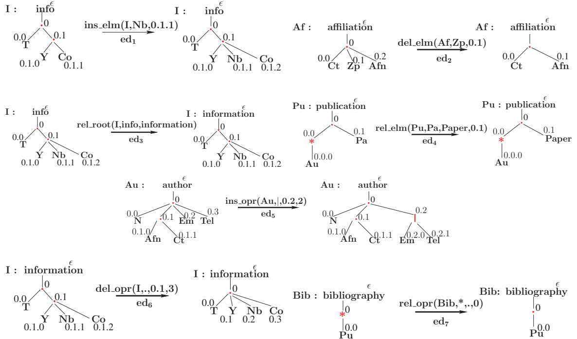
FIGURE 6.3 – Exemple d'opérations d'édition élémentaires sur les grammaires RTG.
