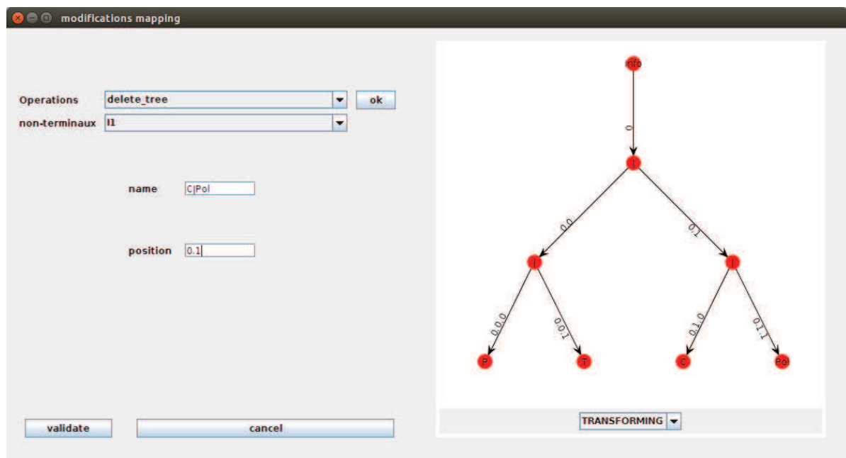
FIGURE 7.8 – Fenêtre de création d’une opération d’édition.
