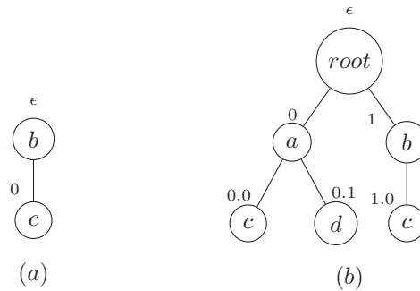
FIGURE 5.2 – (a) Sous-arbre t|_1 et (b) arbre partiel t\langle 1 \rangle de l'arbre t de la Figure 5.1.
