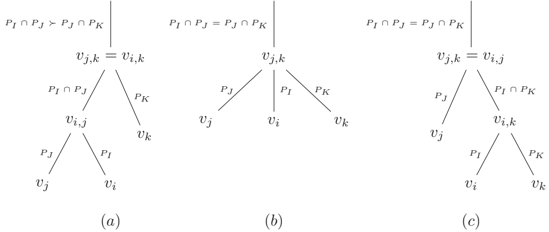
FIGURE A.4 – Trois situations obtenues à partir des conditions du Lemme A.11.
