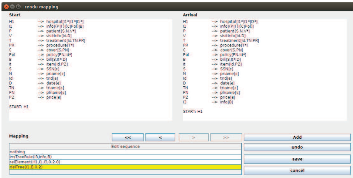
FIGURE 7.7 – Visualisation des modifications apportées par un mapping sur un schéma XML.
