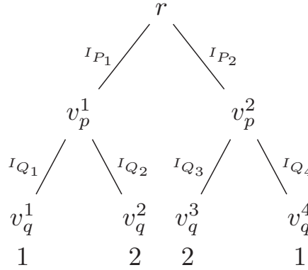
FIGURE A.6 – Un arbre XML montrant l'impossibilité d'avoir toujours deux instances pour tous chemins P et Q tels que P < Q et Last(I_{P_1}) =_V Last(I_{P_2}) et Last(I_{Q_1}) \neq_V Last(I_{Q_2})
