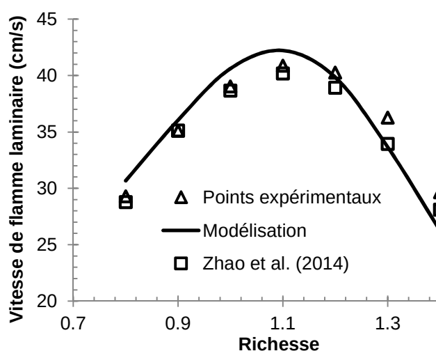
Figure V.23 : Comparaison entre les vitesses de flammes laminaires expérimentales du trans -2-butène obtenues lors de cette étude et par Zhao et al. [Zhao, 2014] (symboles) et la simulation (ligne) pour les conditions : T_i = 300 K ; P = 1 atm.
