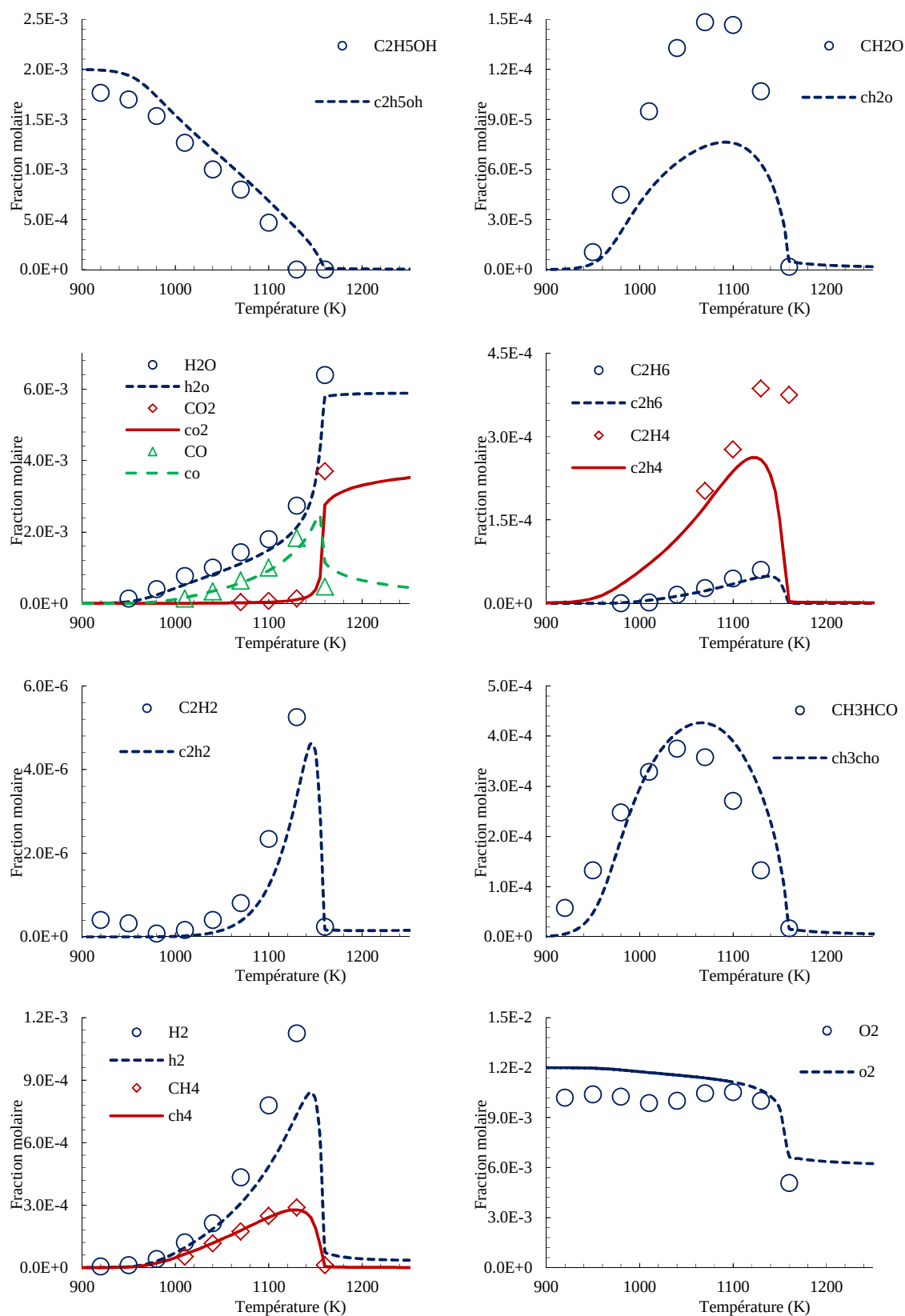
Figure VI.1 : Oxidation de l'éthanol en réacteur auto-agité. \phi = 0,5 ; \tau = 70 ms ; p = 1 atm
