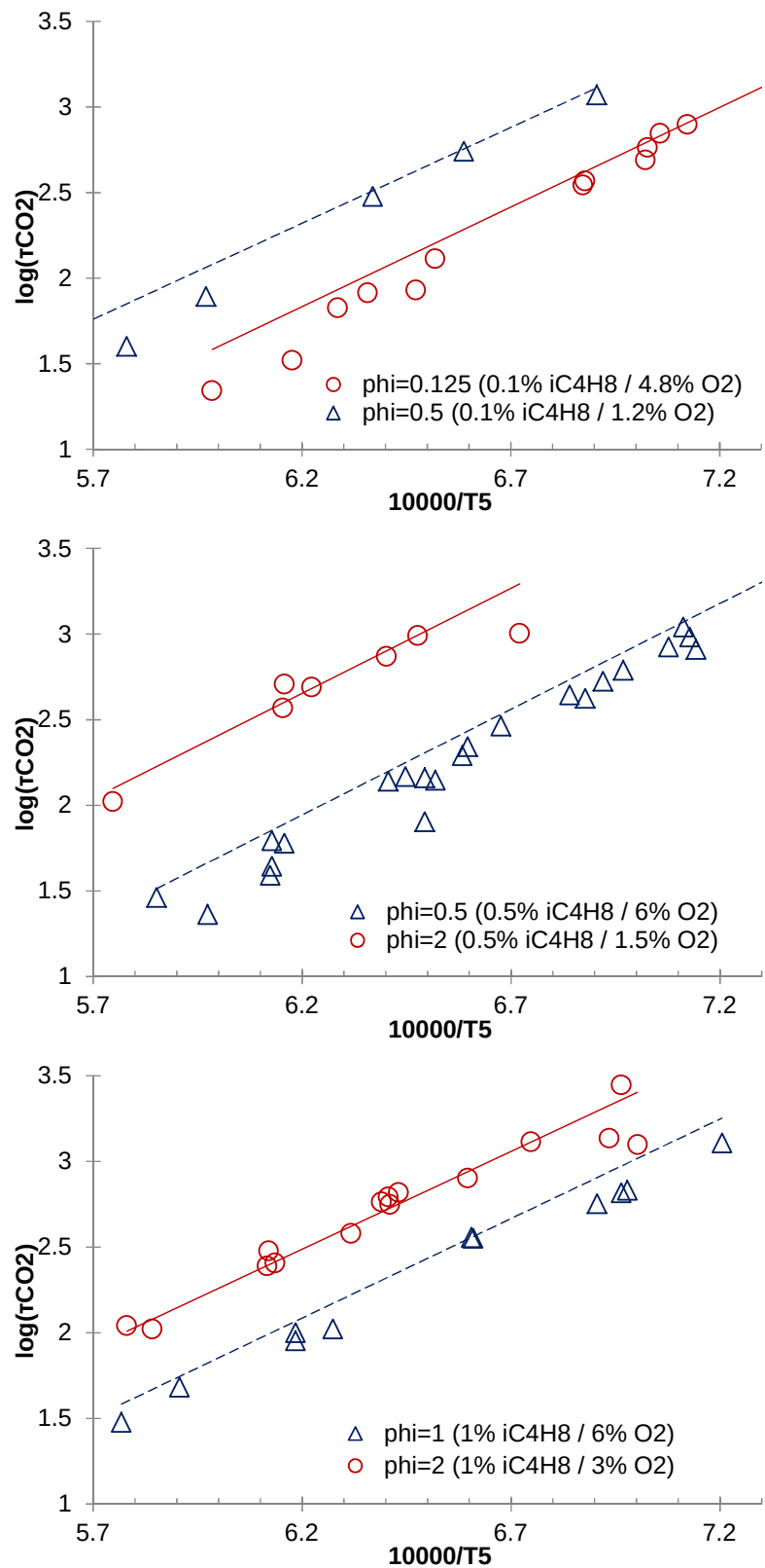
Figure V.47 : Délais d'auto-inflammation de mélanges iC_4H_8/O_2/Ar obtenus en tube à choc – Influence de la richesse.
