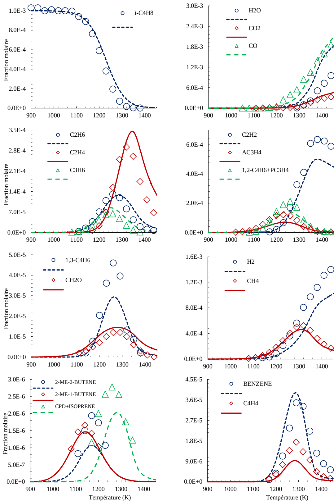
Figure V.39: Confrontation modèle (ligne) et expérience (symboles) pour l'oxydation de l'iso-butène en réacteur auto-agité: p = 1 \text{ atm} ; \phi = 2 ; X_{\text{iso-butène}} = 1000 \text{ ppm} ; \tau = 0,07 \text{ s} .
