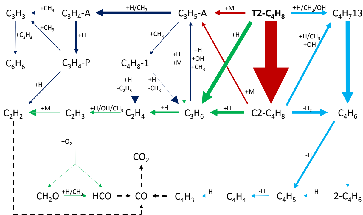
Figure V.21: Analyse de voies réactionnelles pour l'oxydation du trans -2-butène en JSR, \phi = 1 ; \tau = 0,07 s ; P = 1 atm ; T = 1200 K.
