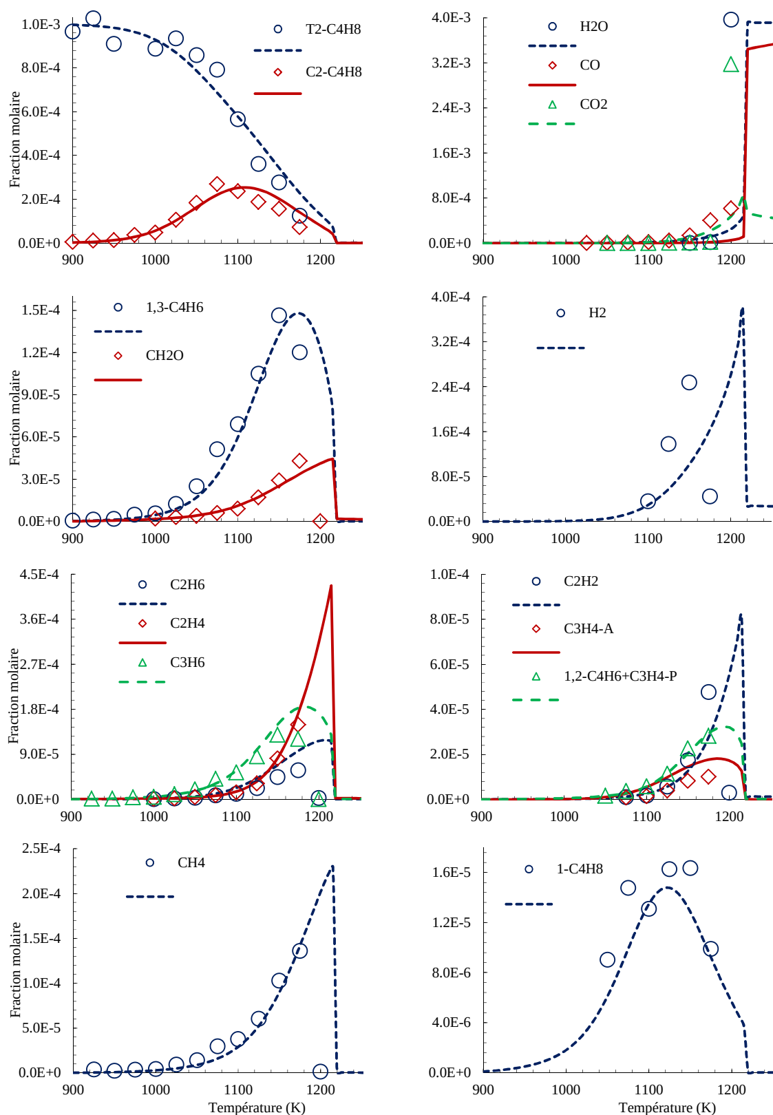
Figure V.18: Confrontation modèle (ligne) et expérience (symboles) pour l'oxydation du trans -2-butène en réacteur auto-agité: P = 1 atm ; \phi = 0,5 ; X_{trans-2-butène} = 1000 ppm ; \tau = 0,07 s.
