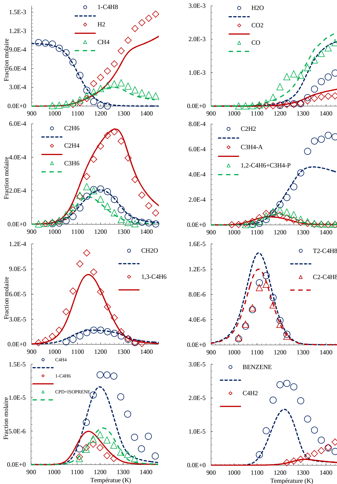
Figure V.6: Confrontation modèle (ligne) et expérience (symboles) pour l'oxydation du 1-butène en réacteur auto-agité: P = 1 atm ; \phi = 2 ; X_{1\text{-butène}} = 1000 ppm ; \tau = 0,07 s.
