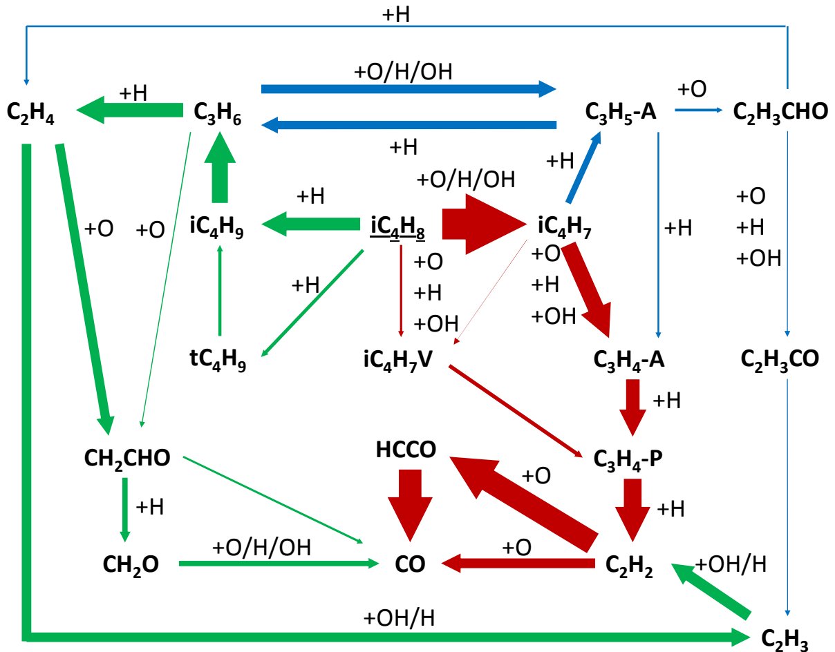
Figure V.40: Analyse de voies réactionnelles pour l'oxydation de l' iso -butène en JSR, \phi = 1 ; \tau = 0,07 s ; p = 1 atm ; T = 1200 K.
