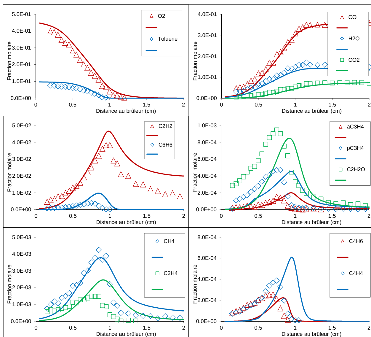
Figure VI.7: Oxidation du toluène en flamme laminaire prémélangée stabilisée sur brûleur. \phi = 1,90 ; p = 30 Torr.
