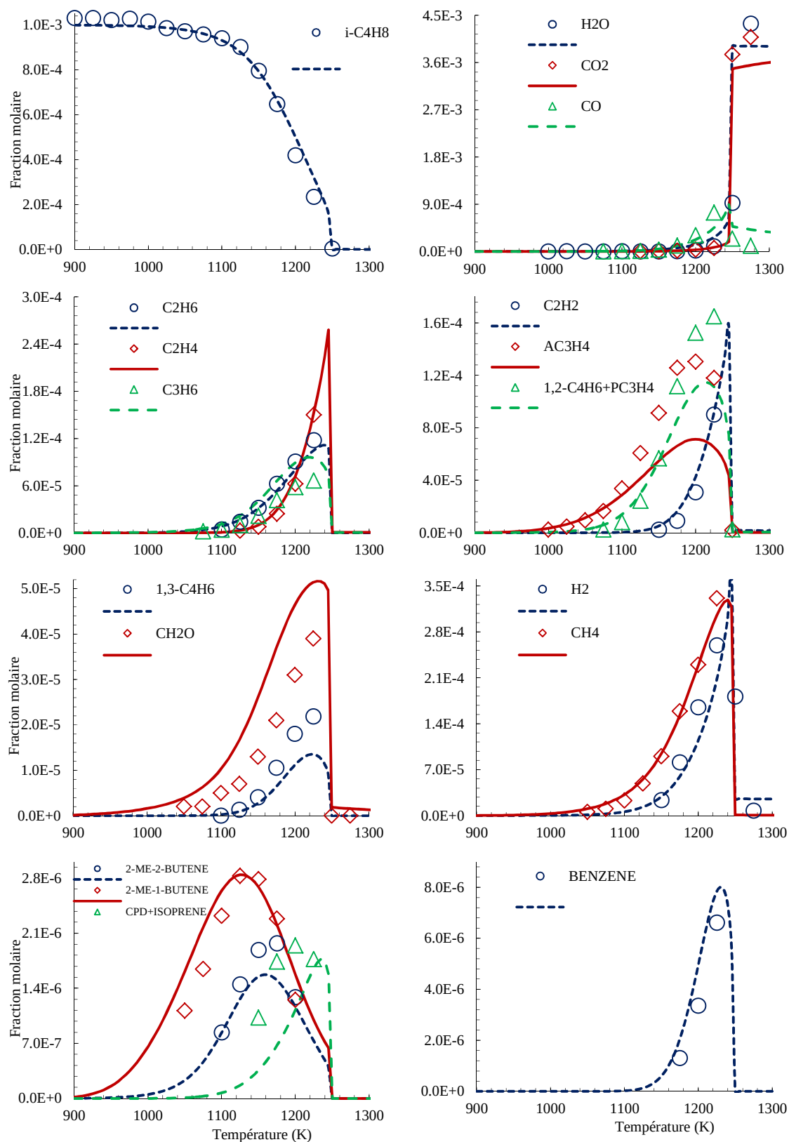
Figure V.37: Confrontation modèle (ligne) et expérience (symboles) pour l'oxydation de l'iso-butène en réacteur auto-agité: p = 1 atm ; \phi = 0,5 ; X_{\text{iso-butène}} = 1000 ppm ; \tau = 0,07 s.
