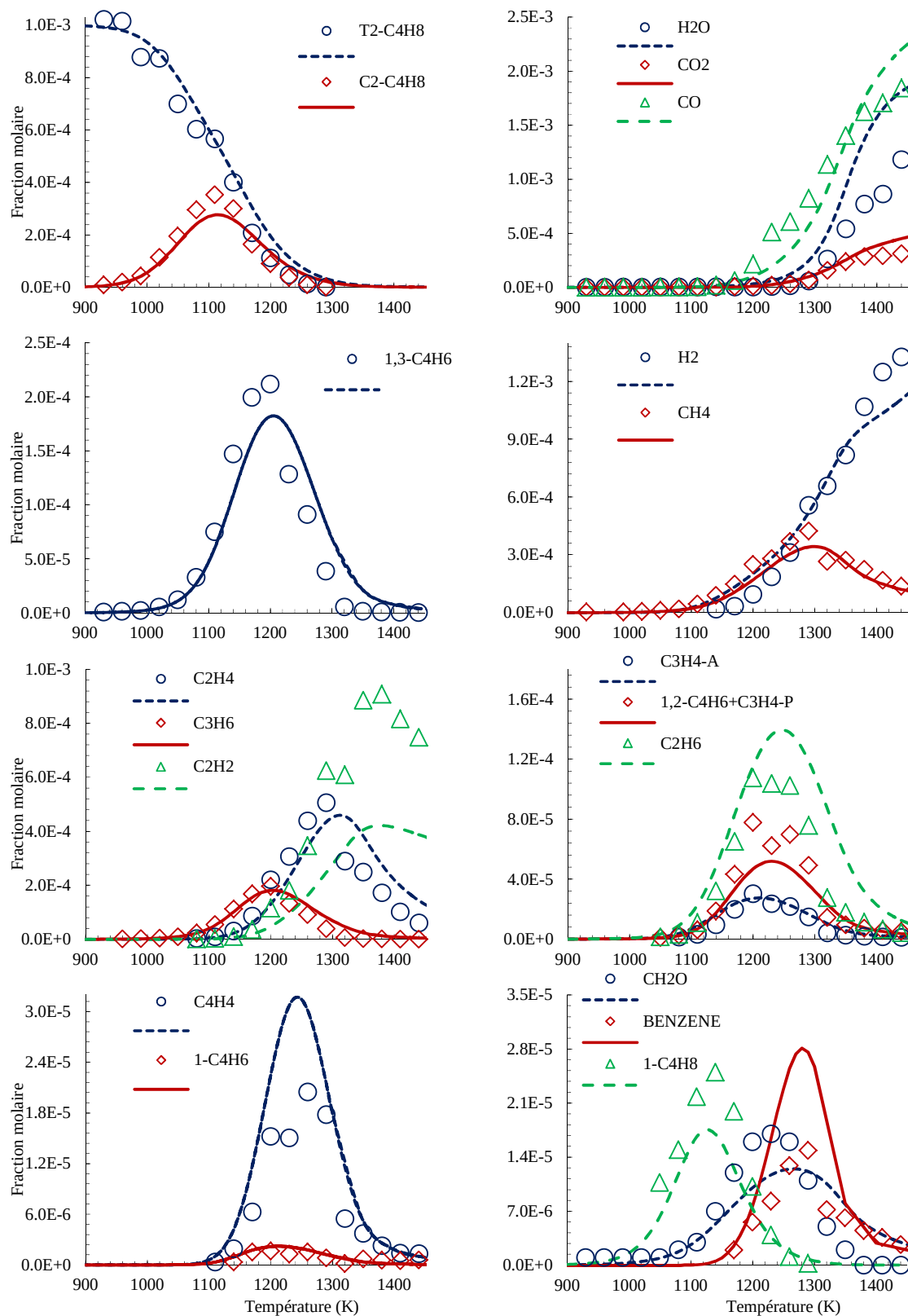
Figure V.20: Confrontation modèle (ligne) et expérience (symboles) pour l'oxydation du trans -2-butène en réacteur auto-agité: P = 1 \text{ atm} ; \phi = 2 ; X_{\text{trans-2-butène}} = 1000 \text{ ppm} ; \tau = 0,07 \text{ s} .
