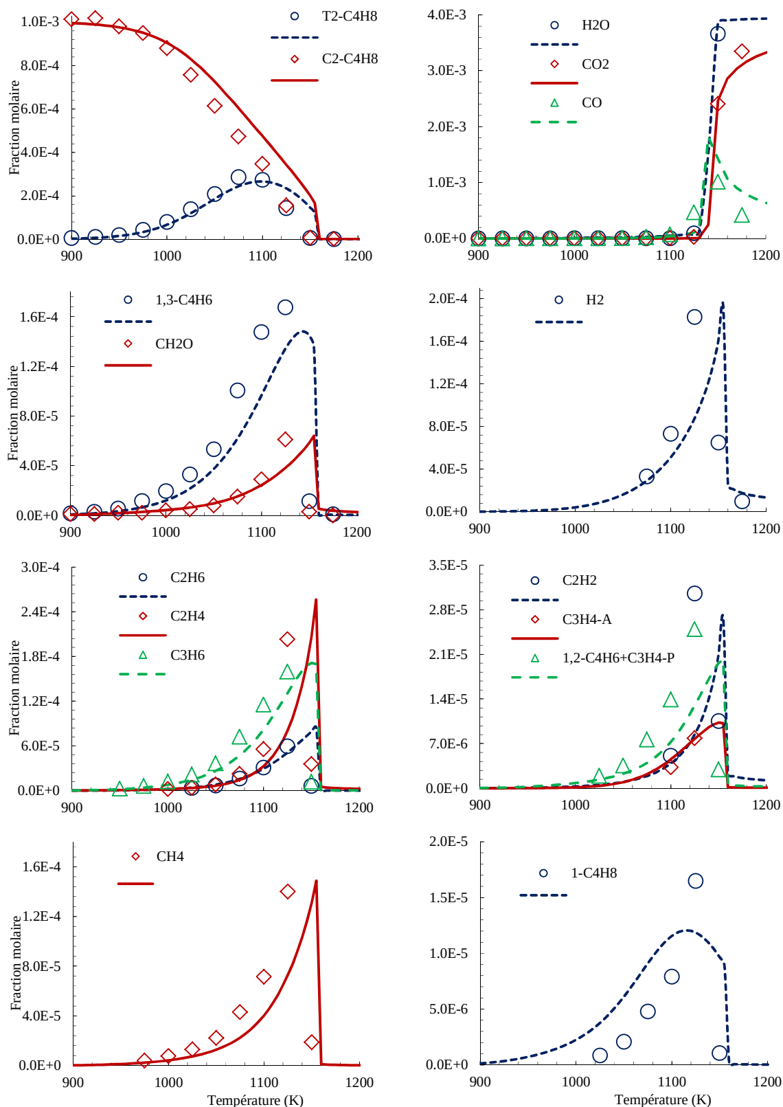
Figure V.27: Confrontation modèle (ligne) et expérience (symboles) pour l'oxydation du cis -2-butène en réacteur auto-agité: p = 1 atm ; \phi = 0,25 ; X_{\text{cis-2-butène}} = 1000 ppm ; \tau = 0,07 s.
