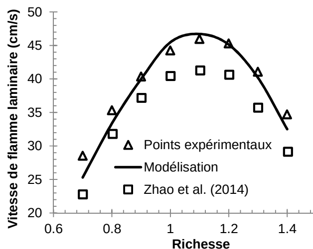
Figure V.9: Comparaison entre les vitesses de flammes laminaires expérimentales du 1-butène obtenues lors de cette étude et par Zhao et al. [Zhao, 2014] (symboles) et la simulation (ligne) pour les conditions : T_i = 300 \text{ K} ; P = 1 \text{ atm} .
