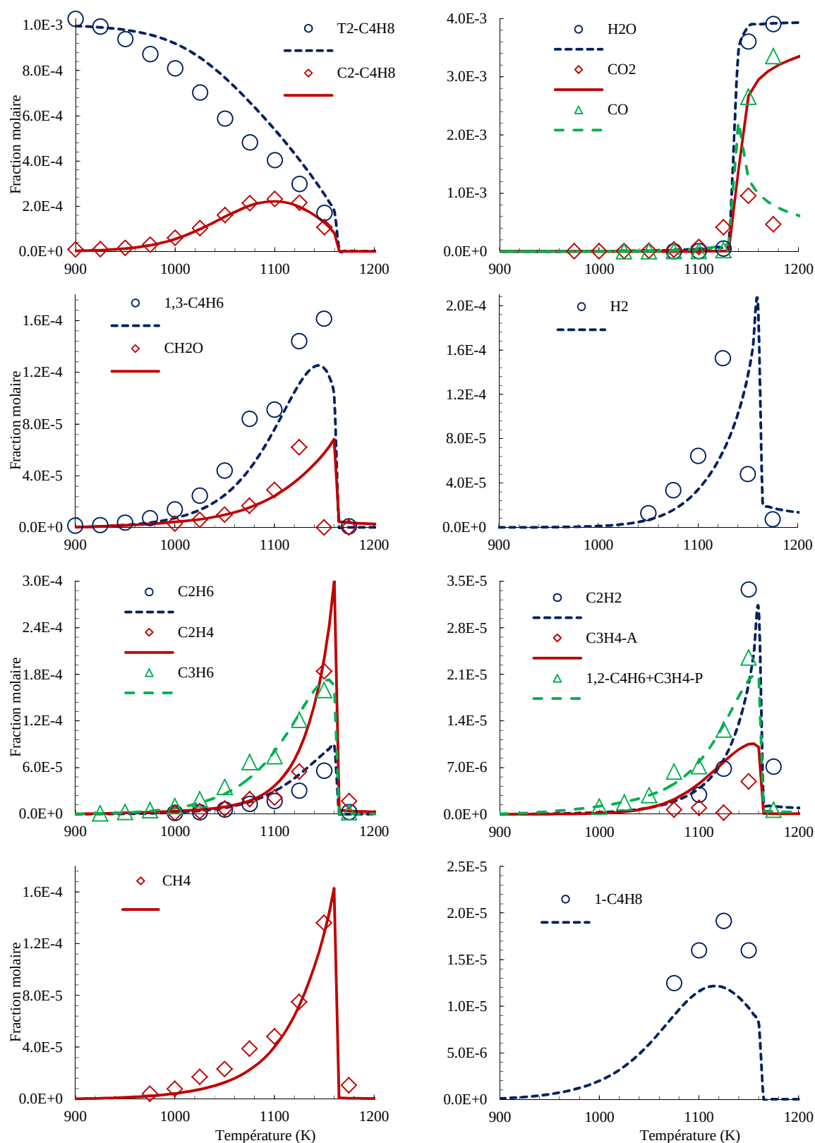
Figure V.17: Confrontation modèle (ligne) et expérience (symboles) pour l'oxydation du trans -2-butène en réacteur auto-agité: P = 1 \text{ atm} ; \phi = 0,25 ; X_{\text{trans-2-butène}} = 1000 \text{ ppm} ; \tau = 0,07 \text{ s} .
