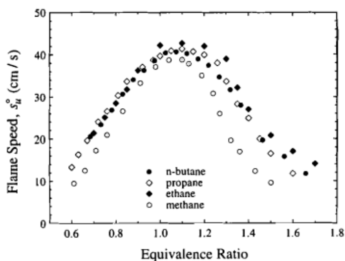
Figure II.13 : Vitesses de flammes laminares mesurées expérimentalement pour des alcanes C_1-C_4 .
