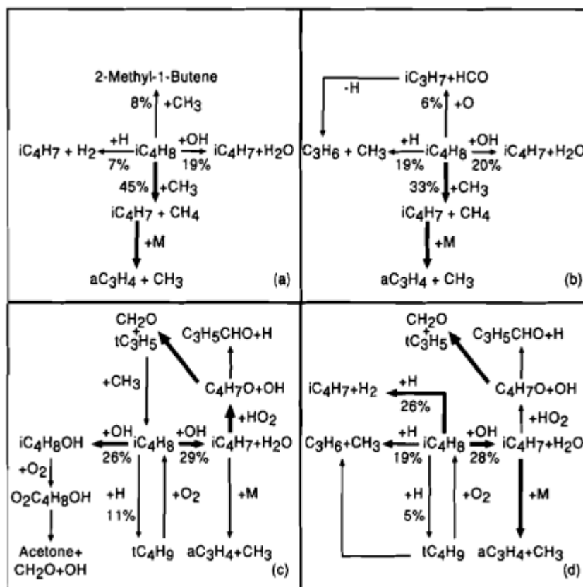
Figure II.8 : Voies réactionnelles primaires pour l'oxydation de l'iso-butène en JSR à pression atmosphérique (a et b : 0,15% iC_4H_8 , \tau = 0,15 s et \phi = 1 ) et 10 atmosphères (c et d : 0,15% iC_4H_8 , \tau = 1,5 s et \phi = 1 ).
