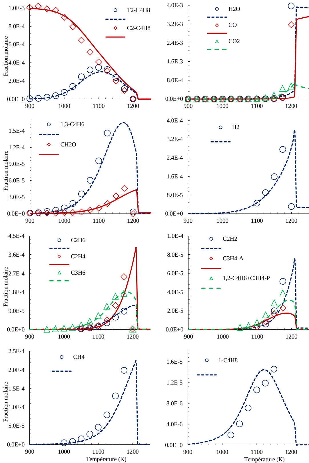
Figure V.28: Confrontation modèle (ligne) et expérience (symboles) pour l'oxydation du cis -2-butène en réacteur auto-agité: p = 1 \text{ atm} ; \phi = 0,5 ; X_{\text{cis-2-butène}} = 1000 \text{ ppm} ; \tau = 0,07 \text{ s} .
