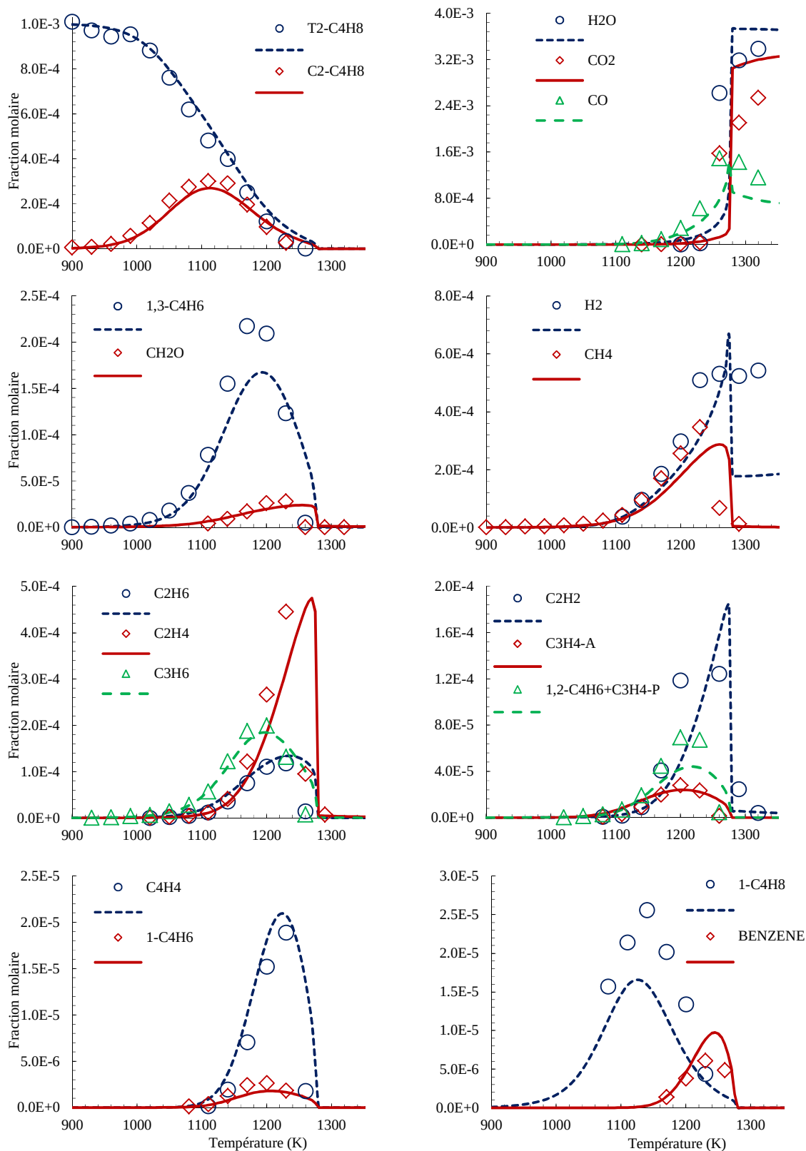
Figure V.19: Confrontation modèle (ligne) et expérience (symboles) pour l'oxydation du trans -2-butène en réacteur auto-agité: P = 1 atm ; \phi = 1 ; X_{\text{trans-2-butène}} = 1000 ppm ; \tau = 0,07 s.
