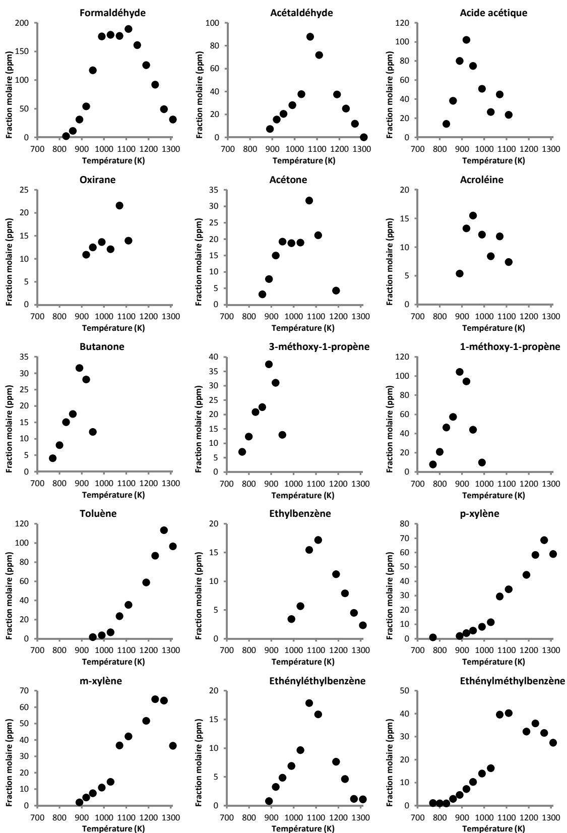
Figure VII.10 : Oxidation du solvant TIFLEX en réacteur auto-agité : p = 1 \text{ atm} ; \tau = 70 \text{ ms} ; X_{\text{TIFLEX}} = 1000 \text{ ppm} ; \phi = 2 . Fractions molaires des produits d'oxydation.
