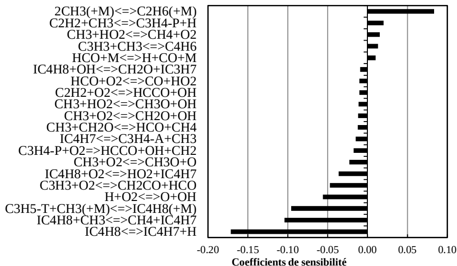
Figure V.41: Analyse de sensibilité sur la concentration d'iso-butène lors de l'oxydation de l'iso-butène en réacteur auto-agité (p = 1 atm ; T = 1200K ; \phi = 1)
