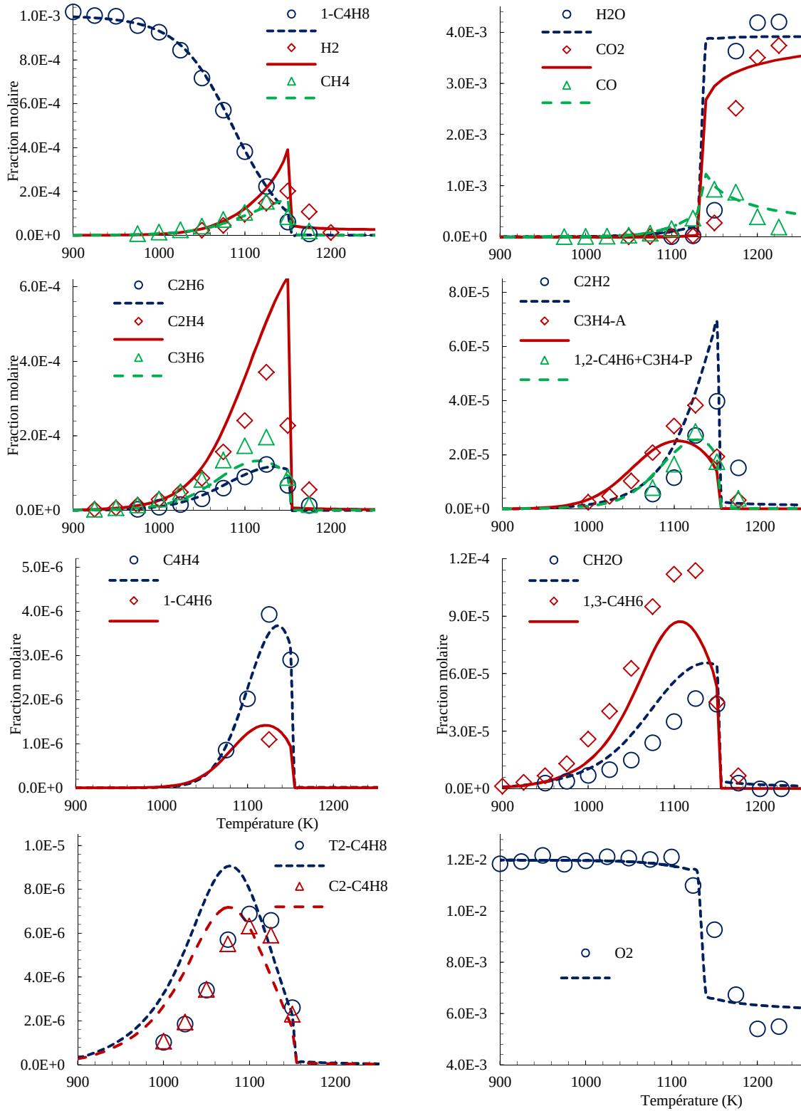
Figure V.4: Confrontation modèle (ligne) et expérience (symboles) pour l'oxydation du 1-butène en réacteur auto-agité; P = 1 \text{ atm} ; \phi = 0,5 ; X_{1\text{-butène}} = 1000 \text{ ppm} ; \tau = 0,07 \text{ s} .
