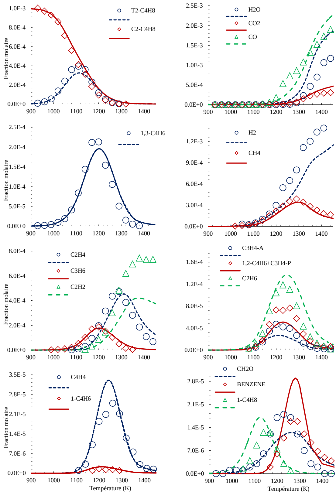
Figure V.30: Confrontation modèle (ligne) et expérience (symboles) pour l'oxydation du cis -2-butène en réacteur auto-agité: p = 1 \text{ atm} ; \varphi = 2 ; X_{\text{cis-2-butène}} = 1000 \text{ ppm} ; \tau = 0,07 \text{ s} .
