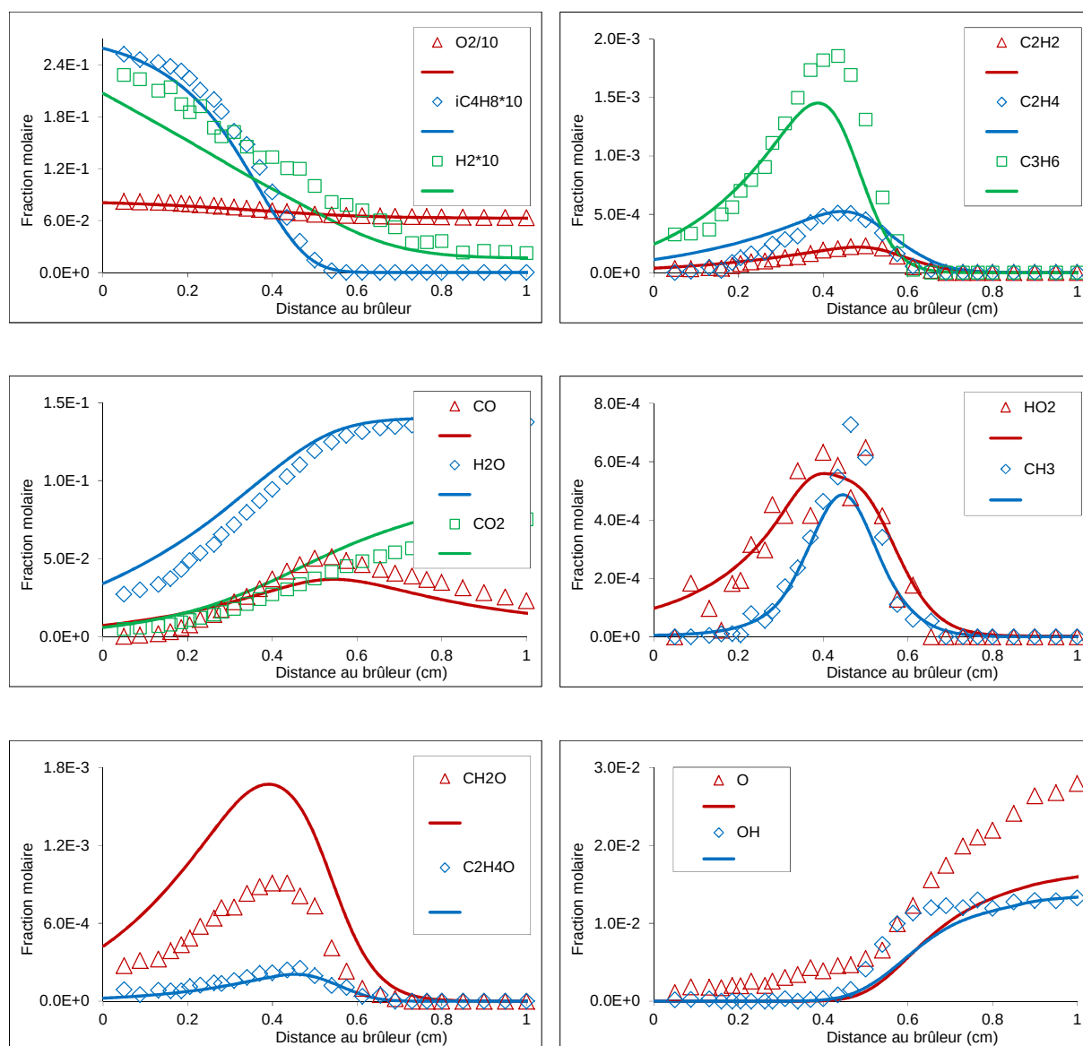
Figure V.46 : Profils de concentration expérimentaux (symboles) et simulés (lignes) obtenus lors de l'oxydation de l' iso -butène en flamme plate (2,7 %mol i-C_4H_8 ; 4,5 %mol H_2 ; 83,0 %mol O_2 ; 9,8 %mol Ar) à basse pression (40 mbar).
