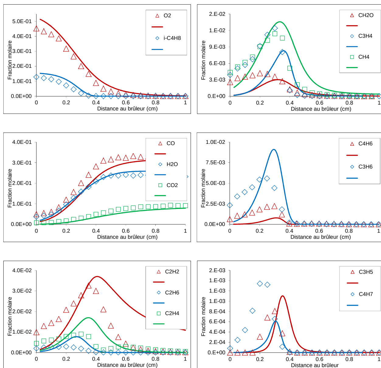
Figure V.44 : Profils de concentration expérimentaux (symboles) et simulés (lignes) obtenus lors de l'oxydation de l'iso-butène en flamme plate (16.5% mol i\text{-C}_4\text{H}_8 / 58.5% mol \text{O}_2 /25% mol Ar) à basse pression (40 mbar).
