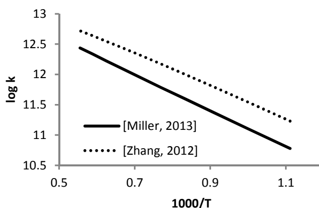
Figure IV.4 : Comparaison graphique des valeurs des constantes de vitesse k en fonction de 1000 K/T pour la réaction 50.
