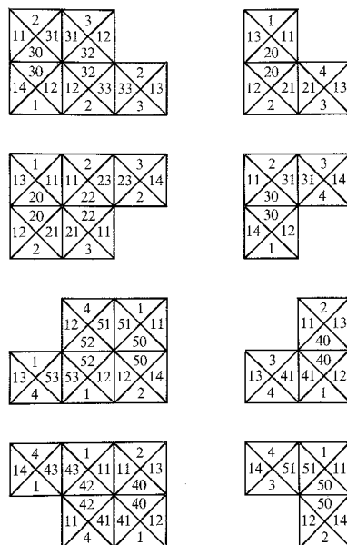
FIGURE 1.27 – 24 tuiles de Wang apériodiques obtenues à partir de A2, extrait de [GS87]
