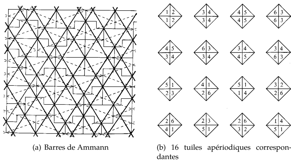
FIGURE 1.28 – 16 tuiles de Wang apériodiques obtenues à partir de A2 [GS87]
