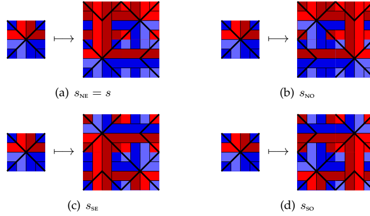
FIGURE 3.7 – Les quatre substitutions symétriques
