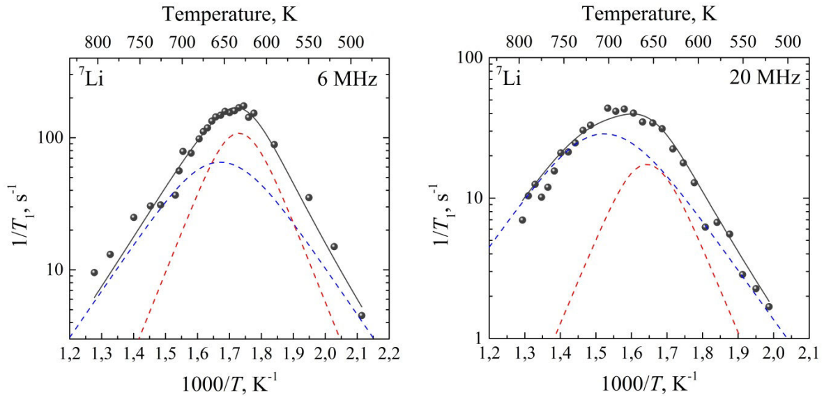
Fig. ii. Dépendance en température des temps de relaxation spin-réseau de ^7\text{Li} dans \text{LiNaSO}_4 à deux champs différents \nu(^7\text{Li}) = 6 \text{ MHz} (à gauche) et 20 \text{ MHz} (à droite) [11]. Les contributions BPP sont reportées en pointillés rouges ( ^7\text{Li} ) et bleus ( ^{23}\text{Na} ), respectivement. Les énergies d'activation sont estimées à E_a^{\text{Li}} = 0.7 \text{ eV} and E_a^{\text{Na}} = 1.2 \text{ eV} .
