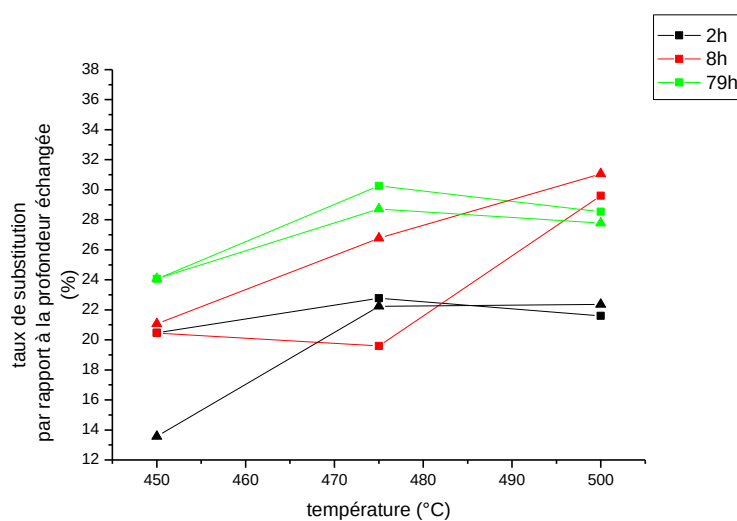
Figure 6-23 Comparaison des taux de substitution pour les verres commerciaux pour les différents temps de trempe
