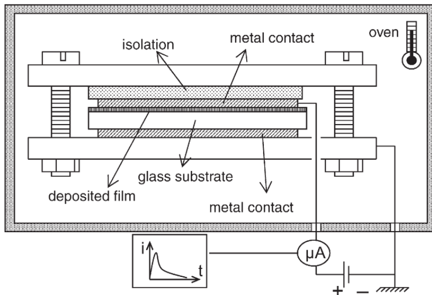
Figure 2-6 Représentation schématique du procédé de poling thermique (70)
