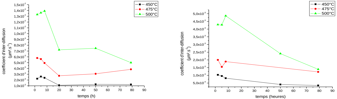
Figure 6-8 Influence du temps sur les coefficients d'interdiffusion pour la lame de microscope (à gauche) et le verre Planilux (à droite)
