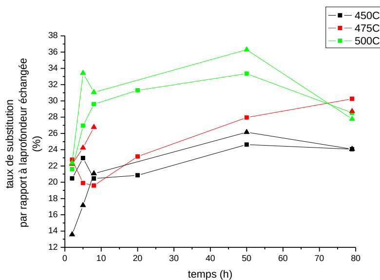
Figure 6-22 Comparaison des taux de substitution pour les verres commerciaux pour les 3 températures de trempe
