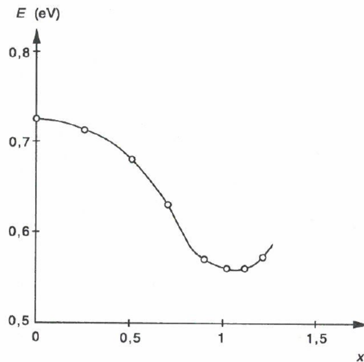
Figure 2-12 Représentation de l'énergie d'activation de la conductivité électrique des verres \text{Na}_2\text{O}; (4 - 2x)\text{SiO}_2; x\text{Al}_2\text{O}_3
