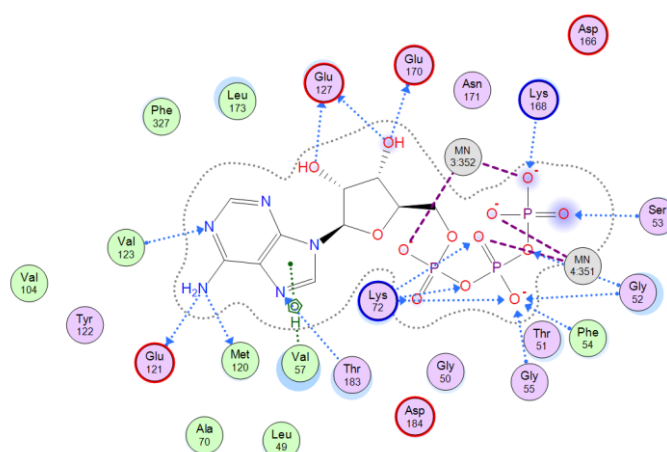
Figure 16 : Schéma représentant les interactions entre l'ATP et les résidus du domaine catalytique de PrcAa (code PDB : 1ATP). L'adénine, entourée de résidus hydrophobes, est maintenue en place par des liaisons hydrogène (tirets bleu clair). Les phosphates réalisent de nombreuses interactions non covalentes avec des résidus du site actif et les ions présents.
