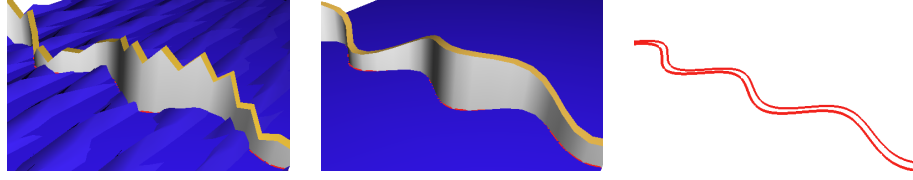
FIGURE 1.1.2 – Graphe de g et décomposition (u, K)
