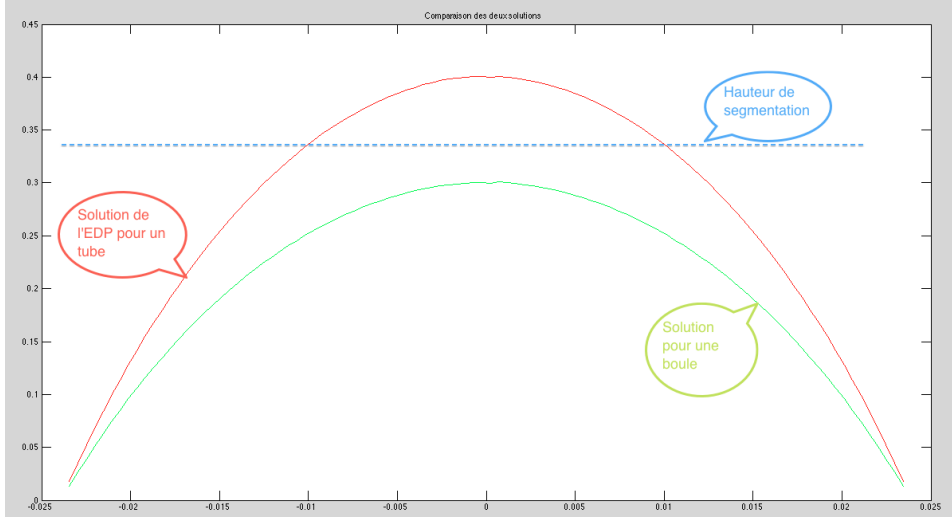
FIGURE 4.1.3 – Seuillage adapté à la segmentation
