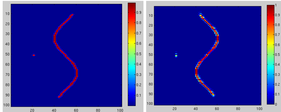
FIGURE 4.4.5 – Diffusion isotrope et anisotrope
