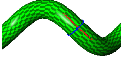
FIGURE 4.2.2 – Les deux lignes de courbure principales
