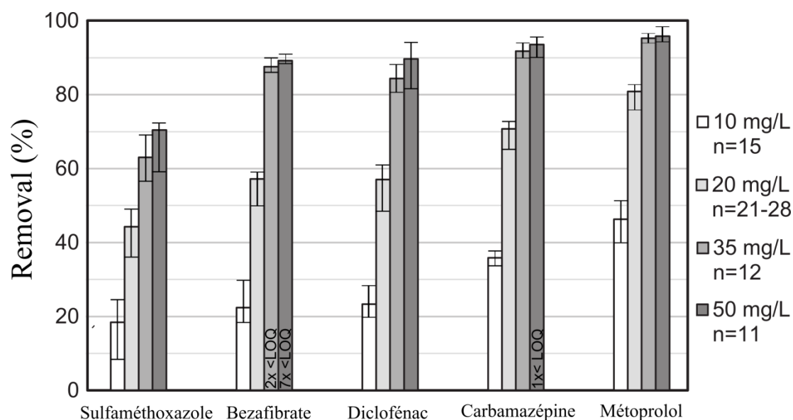
Figure I-7 : Épuration de produits pharmaceutiques par un système de filtration tertiaire aux charbons actifs : effet de la concentration en charbons actifs, les barres d'erreur représentent les premiers et troisièmes quartiles pour chaque série de données tandis que les barres verticales correspondent aux valeurs médianes, adapté de Altmann et al. (2015)
