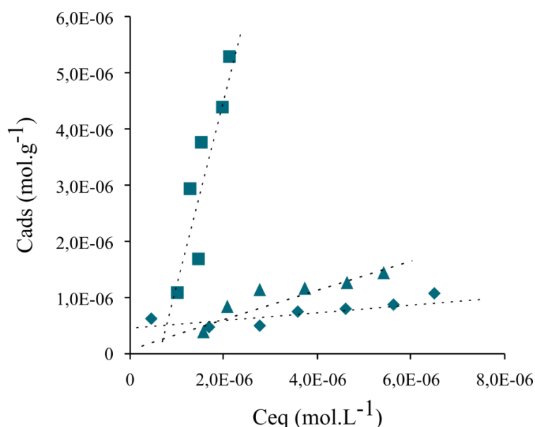
Figure IV-2 Concentration adsorbée en fonction de la concentration à l'équilibre pour le kétoprofène (Triangles), la carbamazépine (Carrés) et le naproxène (Losanges) sur la kaolinite
