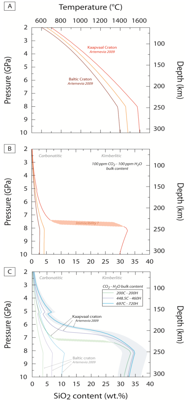
Figure VI-5 : Evolution de (B,C) la teneur en SiO 2 des liquides magmatiques au niveau des cratons comme une fonction (A) des conditions pression – température définies pour le géotherme du craton de Kaapvaal et celui du craton Baltique, et en considérant également un géotherme intermédiaire (seulement pour (B)). (B) La teneur en CO 2 et H 2 O du bulk est fixé à 100 ppm. (C) La teneur en CO 2 et H 2 O du bulk est variable : 200 ppm CO 2 – 200 ppm H 2 O, 448.5 ppm CO 2 – 460 ppm H 2 O, et 697 ppm CO 2 – 720 ppm H 2 O.
