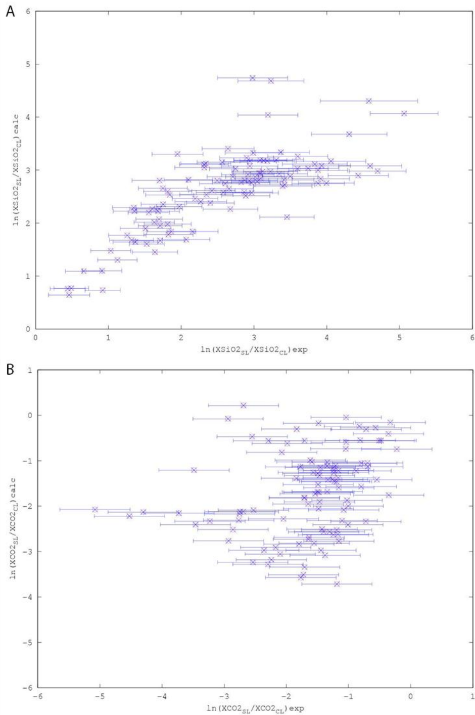
Figure V-10 : Comparaison de (A) \ln(X_{SiO_2(l)}^{SL}/X_{SiO_2(l)}^{CL}) (i.e. \ln(\gamma_{SiO_2(l)}^{CL}/\gamma_{SiO_2(l)}^{SL}) ) et (B) \ln(X_{CO_2(l)}^{SL}/X_{CO_2(l)}^{CL}) (i.e. \ln(\gamma_{CO_2(l)}^{CL}/\gamma_{CO_2(l)}^{SL}) ) calculés avec THERMantle à ceux mesurés dans les expériences d'immiscibilité. Les incertitudes sont reportées sur les valeurs mesurées, et sont définies dans la section V.3.4. (étape 10).
