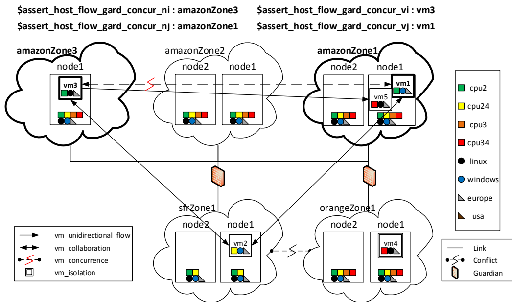
FIGURE 5.10 – Exemple : contre-exemple Alloy prouve la non-satisfiabilité de la propriété de concurrence.
