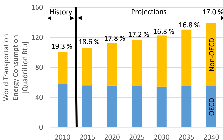
Figure 3. Historique et prévisions de la consommation en énergie des transports entre 2010 et 2040 réparti entre les pays membres de l'OCDE et les pays non membres. Les pourcentages en haut de chaque histogramme représentent la part des transports en référence à la demande énergétique mondiale[1]
