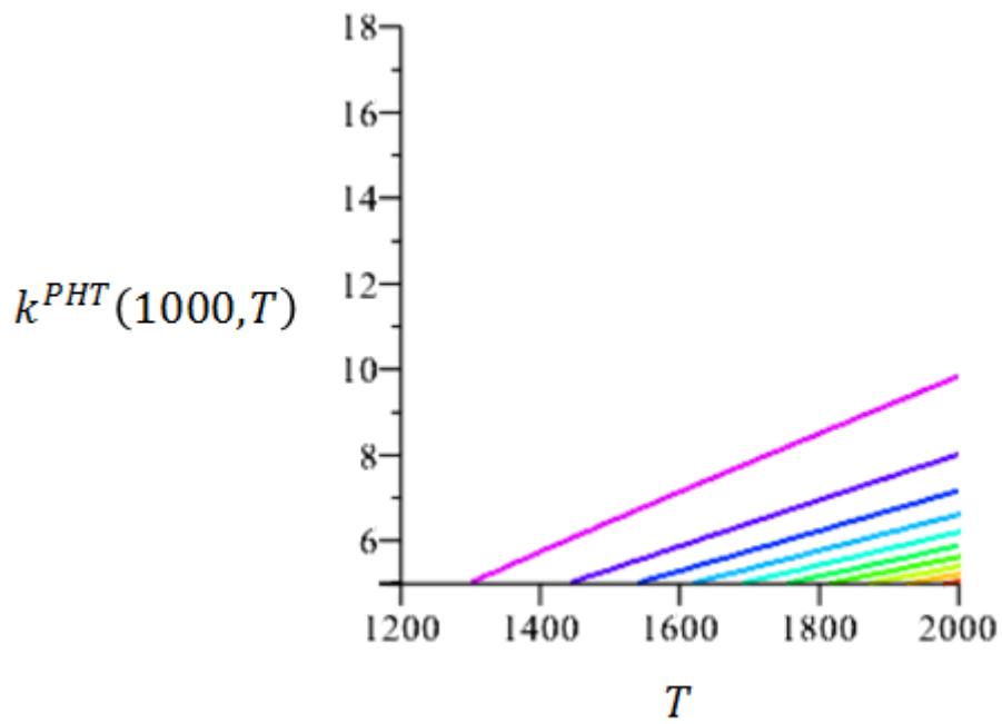
Figure 142 : Evolution de k^{PHT}(1000, T) pour T \in [1200; 2000] , c'est-à-dire pour un rapport signal sur bruit compris entre 5 et 1. Les différentes courbes correspondent à différentes valeurs de \varepsilon . En particulier, la courbe violette correspond à \varepsilon = 0,05 , c'est-à-dire à la valeur de k^{PHT} nécessaire pour avoir 95 % de chances de détecter la droite.
