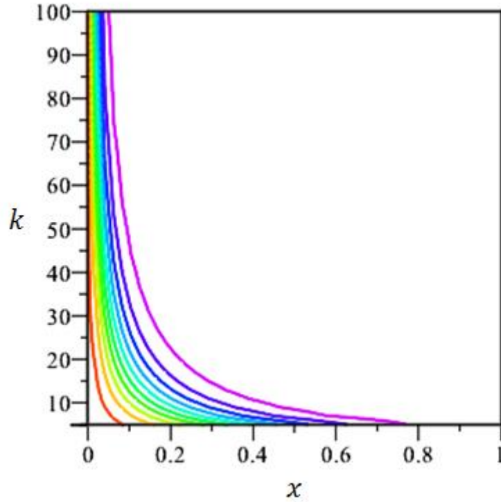
Figure 141 : Graphe des lignes de niveau l(\mathcal{F}, \varepsilon) , le violet correspondant aux petites valeurs de \varepsilon vers les grandes valeurs en rouge. On constatera le comportement décroissant en x des lignes de niveau.
