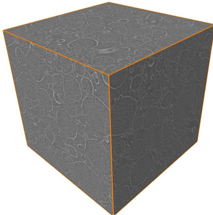
Figure 62 : Image tomographique d'une mousse de silice. Image de taille 700^3 , avec une résolution de 5\text{ }\mu\text{m/vx} .
